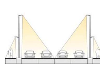
Stâlpi \geq 7m - distribuție asimetrică
