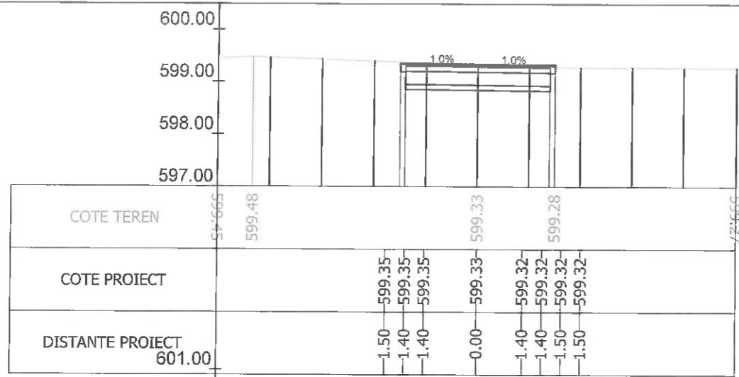
Sectiunea 113 - Km 1+248.364 Ax-Traseul 1
