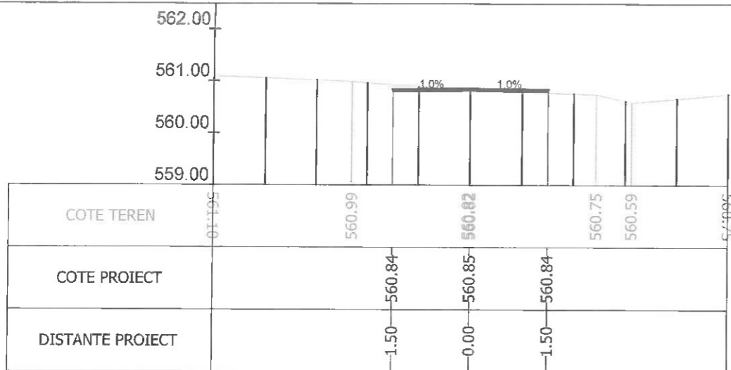
Sectiunea 381 - Km 5+064.292 Ax-Traseul 1
