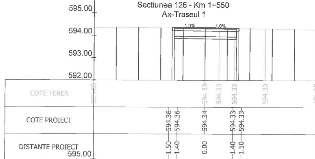
Sectiunea 128 - Km 1+600 Ax-Traseul 1
