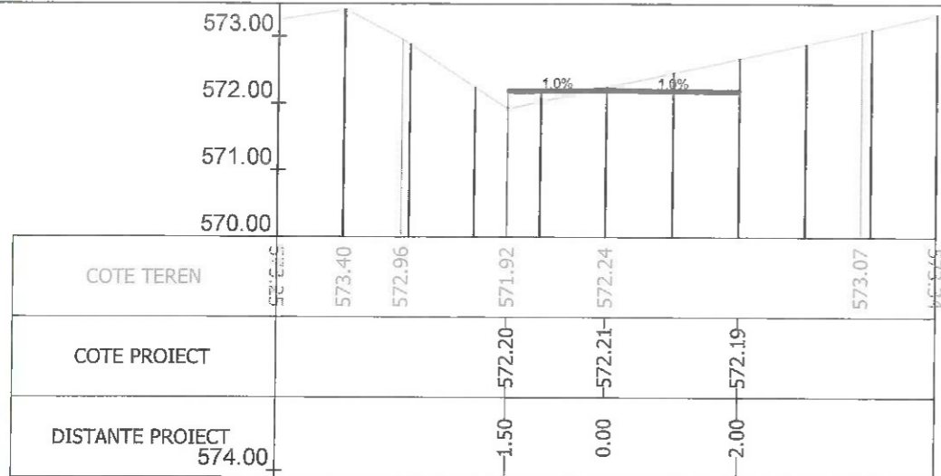
Sectiunea 239 - Km 3+325 Ax-Traseul 1
