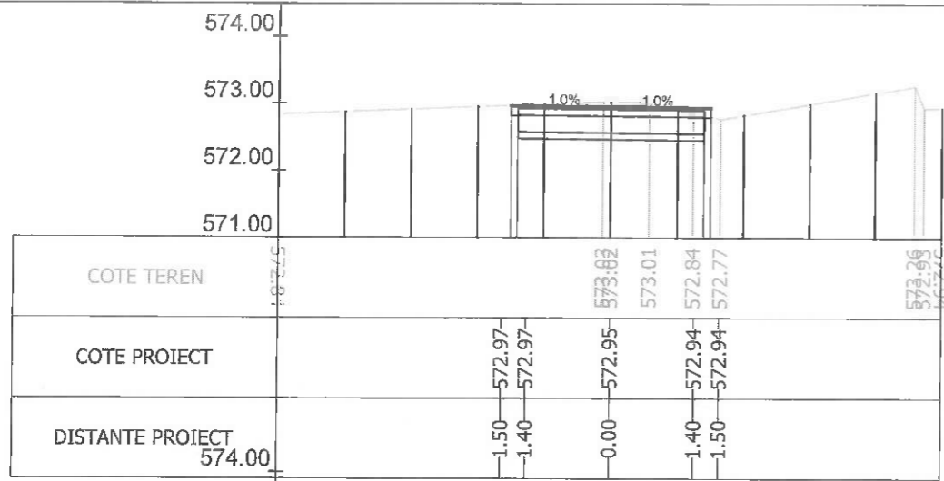
Sectiunea 233 - Km 3+257.500 Ax-Traseul 1
