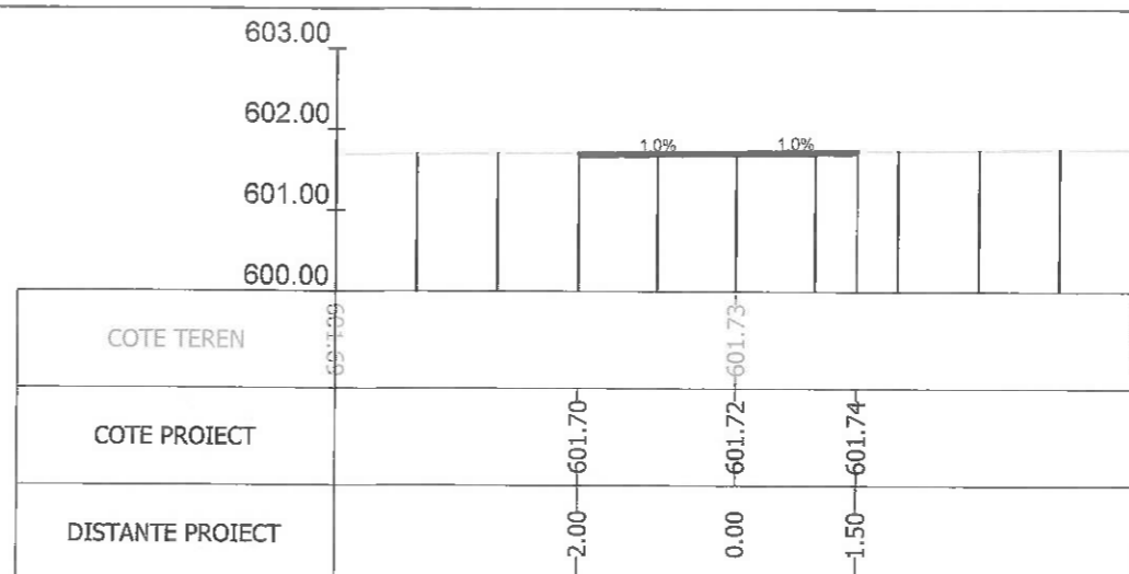
Sectiunea 40 - Km 0+275 Ax-Traseul 1
