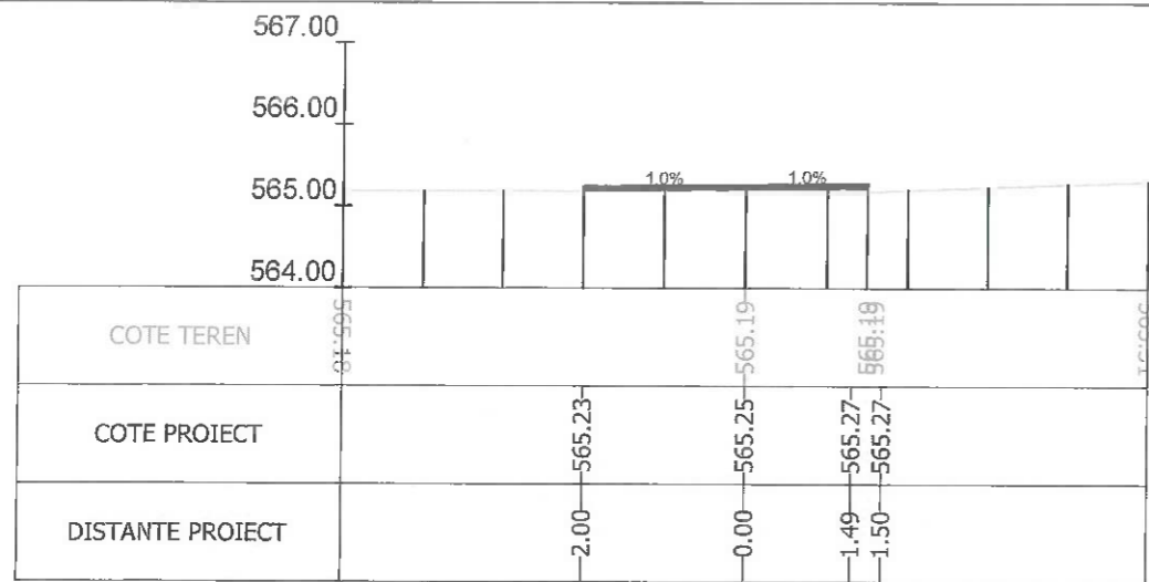
Sectiunea 340 - Km 4+593.592 Ax-Traseul 1
