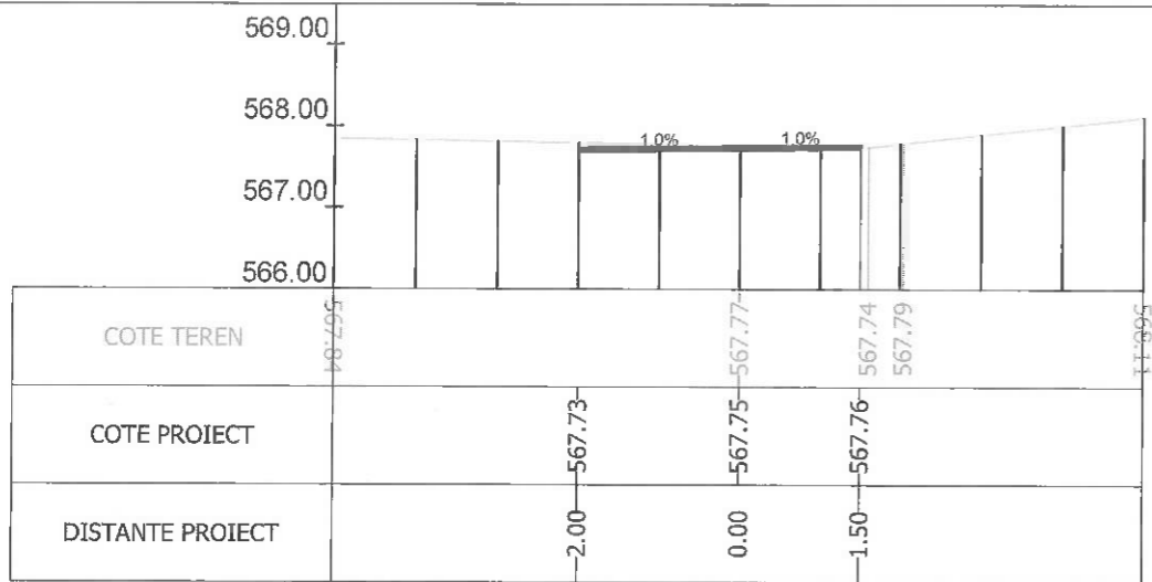
Sectiunea 334 - Km 4+500 Ax-Traseul 1
