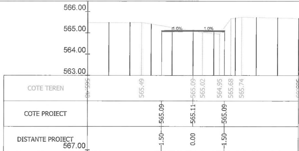
Sectiunea 448 - Km 5+998.856 Ax-Traseul 1
