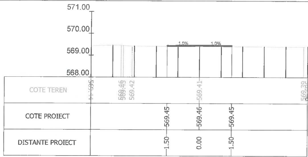
Sectiunea 283 - Km 4+075 Ax-Traseul 1
