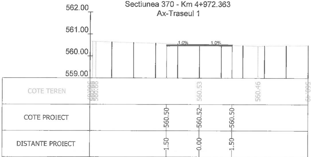
Sectiunea 377 - Km 5+008.491 Ax-Traseul 1
