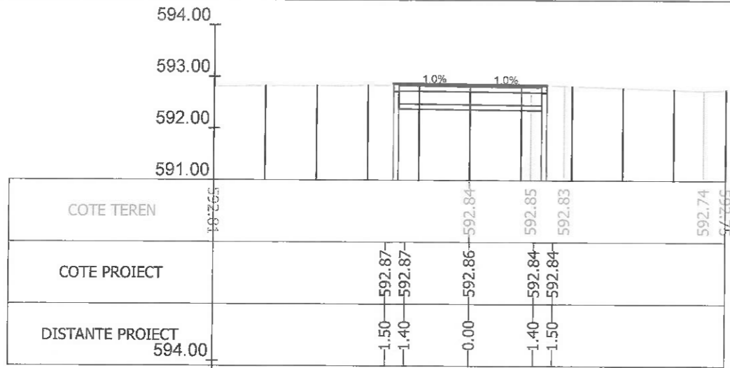
Sectiunea 131 - Km 1+675 Ax-Traseul 1
