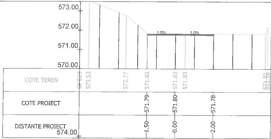
Sectiunea 245 - Km 3+425 Ax-Traseul 1
