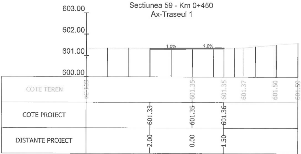
Sectiunea 61 - Km 0+500 Ax-Traseul 1
