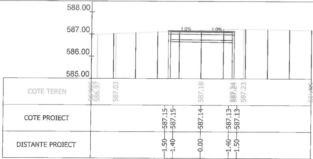
Sectiunea 155 - Km 2+100 Ax-Traseul 1
