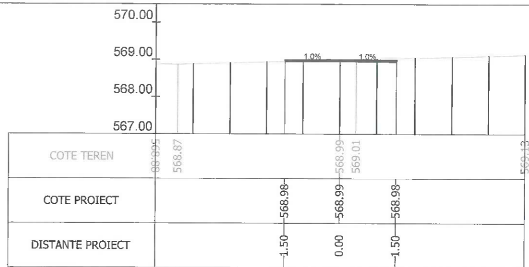
Sectiunea 284 - Km 4+100 Ax-Traseul 1
