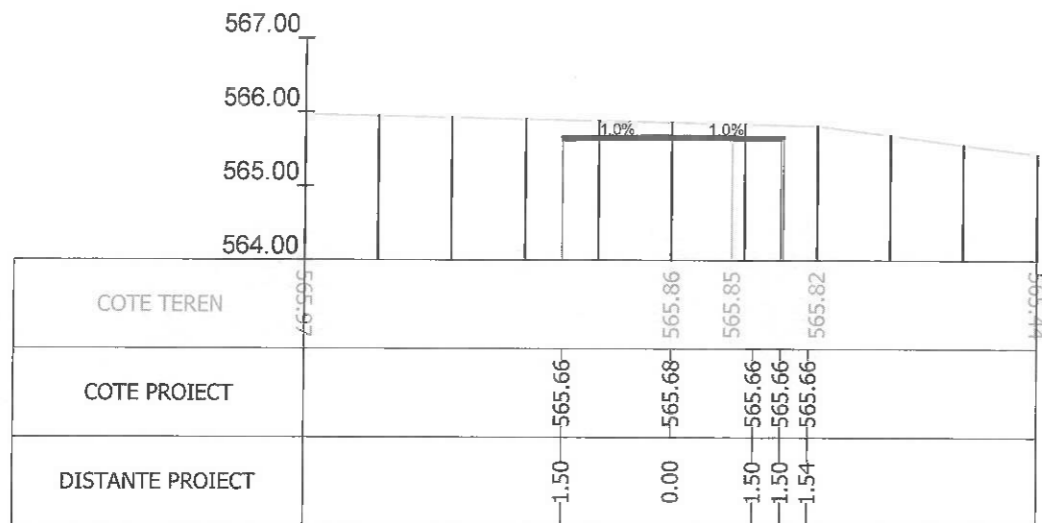
Sectiunea 467 - Km 6+138.881 Ax-Traseul 1
