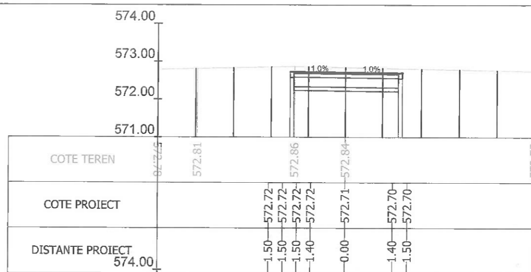
Sectiunea 234 - Km 3+266.013 Ax-Traseul 1
