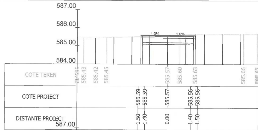
Sectiunea 162 - Km 2+225 Ax-Traseul 1
