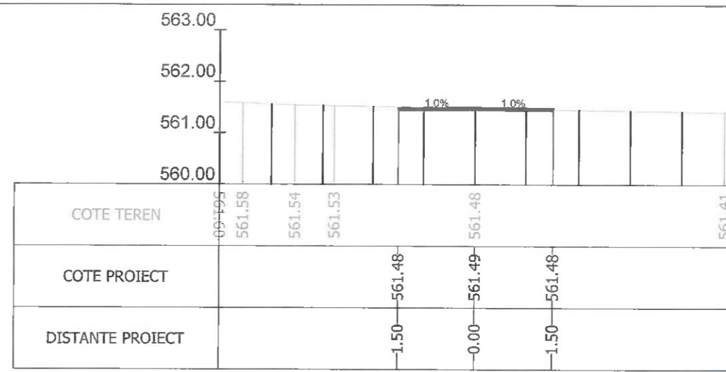
Sectiunea 388 - Km 5+125 Ax-Traseul 1
