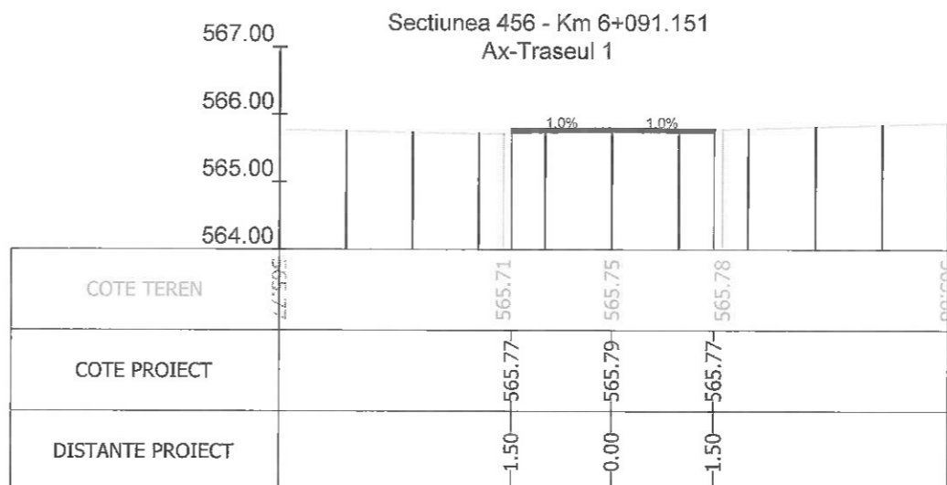
Sectiunea 456 - Km 6+091.151 Ax-Traseul 1
