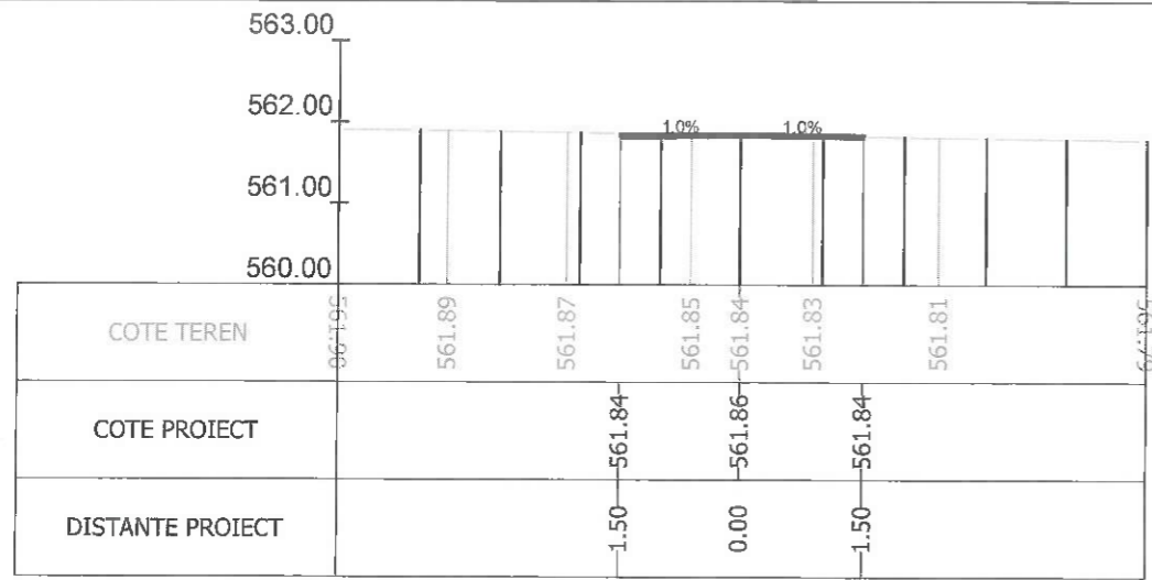
Sectiunea 393 - Km 5+175 Ax-Traseul 1
