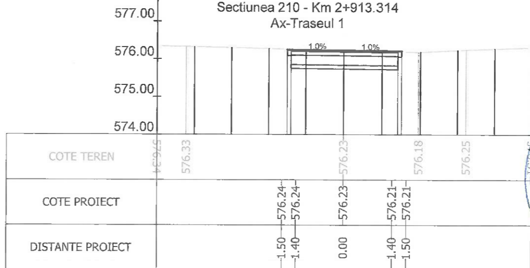
Sectiunea 212 - Km 2+950 Ax-Traseul 1
