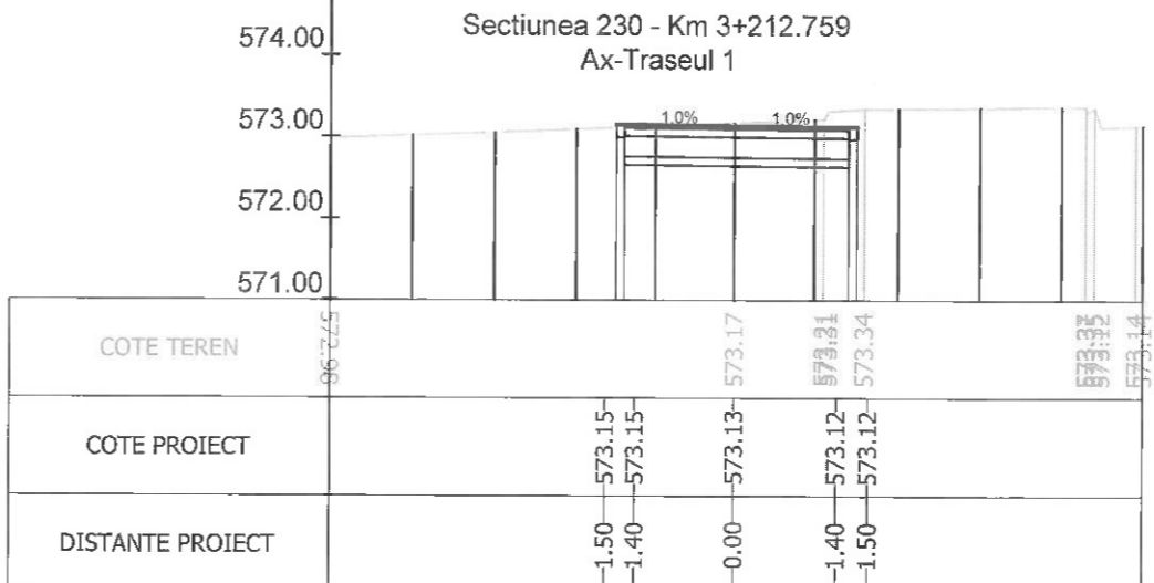
Sectiunea 232 - Km 3+250 Ax-Traseul 1
