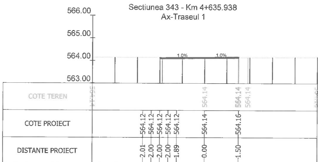
Sectiunea 345 - Km 4+653.858 Ax-Traseul 1
