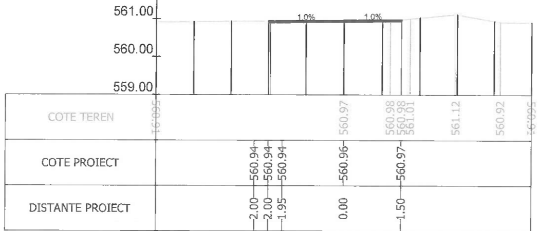
Sectiunea 366 - Km 4+924.303 Ax-Traseul 1
