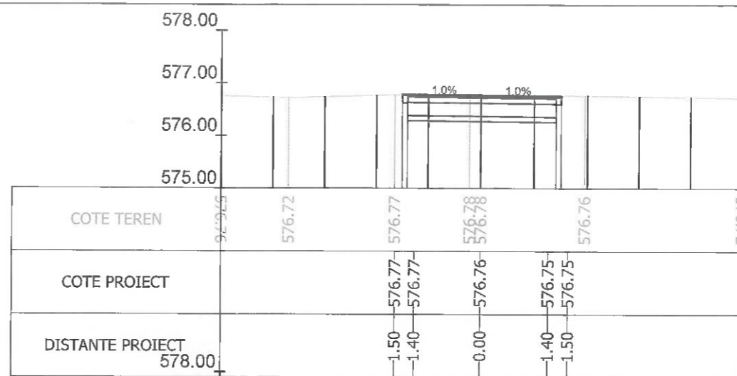
Sectiunea 210 - Km 2+913.314 Ax-Traseul 1
