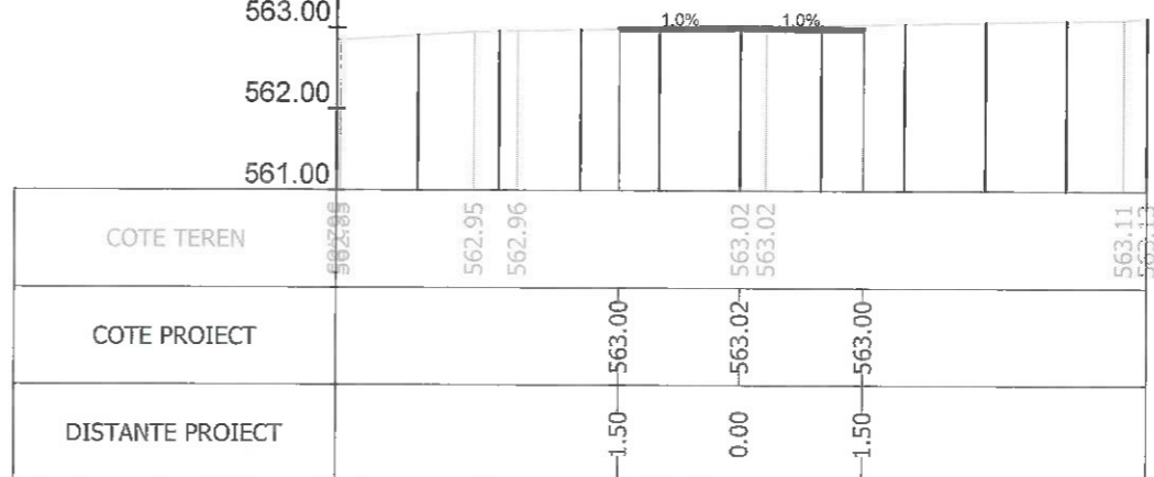
Sectiunea 402 - Km 5+300 Ax-Traseul 1
