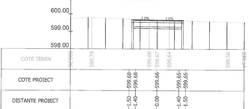
Sectiunea 112 - Km 1+225 Ax-Traseul 1
