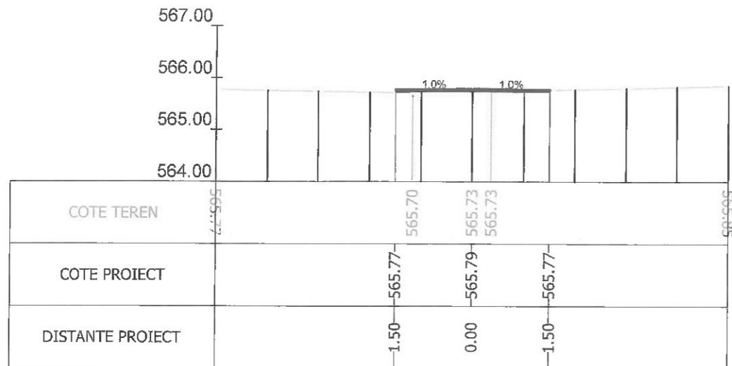
Sectiunea 459 - Km 6+116.317 Ax-Traseul 1
