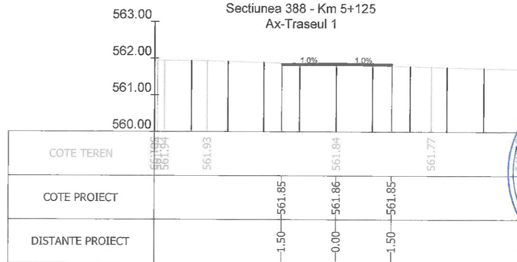
Sectiunea 390 - Km 5+157.555 Ax-Traseul 1
