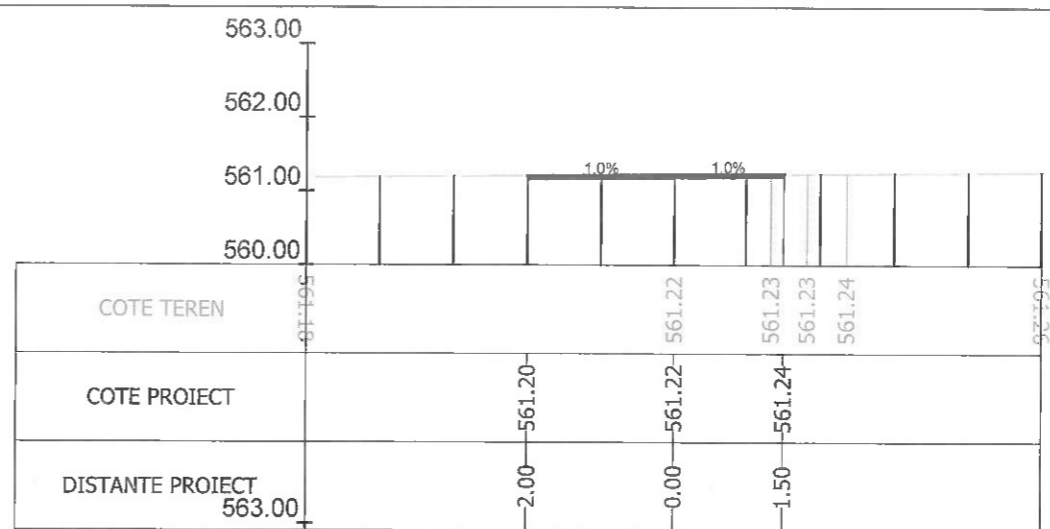
Sectiunea 365 - Km 4+900 Ax-Traseul 1
