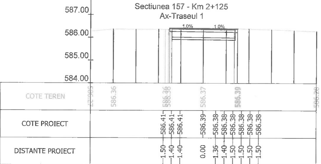
Sectiunea 159 - Km 2+164.829 Ax-Traseul 1
