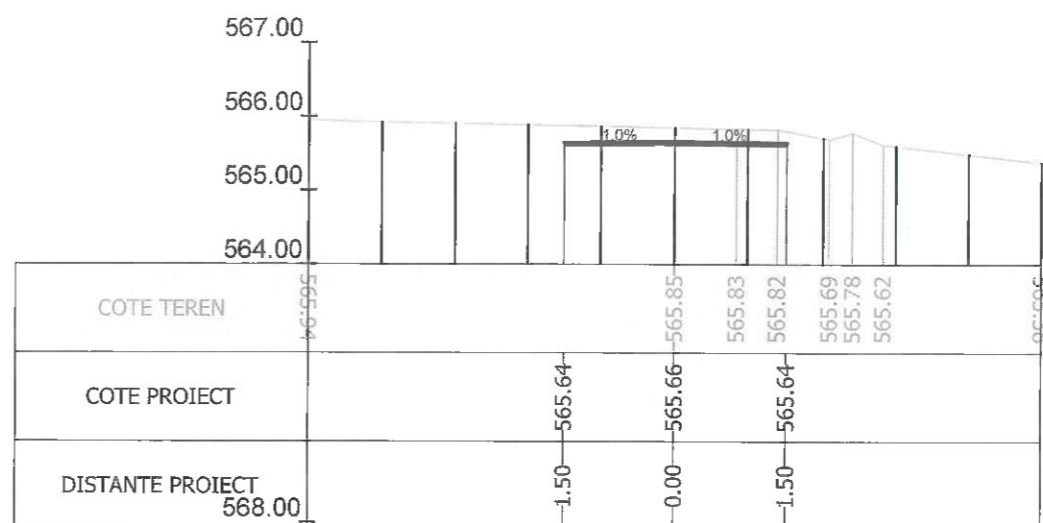
Sectiunea 468 - Km 6+141.651 Ax-Traseul 1
