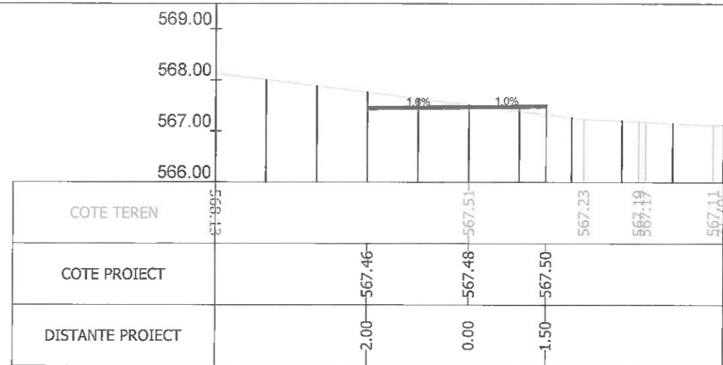
Sectiunea 302 - Km 4+300 Ax-Traseul 1
