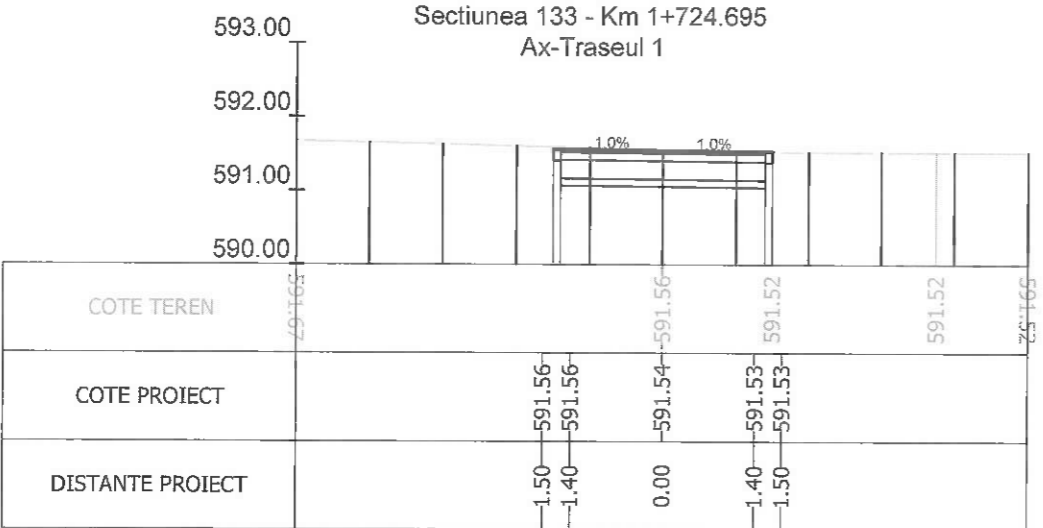
Sectiunea 135 - Km 1+750 Ax-Traseul 1
