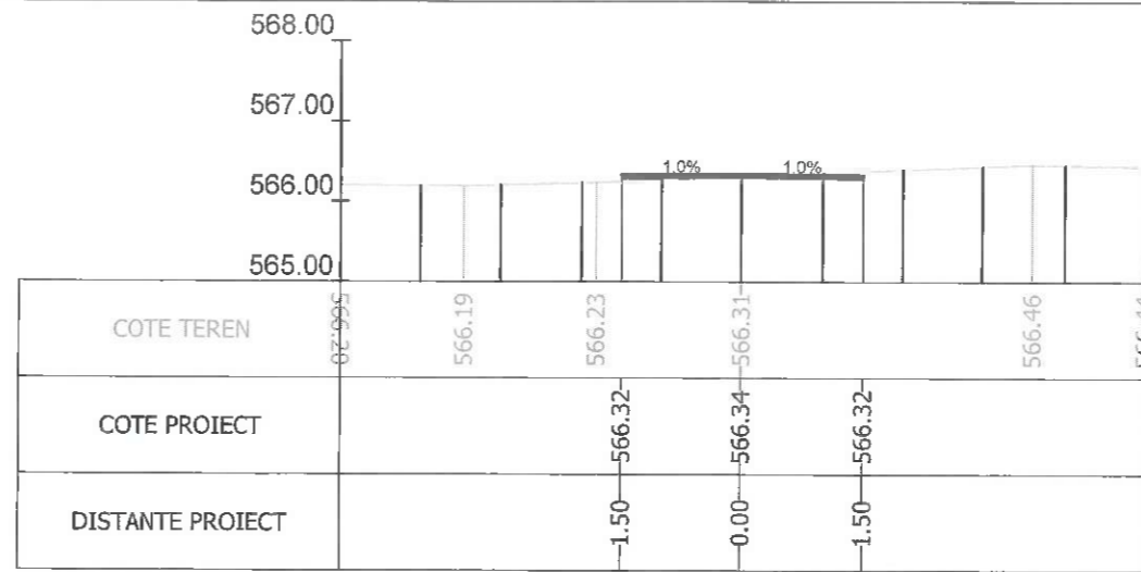
Sectiunea 430 - Km 5+818.635 Ax-Traseul 1
