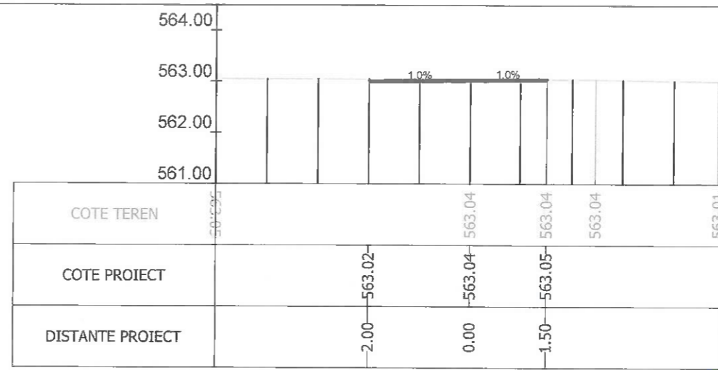
Sectiunea 353 - Km 4+750 Ax-Traseul 1
