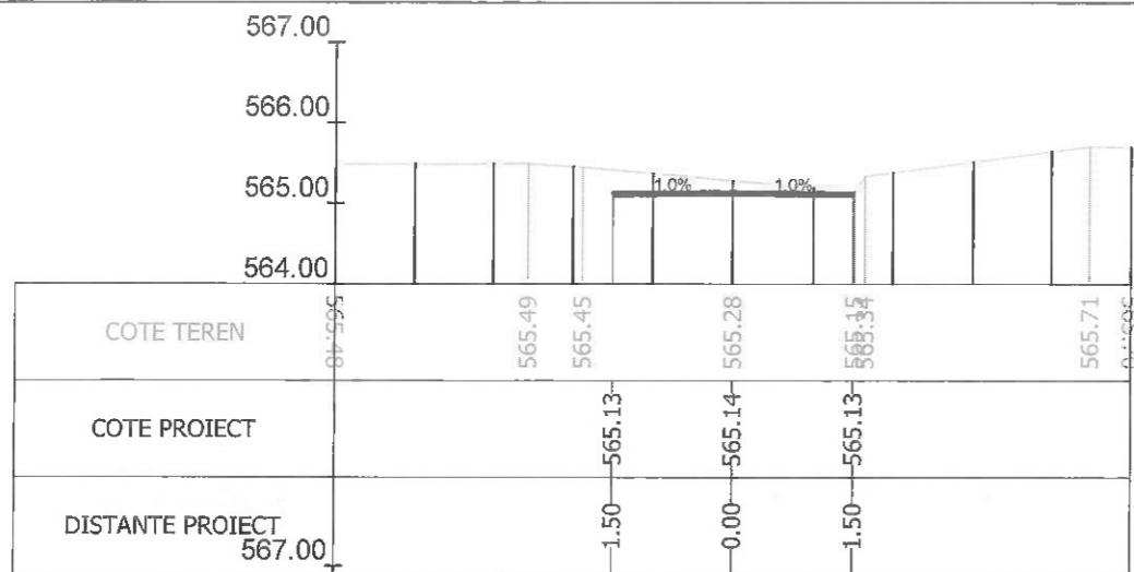
Sectiunea 447 - Km 5+995.821 Ax-Traseul 1
