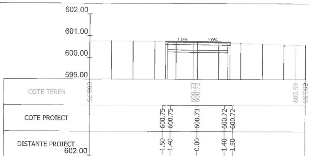
Sectiunea 108 - Km 1+150 Ax-Traseul 1
