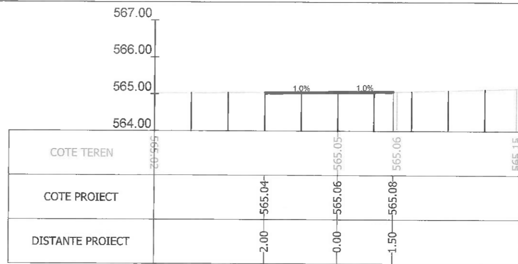
Sectiunea 341 - Km 4+600 Ax-Traseul 1
