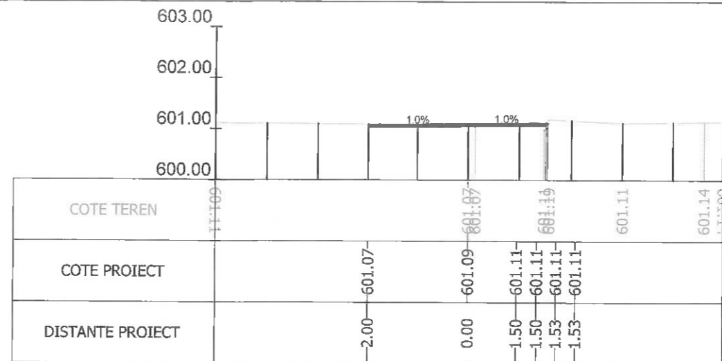
Sectiunea 26 - Km 0+153.895 Ax-Traseul 1
