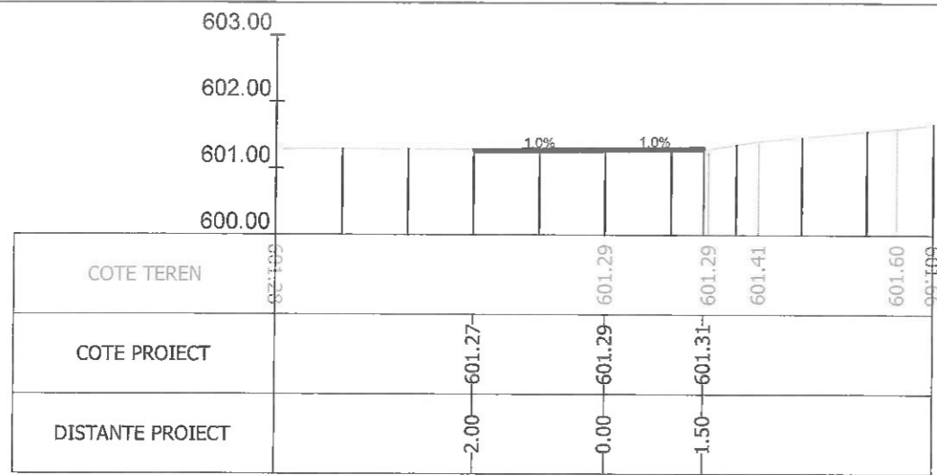
Sectiunea 45 - Km 0+325 Ax-Traseul 1
