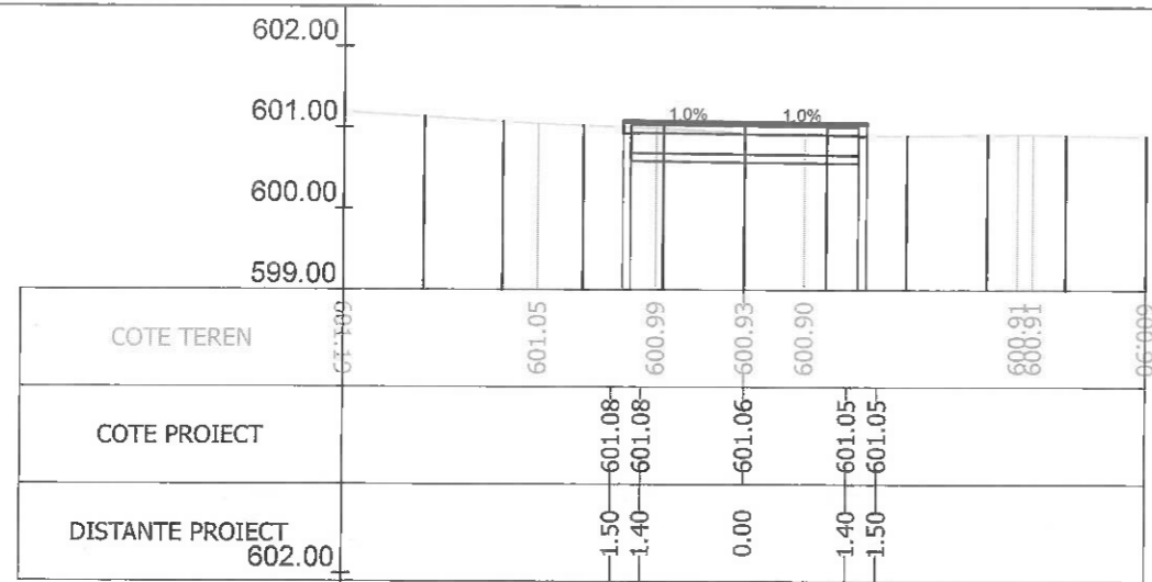
Sectiunea 107 - Km 1+128.989 Ax-Traseul 1
