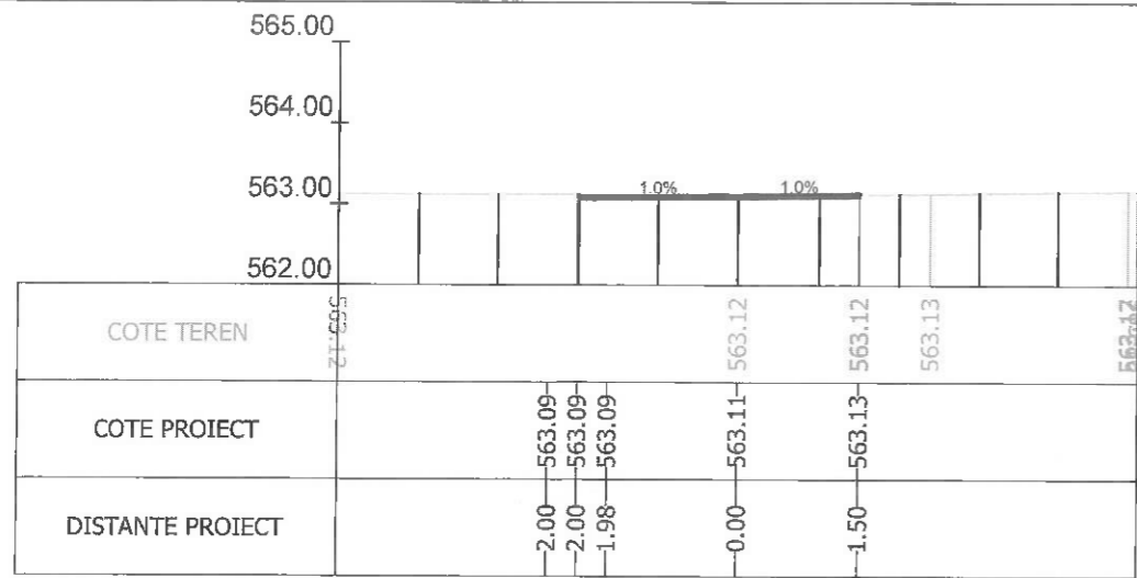
Sectiunea 352 - Km 4+743.422 Ax-Traseul 1
