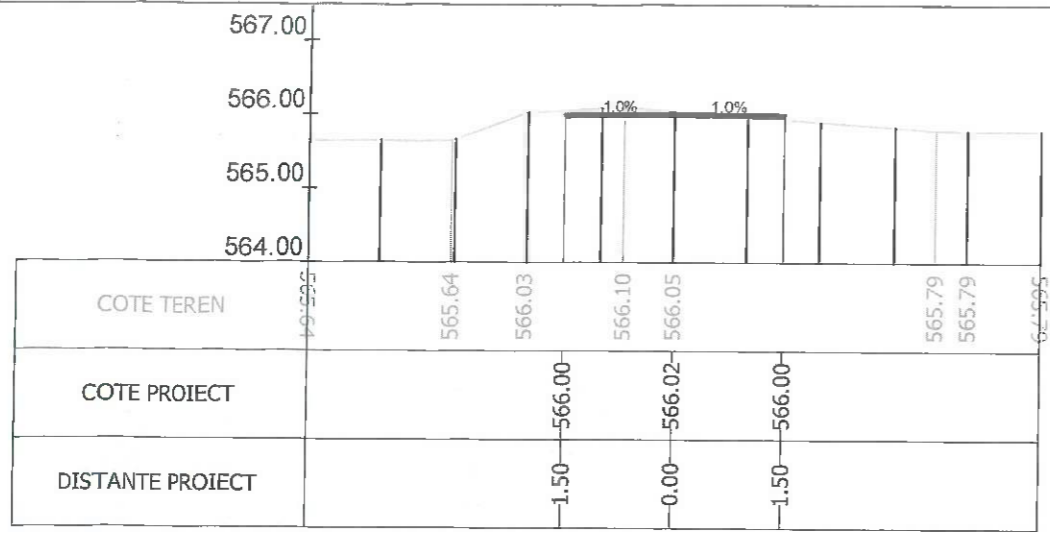
Sectiunea 441 - Km 5+925 Ax-Traseul 1
