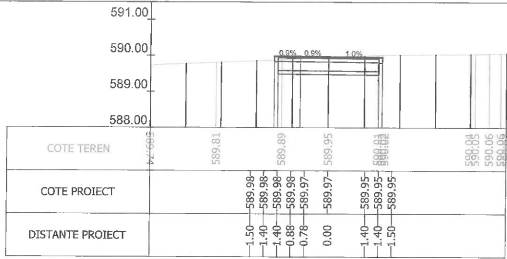
Sectiunea 143 - Km 1+879.943 Ax-Traseul 1
