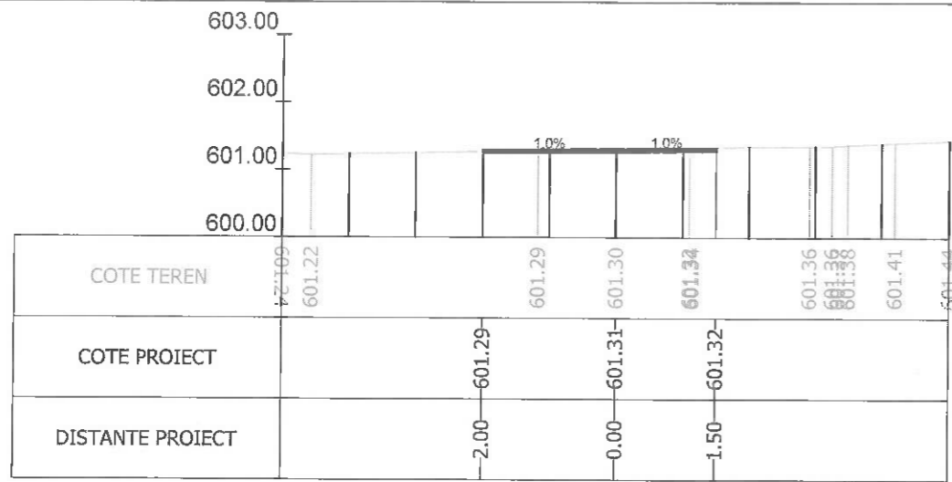
Sectiunea 63 - Km 0+525 Ax-Traseul 1
