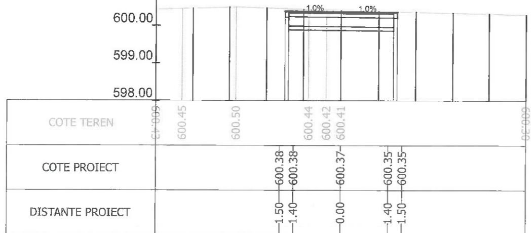
Sectiunea 109 - Km 1+175 Ax-Traseul 1
