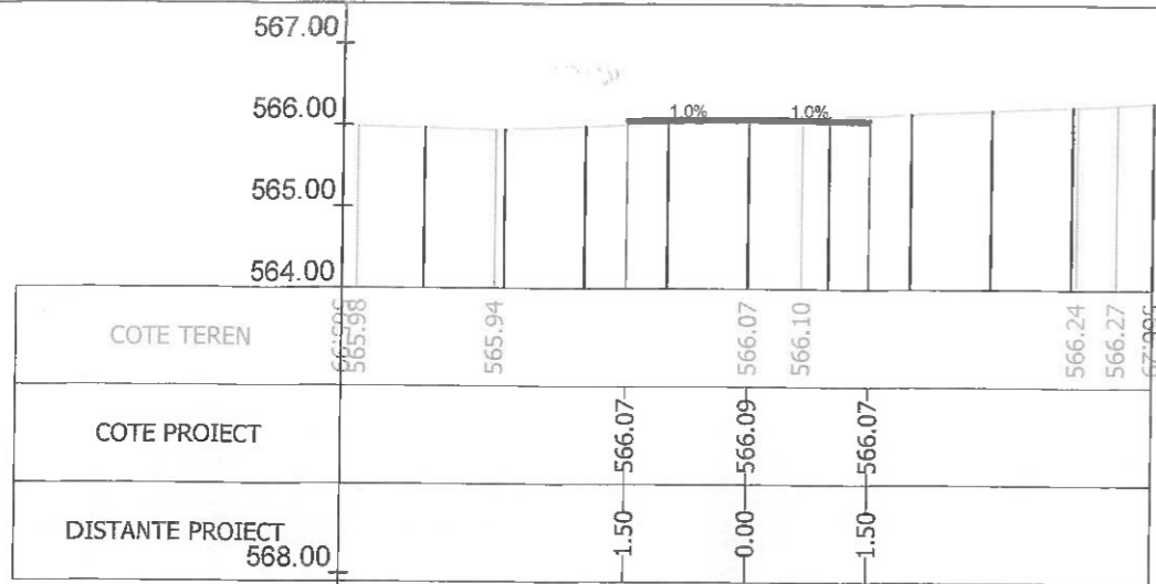
Sectiunea 435 - Km 5+856.096 Ax-Traseul 1
