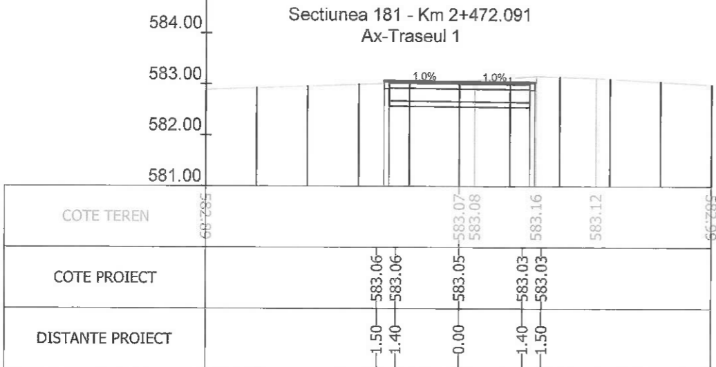
Sectiunea 183 - Km 2+475 Ax-Traseul 1
