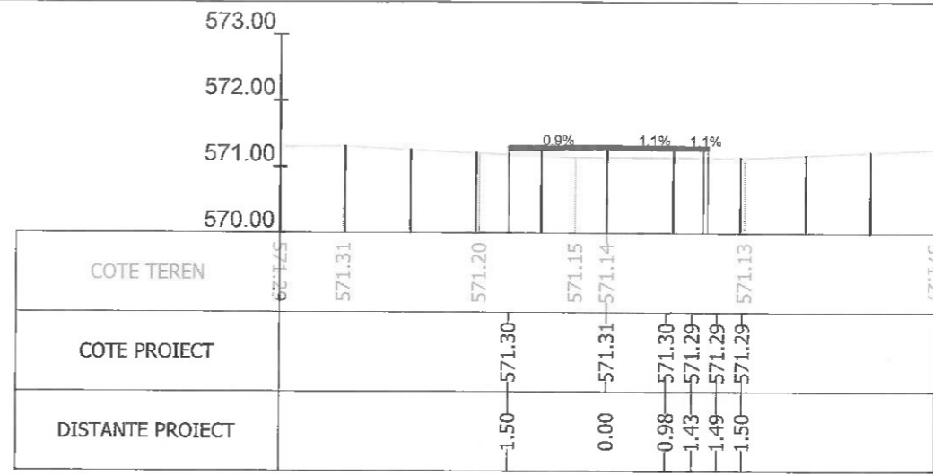
Sectiunea 278 - Km 3+952.863 Ax-Traseul 1
