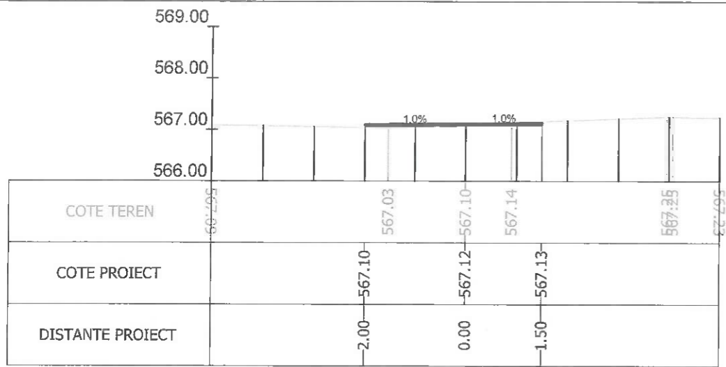
Sectiunea 301 - Km 4+275 Ax-Traseul 1
