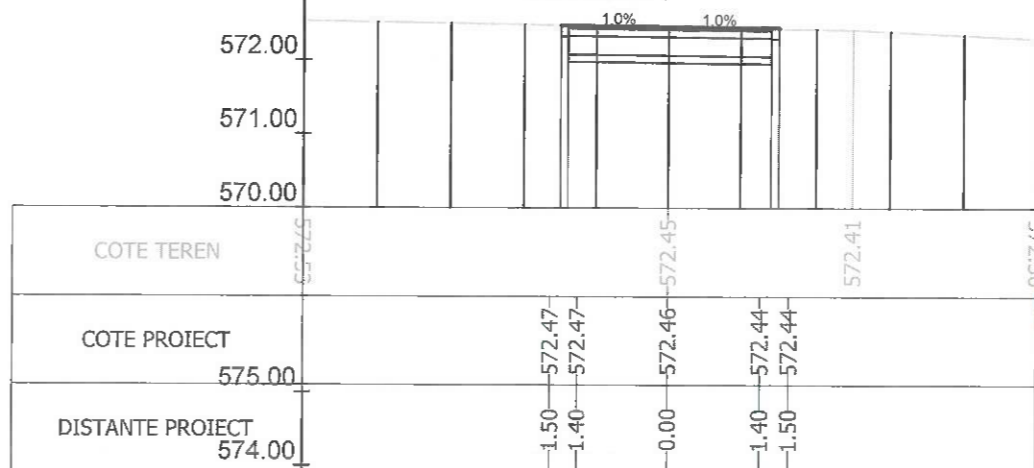
Sectiunea 236 - Km 3+275 Ax-Traseul 1
