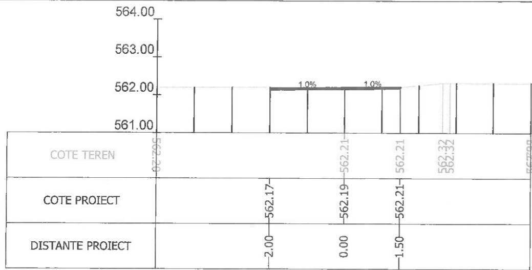
Sectiunea 358 - Km 4+820.304 Ax-Traseul 1
