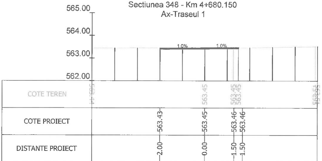
Sectiunea 348 - Km 4+680.150 Ax-Traseul 1
