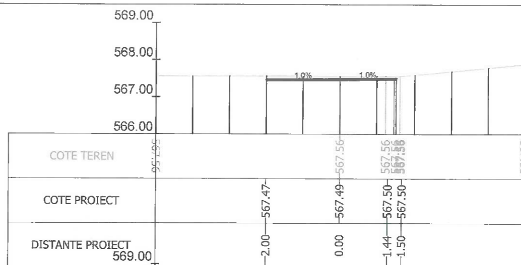
Sectiunea 335 - Km 4+517.333 Ax-Traseul 1
