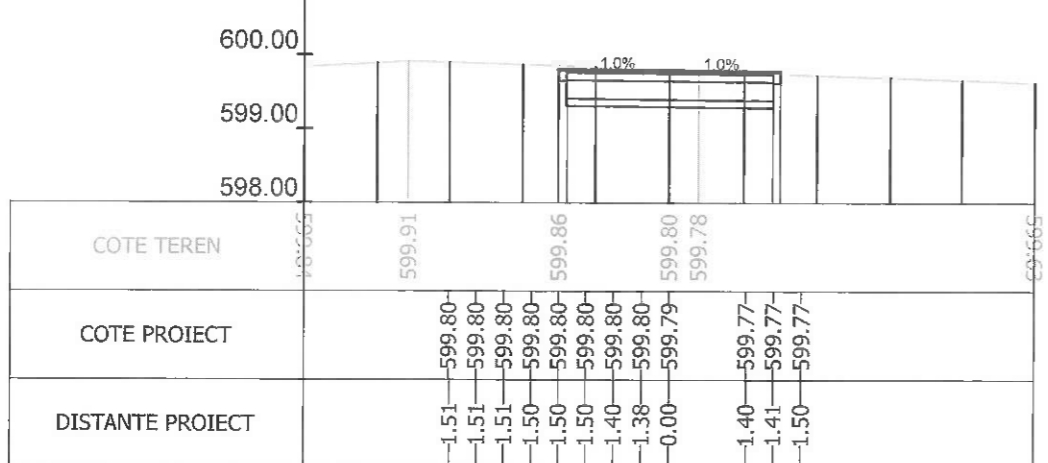
Sectiunea 111 - Km 1+216.073 Ax-Traseul 1
