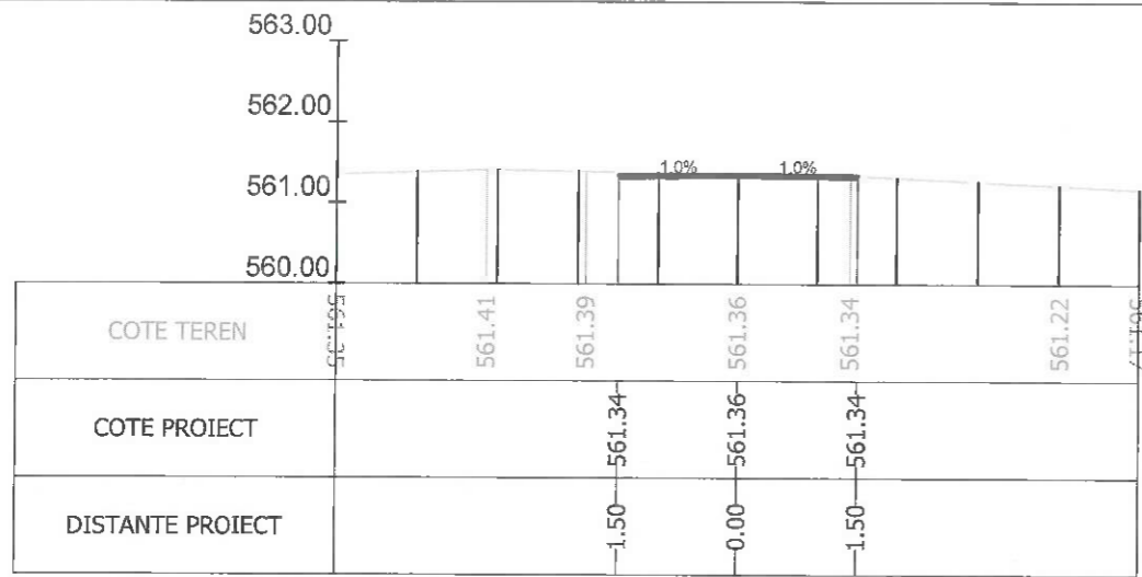
Sectiunea 387 - Km 5+100 Ax-Traseul 1
