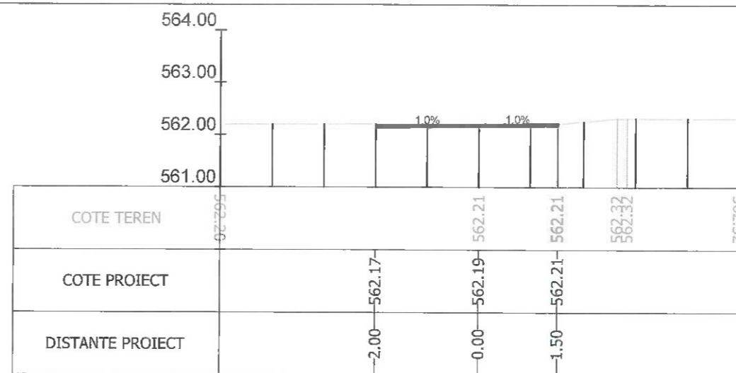
Sectiunea 359 - Km 4+820.305 Ax-Traseul 1
