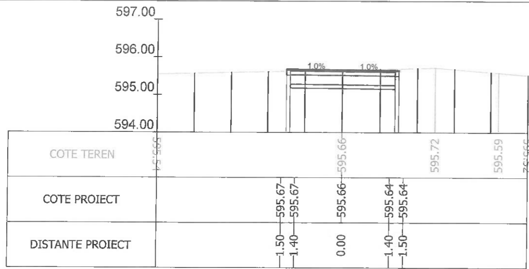
Sectiunea 125 - Km 1+525 Ax-Traseul 1
