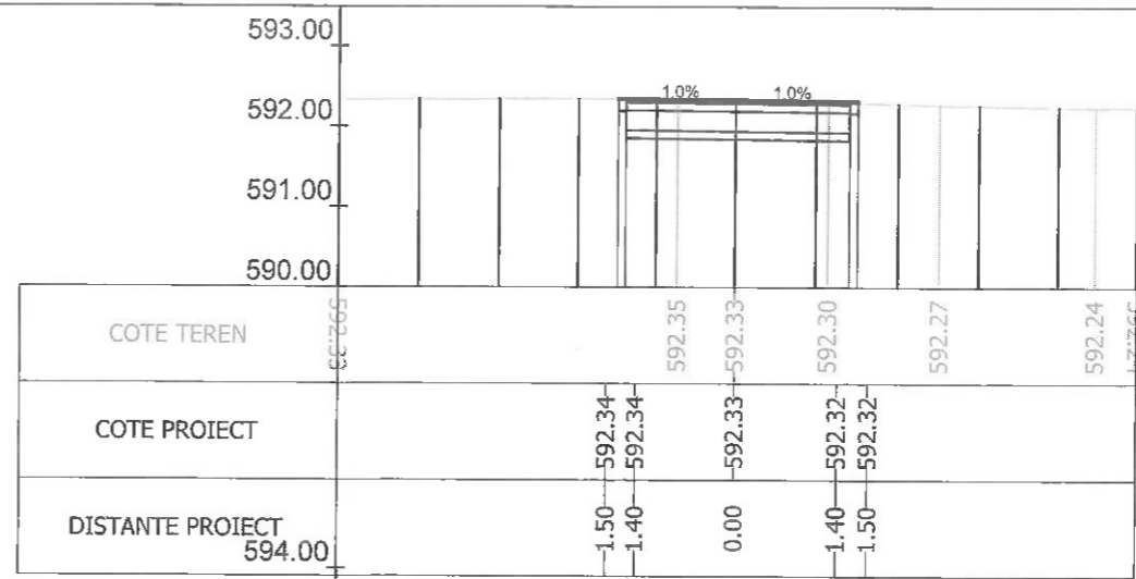
Sectiunea 132 - Km 1+700 Ax-Traseul 1
