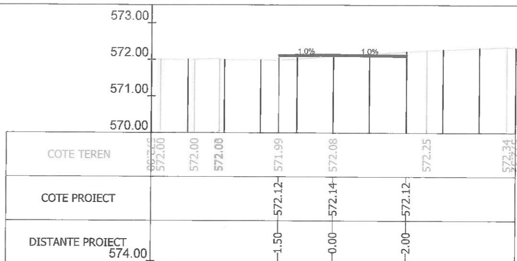
Sectiunea 240 - Km 3+350 Ax-Traseul 1
