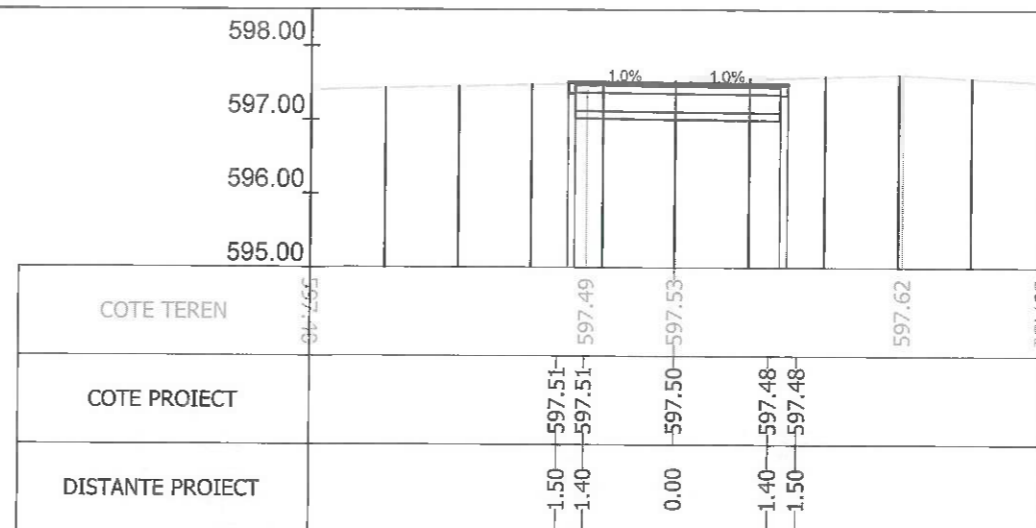
Sectiunea 120 - Km 1+400 Ax-Traseul 1
