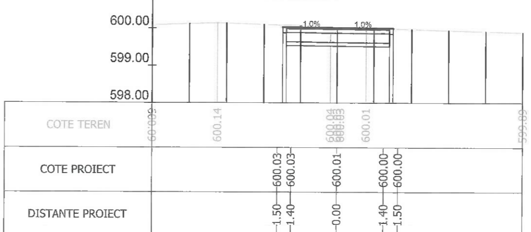
Sectiunea 110 - Km 1+200 Ax-Traseul 1
