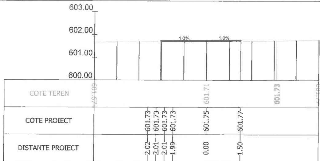
Sectiunea 39 - Km 0+266.560 Ax-Traseul 1
