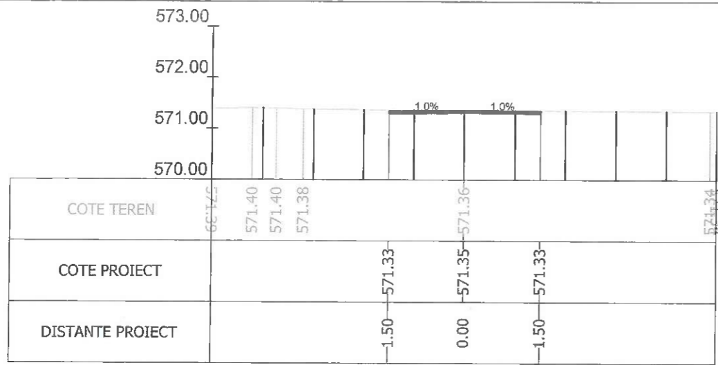
Sectiunea 277 - Km 3+950 Ax-Traseul 1
