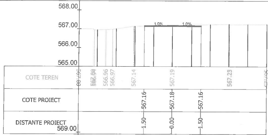
Sectiunea 423 - Km 5+725 Ax-Traseul 1
