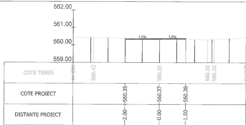
Sectiunea 371 - Km 4+975 Ax-Traseul 1
