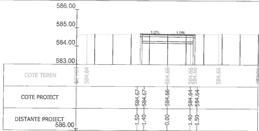
Sectiunea 167 - Km 2+300 Ax-Traseul 1
