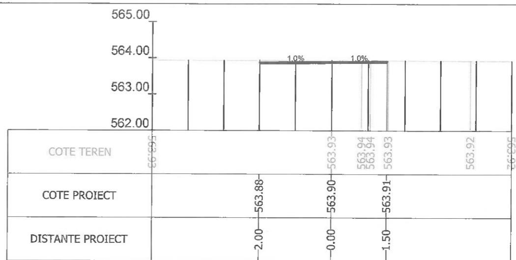
Sectiunea 349 - Km 4+700 Ax-Traseul 1
