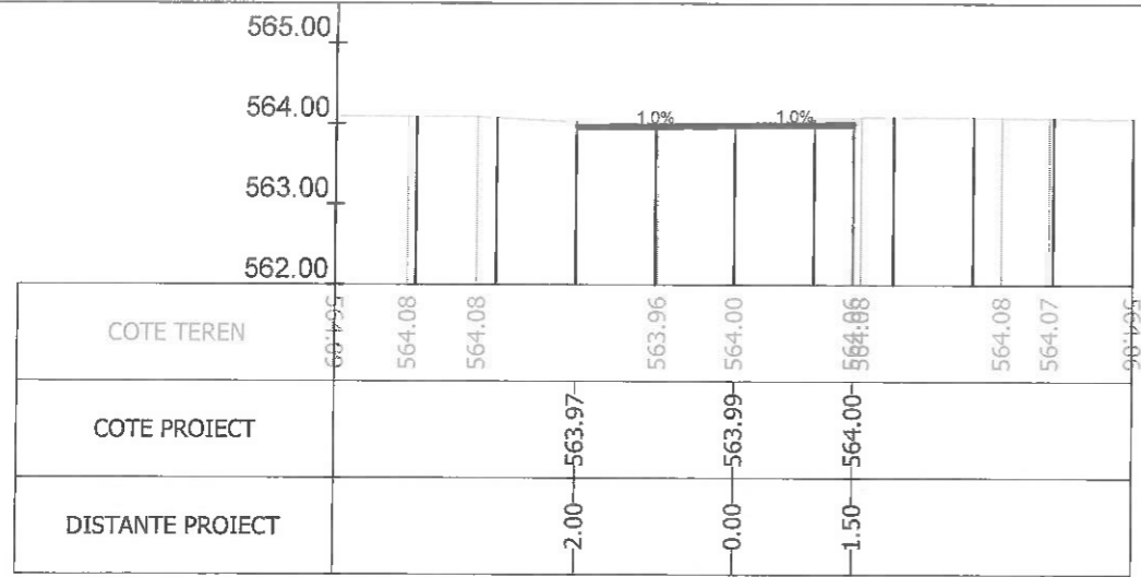
Sectiunea 346 - Km 4+666.984 Ax-Traseul 1
