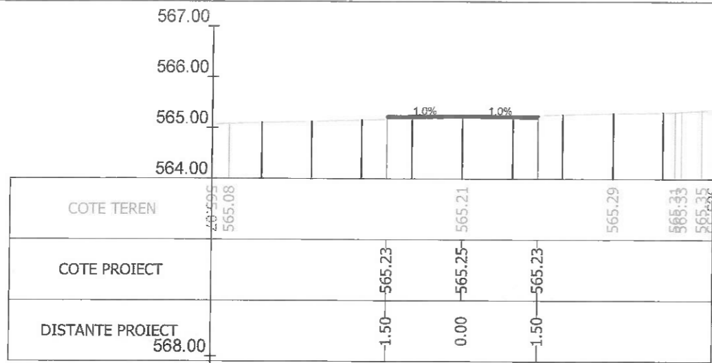
Sectiunea 411 - Km 5+525 Ax-Traseul 1
