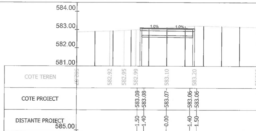
Sectiunea 180 - Km 2+470.754 Ax-Traseul 1
