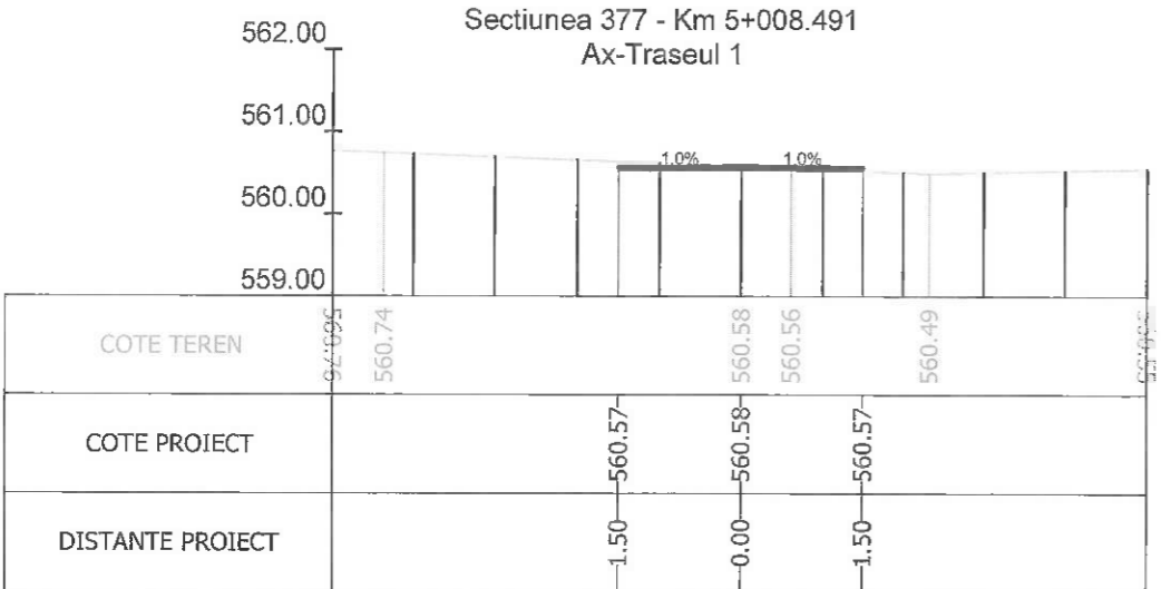
Sectiunea 379 - Km 5+043.449 Ax-Traseul 1
