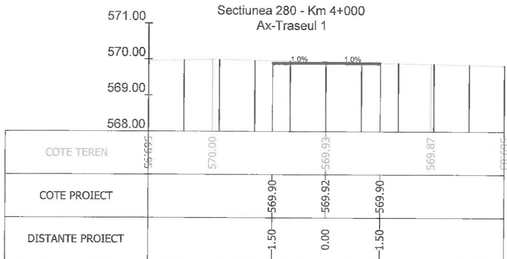
Sectiunea 282 - Km 4+050 Ax-Traseul 1
