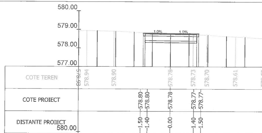
Sectiunea 198 - Km 2+725 Ax-Traseul 1
