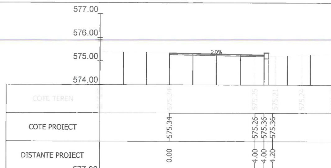
Sectiunea 201 - Km 2+900
