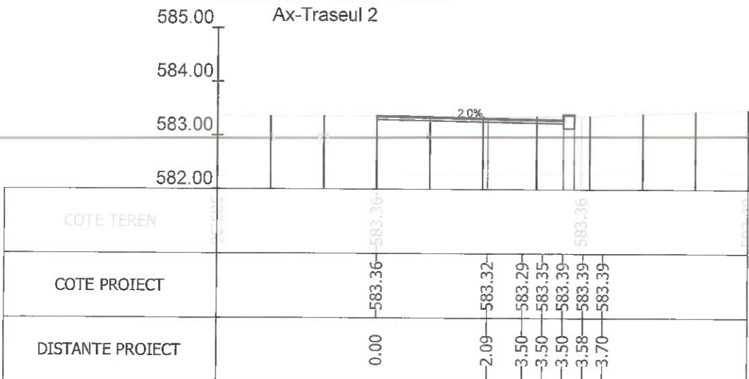
Sectiunea 379 - Km 5+475 Ax-Traseul 2
