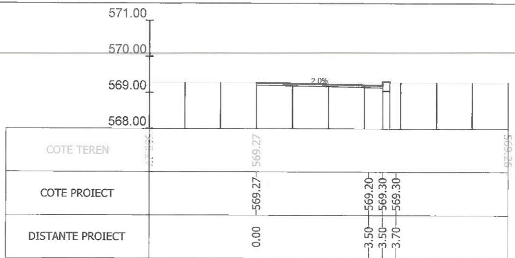
Sectiunea 430 - Km 5+790.250 Ax-Traseul 1
