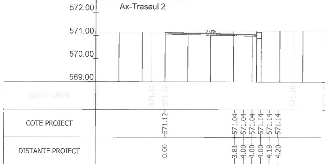
Sectiunea 304 - Km 4+475 Ax-Traseul 2
