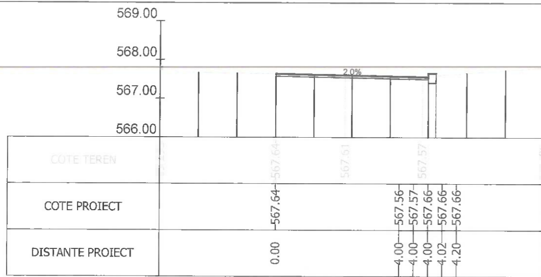
Sectiunea 278 - Km 4+102.825
