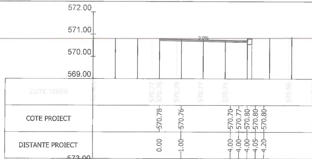
Sectiunea 302 - Km 4+425 Ax-Traseul 2
