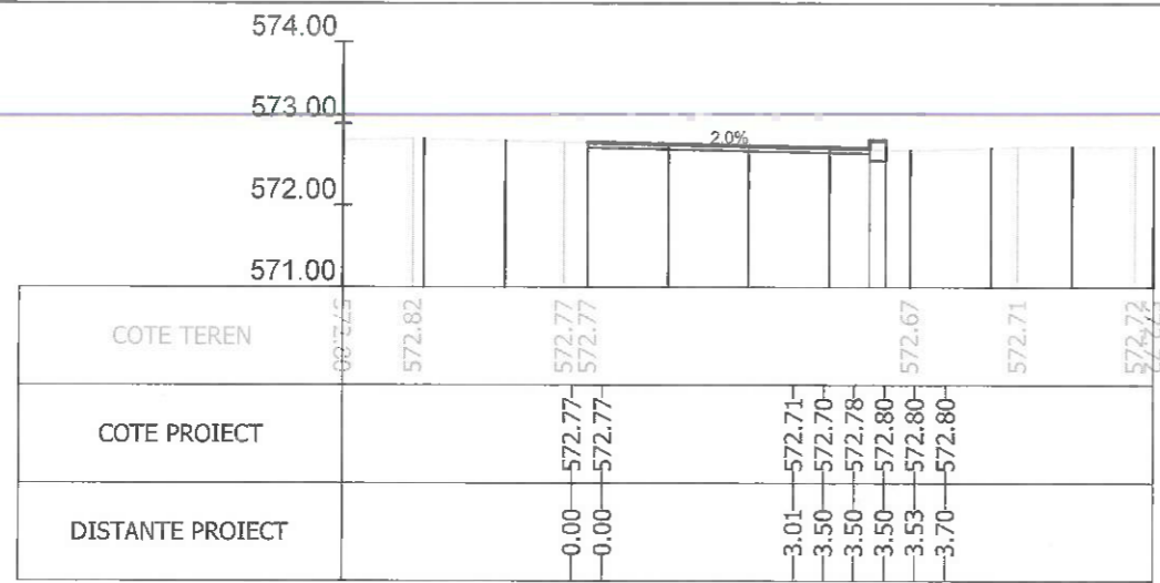
Sectiunea 200 - Km 2+675 Ax-Traseul 1
