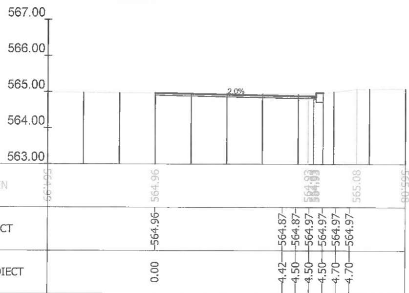
Sectiunea 300 - Km 4+158.374 Ax-Traseul 1
