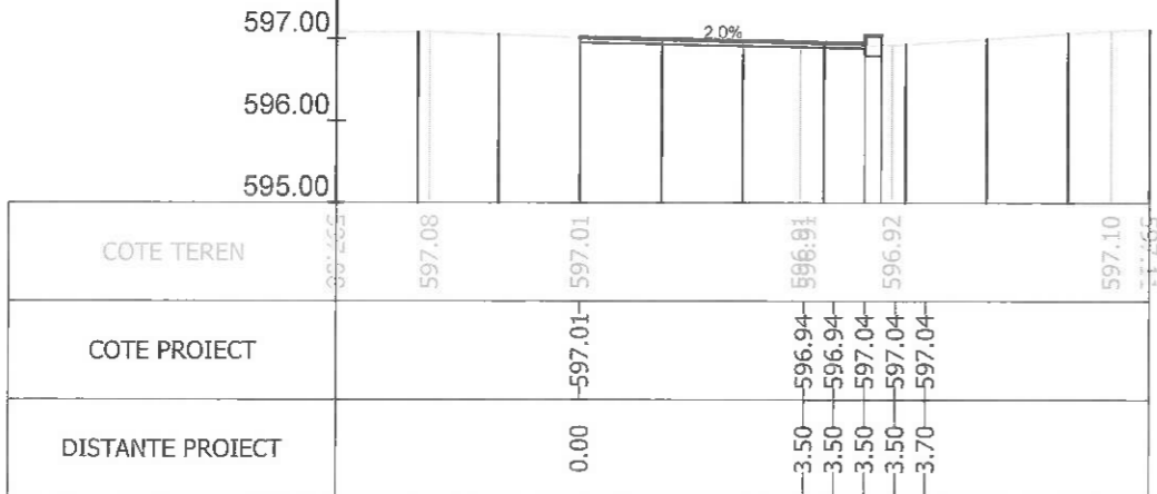
Sectiunea 46 - Km 0+550 Ax-Traseul 1
