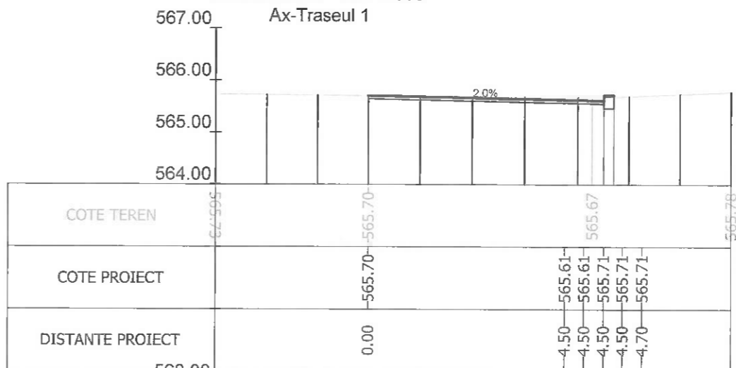
Sectiunea 313 - Km 4+325.968 Ax-Traseul 1
