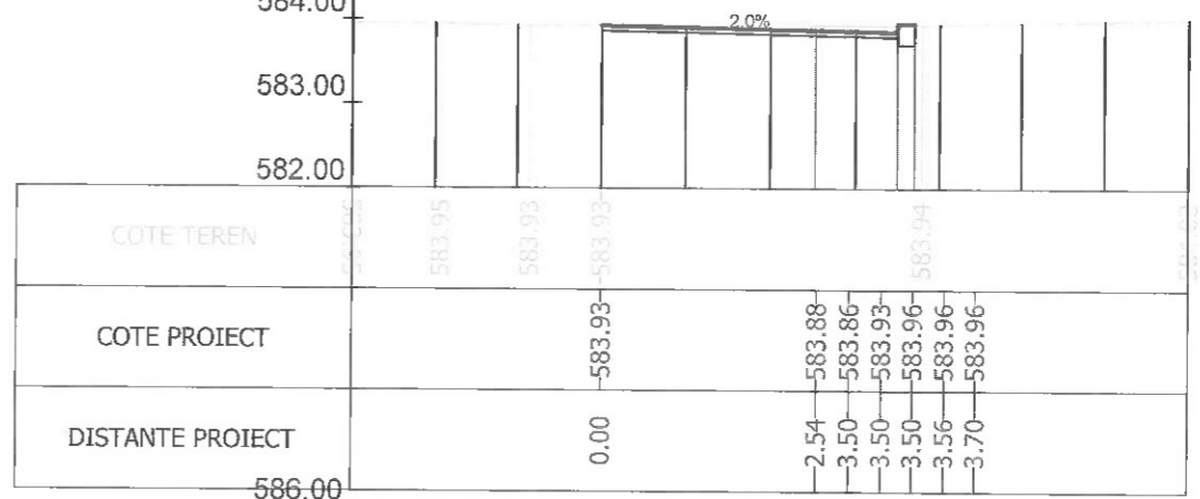
Sectiunea 384 - Km 5+575 Ax-Traseul 2
