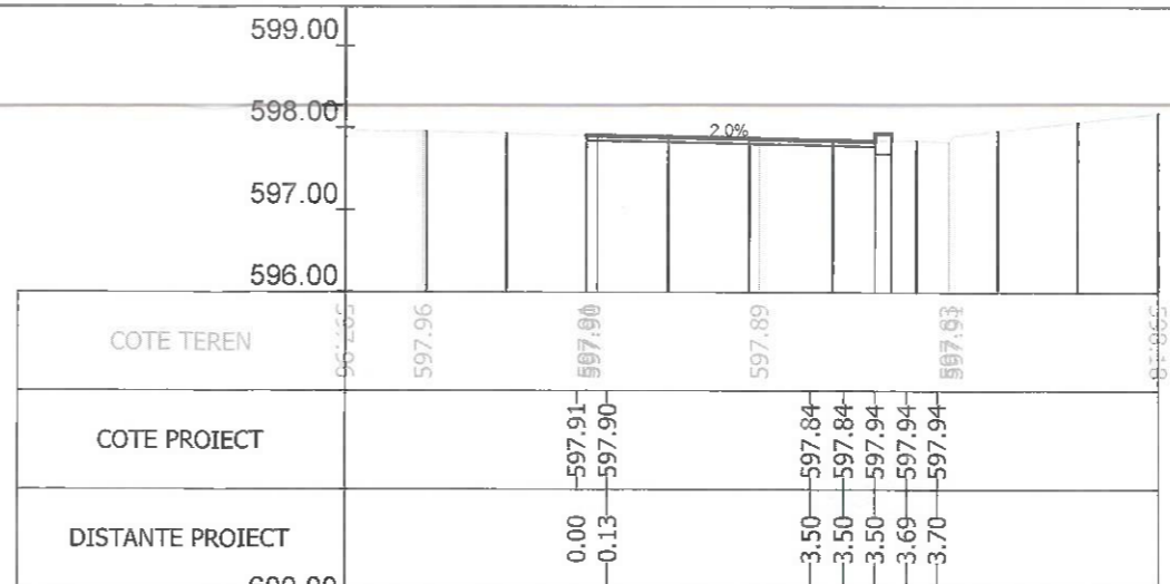
Sectiunea 41 - Km 0+475 Ax-Traseul 1
