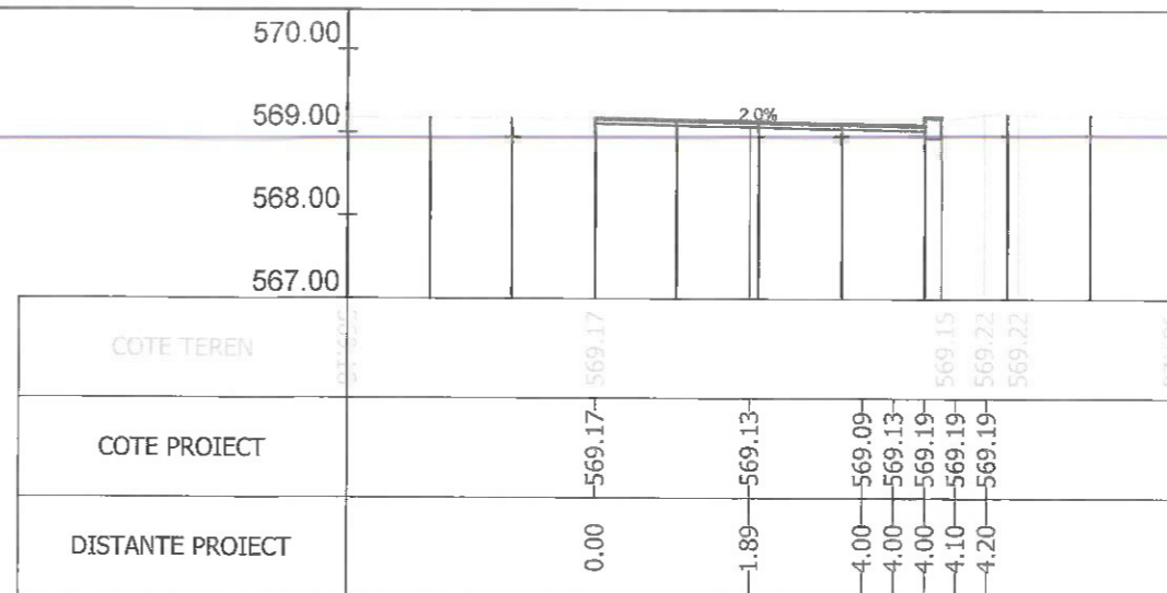
Sectiunea 237 - Km 3+375 Ax-Traseul 2
