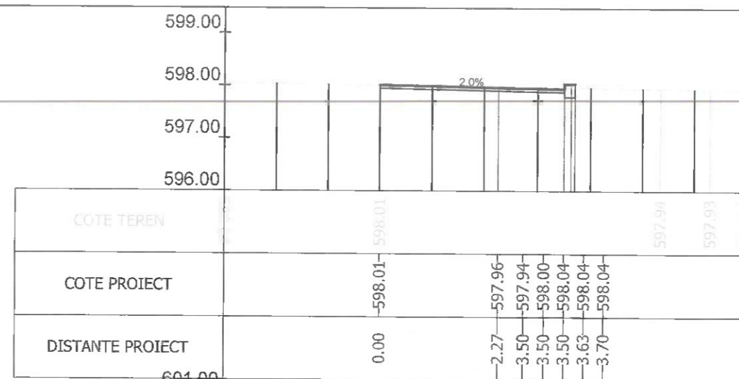
Sectiunea 457 - Km 6+775 Ax-Traseul 2
