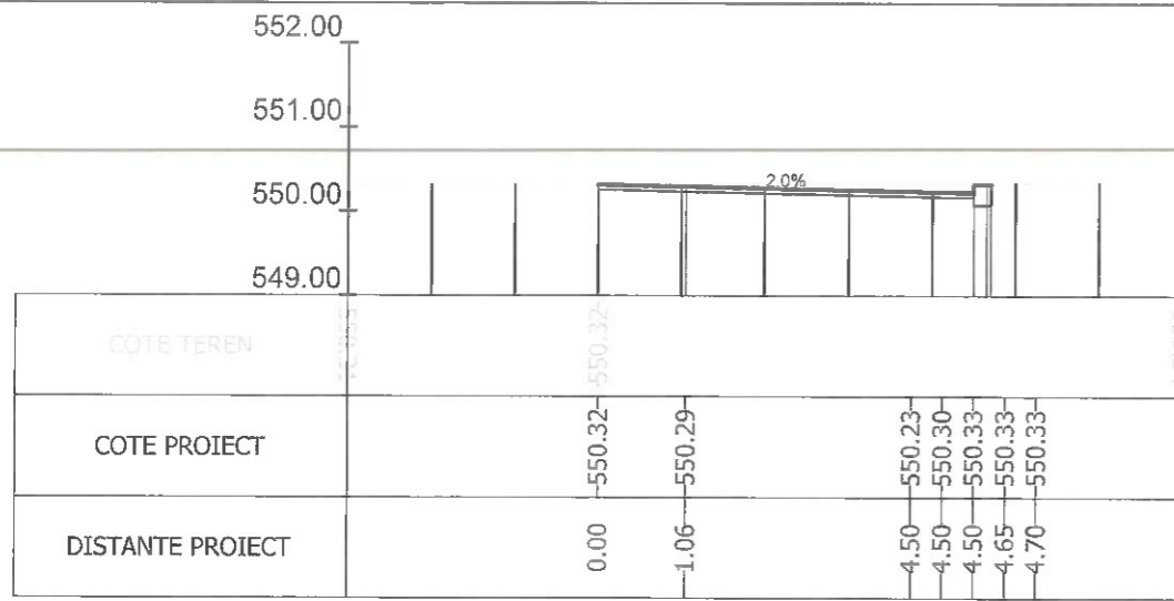
Sectiunea 36 - Km 0+550 Ax-Traseul 2
