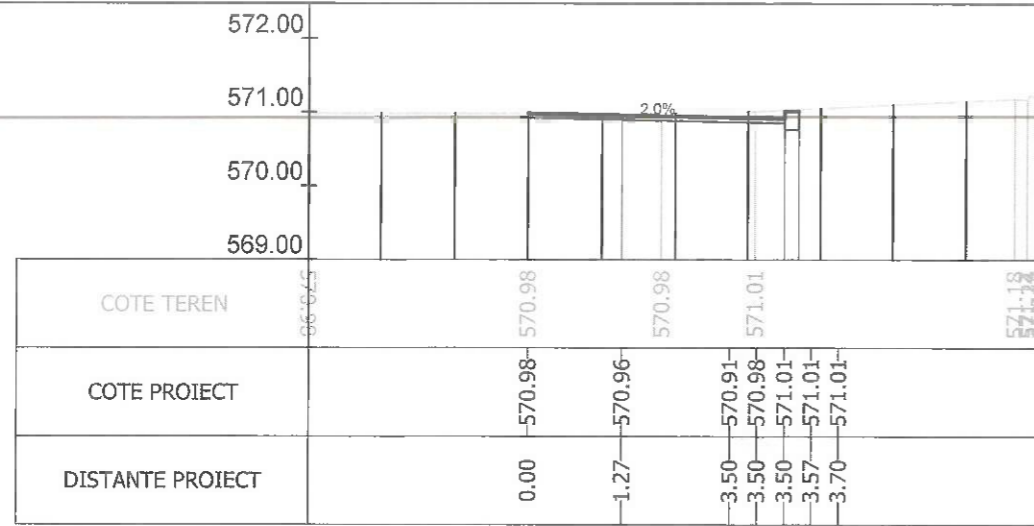
Sectiunea 423 - Km 5+675 Ax-Traseul 1
