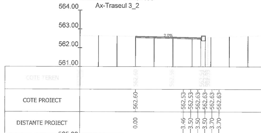
Sectiunea 16 - Km 0+176.633 Ax-Traseul 3_2
