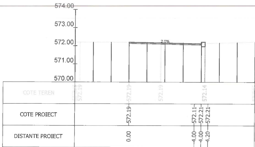
Sectiunea 216 - Km 3+107.934 Ax-Traseul 2
