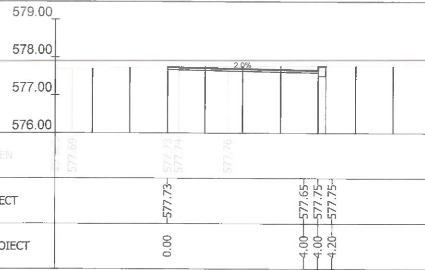
Sectiunea 183 - Km 2+750
