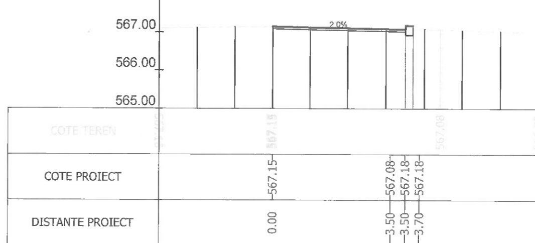
Sectiunea 46 - Km 0+600 Ax-Traseul 3_2
