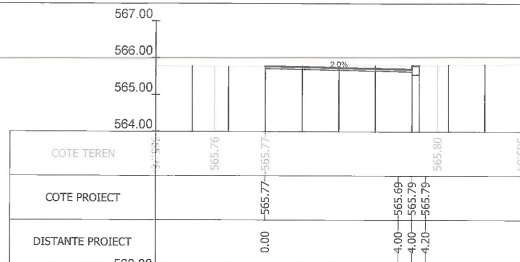
Sectiunea 256 - Km 3+500 Ax-Traseul 1
