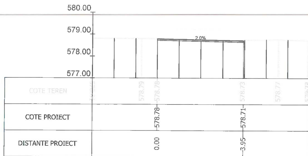
Sectiunea 152 - Km 2+286.877 Ax-Traseul 2
