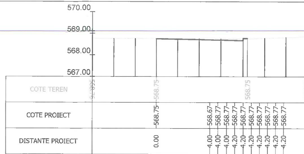
Sectiunea 219 - Km 2+983.257 Ax-Traseul 1
