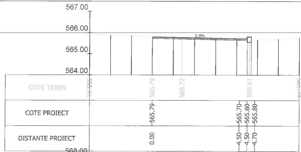
Sectiunea 286 - Km 3+961.401 Ax-Traseul 1
