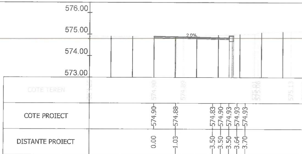
Sectiunea 328 - Km 4+750
