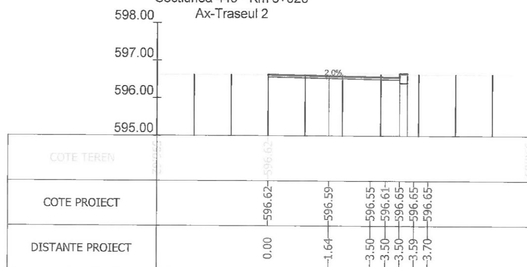
Sectiunea 447 - Km 6+575 Ax-Traseul 2
