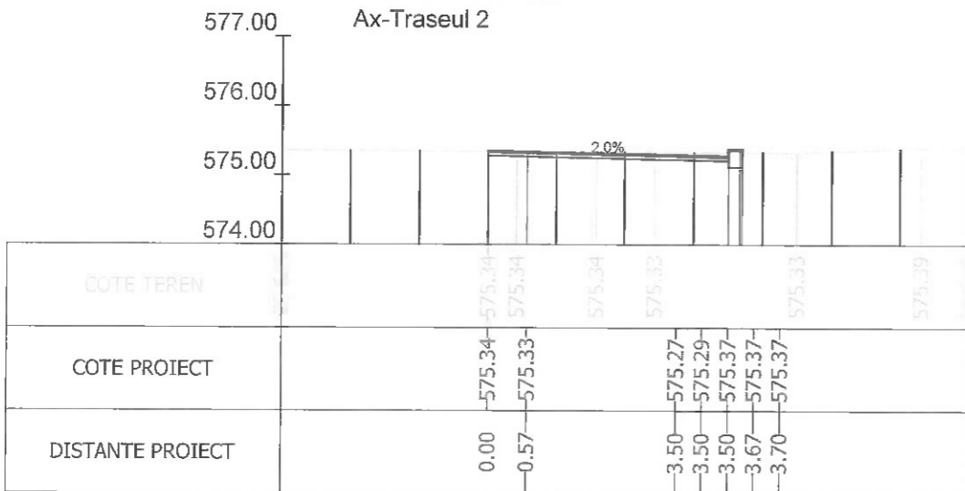
Sectiunea 330 - Km 4+775
