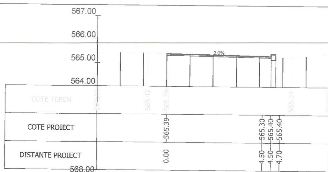
Sectiunea 97 - Km 1+552.215 Ax-Traseul 2
