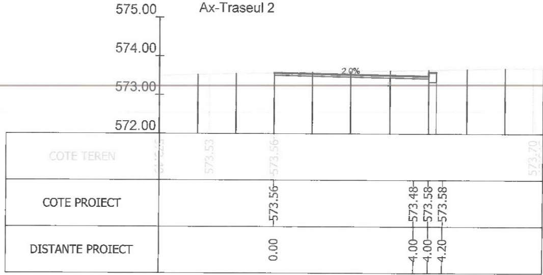
Sectiunea 211 - Km 3+043.647
