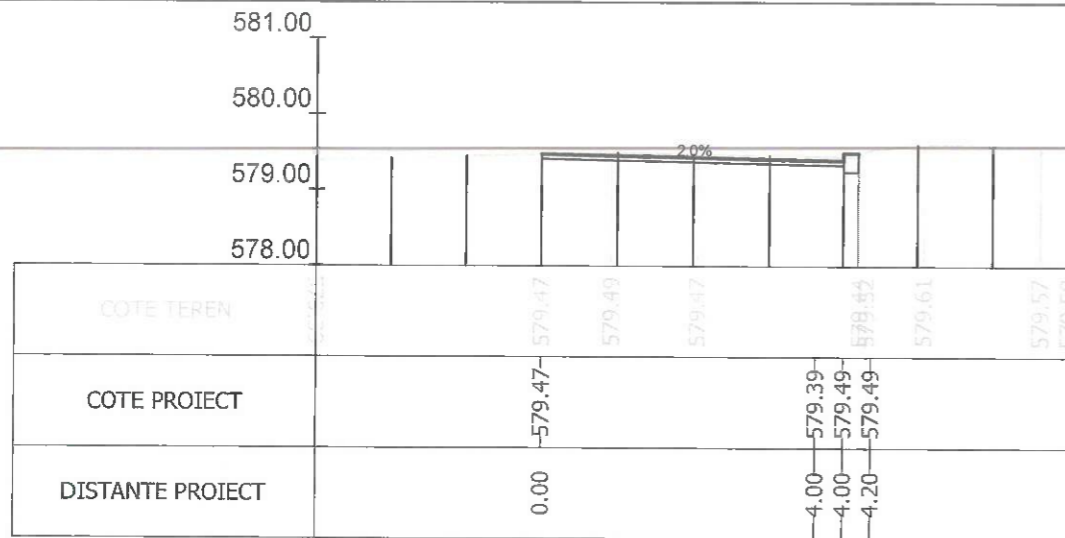
Sectiunea 164 - Km 2+405.719 Ax-Traseul 2
