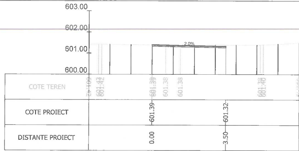
Sectiunea 9 - Km 0+058.875 Ax-Traseul 1
