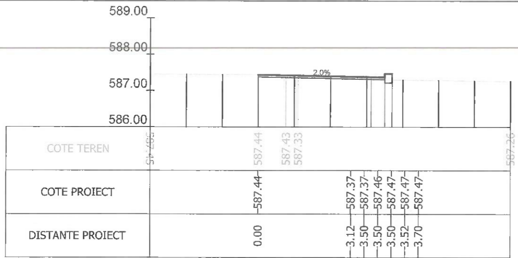
Sectiunea 100 - Km 1+375 Ax-Traseul 1
