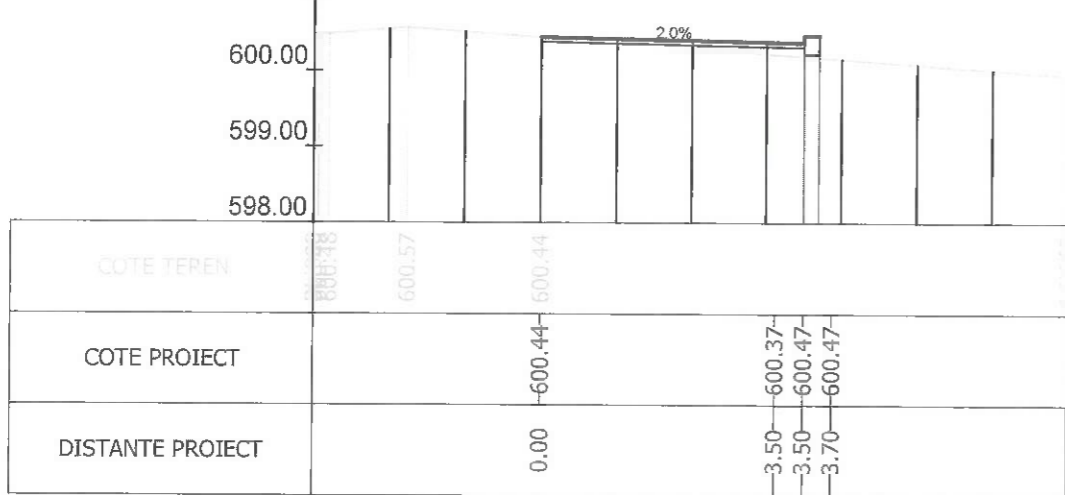
Sectiunea 458 - Km 6+800 Ax-Traseul 2
