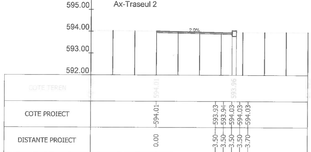
Sectiunea 428 - Km 6+270.412 Ax-Traseul 2
