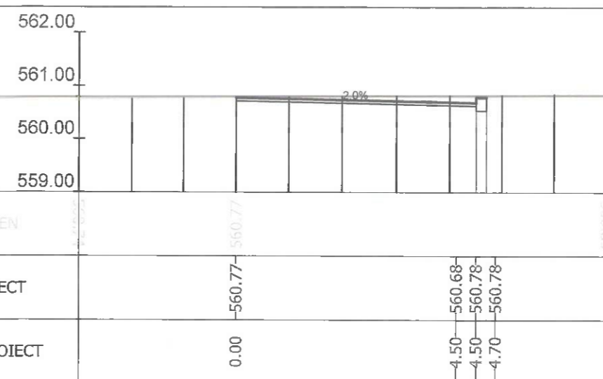
Sectiunea 78 - Km 1+286.630 Ax-Traseul 2
