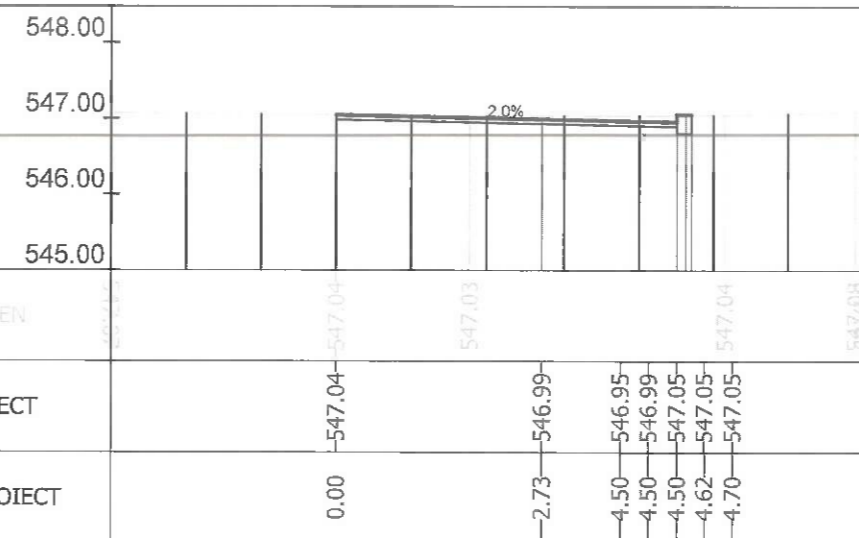
Sectiunea 19 - Km 0+225 Ax-Traseul 2
