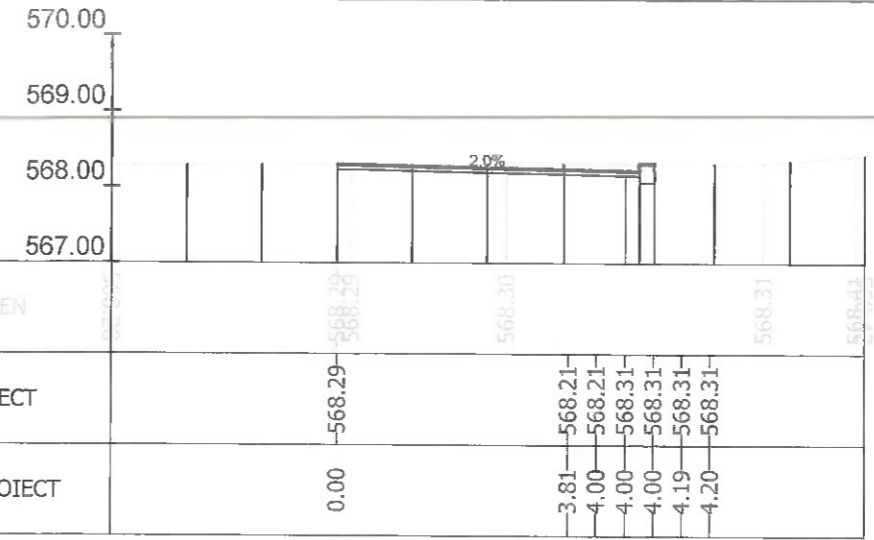
Sectiunea 285 - Km 4+175
