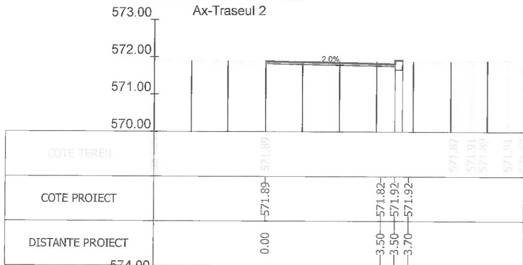
Sectiunea 123 - Km 1+946.315 Ax-Traseul 2
