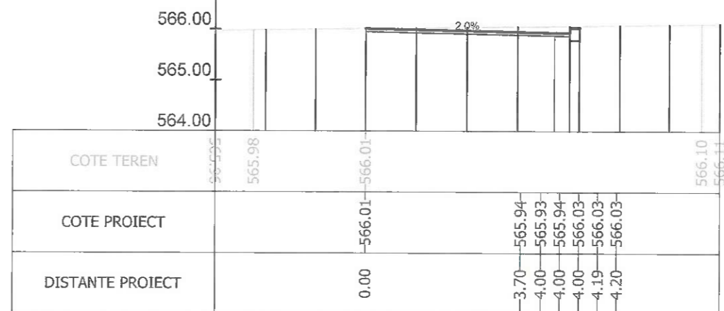
Sectiunea 246 - Km 3+350 Ax-Traseul 1
