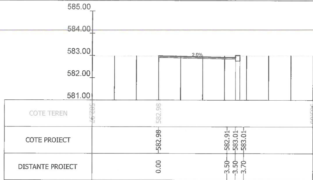
Sectiunea 130 - Km 1+800 Ax-Traseul 1
