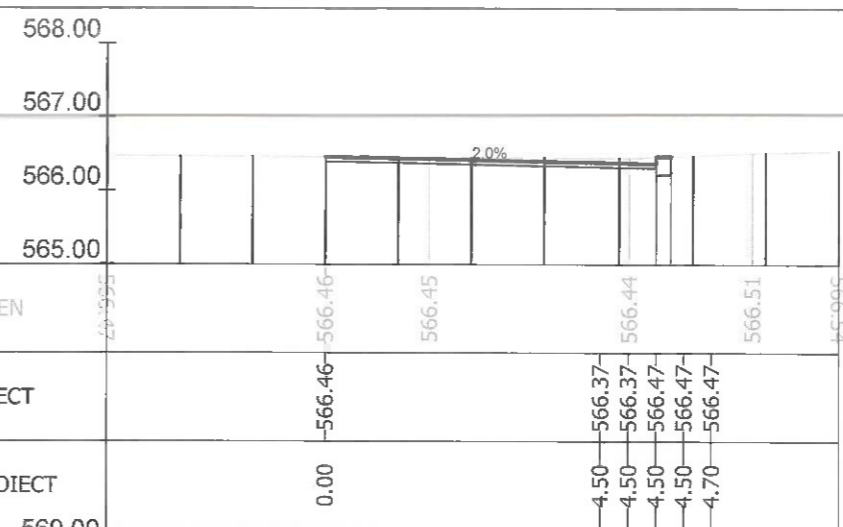
Sectiunea 317 - Km 4+400.843 Ax-Traseul 1
