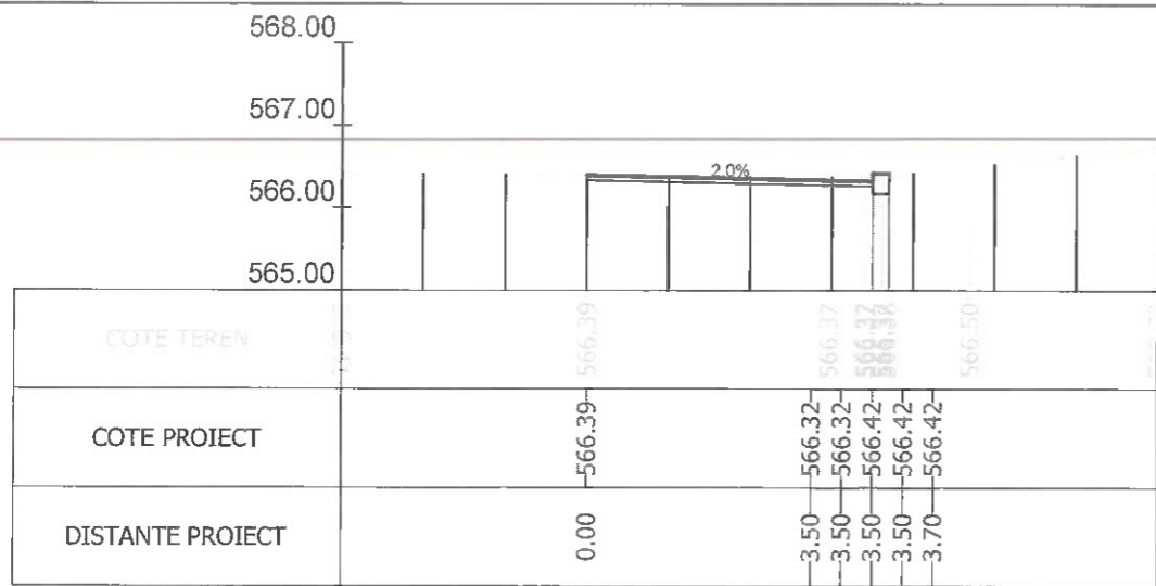
Sectiunea 7 - Km 0+072.264
