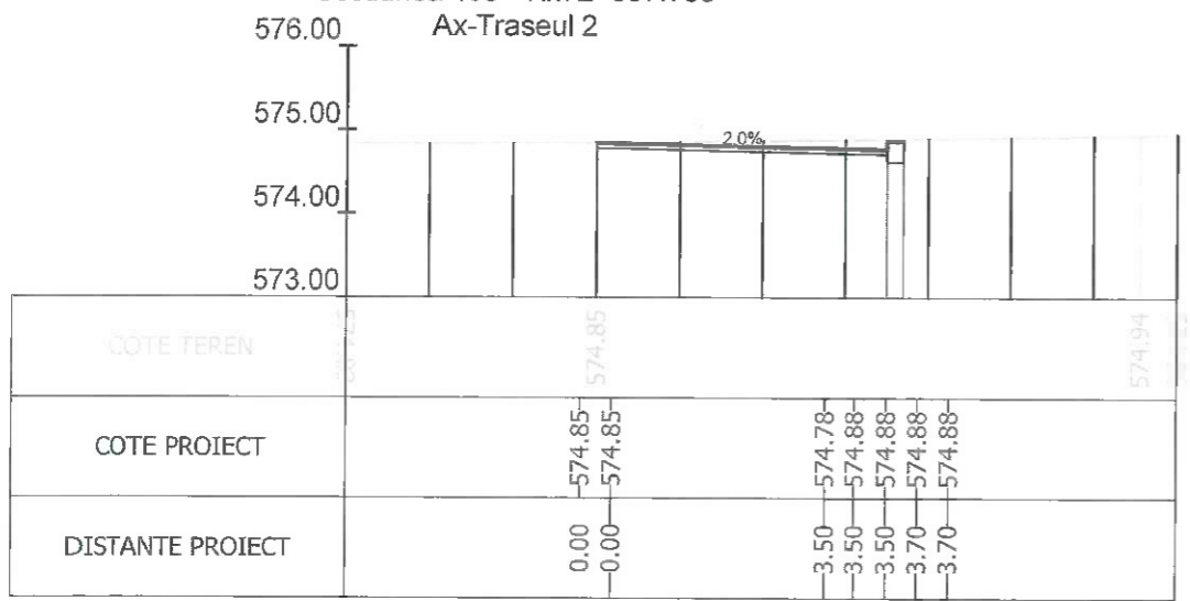
Sectiunea 141 - Km 2+125 Ax-Traseul 2
