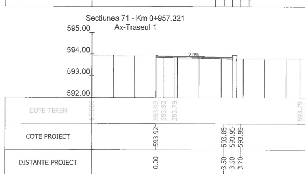
Sectiunea 72 - Km 1+000 Ax-Traseul 1
