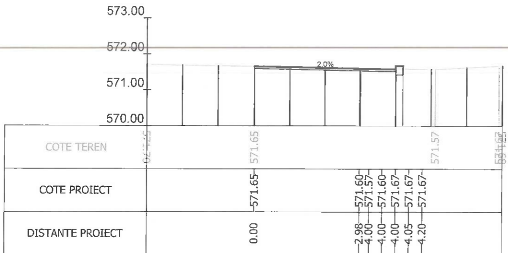
Sectiunea 204 - Km 2+750 Ax-Traseul 1
