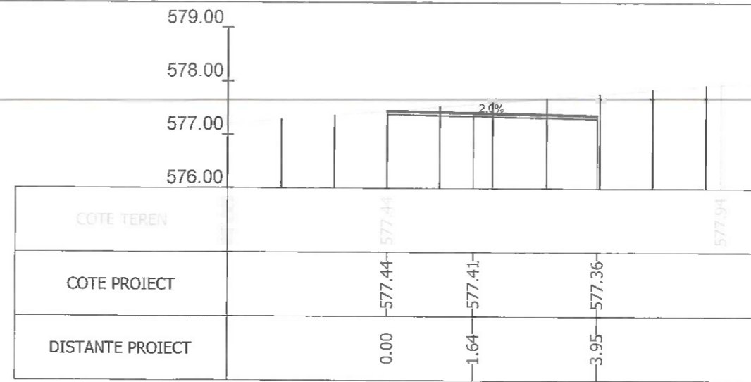
Sectiunea 149 - Km 2+250 Ax-Traseul 2
