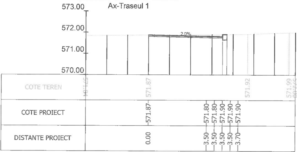
Sectiunea 419 - Km 5+625.756 Ax-Traseul 1
