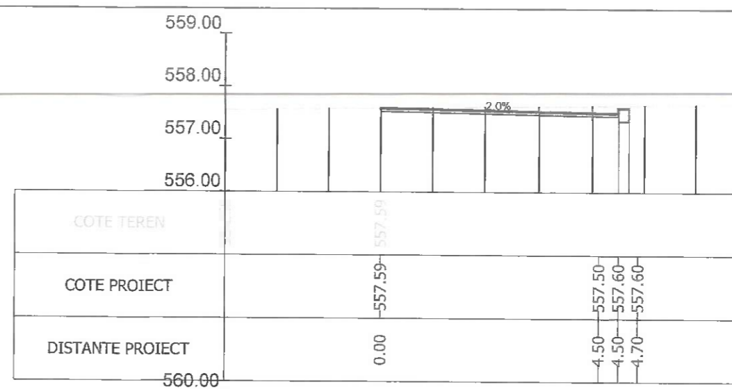
Sectiunea 67 - Km 1+100 Ax-Traseul 2
