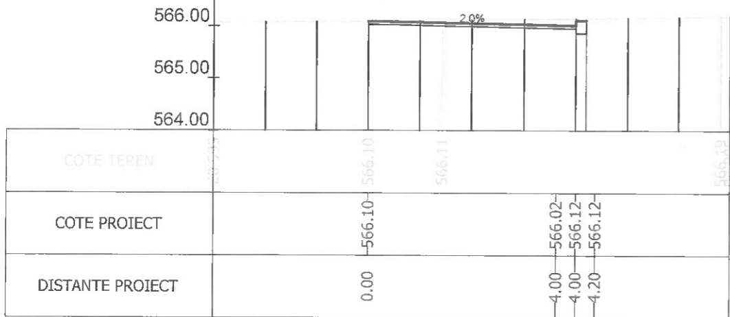
Sectiunea 262 - Km 3+800 Ax-Traseul 2
