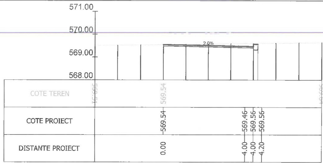
Sectiunea 212 - Km 2+913.633 Ax-Traseul 1
