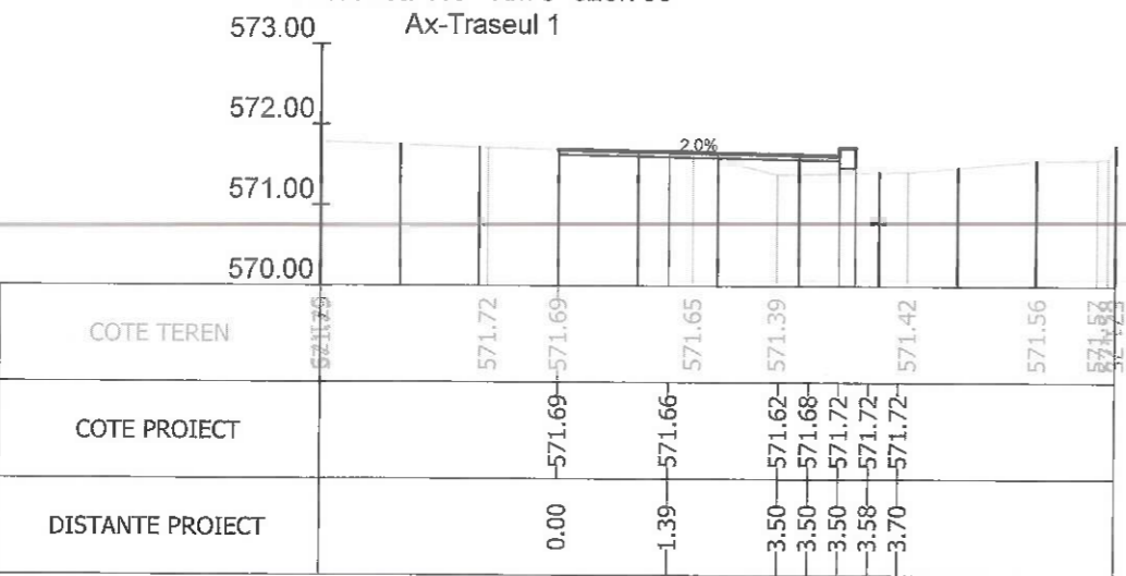
Sectiunea 421 - Km 5+650 Ax-Traseul 1
