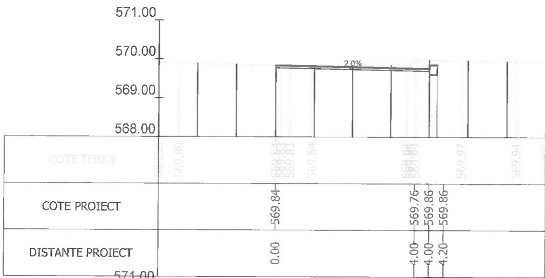
Sectiunea 232 - Km 3+323.229 Ax-Traseul 2
