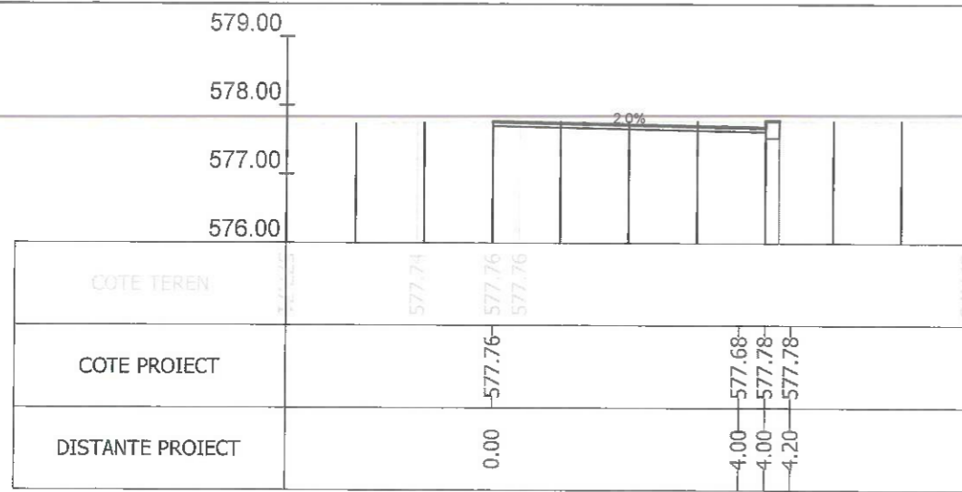
Sectiunea 182 - Km 2+748.133
