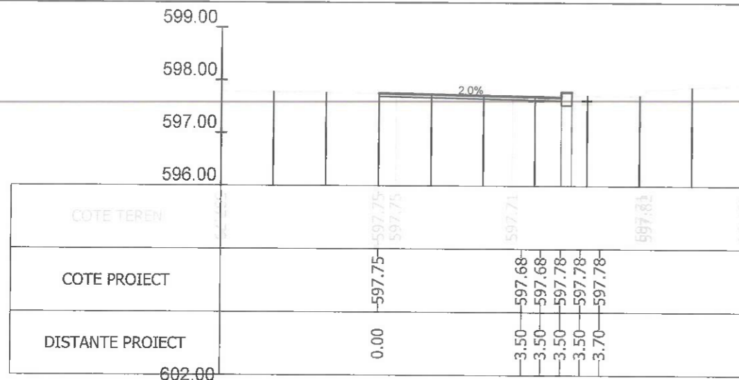
Sectiunea 456 - Km 6+765.747 Ax-Traseul 2
