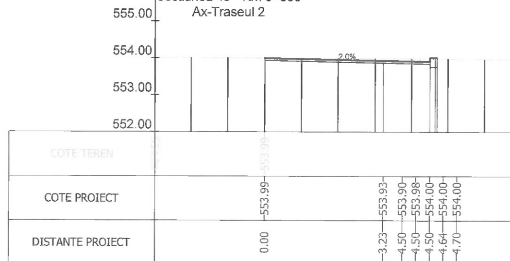
Sectiunea 51 - Km 0+850 Ax-Traseul 2
