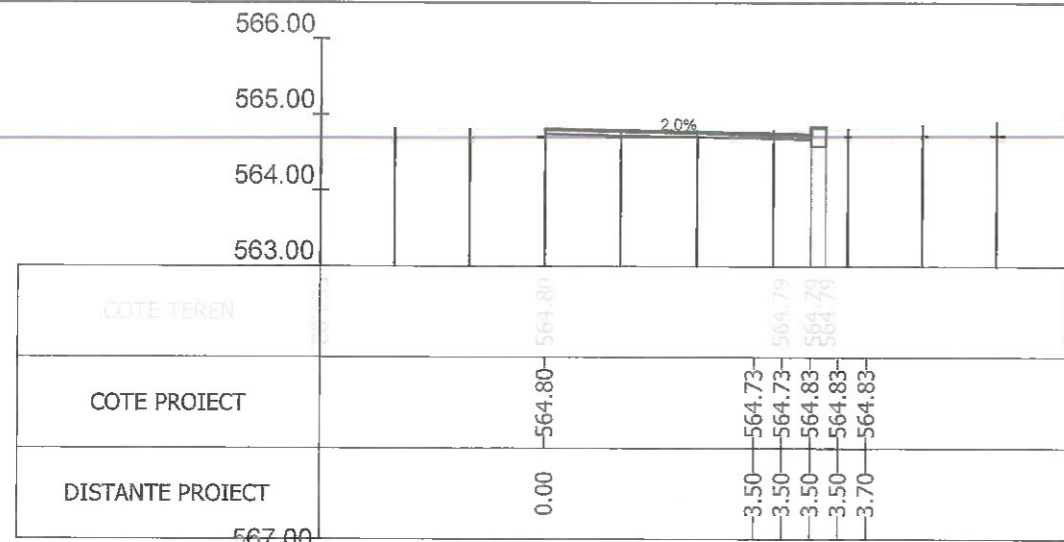
Sectiunea 31 - Km 0+402.090 Ax-Traseul 3_2
