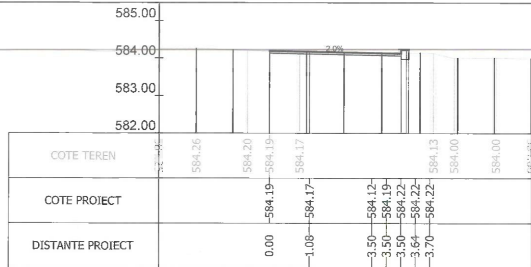
Sectiunea 119 - Km 1+650 Ax-Traseul 1
