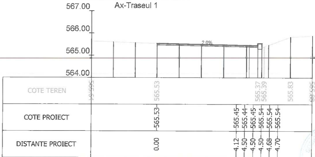
Sectiunea 285 - Km 3+950 Ax-Traseul 1
