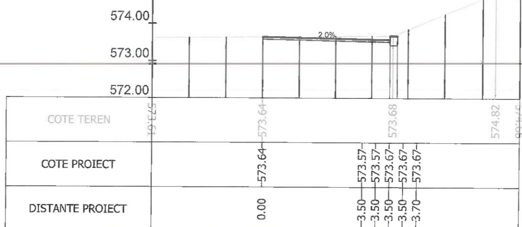
Sectiunea 404 - Km 5+511.245 Ax-Traseul 1
