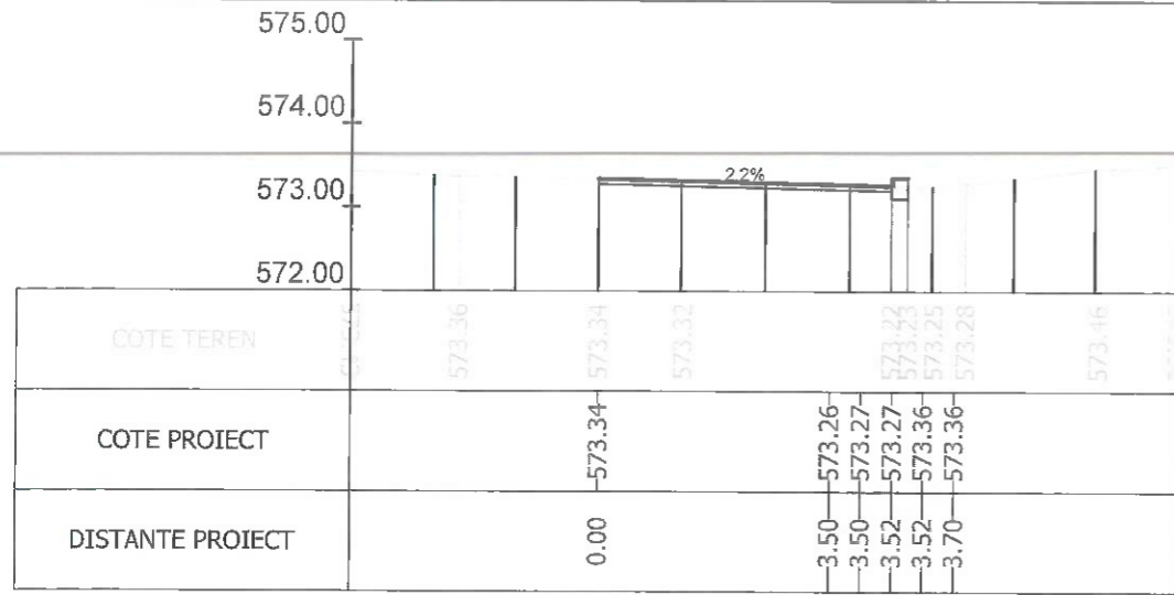
Sectiunea 133 - Km 2+033.664 Ax-Traseul 2
