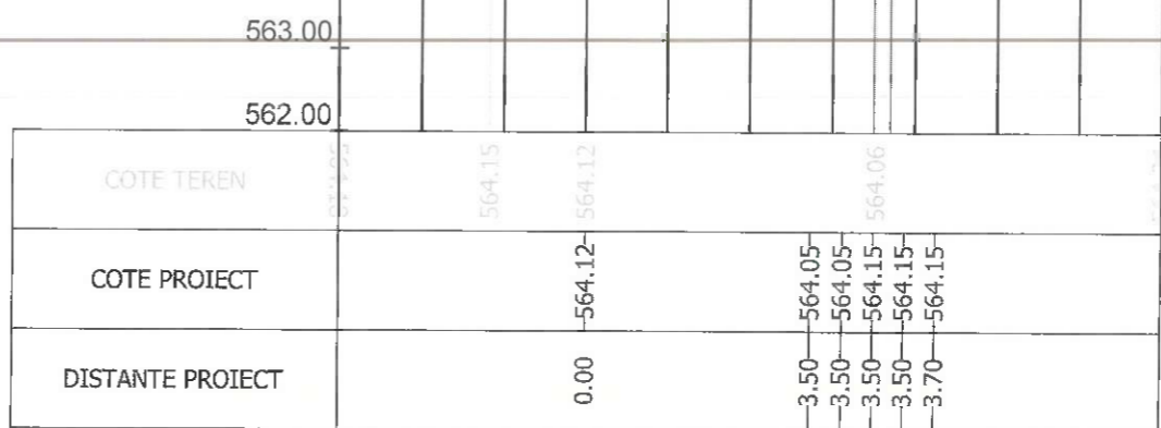
Sectiunea 24 - Km 0+329.038 Ax-Traseul 3_2
