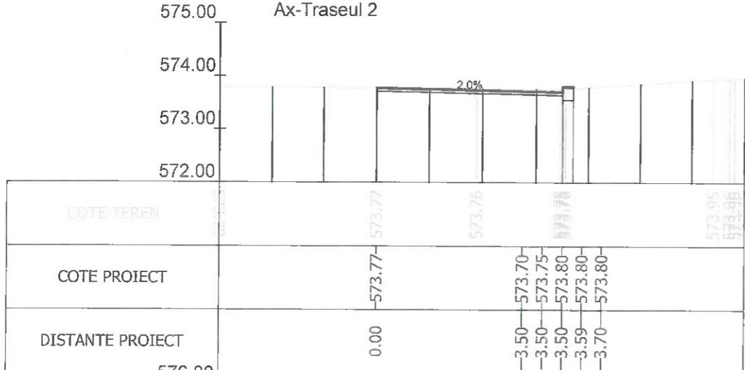
Sectiunea 135 - Km 2+069.815 Ax-Traseul 2
