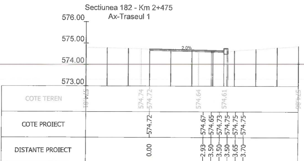
Sectiunea 182 - Km 2+475 Ax-Traseul 1
