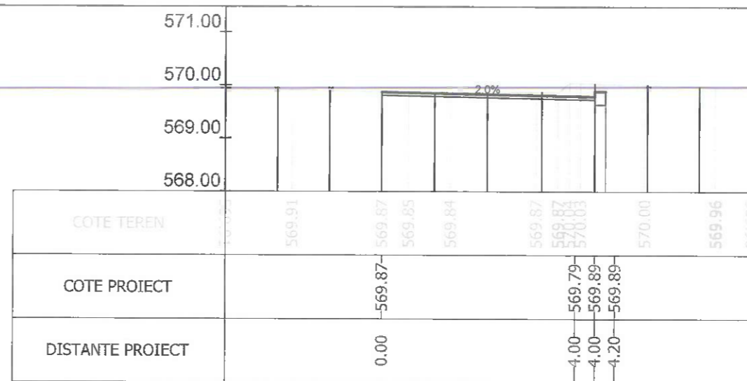
Sectiunea 231 - Km 3+322.572 Ax-Traseul 2
