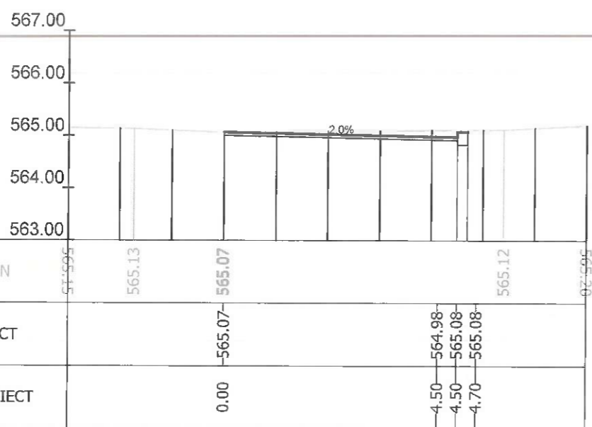
Sectiunea 302 - Km 4+200 Ax-Traseul 1
