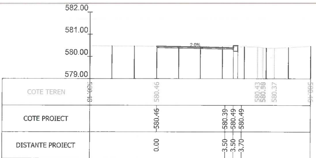
Sectiunea 146 - Km 2+000 Ax-Traseul 1
