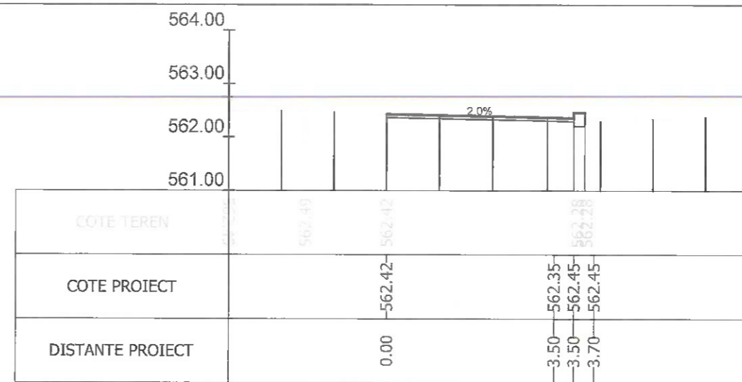
Sectiunea 14 - Km 0+150 Ax-Traseul 3_2
