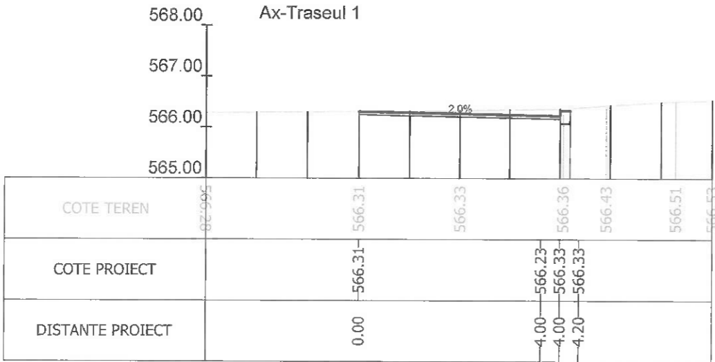
Sectiunea 233 - Km 3+224.601 Ax-Traseul 1
