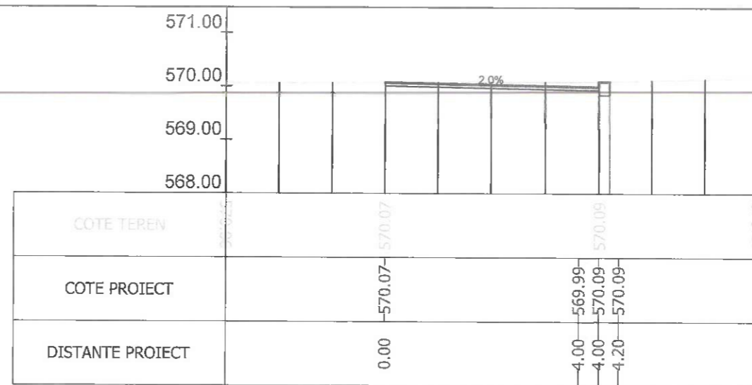
Sectiunea 297 - Km 4+350 Ax-Traseul 2
