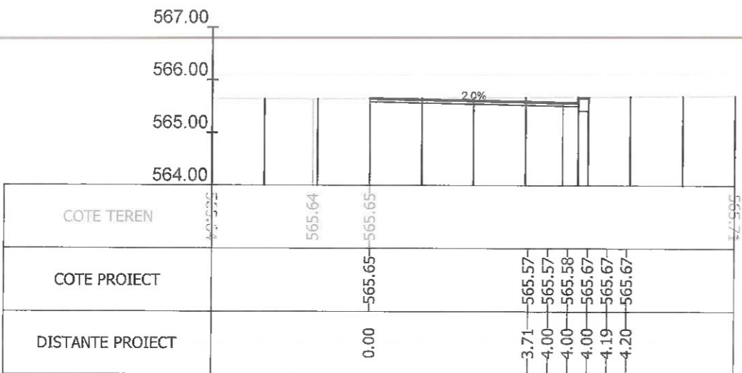
Sectiunea 247 - Km 3+375 Ax-Traseul 1
