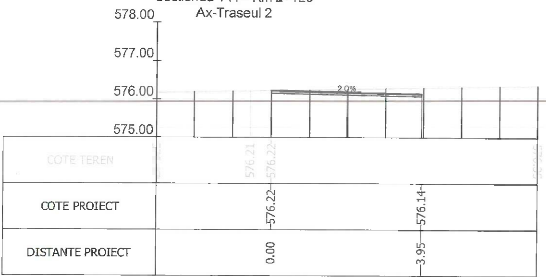
Sectiunea 146 - Km 2+197.733 Ax-Traseul 2
