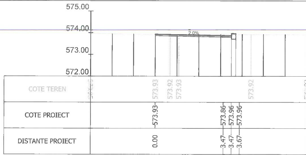
Sectiunea 191 - Km 2+570.241 Ax-Traseul 1
