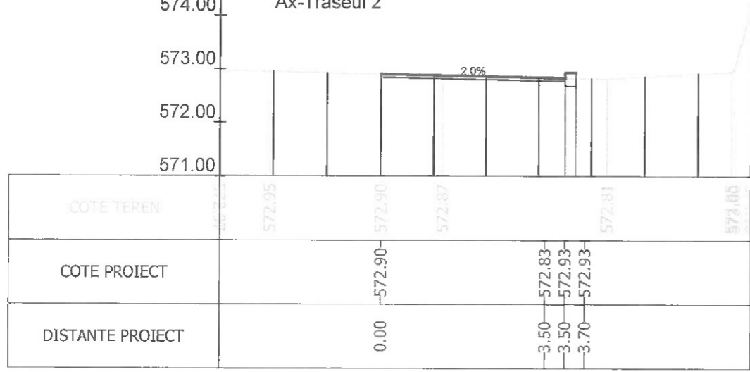
Sectiunea 318 - Km 4+629.848 Ax-Traseul 2
