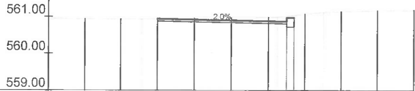
Sectiunea 47 - Km 0+614.021 Ax-Traseul 3_1
