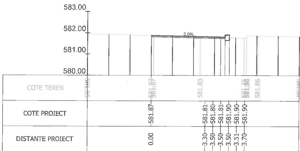
Sectiunea 134 - Km 1+850 Ax-Traseul 1
