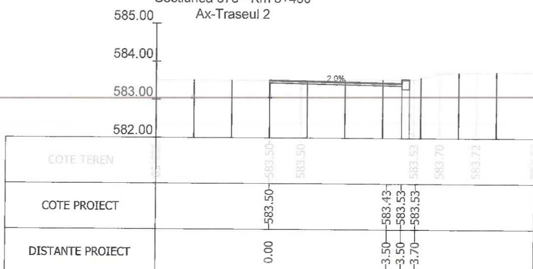
Sectiunea 380 - Km 5+500 Ax-Traseul 2
