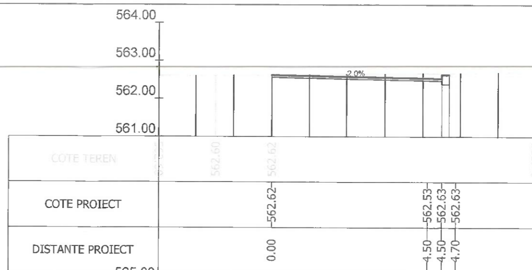
Sectiunea 85 - Km 1+400 Ax-Traseul 2
