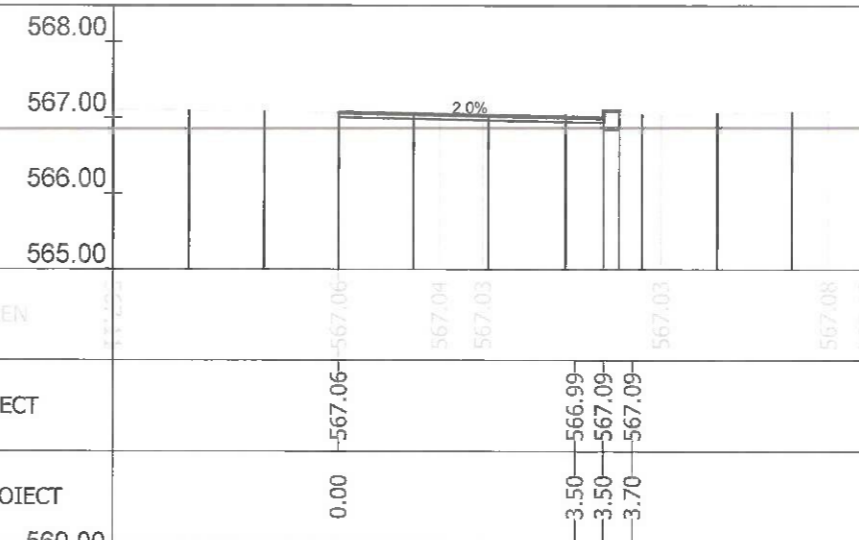
Sectiunea 2 - Km 0+011.721 Ax-Traseul 3_1
