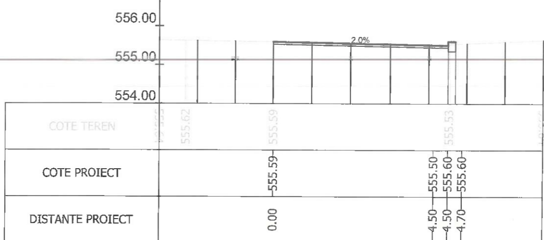
Sectiunea 59 - Km 0+981.838 Ax-Traseul 2
