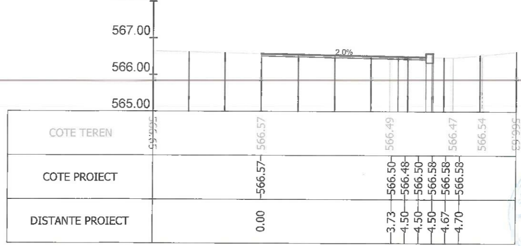
Sectiunea 279 - Km 3+825 Ax-Traseul 1
