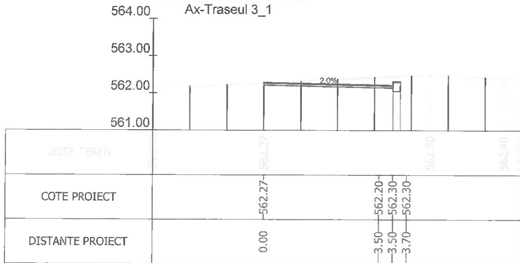
Sectiunea 45 - Km 0+575 Ax-Traseul 3_1
