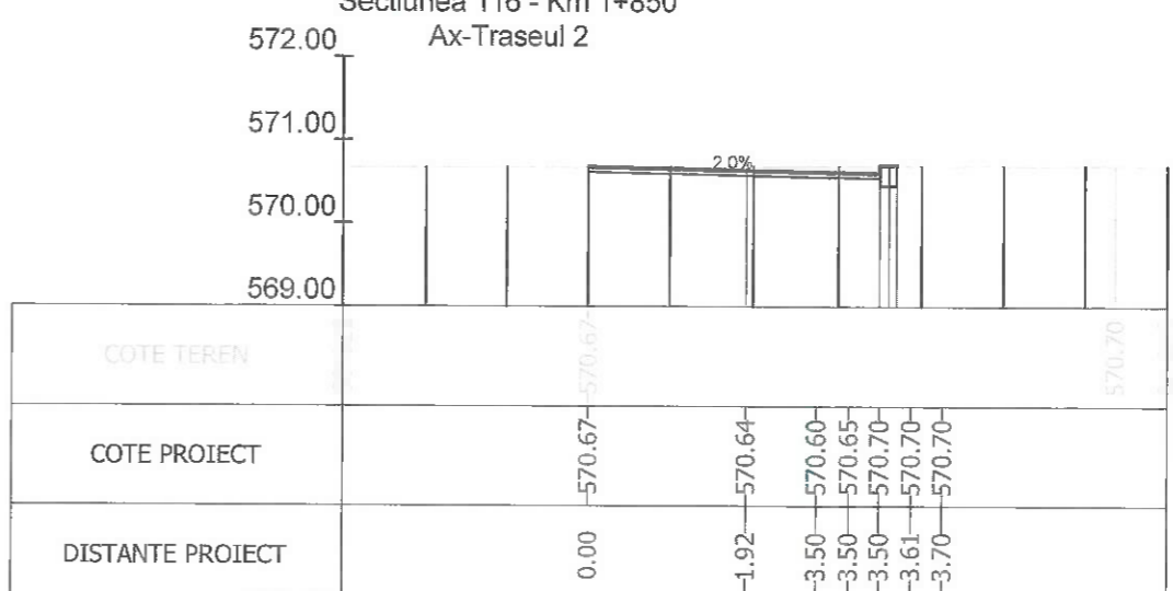
Sectiunea 118 - Km 1+875 Ax-Traseul 2
