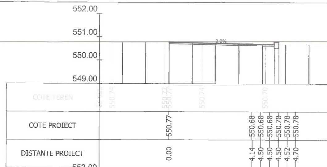
Sectiunea 37 - Km 0+575 Ax-Traseul 2
