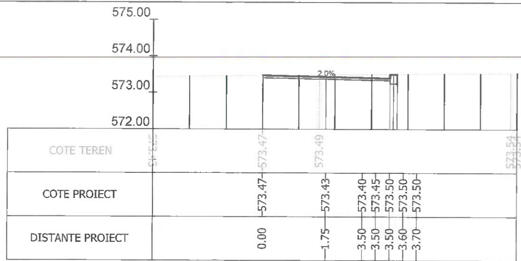
Sectiunea 405 - Km 5+525 Ax-Traseul 1
