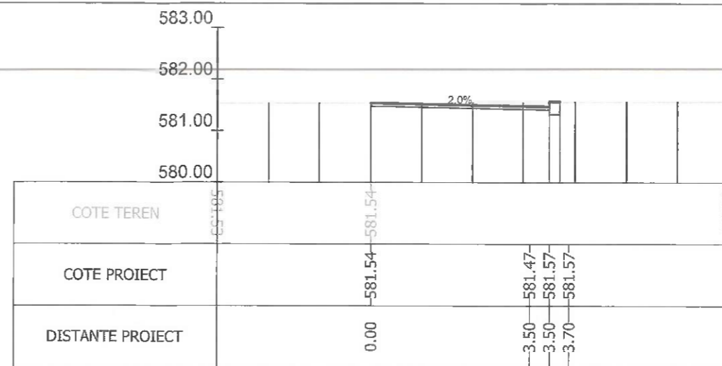
Sectiunea 137 - Km 1+888.153 Ax-Traseul 1
