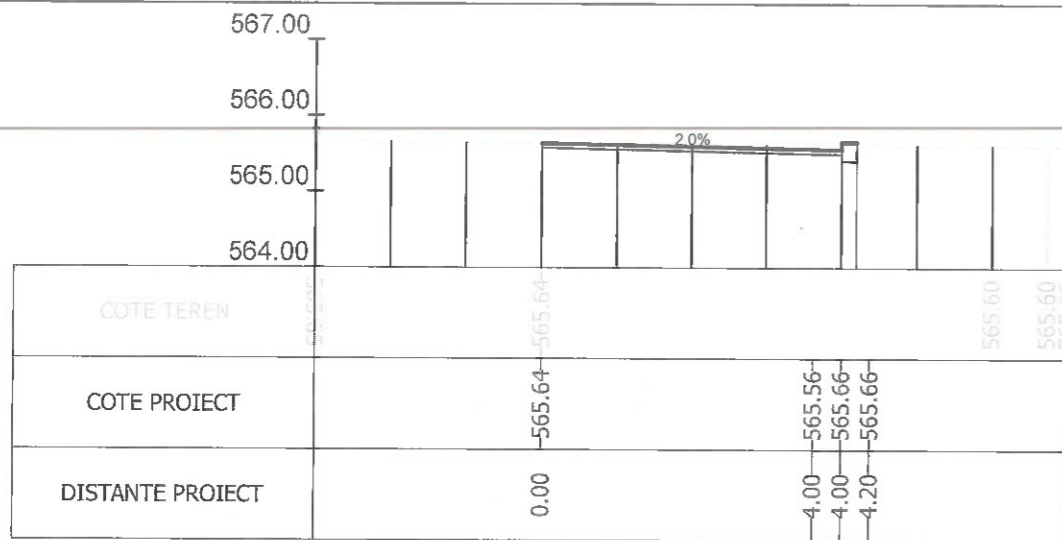
Sectiunea 254 - Km 3+658.462
