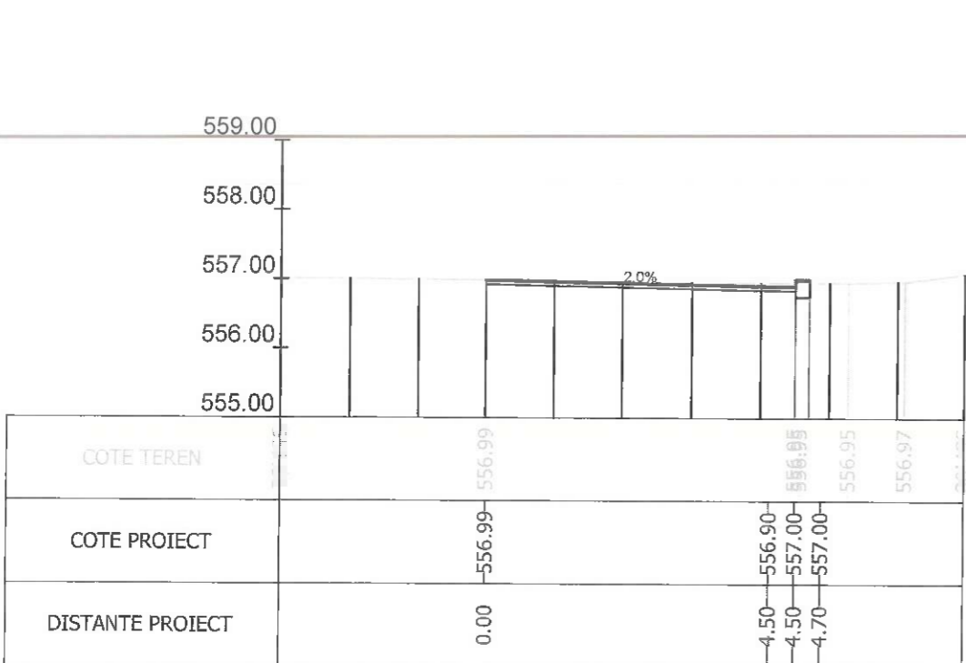
Sectiunea 64 - Km 1+069.109 Ax-Traseul 2
