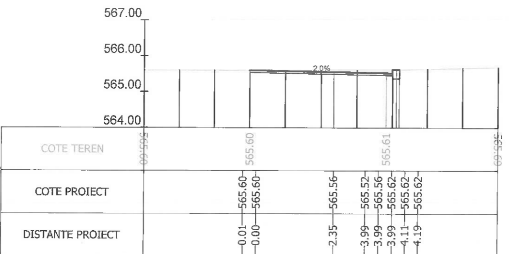
Sectiunea 253 - Km 3+475 Ax-Traseul 1
