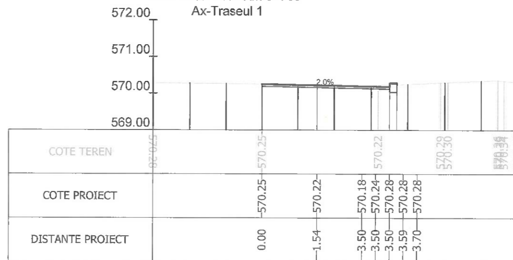
Sectiunea 426 - Km 5+725 Ax-Traseul 1
