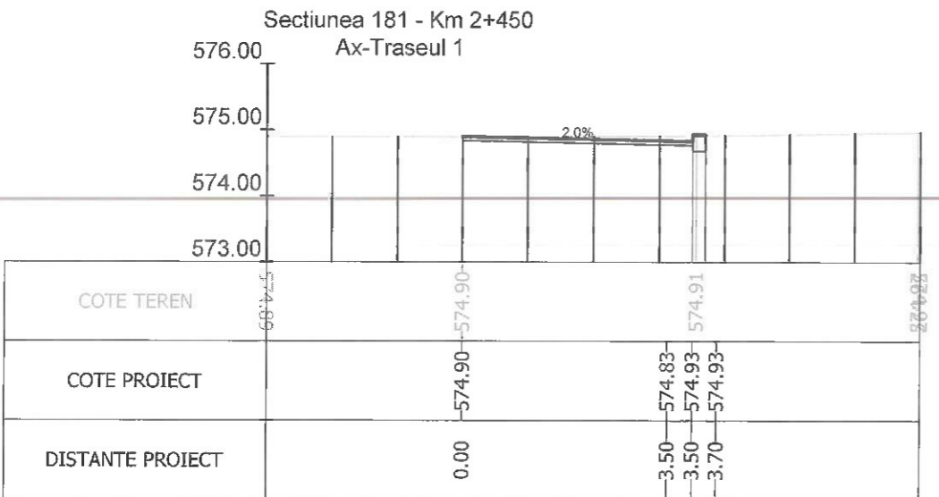
Sectiunea 181 - Km 2+450 Ax-Traseul 1
