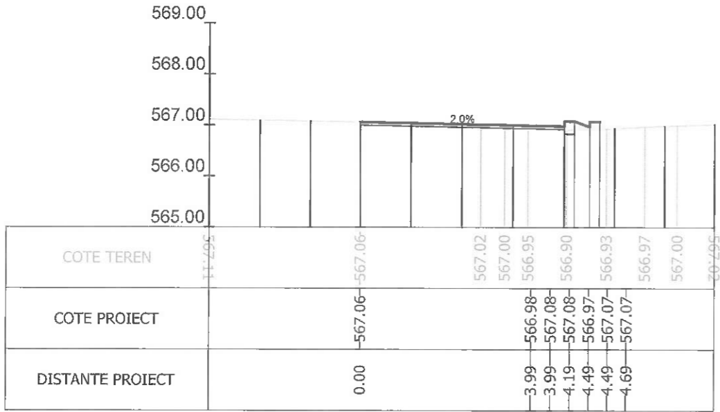
Sectiunea 276 - Km 3+773.896 Ax-Traseul 1
