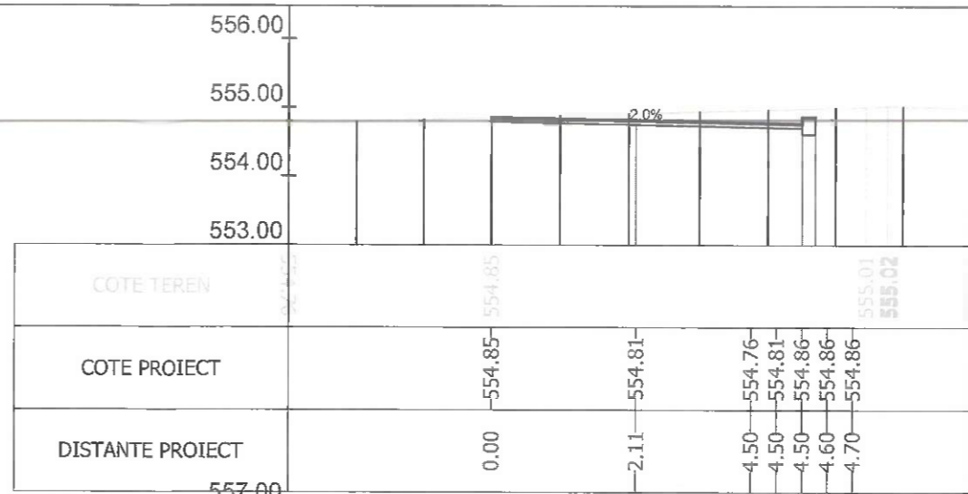
Sectiunea 55 - Km 0+925 Ax-Traseul 2
