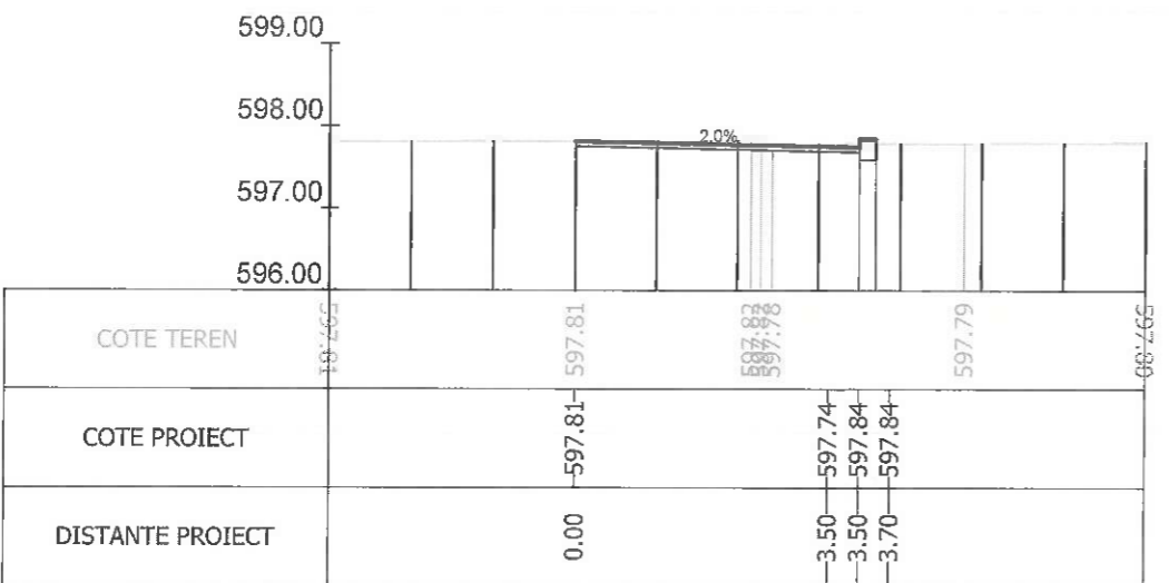
Sectiunea 44 - Km 0+500 Ax-Traseul 1
