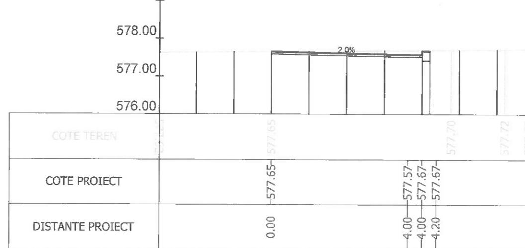
Sectiunea 185 - Km 2+757.157
