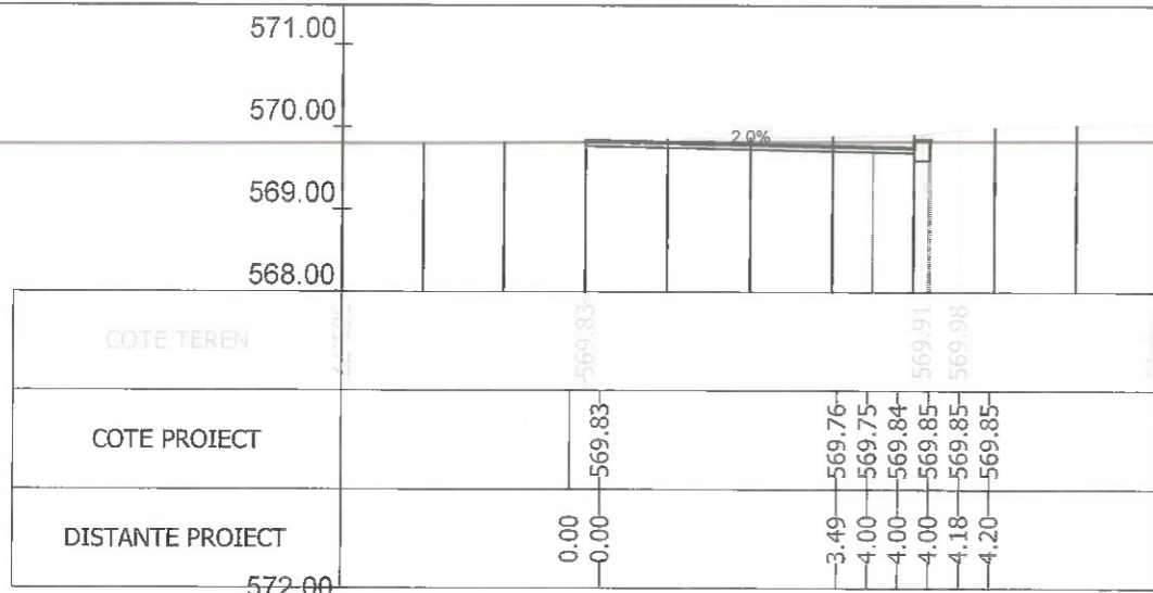
Sectiunea 296 - Km 4+325 Ax-Traseul 2
