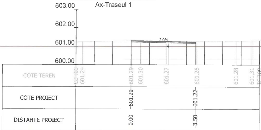
Sectiunea 13 - Km 0+075 Ax-Traseul 1
