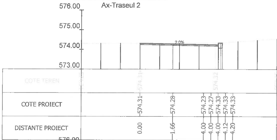
Sectiunea 206 - Km 2+955.677
