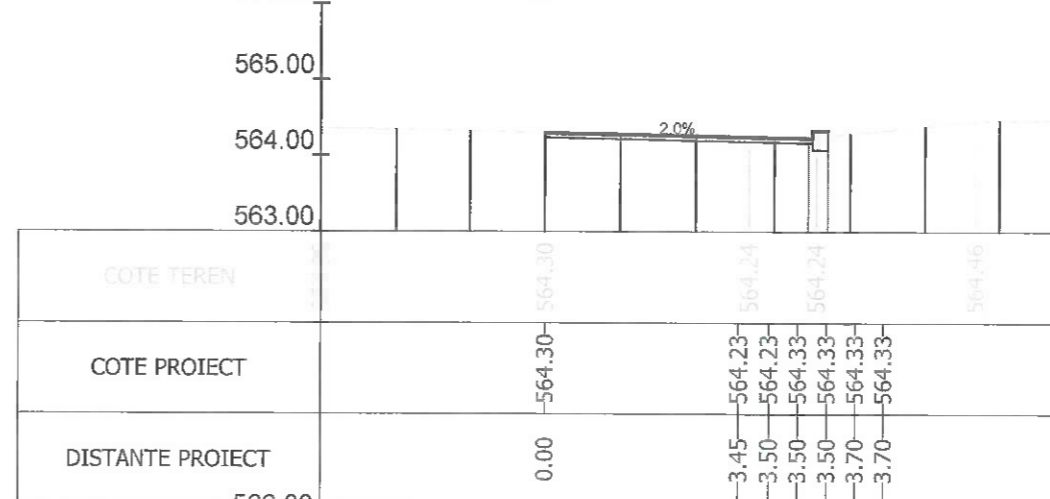
Sectiunea 22 - Km 0+283.608 Ax-Traseul 3_1
