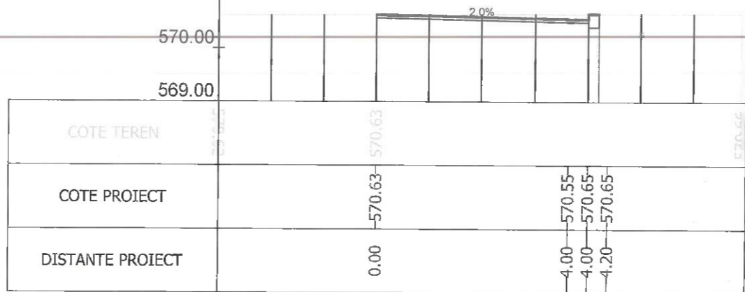
Sectiunea 301 - Km 4+400
