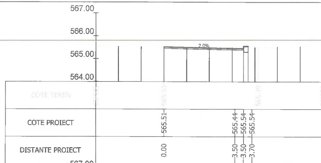
Sectiunea 14 - Km 0+175 Ax-Traseul 3_1
