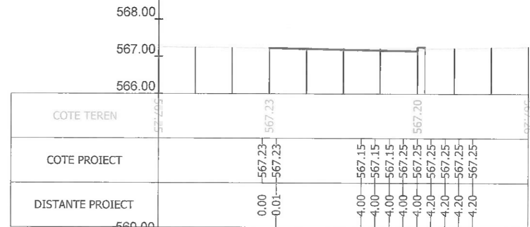
Sectiunea 227 - Km 3+100.533 Ax-Traseul 1
