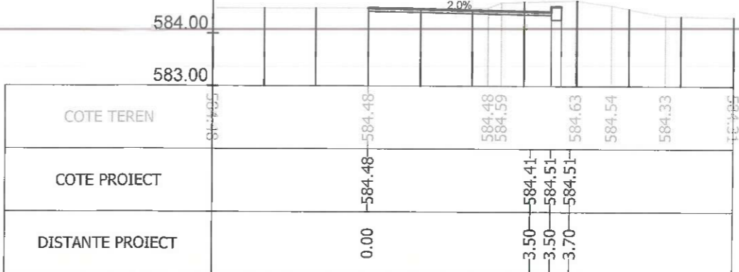
Sectiunea 117 - Km 1+638.111 Ax-Traseul 1
