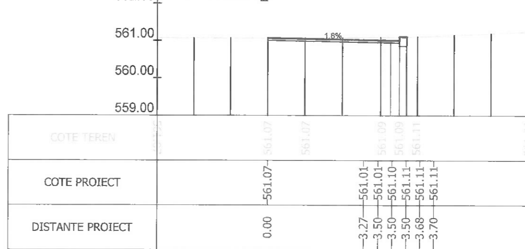
Sectiunea 4 - Km 0+021.847 Ax-Traseul 3_2
