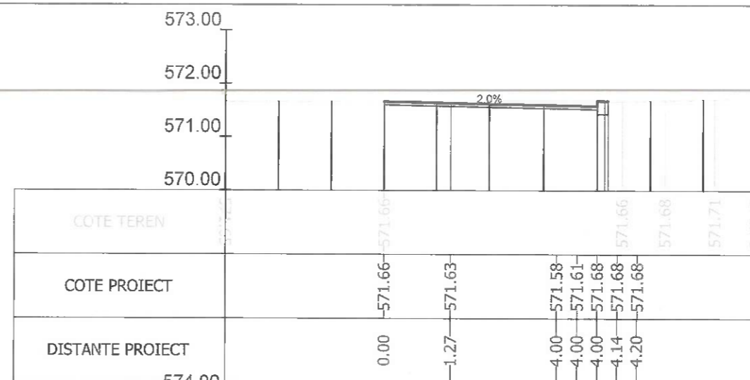
Sectiunea 309 - Km 4+550
