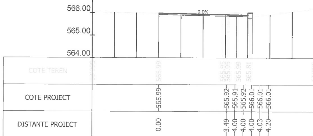
Sectiunea 263 - Km 3+825 Ax-Traseul 2
