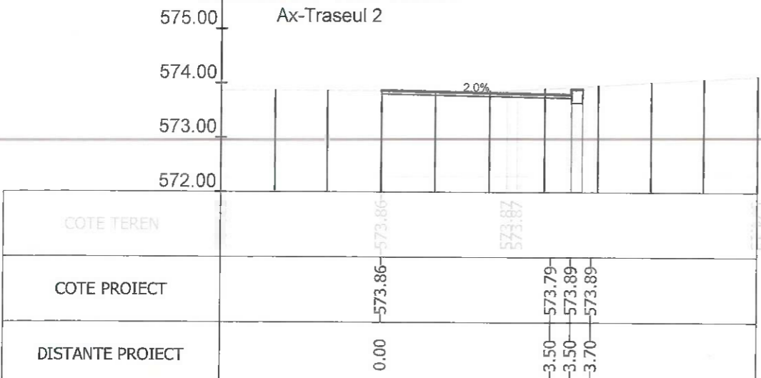
Sectiunea 137 - Km 2+080.207 Ax-Traseul 2
