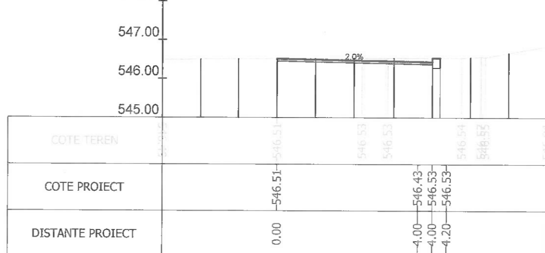
Sectiunea 6 - Km 0+100 Ax-Traseul 2
