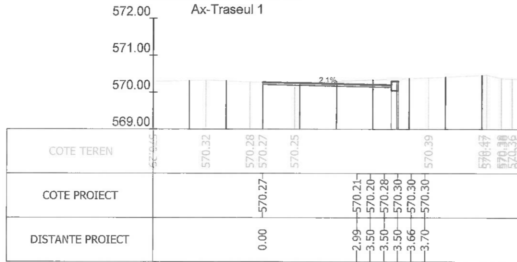
Sectiunea 425 - Km 5+719.664 Ax-Traseul 1
