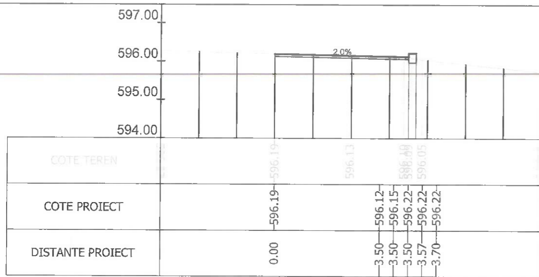
Sectiunea 444 - Km 6+511.550 Ax-Traseul 2
