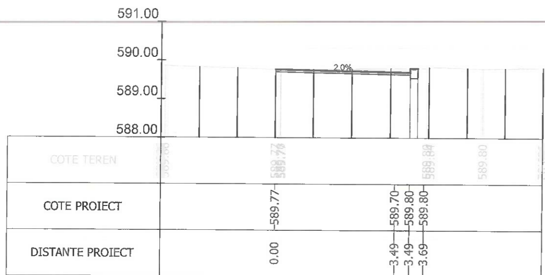
Sectiunea 408 - Km 5+975 Ax-Traseul 2
