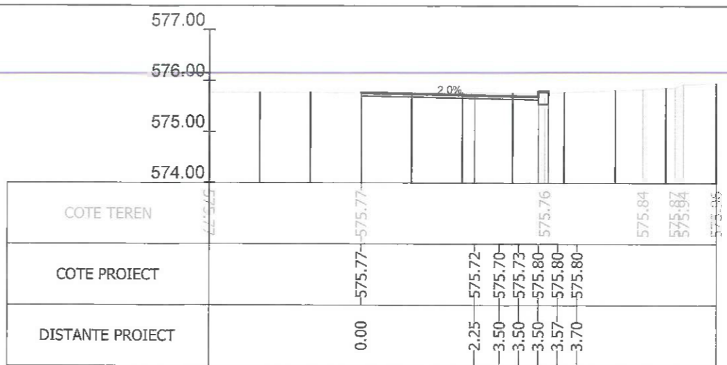
Sectiunea 180 - Km 2+425 Ax-Traseul 1
