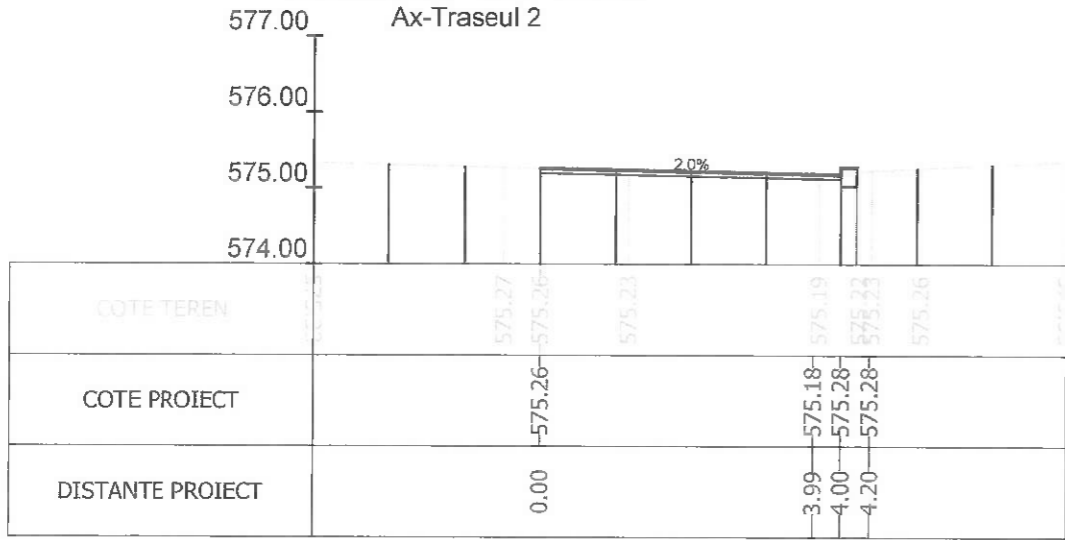
Sectiunea 202 - Km 2+902.252
