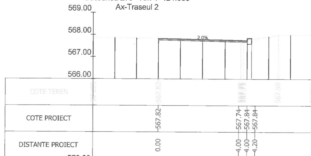
Sectiunea 281 - Km 4+125.916
