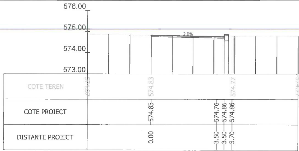
Sectiunea 185 - Km 2+518.366 Ax-Traseul 1
