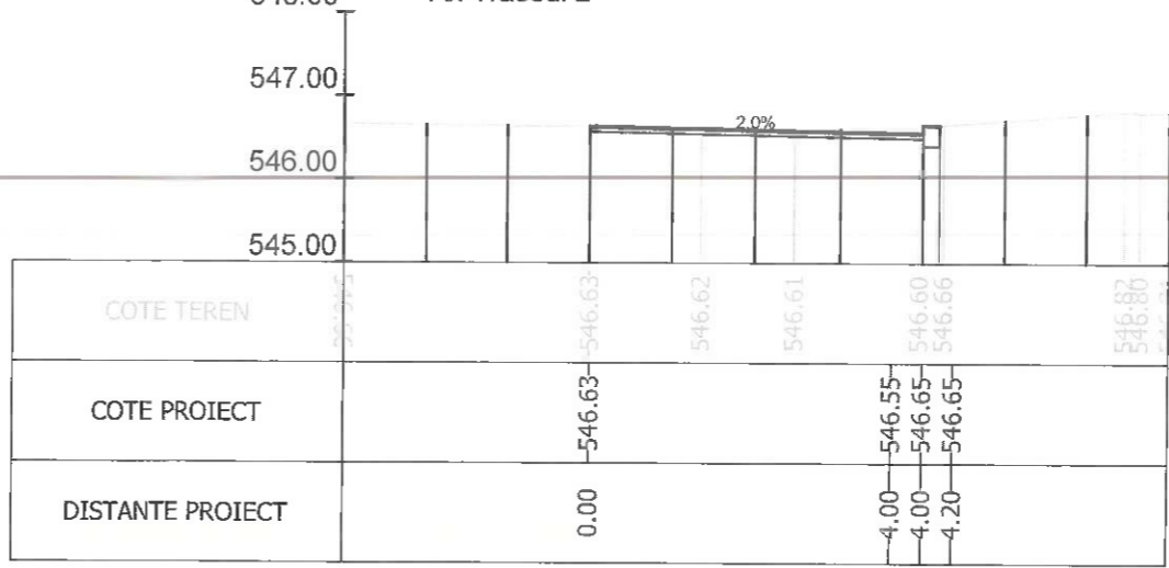
Sectiunea 8 - Km 0+127.604 Ax-Traseul 2
