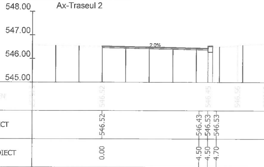
Sectiunea 14 - Km 0+151.794
