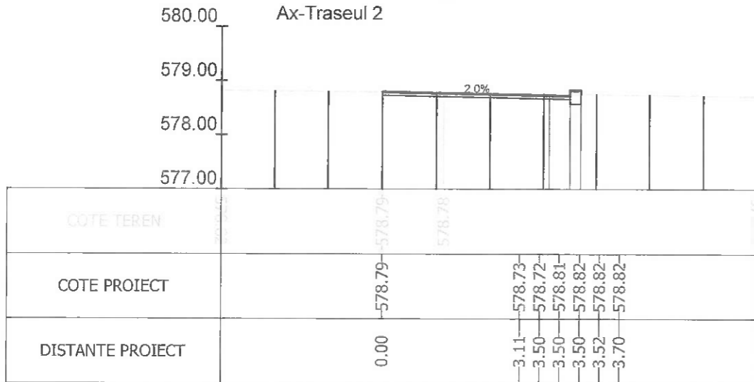
Sectiunea 348 - Km 5+075
