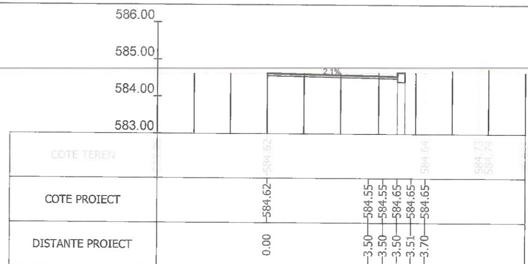
Sectiunea 388 - Km 5+608.639 Ax-Traseul 2
