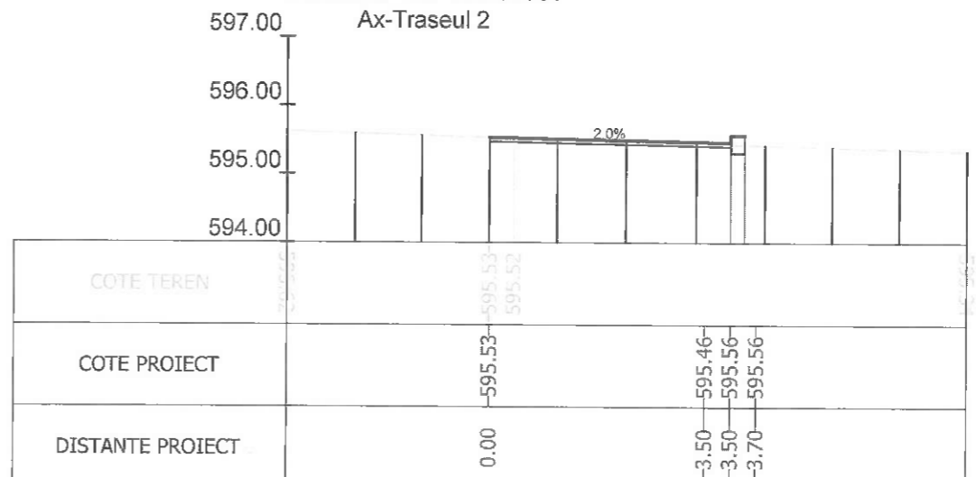
Sectiunea 434 - Km 6+375 Ax-Traseul 2
