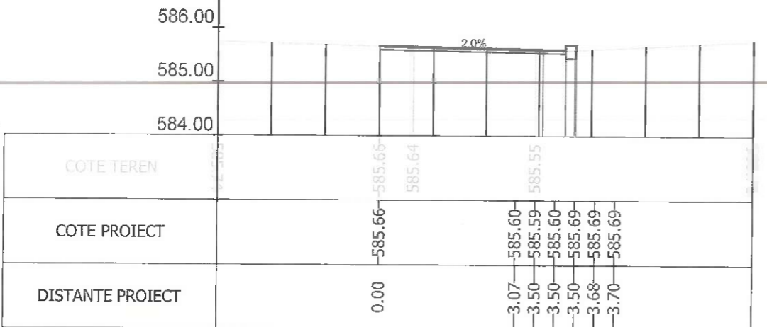
Sectiunea 391 - Km 5+675 Ax-Traseul 2
