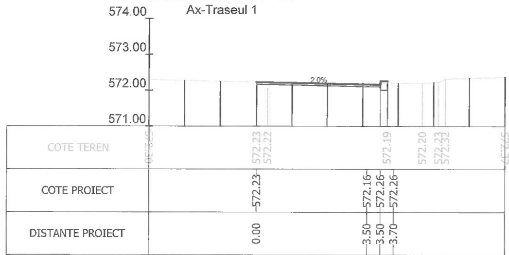
Sectiunea 202 - Km 2+700 Ax-Traseul 1
