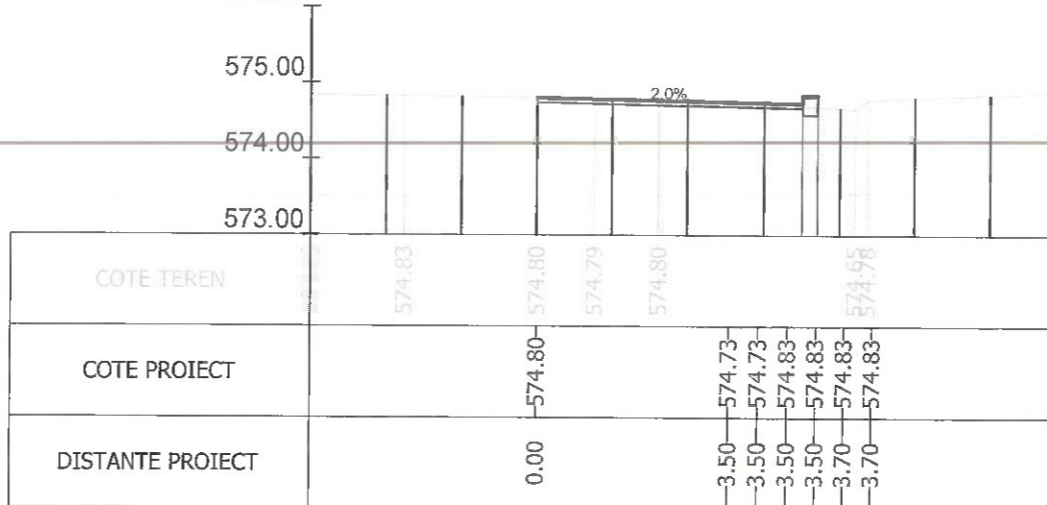
Sectiunea 327 - Km 4+734.073
