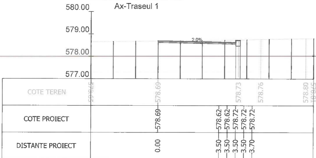
Sectiunea 165 - Km 2+185.455 Ax-Traseul 1
