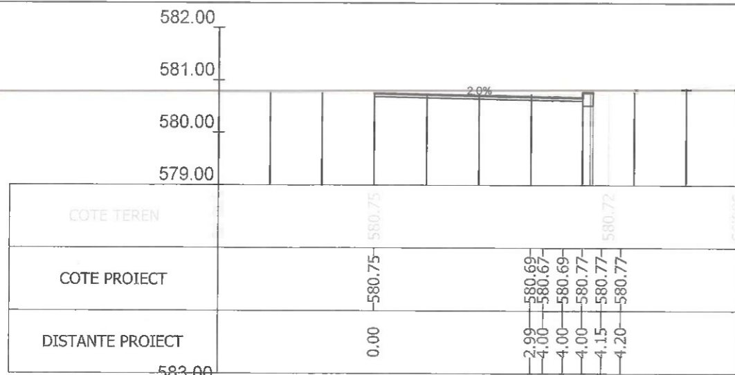
Sectiunea 363 - Km 5+275 Ax-Traseul 2
