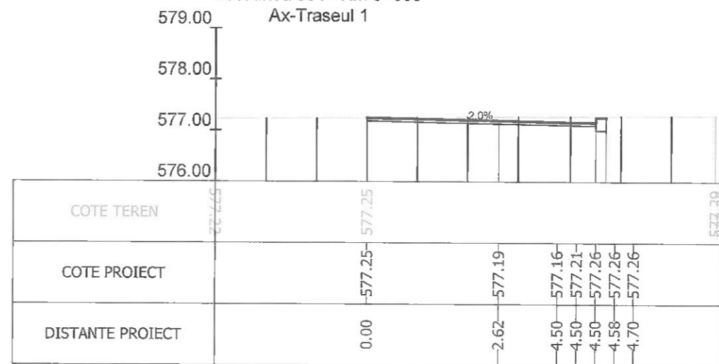
Sectiunea 386 - Km 5+325 Ax-Traseul 1
