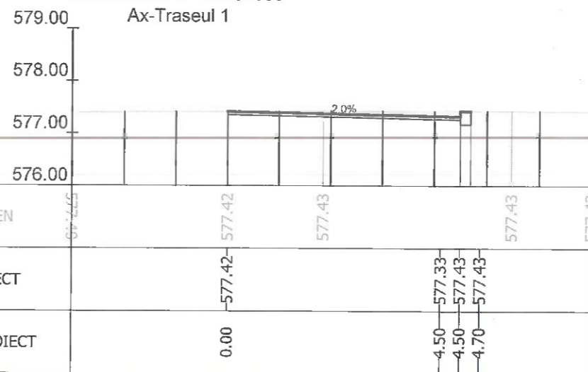
Sectiunea 375 - Km 5+075 Ax-Traseul 1
