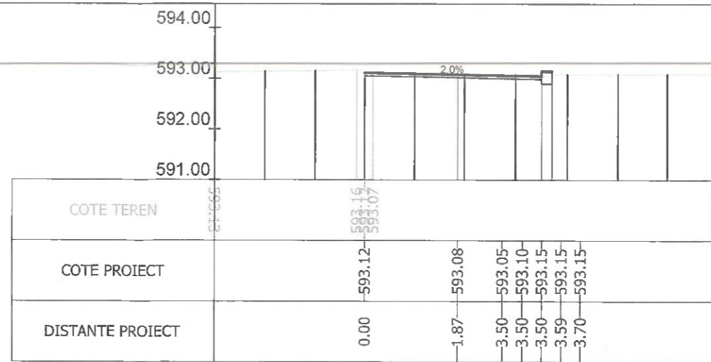
Sectiunea 77 - Km 1+050 Ax-Traseul 1
