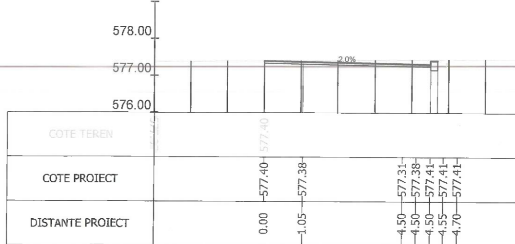
Sectiunea 187 - Km 2+775
