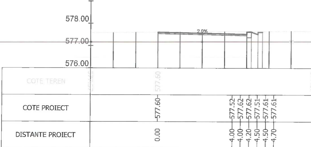
Sectiunea 186 - Km 2+762.659
