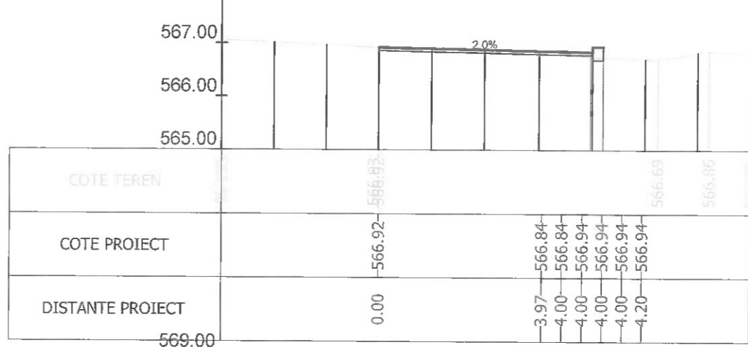
Sectiunea 269 - Km 3+950 Ax-Traseul 2
