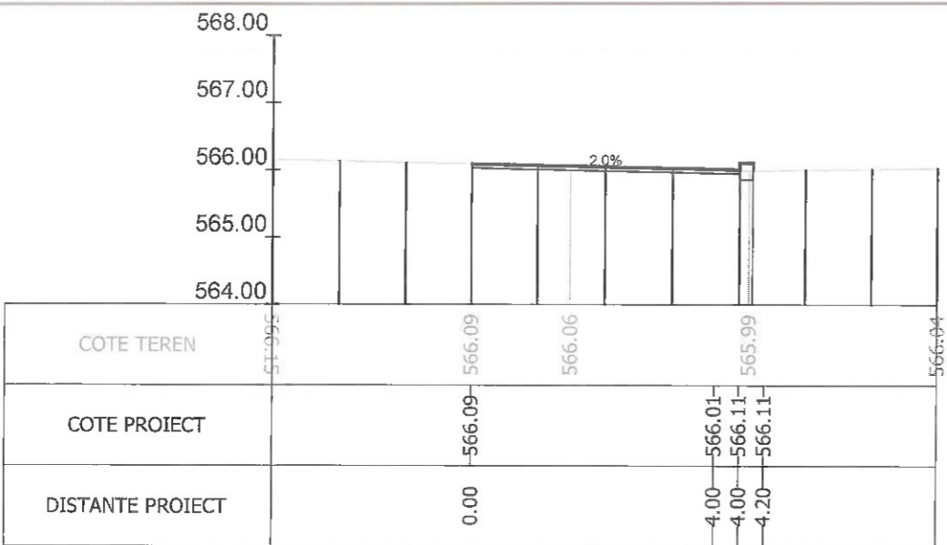
Sectiunea 260 - Km 3+567.349 Ax-Traseul 1
