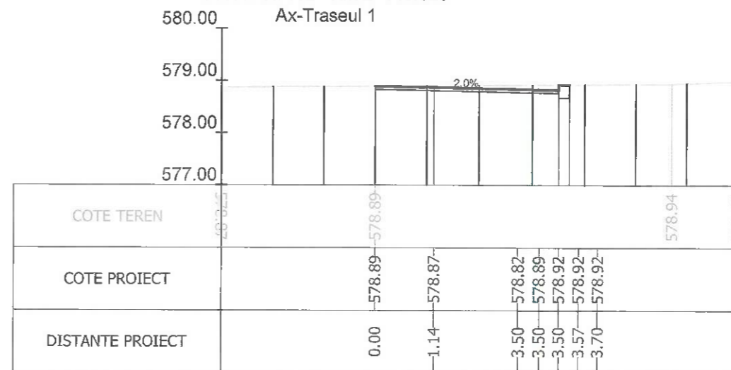
Sectiunea 164 - Km 2+175 Ax-Traseul 1
