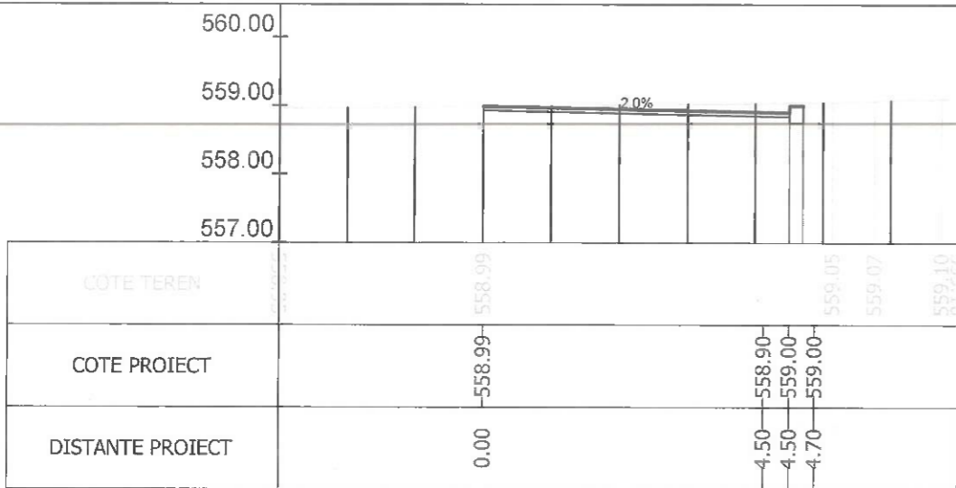
Sectiunea 72 - Km 1+187.376 Ax-Traseul 2
