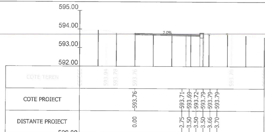
Sectiunea 427 - Km 6+250 Ax-Traseul 2
