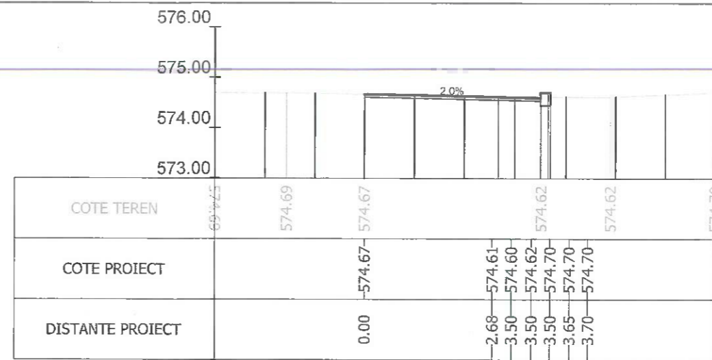
Sectiunea 186 - Km 2+525 Ax-Traseul 1
