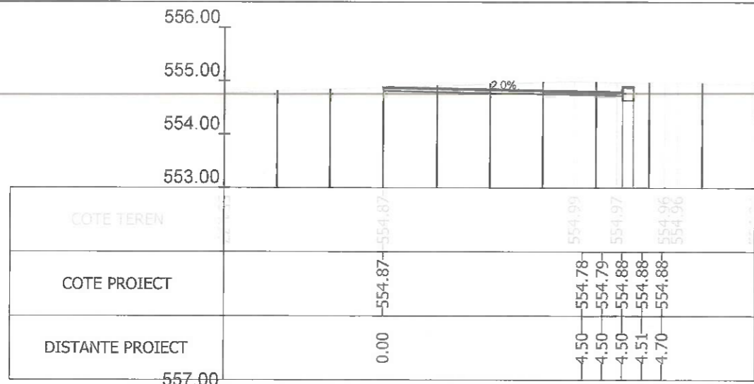
Sectiunea 54 - Km 0+921.617 Ax-Traseul 2
