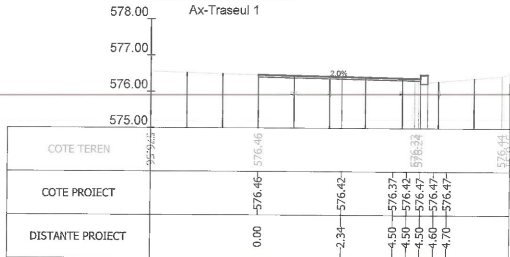
Sectiunea 388 - Km 5+375 Ax-Traseul 1
