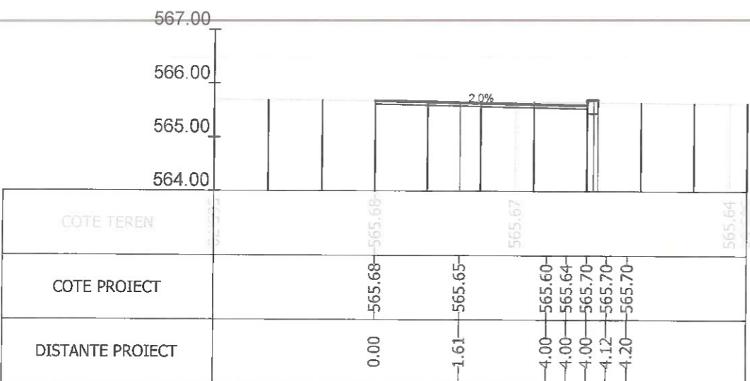
Sectiunea 252 - Km 3+650 Ax-Traseul 2
