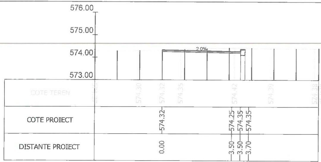
Sectiunea 139 - Km 2+097.753 Ax-Traseul 2
