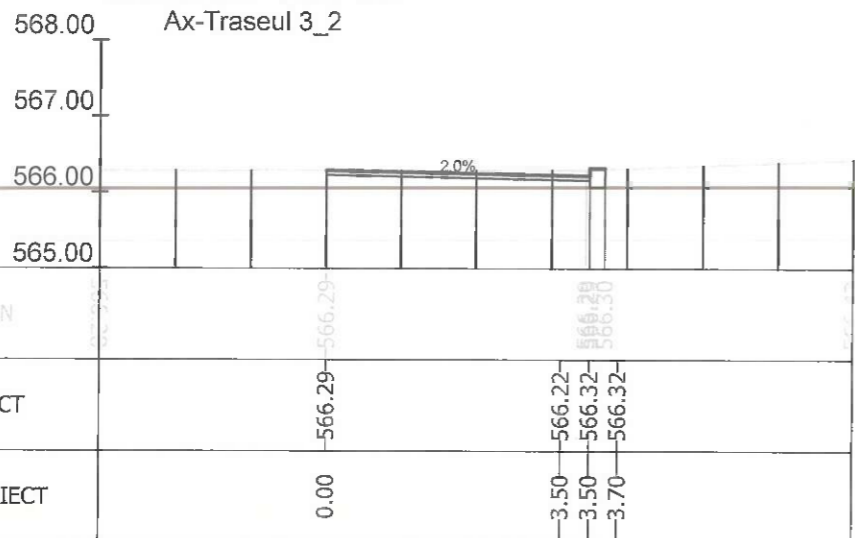
Sectiunea 41 - Km 0+525
