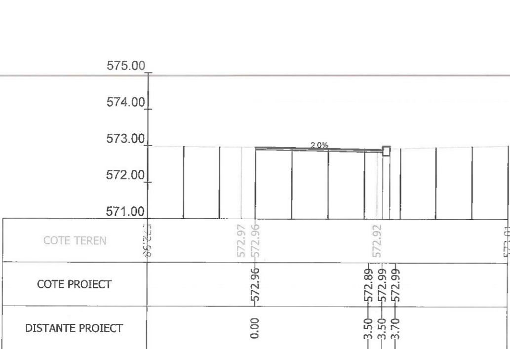
Sectiunea 198 - Km 2+650 Ax-Traseul 1
