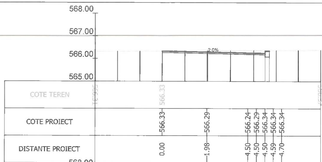
Sectiunea 281 - Km 3+875 Ax-Traseul 1
