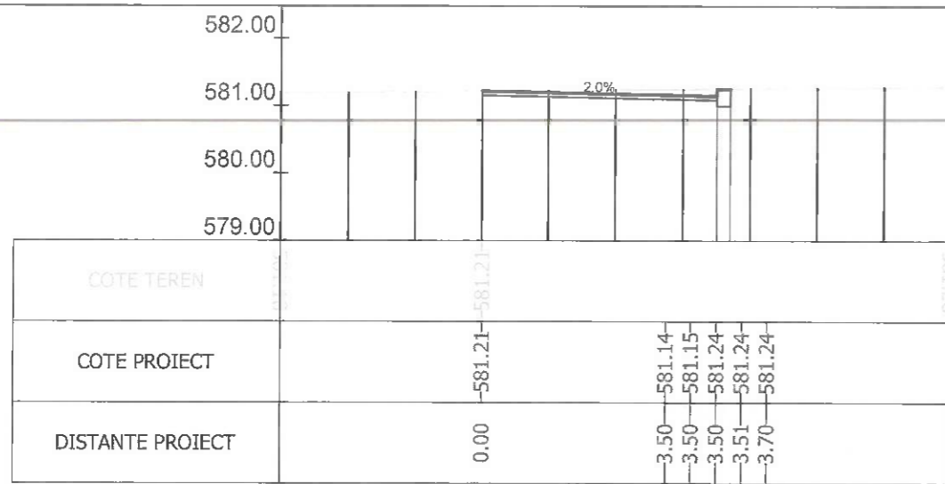
Sectiunea 369 - Km 5+314.079
