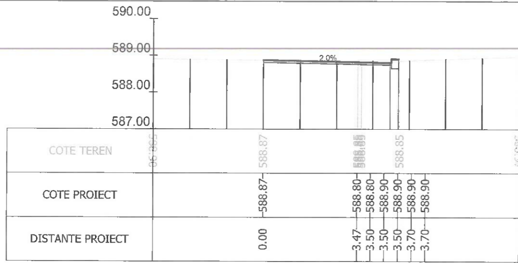
Sectiunea 94 - Km 1+296.601 Ax-Traseul 1
