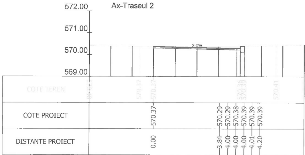
Sectiunea 226 - Km 3+275 Ax-Traseul 2
