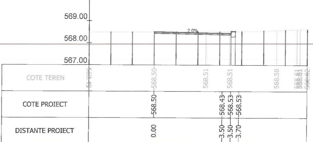
Sectiunea 434 - Km 5+830.002 Ax-Traseul 1
