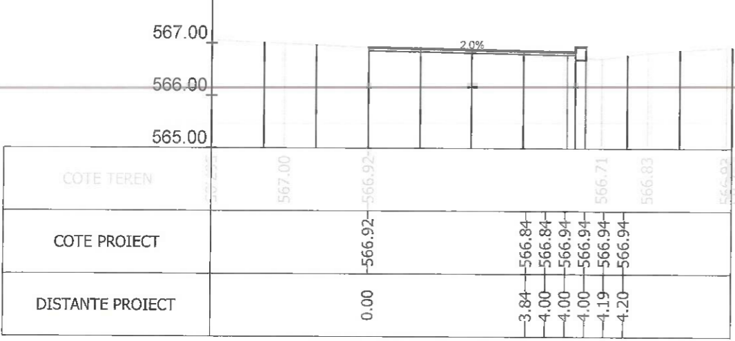
Sectiunea 270 - Km 3+952.719 Ax-Traseul 2
