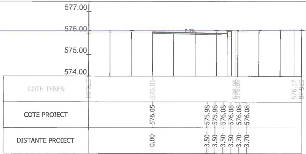
Sectiunea 179 - Km 2+403.881 Ax-Traseul 1
