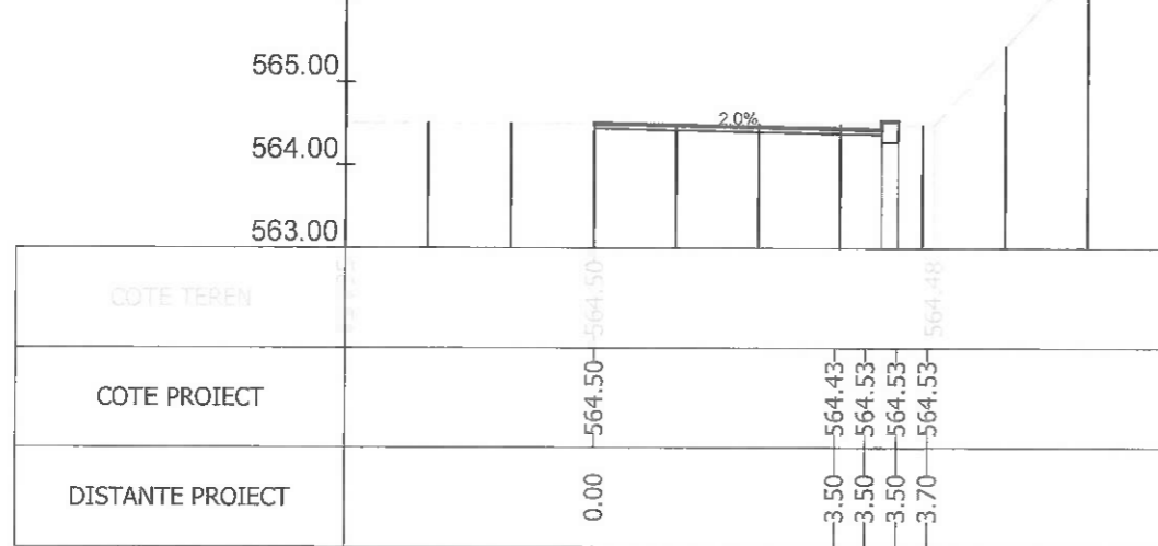
Sectiunea 21 - Km 0+278.258 Ax-Traseul 3_1
