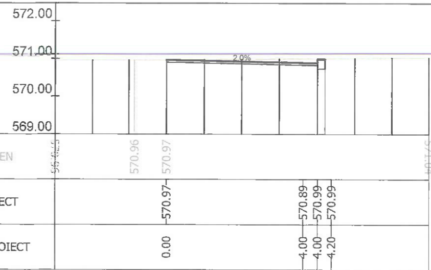
Sectiunea 207 - Km 2+800 Ax-Traseul 1
