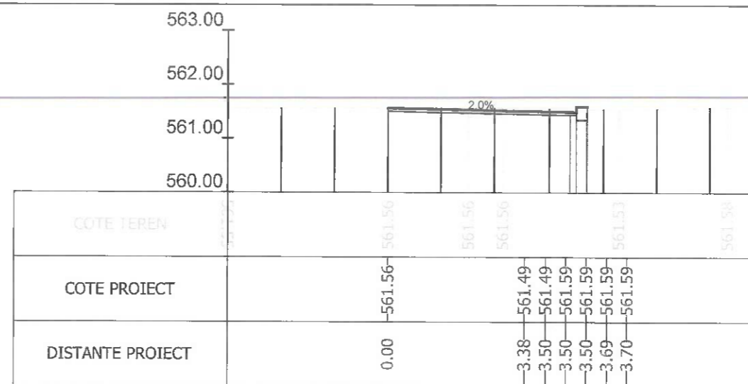
Sectiunea 8 - Km 0+074.373 Ax-Traseul 3_2
