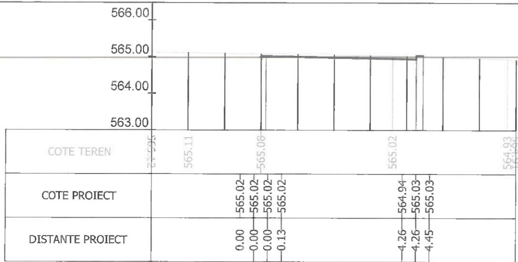
Sectiunea 298 - Km 4+150 Ax-Traseul 1
