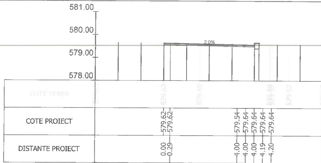
Sectiunea 170 - Km 2+525 Ax-Traseul 2
