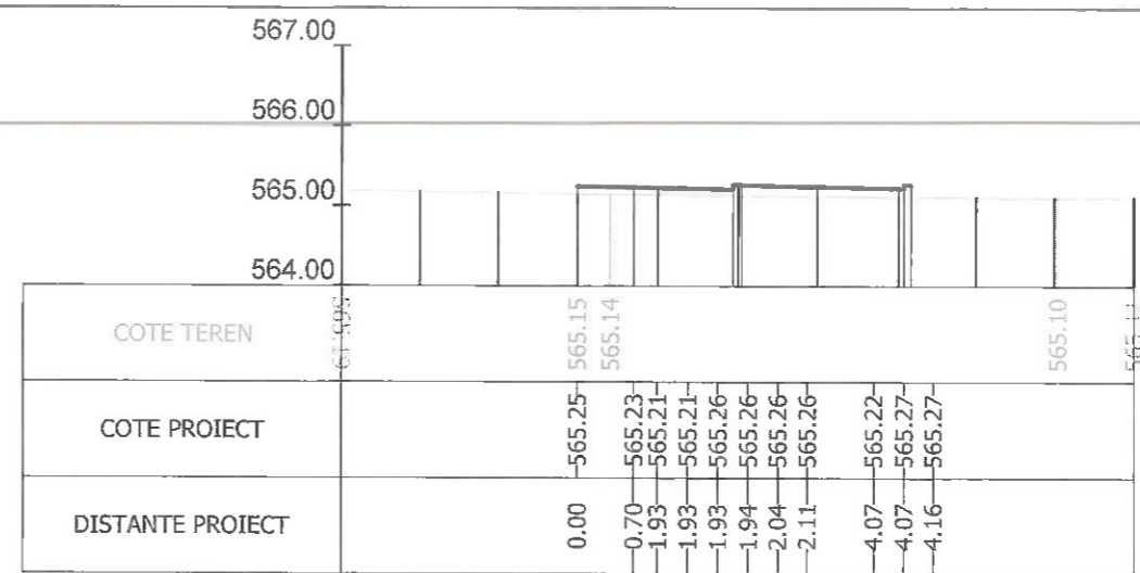
Sectiunea 293 - Km 4+075
