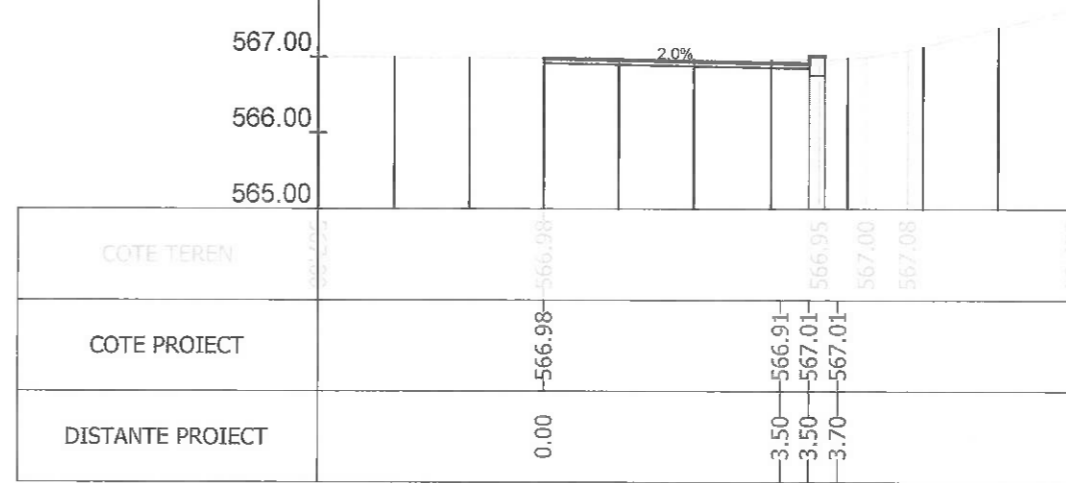
Sectiunea 4 - Km 0+025 Ax-Traseul 3_1
