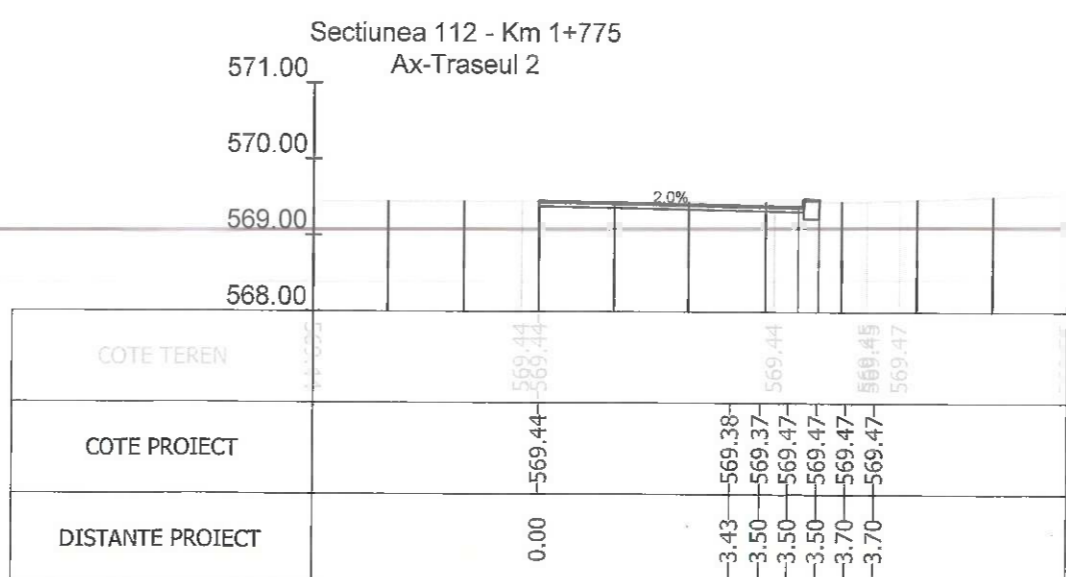
Sectiunea 112 - Km 1+775 Ax-Traseul 2
