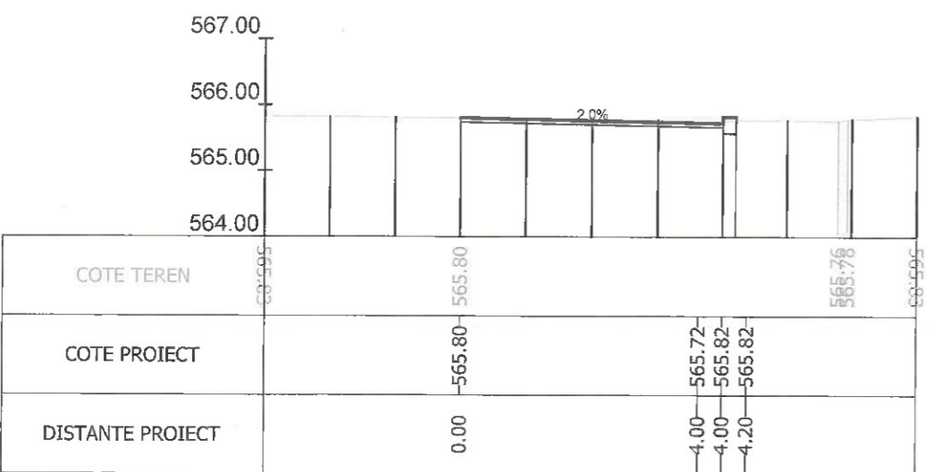
Sectiunea 241 - Km 3+300 Ax-Traseul 1
