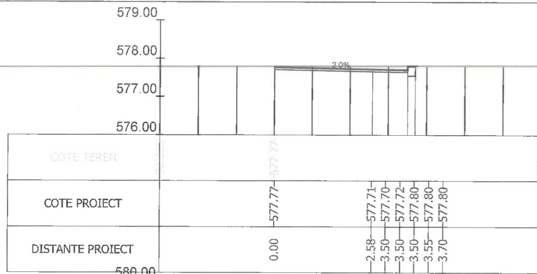
Sectiunea 340 - Km 4+975 Ax-Traceul 2
