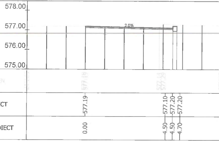
Sectiunea 188 - Km 2+800
