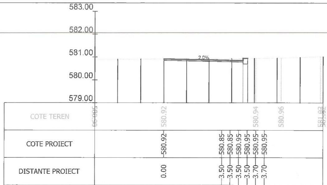
Sectiunea 142 - Km 1+948.400 Ax-Traseul 1
