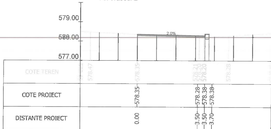
Sectiunea 345 - Km 5+041.048 Ax-Traceul 2
