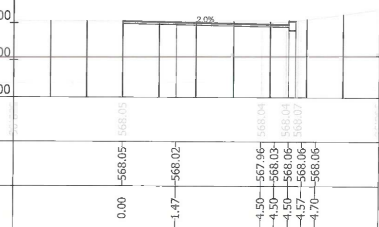
Sectiunea 106 - Km 1+722.570 Ax-Traseul 2
