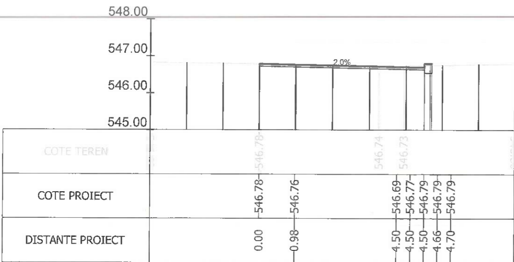
Sectiunea 16 - Km 0+175
