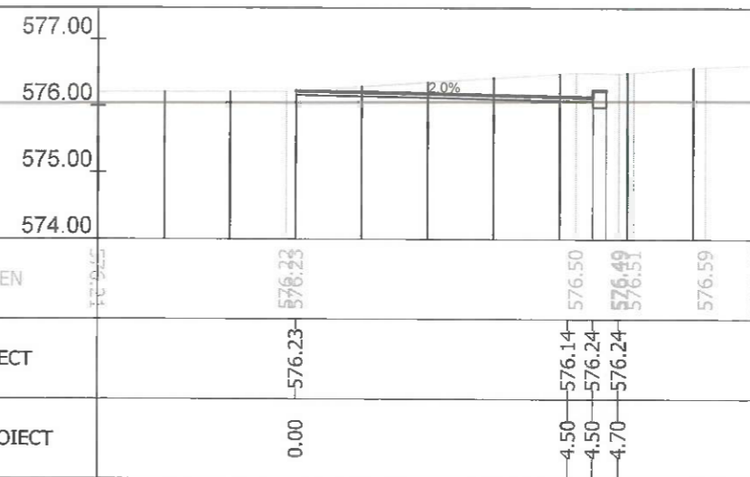
Sectiunea 372 - Km 5+024.085 Ax-Traseul 1
