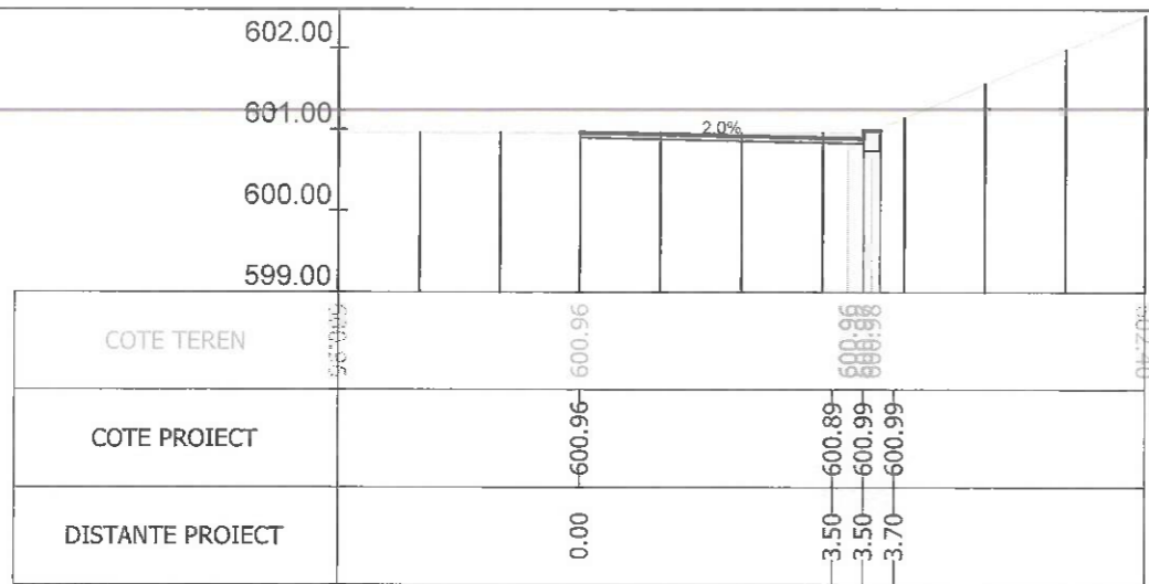
Sectiunea 34 - Km 0+326.302
