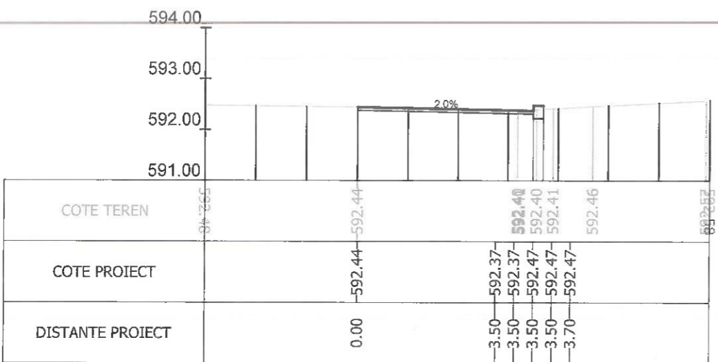
Sectiunea 80 - Km 1+087.394 Ax-Traseul 1
