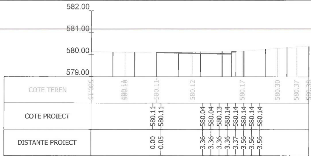
Sectiunea 148 - Km 2+022.230 Ax-Traseul 1
