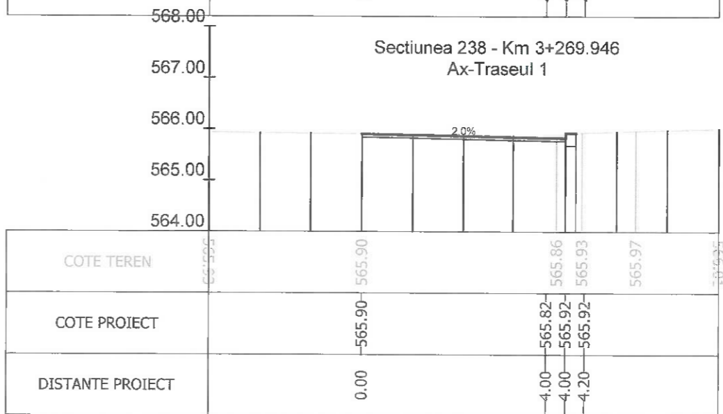
Sectiunea 240 - Km 3+295.187 Ax-Traseul 1
