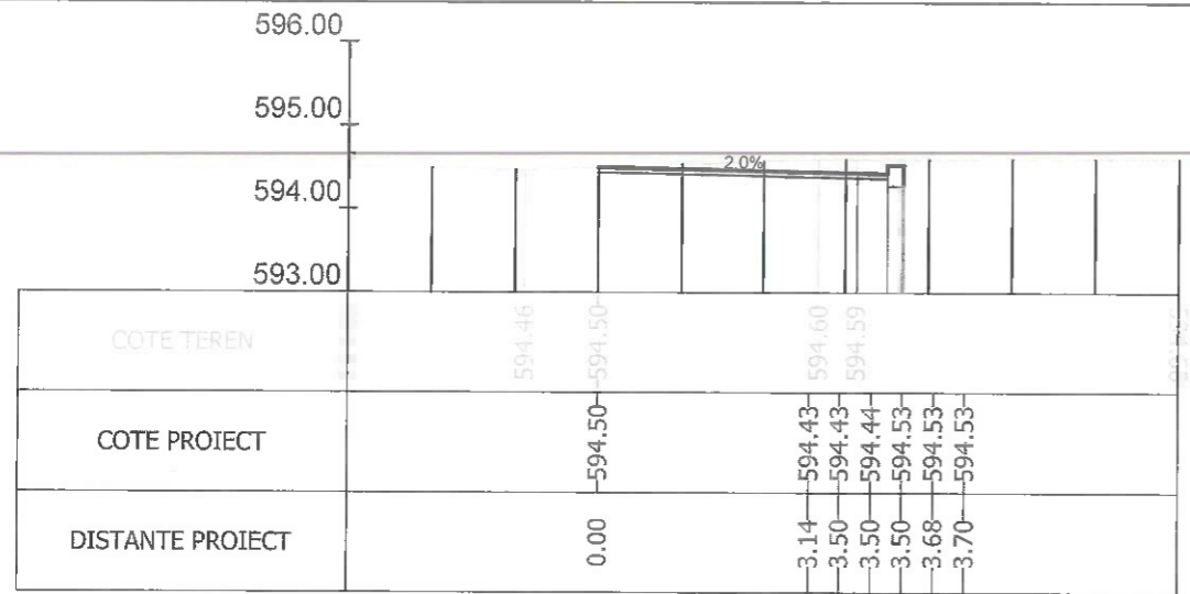
Sectiunea 432 - Km 6+325 Ax-Traseul 2
