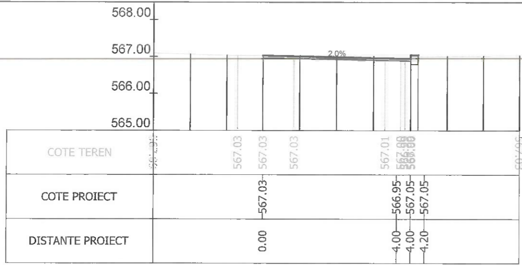
Sectiunea 274 - Km 3+760.591 Ax-Traseul 1
