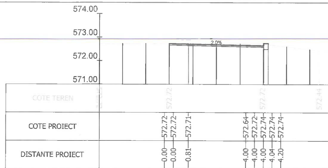
Sectiunea 213 - Km 3+075 Ax-Traseul 2
