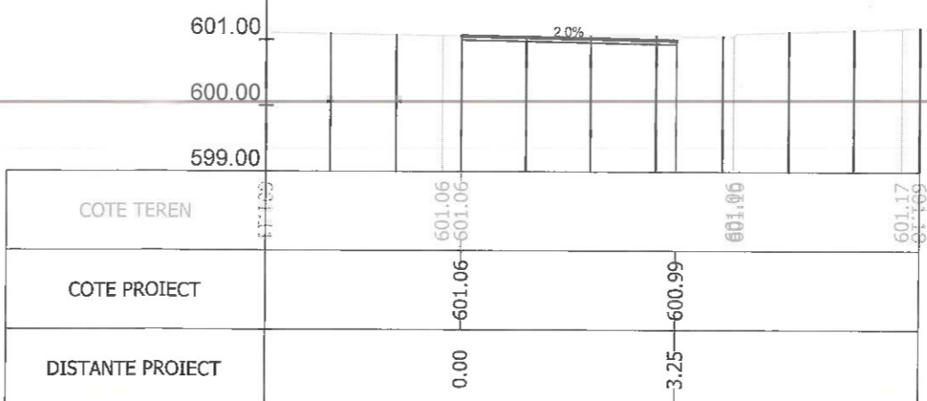
Sectiunea 20 - Km 0+148.906 Ax-Traseul 1
