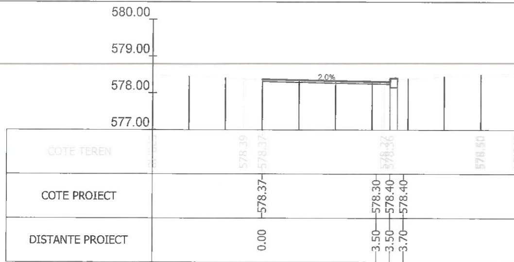
Sectiunea 346 - Km 5+043.508
