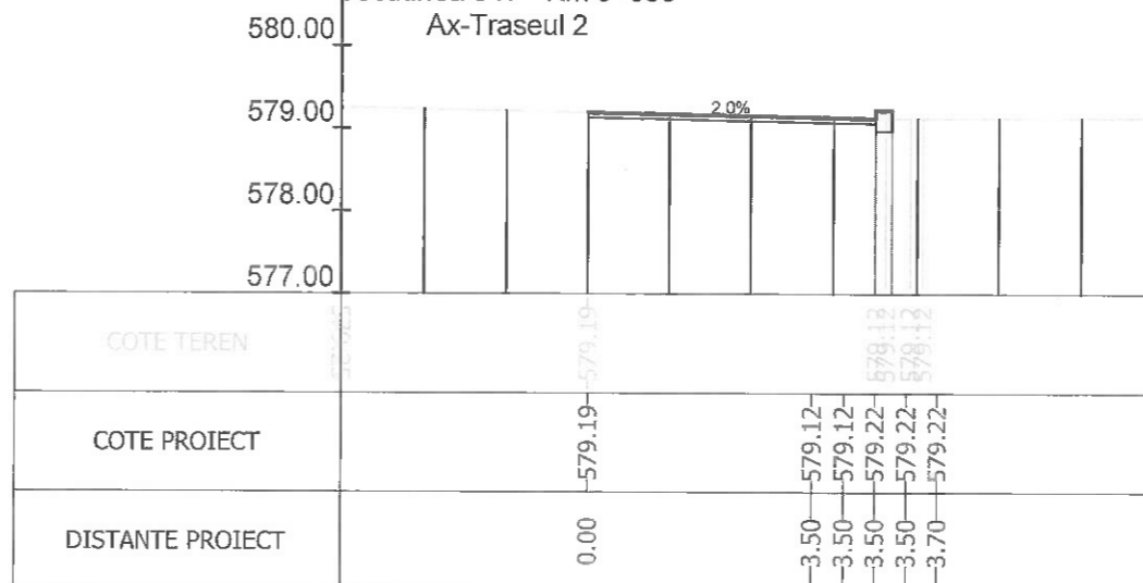
Sectiunea 349 - Km 5+098.175
