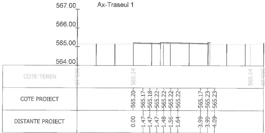
Sectiunea 294 - Km 4+088.360
