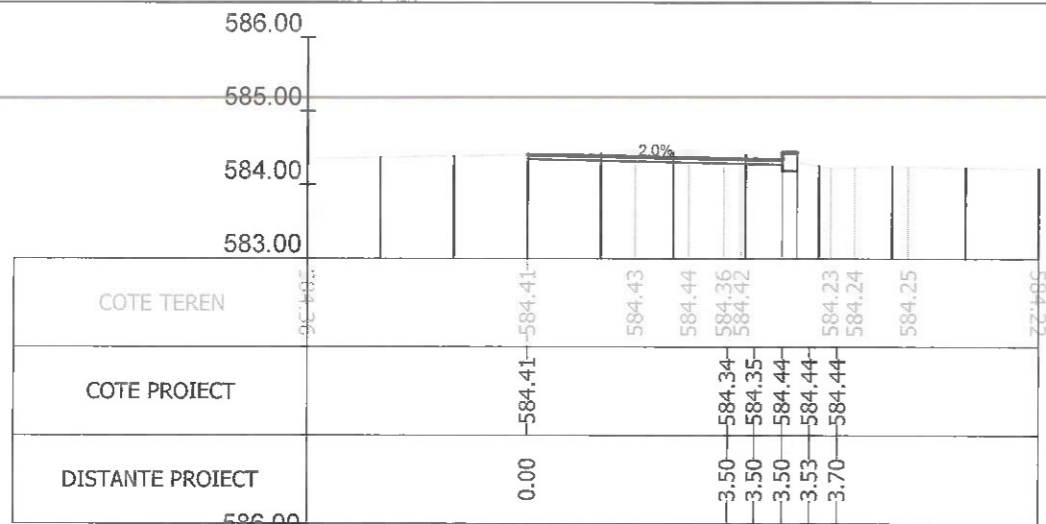
Sectiunea 118 - Km 1+641.115 Ax-Traseul 1
