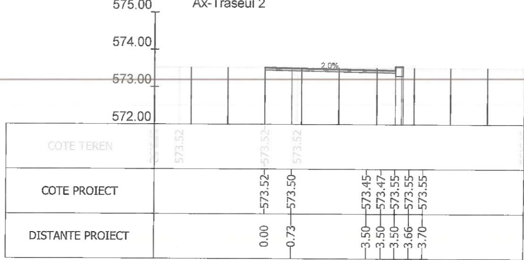
Sectiunea 321 - Km 4+650 Ax-Traseul 2
