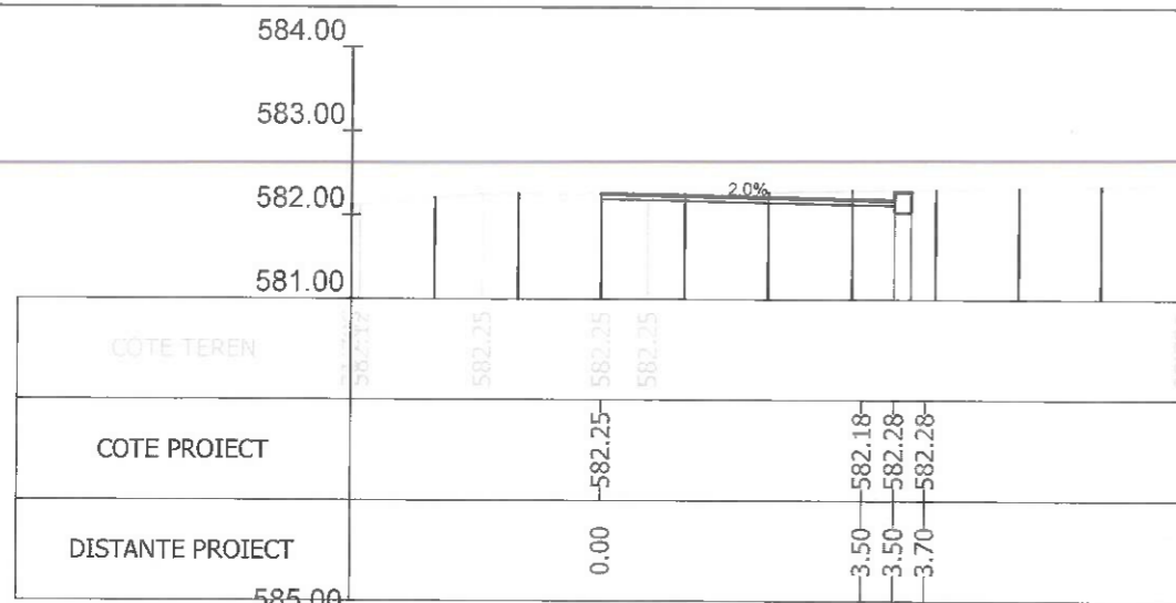
Sectiunea 375 - Km 5+400 Ax-Traseul 2
