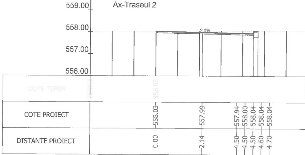
Sectiunea 68 - Km 1+125 Ax-Traseul 2
