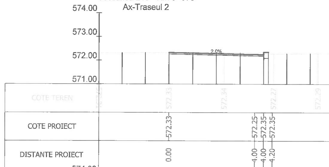
Sectiunea 215 - Km 3+100 Ax-Traseul 2
