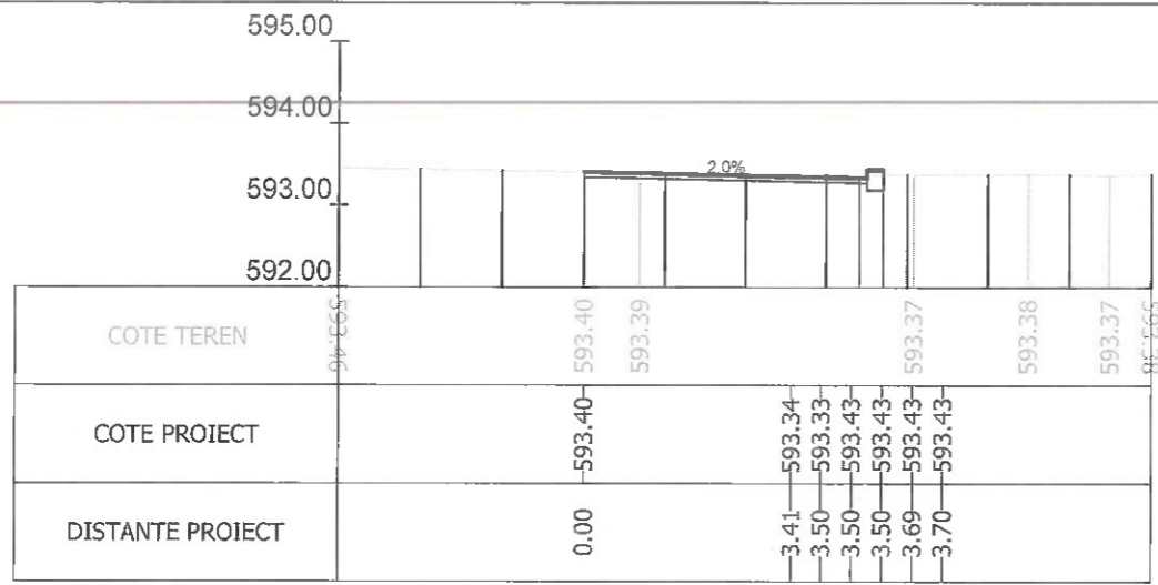
Sectiunea 76 - Km 1+025.562 Ax-Traseul 1
