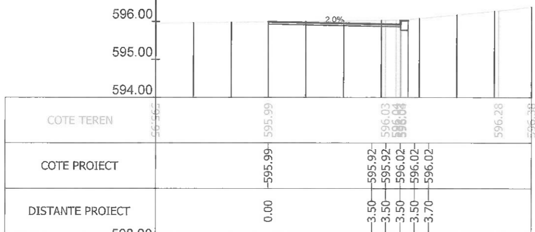
Sectiunea 60 - Km 0+772.950 Ax-Traseul 1
