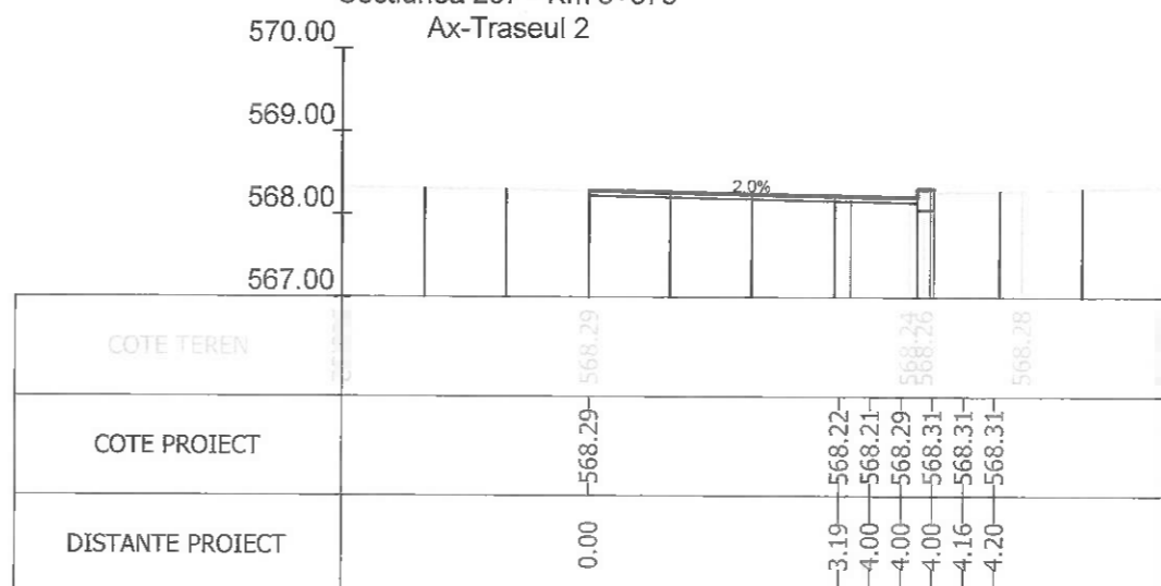
Sectiunea 239 - Km 3+425 Ax-Traseul 2
