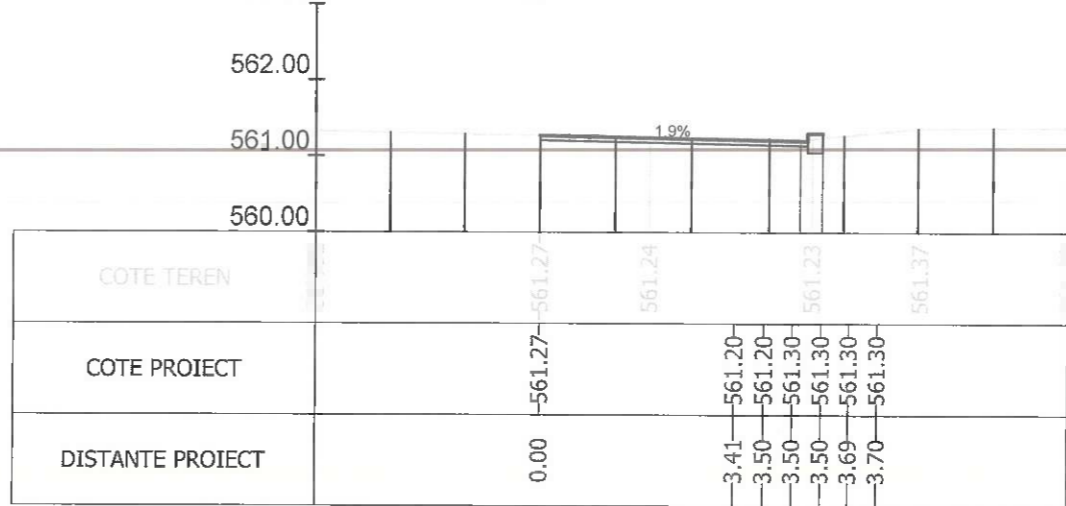
Sectiunea 6 - Km 0+039.365 Ax-Traseul 3_2
