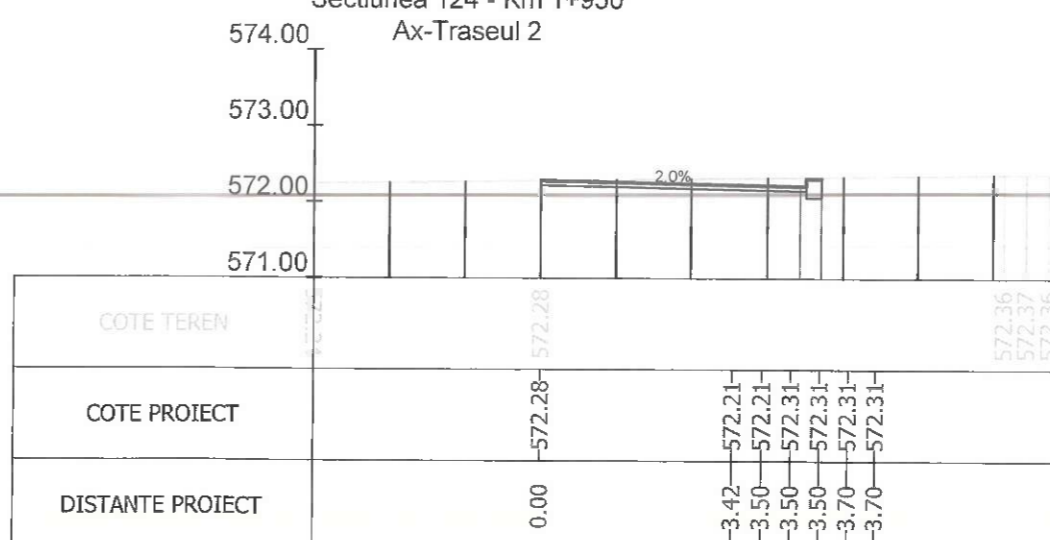
Sectiunea 126 - Km 1+971.988 Ax-Traseul 2
