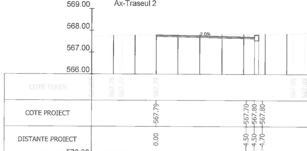
Sectiunea 104 - Km 1+675 Ax-Traseul 2
