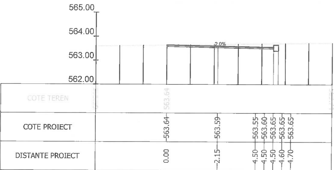
Sectiunea 88 - Km 1+450 Ax-Traseul 2
