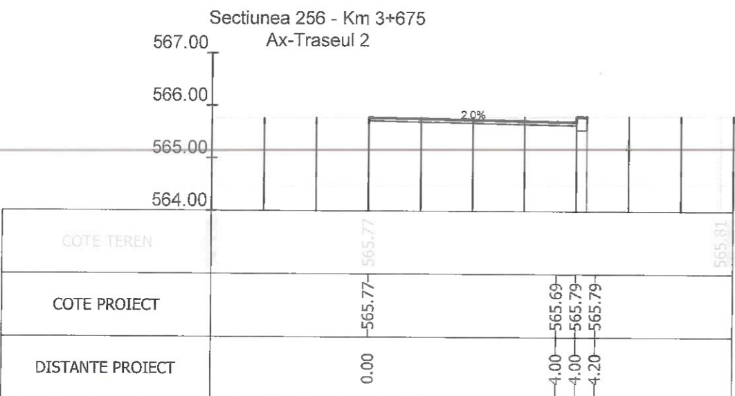
Sectiunea 256 - Km 3+675
