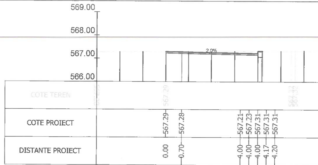
Sectiunea 273 - Km 4+025
