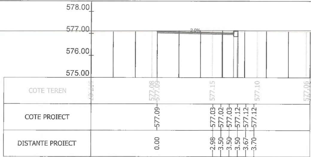
Sectiunea 173 - Km 2+325 Ax-Traseul 1
