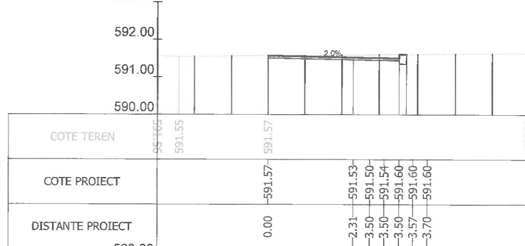
Sectiunea 84 - Km 1+125 Ax-Traseul 1
