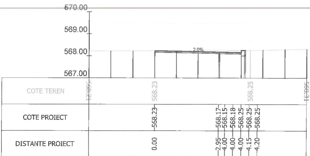
Sectiunea 222 - Km 3+025 Ax-Traseul 1
