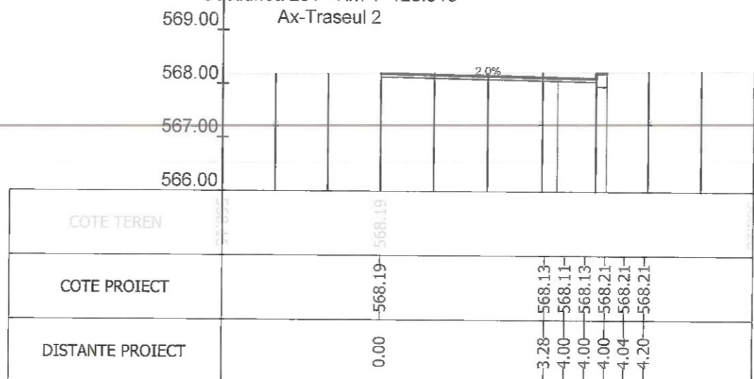
Sectiunea 283 - Km 4+150
