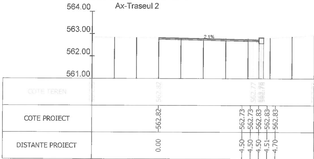
Sectiunea 86 - Km 1+414.592 Ax-Traseul 2
