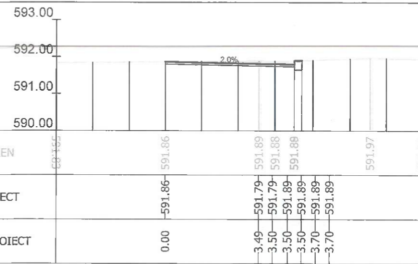
Sectiunea 83 - Km 1+114.550 Ax-Traseul 1
