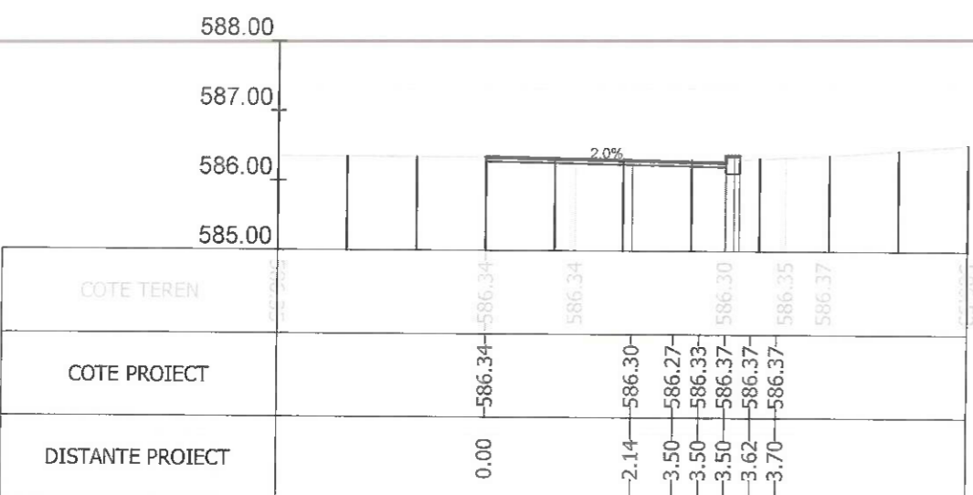
Sectiunea 397 - Km 5+775 Ax-Traseul 2
