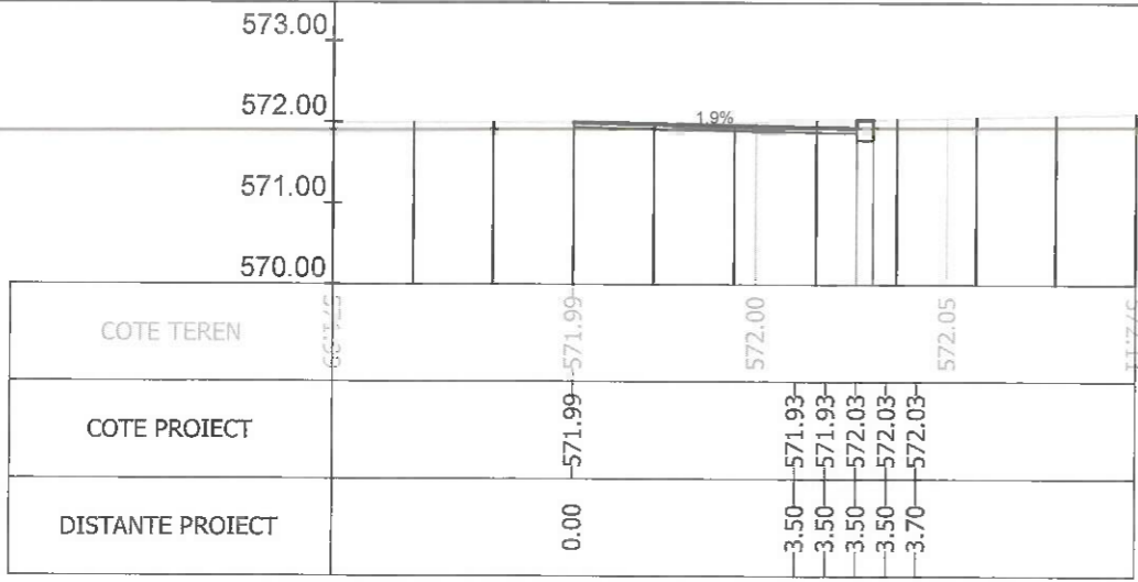
Sectiunea 417 - Km 5+616.216 Ax-Traseul 1
