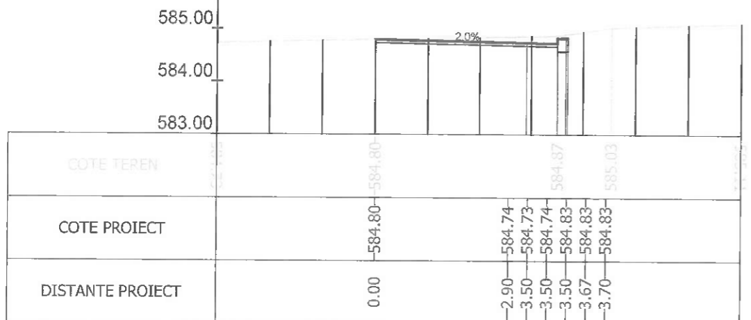
Sectiunea 389 - Km 5+625 Ax-Traseul 2
