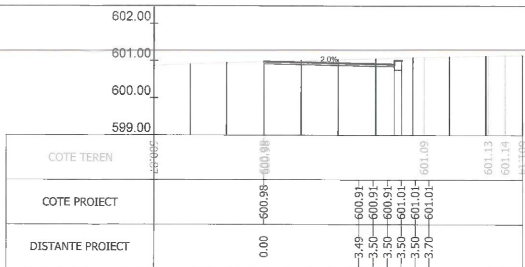
Sectiunea 35 - Km 0+350
