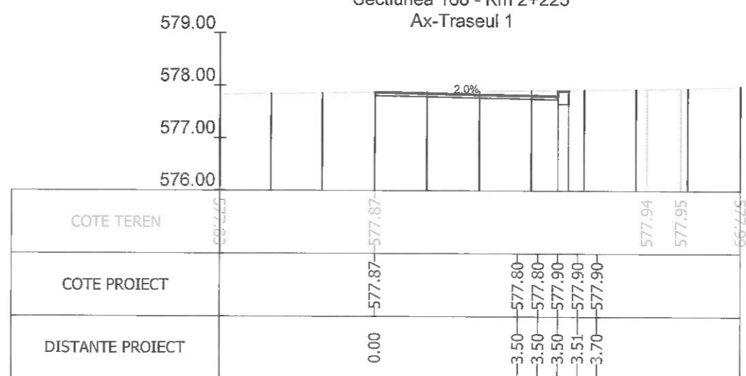
Sectiunea 170 - Km 2+260.630 Ax-Traseul 1
