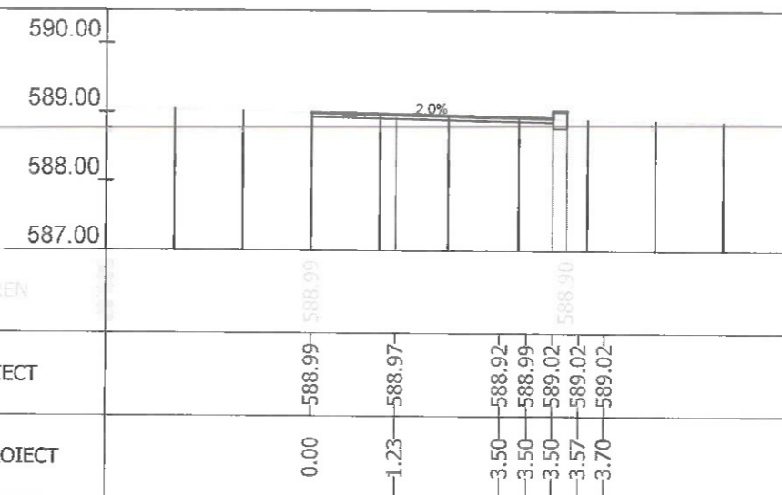
Sectiunea 406 - Km 5+950 Ax-Traseul 2
