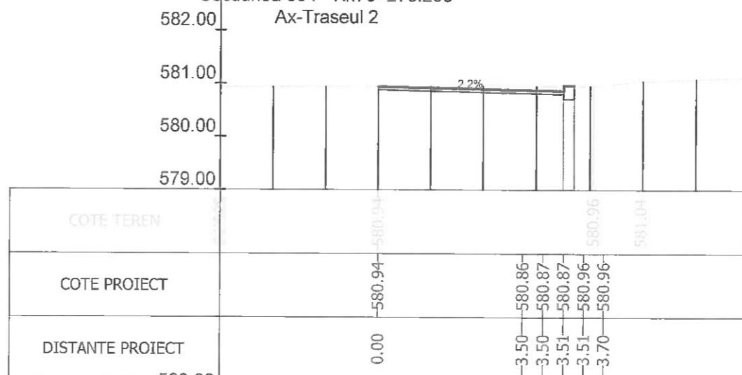
Sectiunea 366 - Km 5+295.740 Ax-Traseul 2
