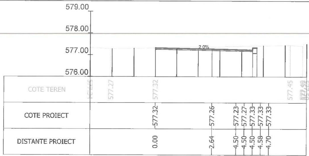
Sectiunea 377 - Km 5+125 Ax-Traseul 1
