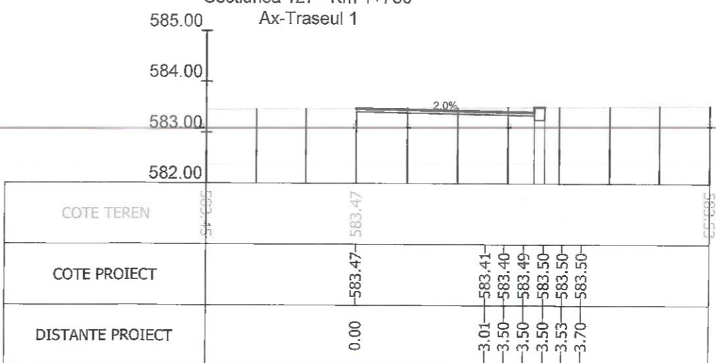
Sectiunea 129 - Km 1+775 Ax-Traseul 1
