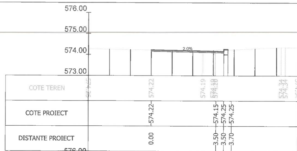
Sectiunea 400 - Km 5+476.522 Ax-Traseul 1
