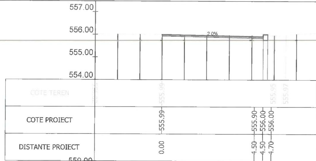
Sectiunea 60 - Km 1+000 Ax-Traseul 2
