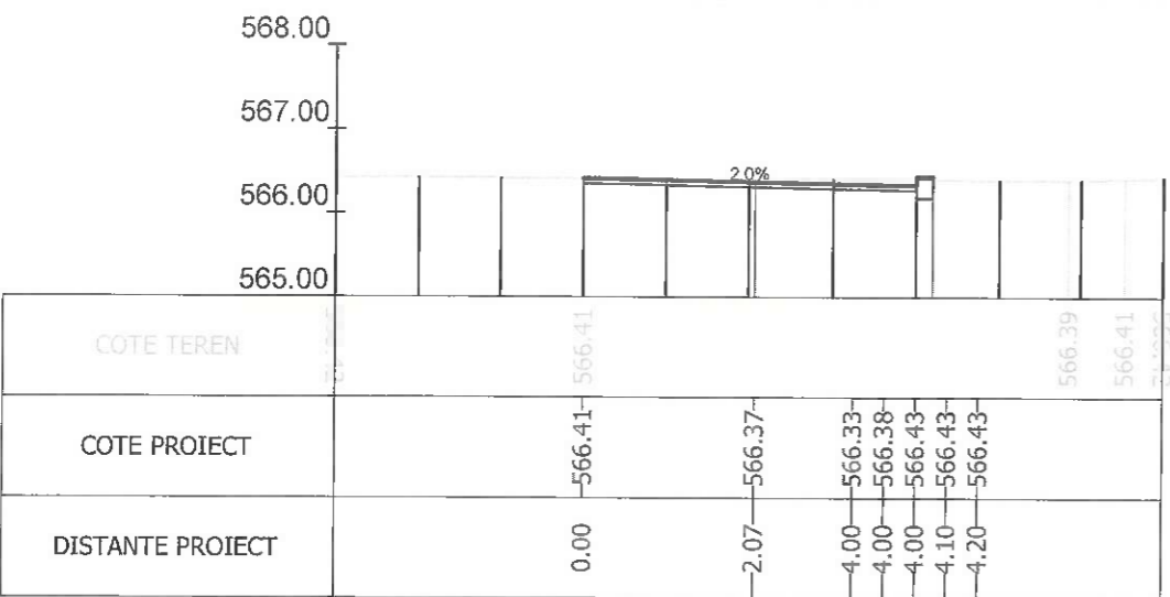
Sectiunea 264 - Km 3+850 Ax-Traseul 2
