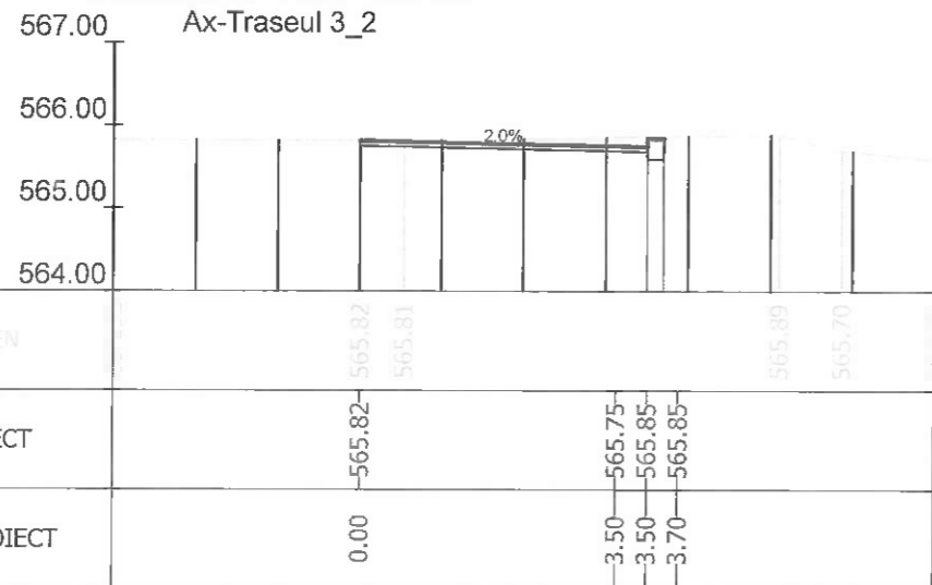
Sectiunea 39 - Km 0+500
