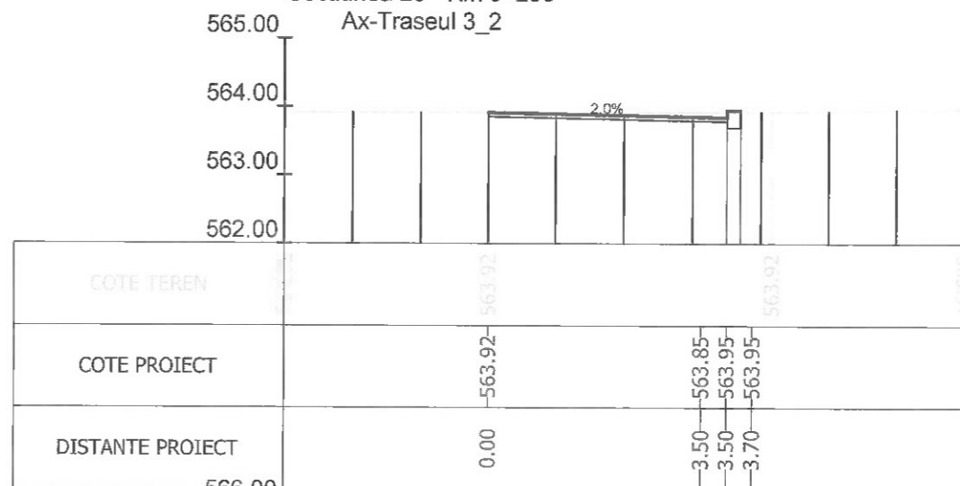
Sectiunea 22 - Km 0+300 Ax-Traseul 3_2
