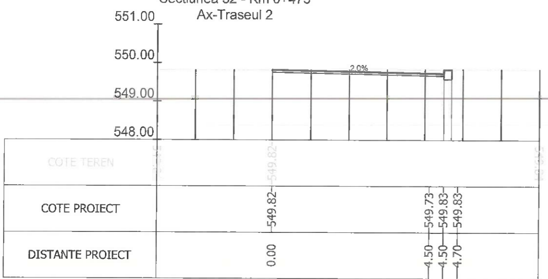
Sectiunea 34 - Km 0+500 Ax-Traseul 2
