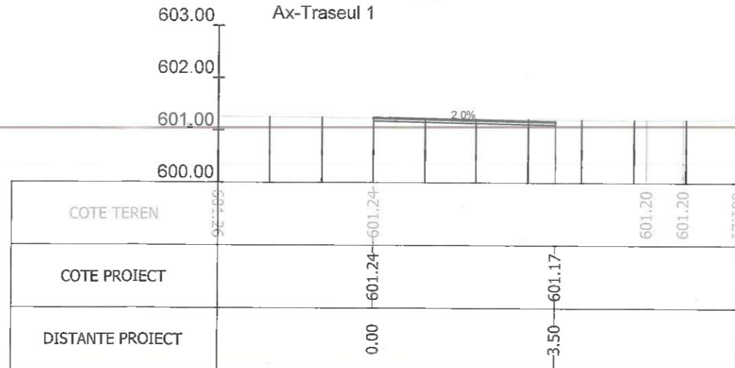
Sectiunea 14 - Km 0+100 Ax-Traseul 1
