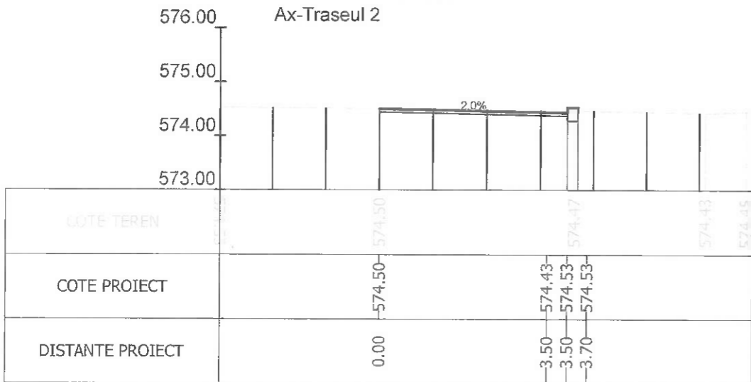
Sectiunea 324 - Km 4+700
