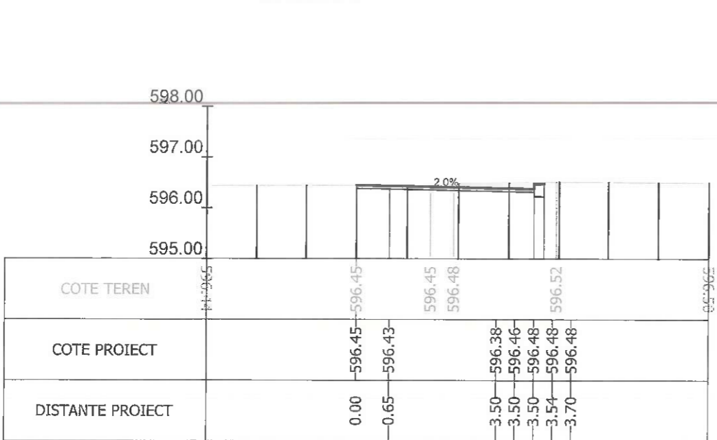
Sectiunea 56 - Km 0+725 Ax-Traseul 1
