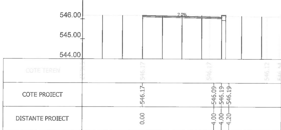
Sectiunea 5 - Km 0+075 Ax-Traseul 2
