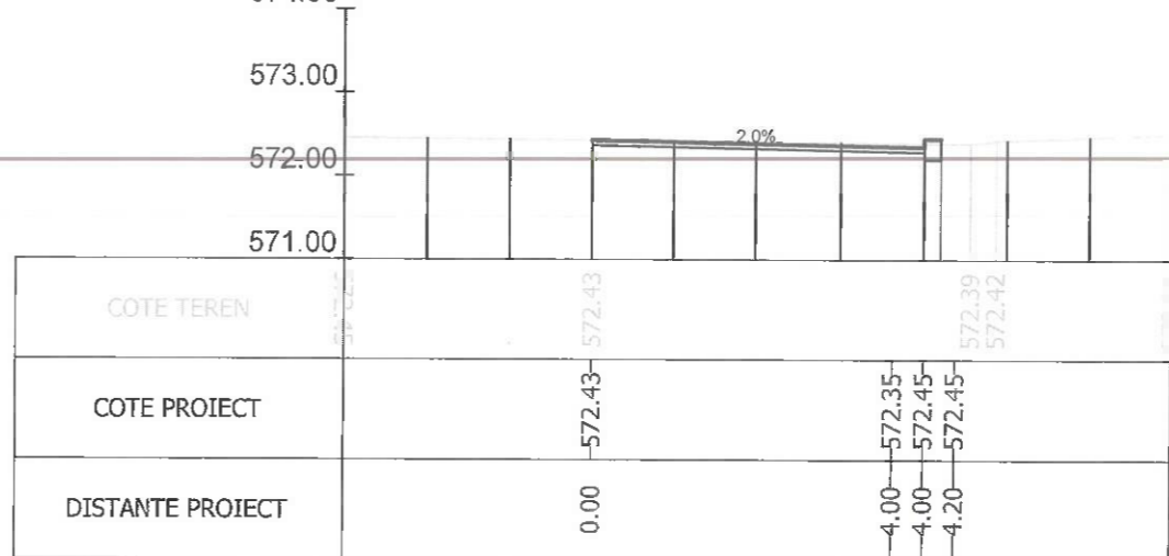
Sectiunea 313 - Km 4+600
