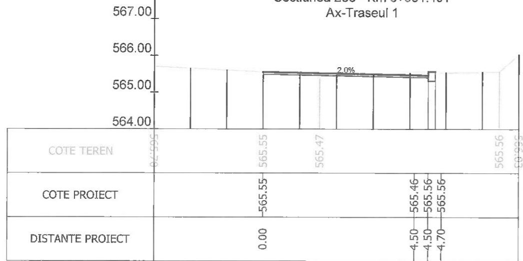
Sectiunea 288 - Km 4+000 Ax-Traseul 1
