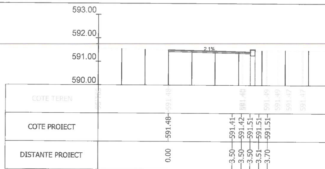
Sectiunea 415 - Km 6+088.821 Ax-Traseul 2
