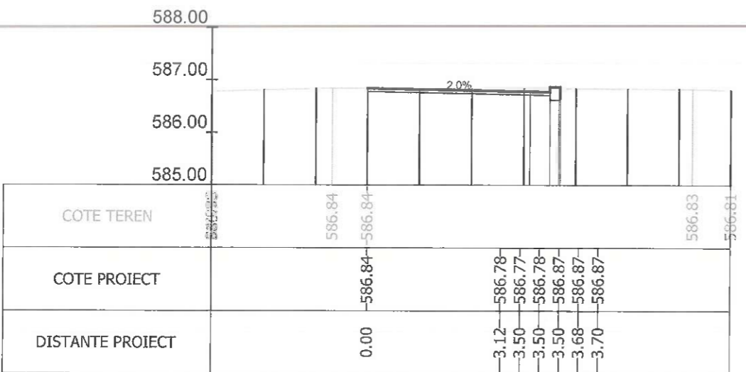
Sectiunea 104 - Km 1+425 Ax-Traseul 1
