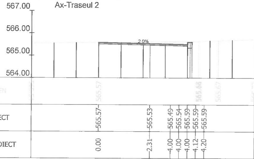
Sectiunea 254 - Km 3+658.462
