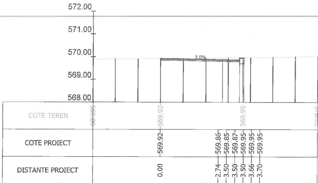
Sectiunea 427 - Km 5+750 Ax-Traseul 1
