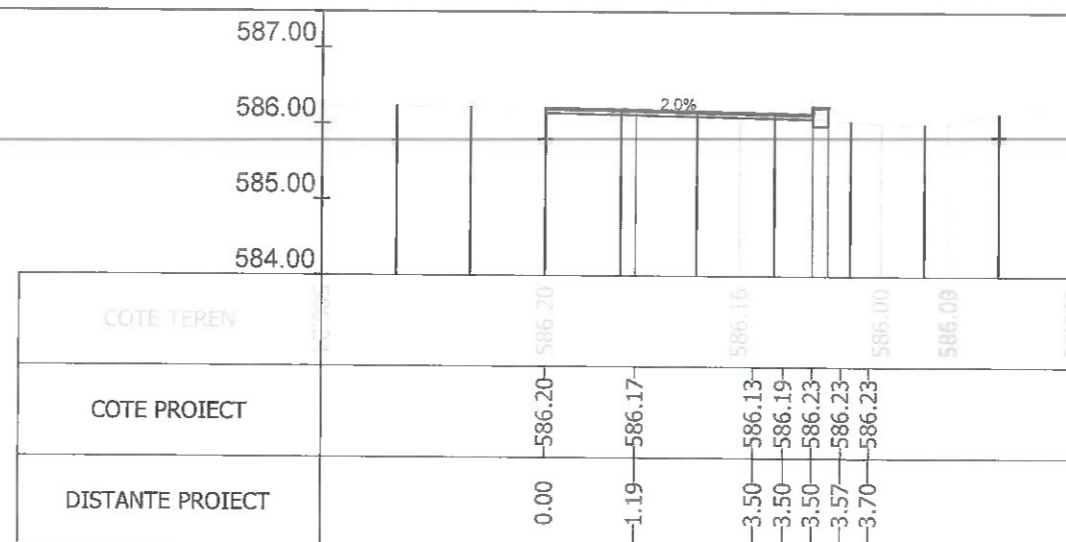
Sectiunea 394 - Km 5+725 Ax-Traseul 2
