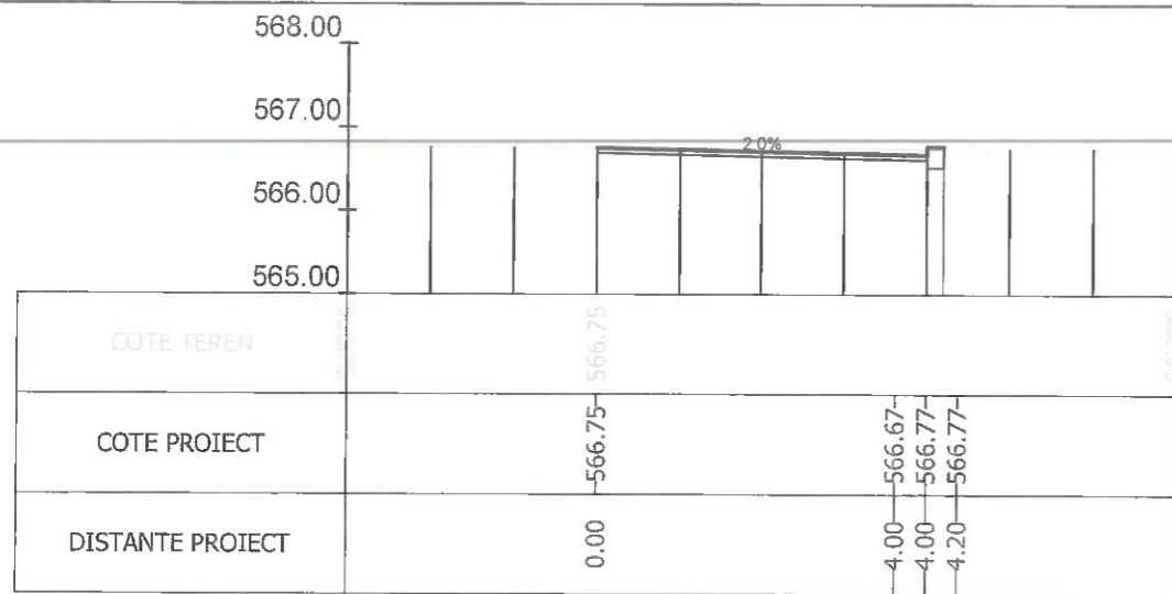
Sectiunea 266 - Km 3+900 Ax-Traseul 2
