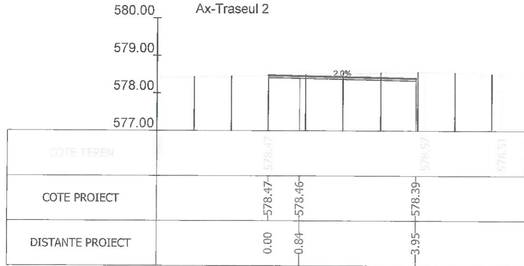
Sectiunea 150 - Km 2+275 Ax-Traseul 2
