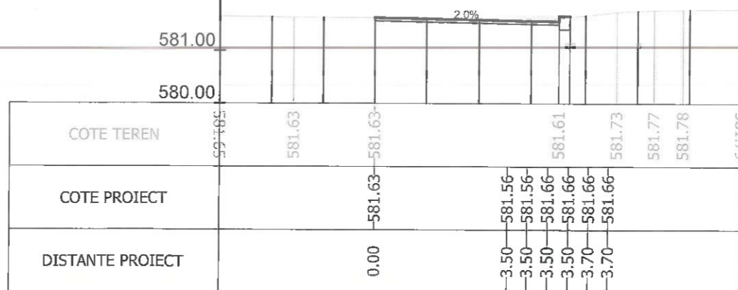
Sectiunea 135 - Km 1+863.140 Ax-Traseul 1
