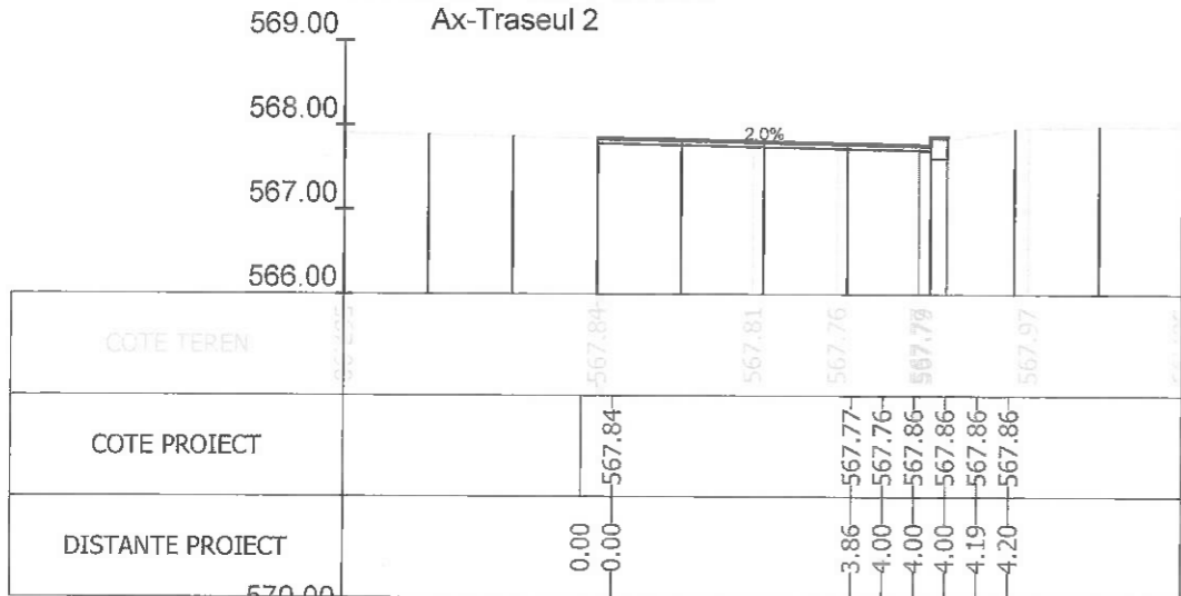
Sectiunea 278 - Km 4+102.825
