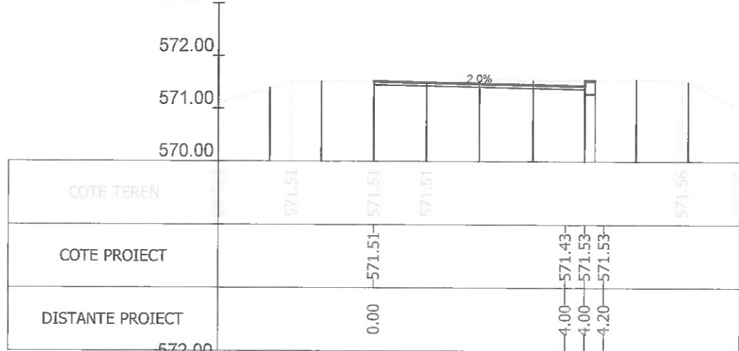
Sectiunea 293 - Km 4+304.835 Ax-Traseul 2
