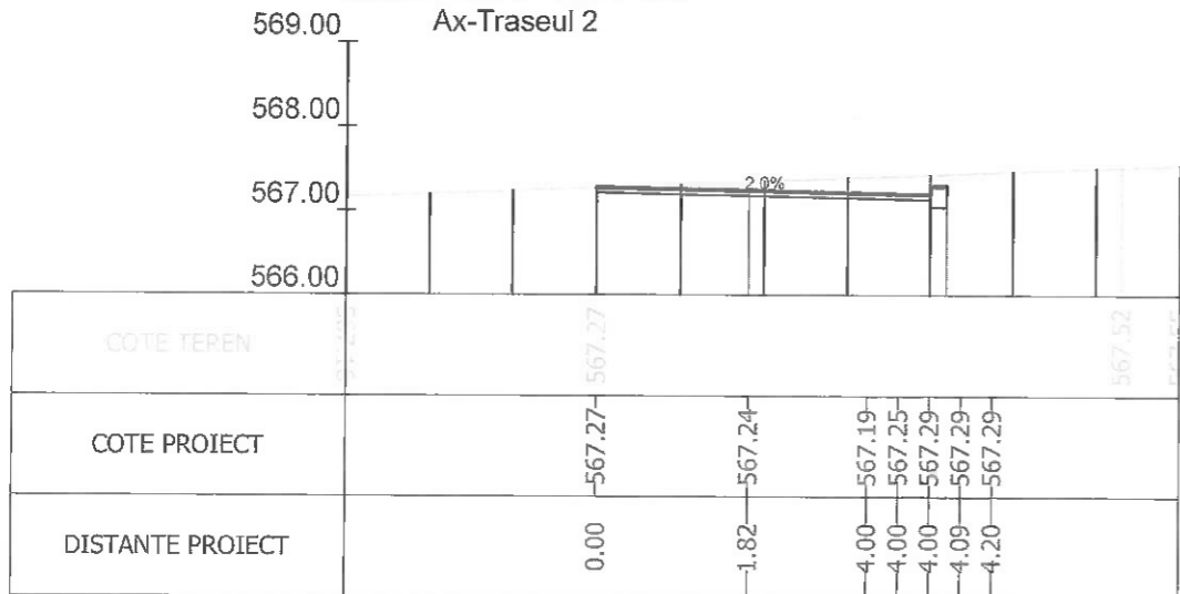
Sectiunea 274 - Km 4+050
