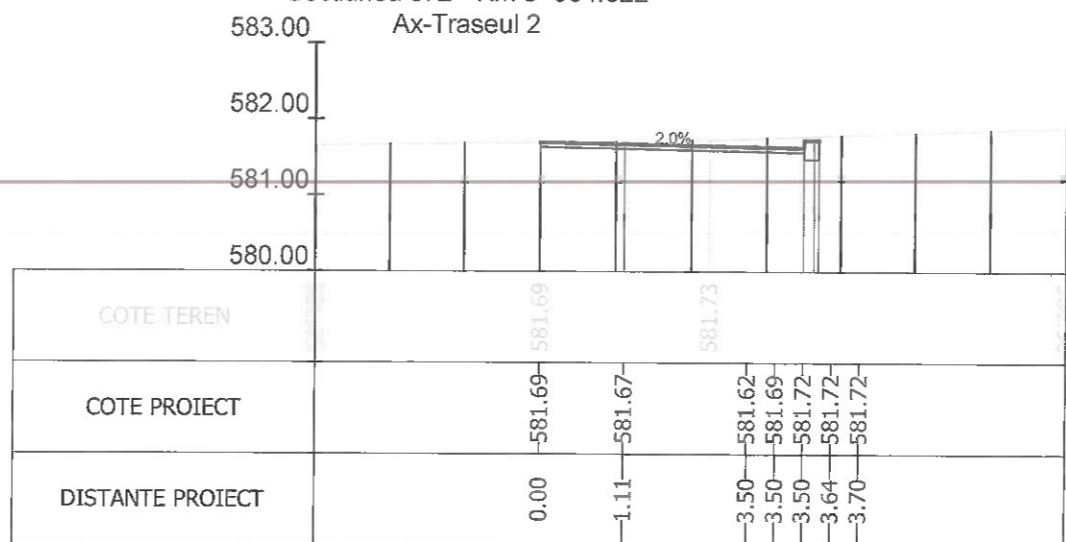
Sectiunea 374 - Km 5+375
