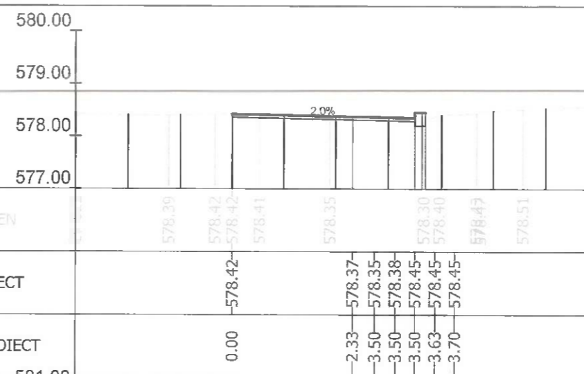
Sectiunea 347 - Km 5+050
