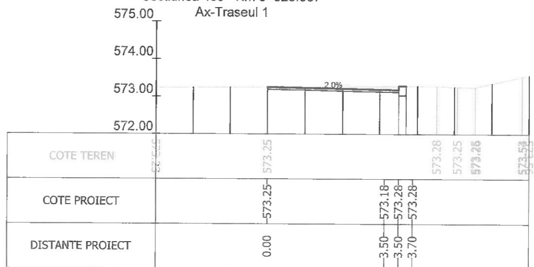
Sectiunea 408 - Km 5+545.393 Ax-Traseul 1
