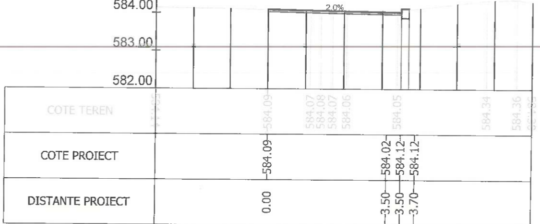
Sectiunea 386 - Km 5+600 Ax-Traseul 2
