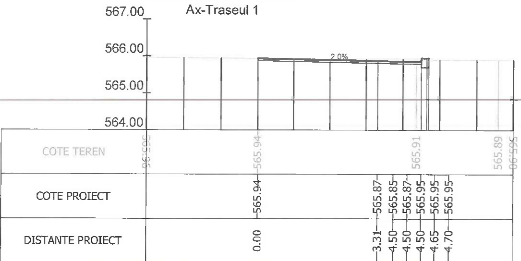
Sectiunea 314 - Km 4+350 Ax-Traseul 1
