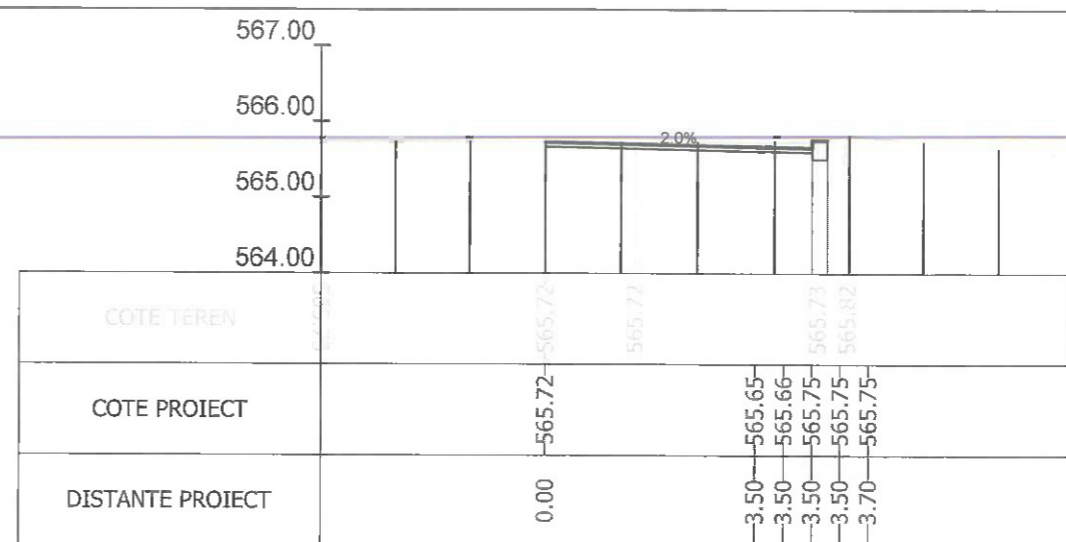
Sectiunea 38 - Km 0+494.578
