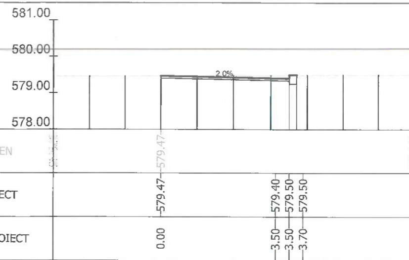
Sectiunea 162 - Km 2+148.823 Ax-Traseul 1
