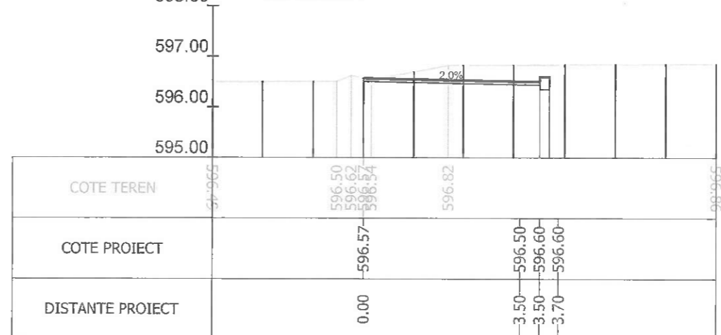
Sectiunea 53 - Km 0+675 Ax-Traseul 1
