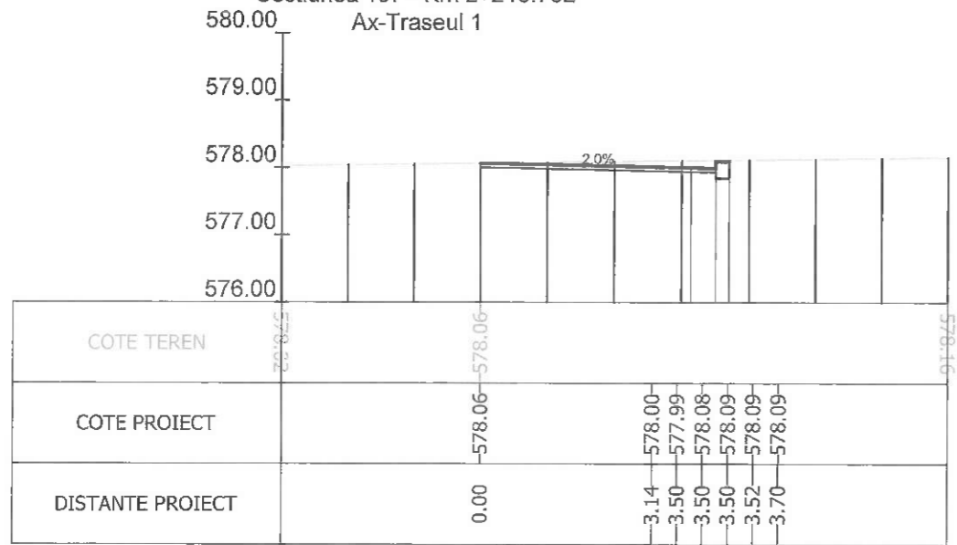
Sectiunea 169 - Km 2+250 Ax-Traseul 1
