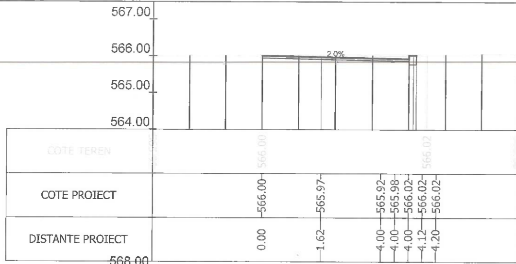
Sectiunea 260 - Km 3+750 Ax-Traseul 2
