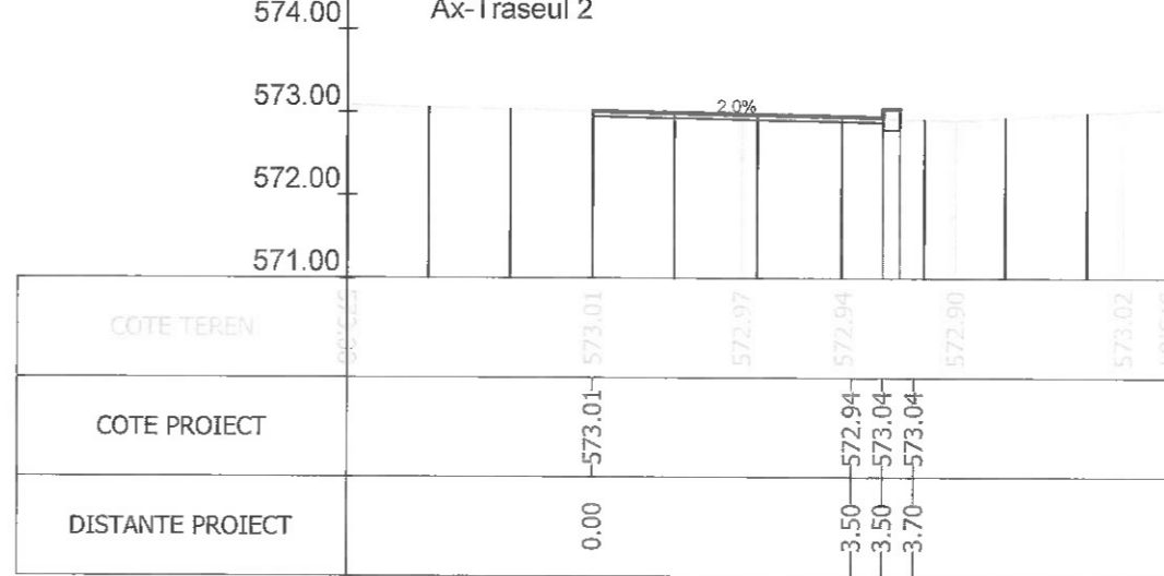
Sectiunea 319 - Km 4+633.896 Ax-Traseul 2
