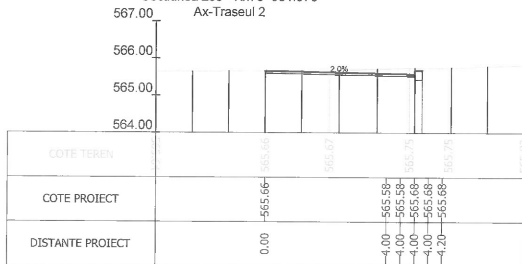
Sectiunea 257 - Km 3+686.069
