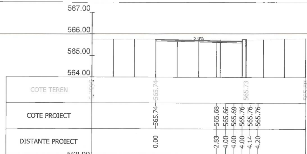
Sectiunea 244 - Km 3+325 Ax-Traseul 1
