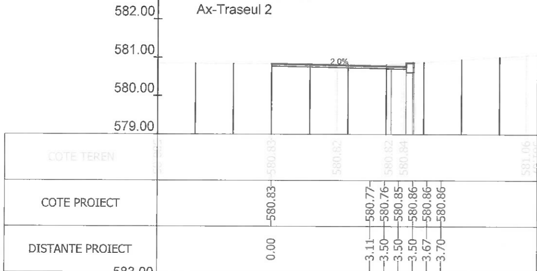
Sectiunea 365 - Km 5+290.051 Ax-Traseul 2
