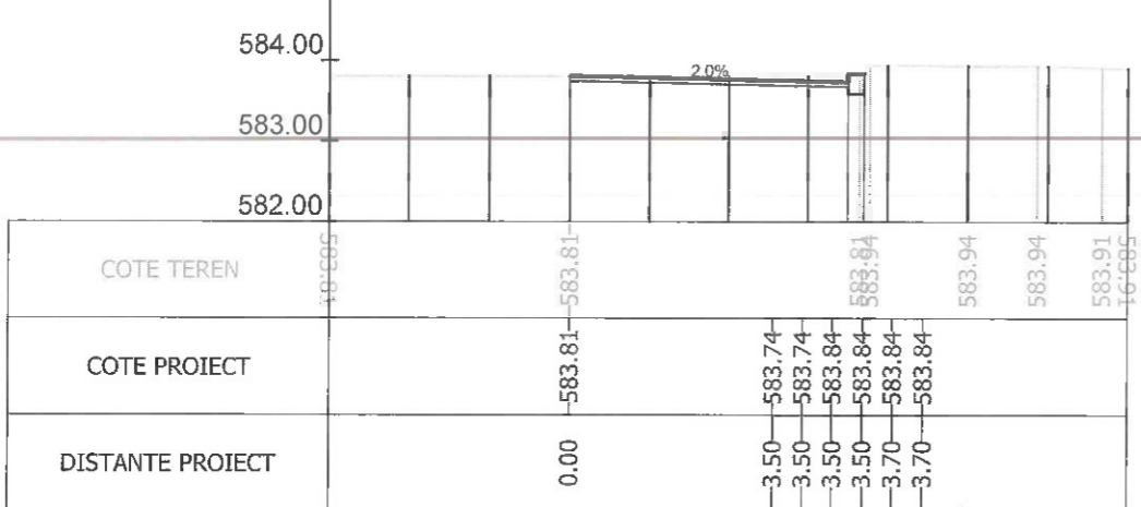
Sectiunea 122 - Km 1+676.146 Ax-Traseul 1
