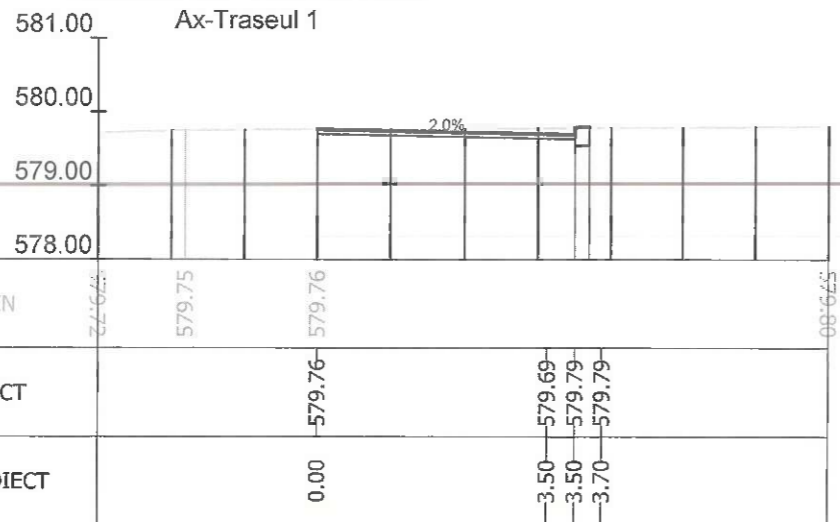
Sectiunea 159 - Km 2+111.013 Ax-Traseul 1
