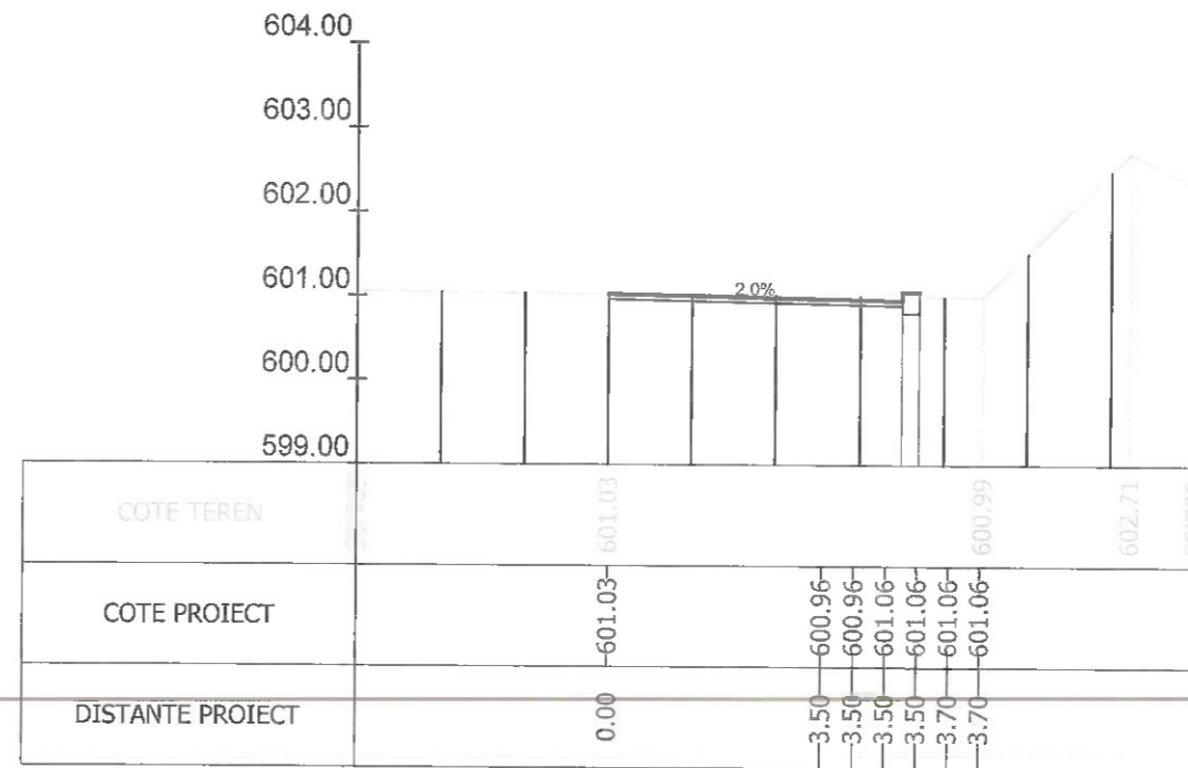
Sectiunea 465 - Km 6+928.790 Ax-Traseul 2
