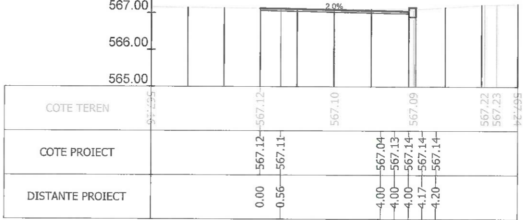
Sectiunea 265 - Km 3+650 Ax-Traseul 1
