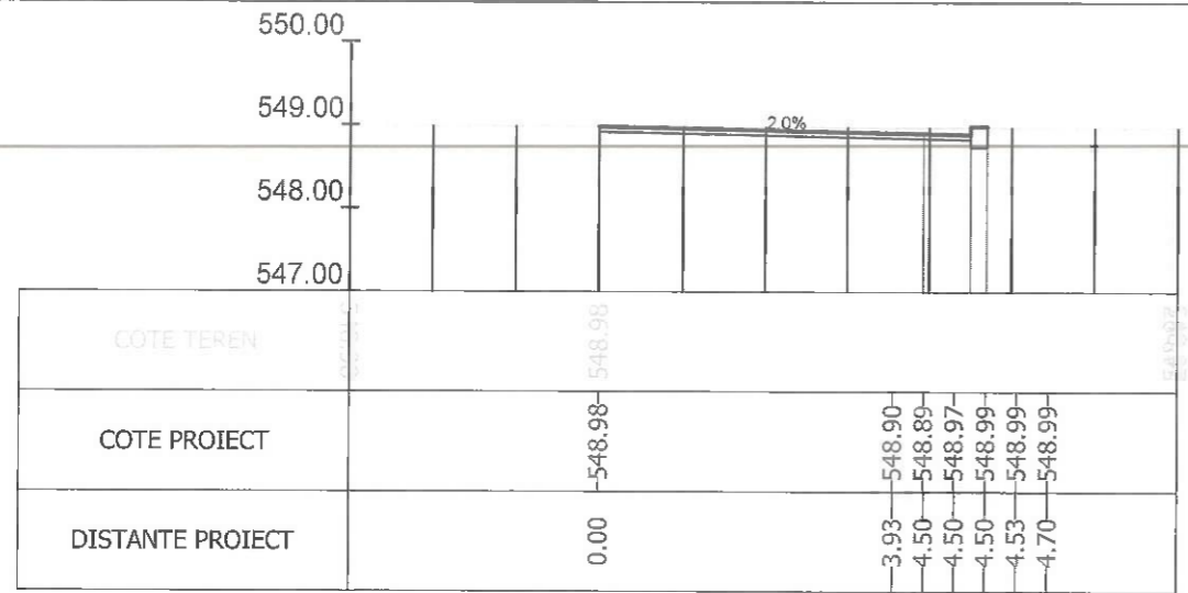
Sectiunea 30 - Km 0+425 Ax-Traseul 2
