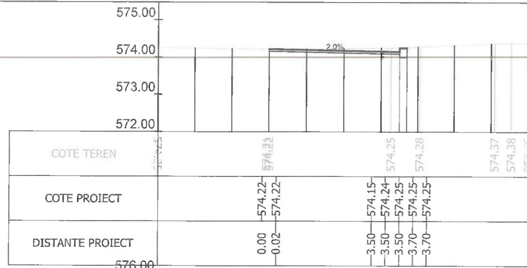
Sectiunea 399 - Km 5+475 Ax-Traseul 1
