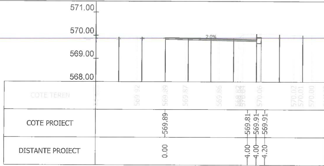
Sectiunea 230 - Km 3+321.916 Ax-Traseul 2
