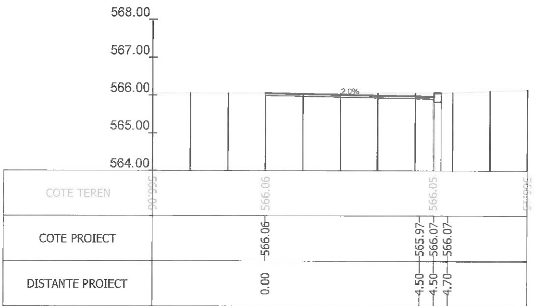
Sectiunea 282 - Km 3+900 Ax-Traseul 1
