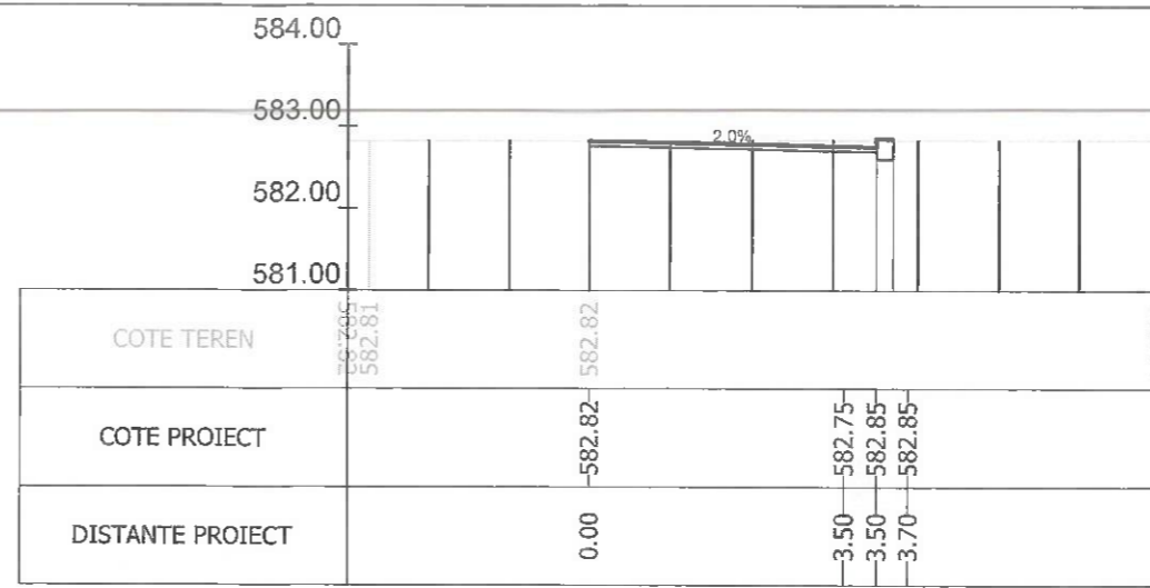
Sectiunea 131 - Km 1+805.998 Ax-Traseul 1
