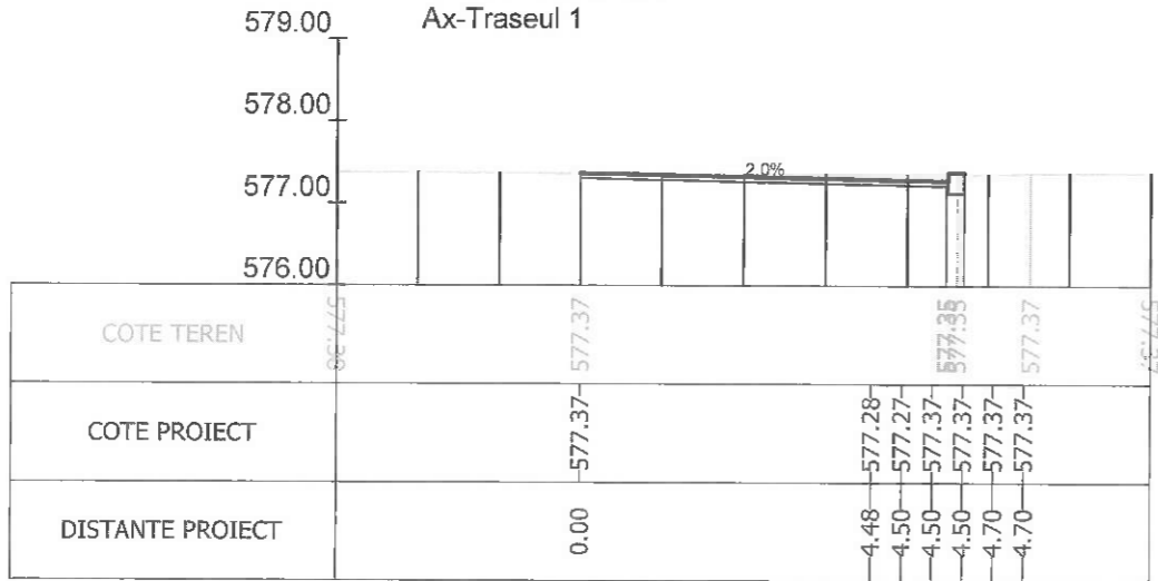
Sectiunea 385 - Km 5+313.849 Ax-Traseul 1
