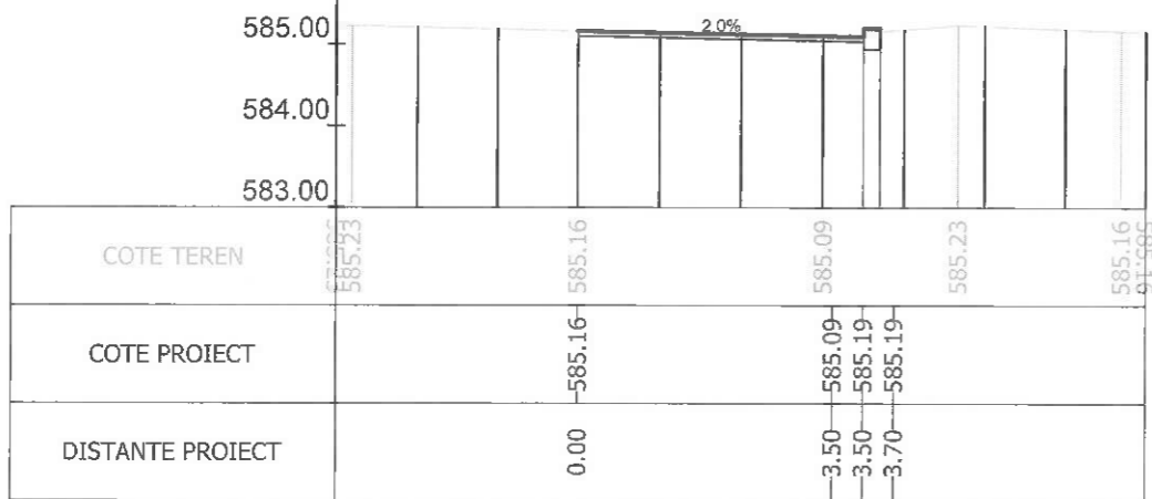
Sectiunea 114 - Km 1+601.136 Ax-Traseul 1
