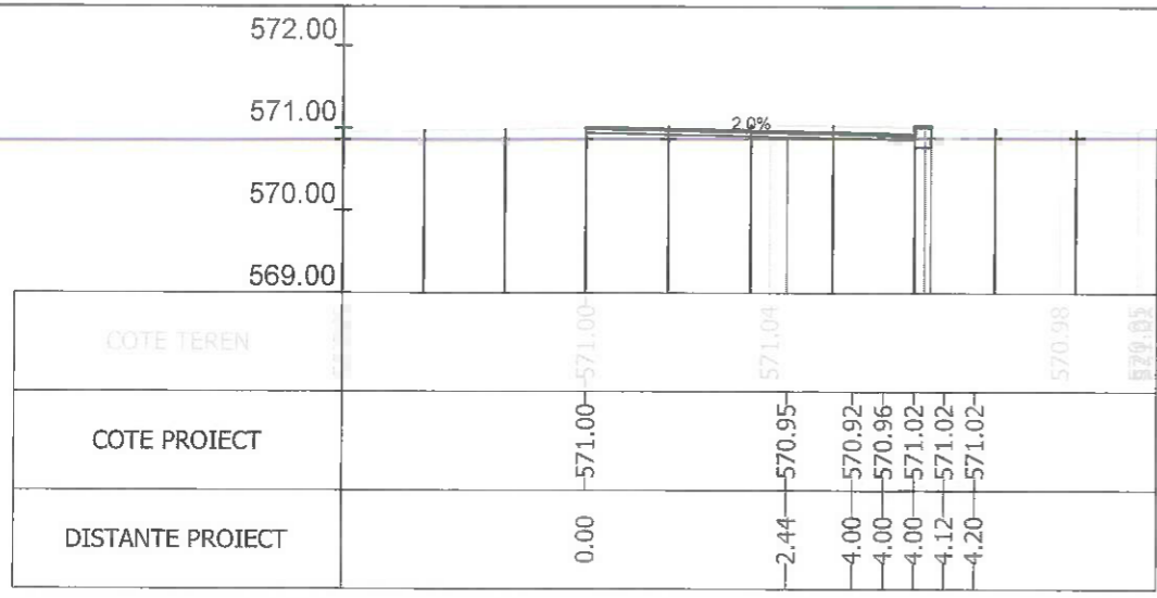
Sectiunea 224 - Km 3+225 Ax-Traseul 2
