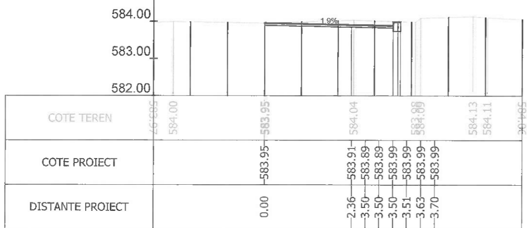
Sectiunea 120 - Km 1+659.844 Ax-Traseul 1
