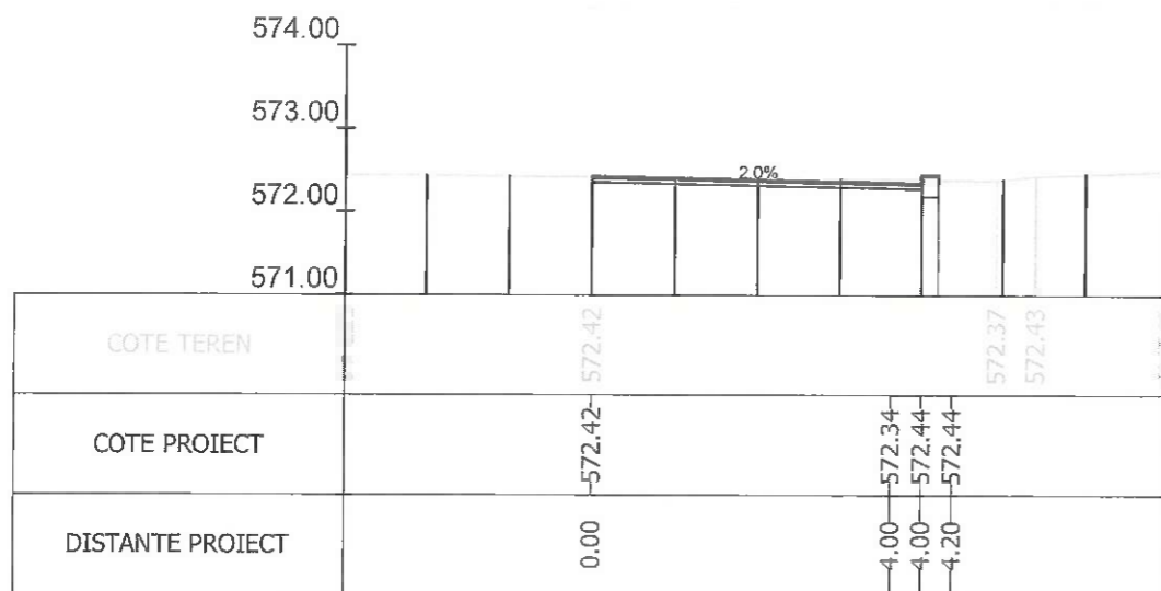
Sectiunea 312 - Km 4+597.927
