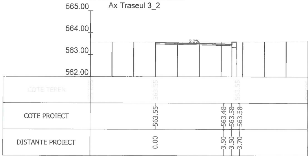
Sectiunea 21 - Km 0+275 Ax-Traseul 3_2
