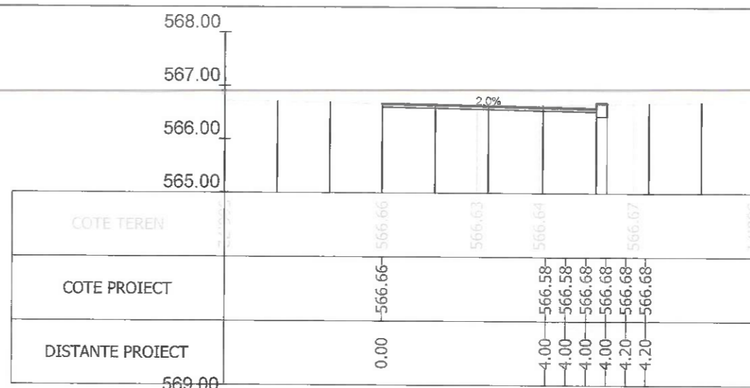
Sectiunea 267 - Km 3+923.437 Ax-Traseul 2
