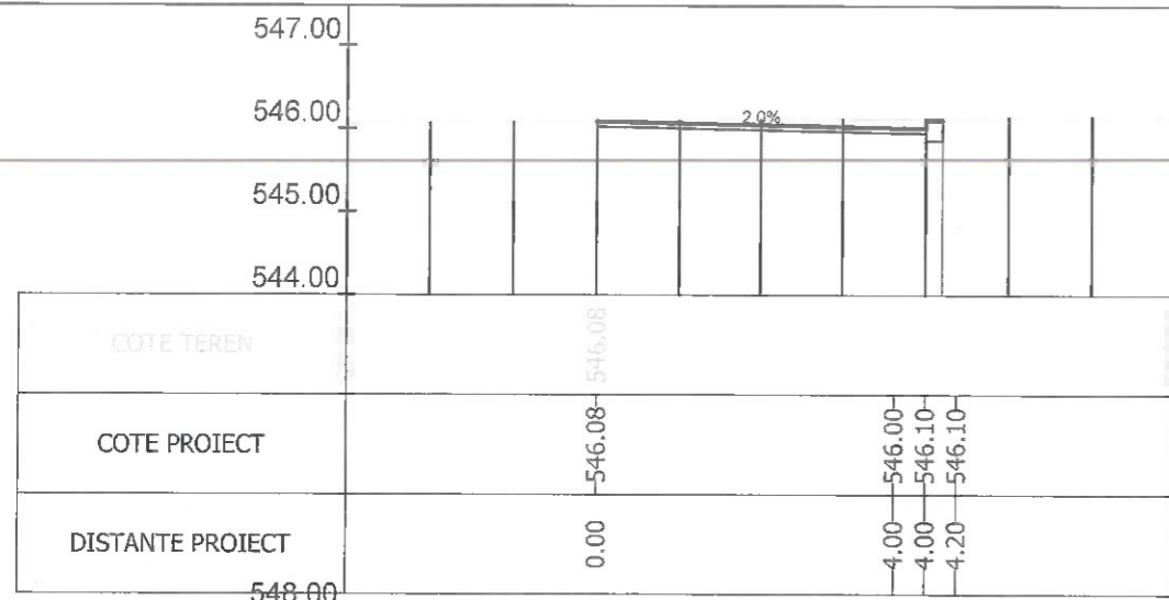
Sectiunea 3 - Km 0+050 Ax-Traseul 2
