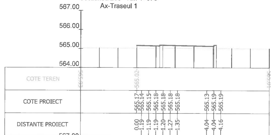
Sectiunea 295 - Km 4+100
