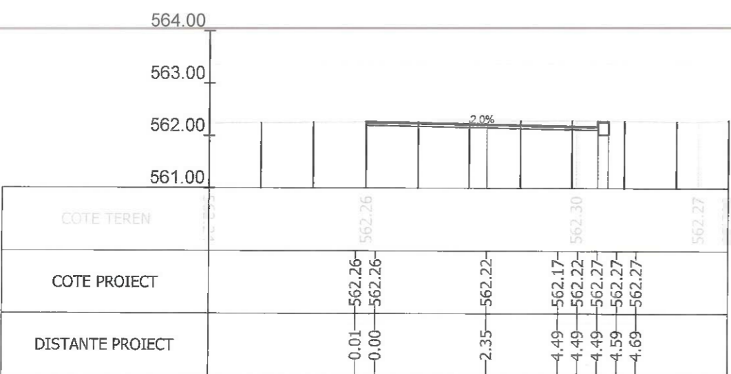
Sectiunea 83 - Km 1+375 Ax-Traseul 2
