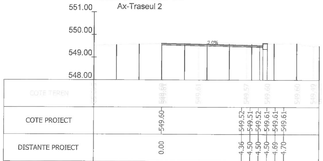
Sectiunea 32 - Km 0+475 Ax-Traseul 2
