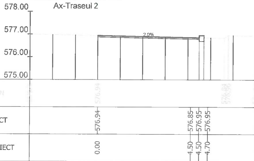
Sectiunea 190 - Km 2+804.233
