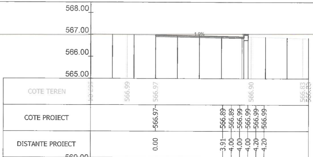
Sectiunea 263 - Km 3+607.563 Ax-Traseul 1
