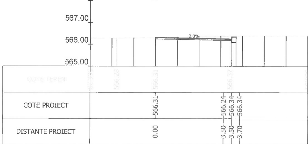
Sectiunea 9 - Km 0+100
