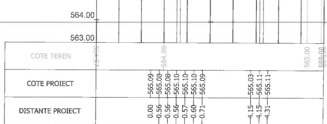
Sectiunea 297 - Km 4+126.386
