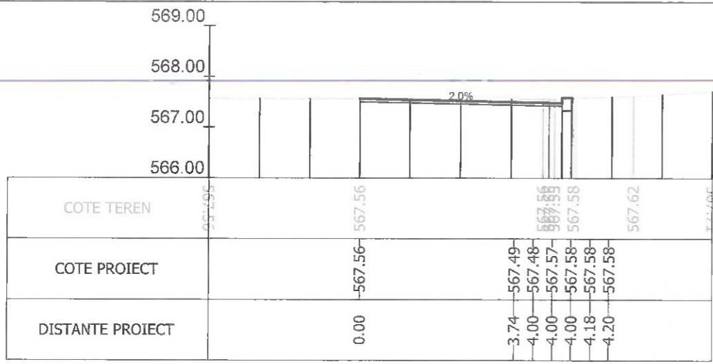
Sectiunea 224 - Km 3+070.200 Ax-Traseul 1
