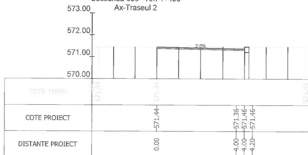
Sectiunea 305 - Km 4+500 Ax-Traseul 2
