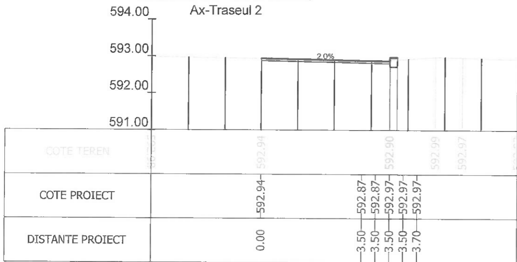
Sectiunea 422 - Km 6+192.447 Ax-Traceul 2
