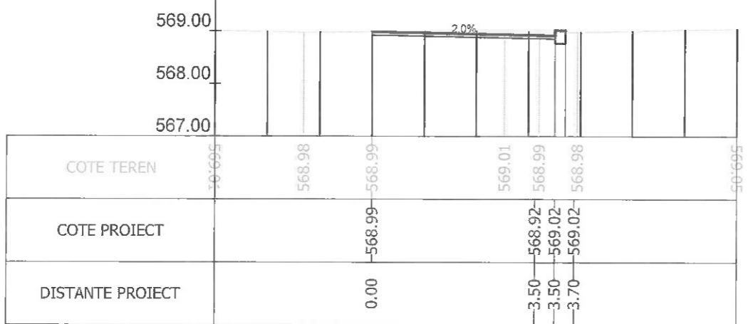
Sectiunea 431 - Km 5+800 Ax-Traseul 1
