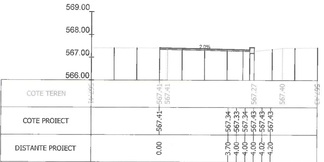
Sectiunea 266 - Km 3+675 Ax-Traseul 1
