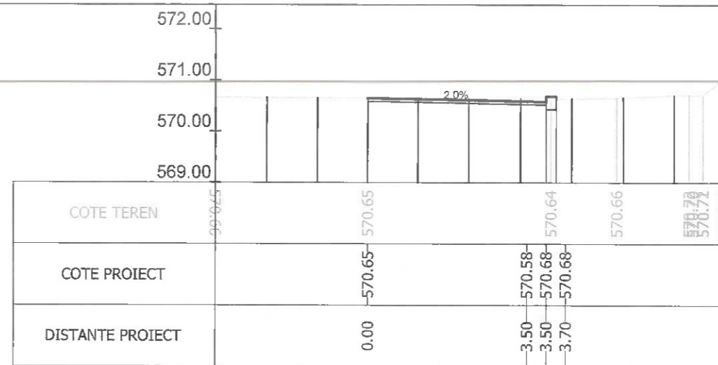
Sectiunea 424 - Km 5+700 Ax-Traseul 1
