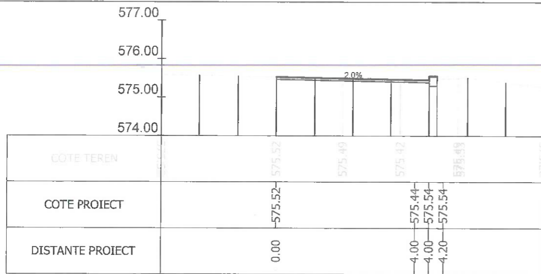
Sectiunea 200 - Km 2+894.819
