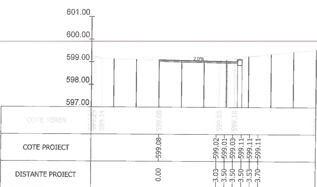
Sectiunea 460 - Km 6+825 Ax-Traseul 2
