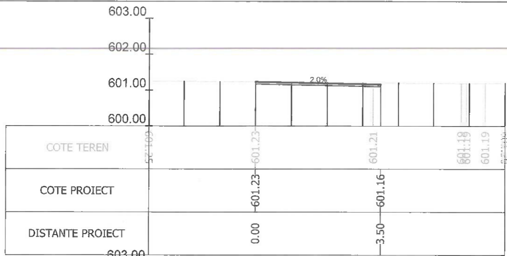
Sectiunea 15 - Km 0+103.169 Ax-Traseul 1
