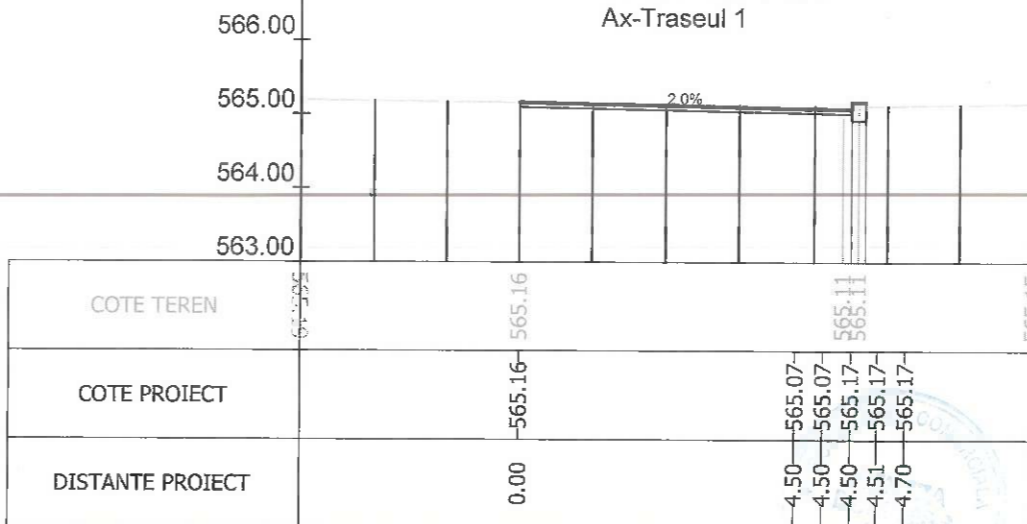
Sectiunea 303 - Km 4+203.970
