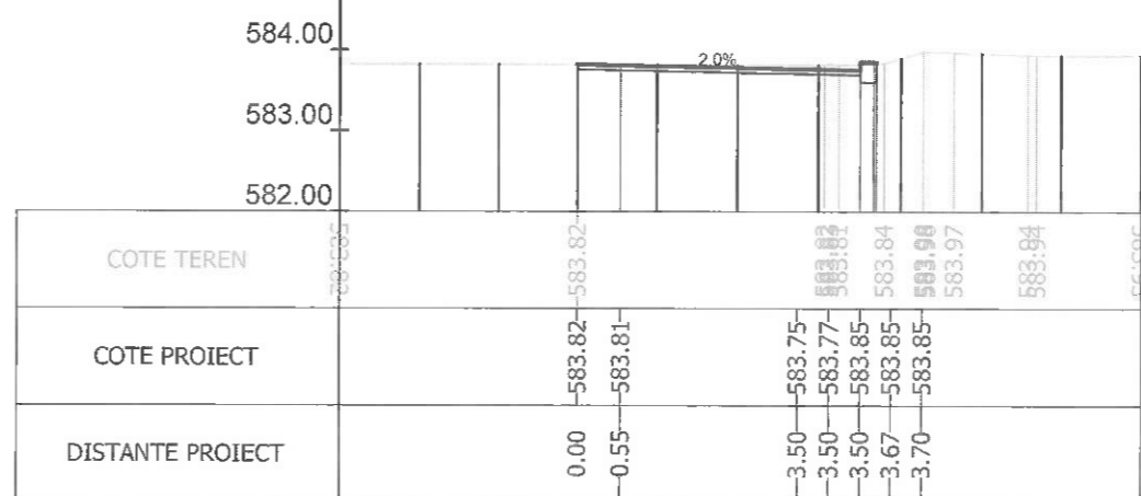
Sectiunea 121 - Km 1+675 Ax-Traseul 1
