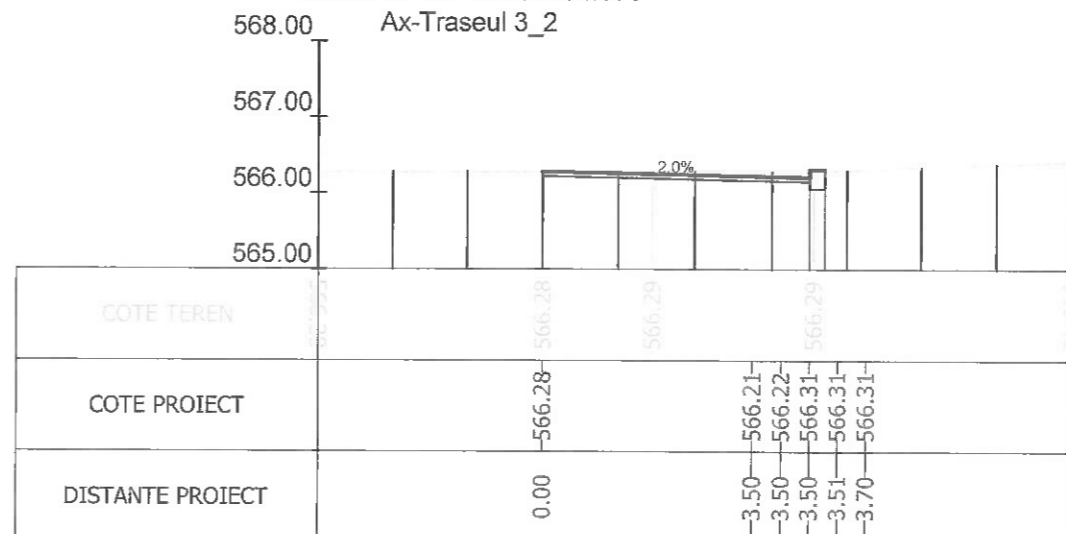
Sectiunea 40 - Km 0+524.505
