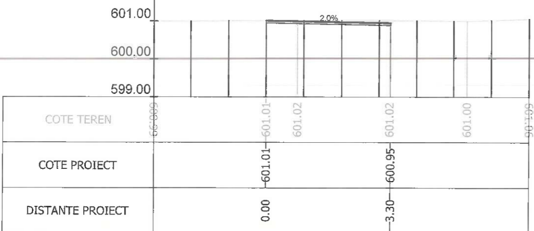
Sectiunea 19 - Km 0+138.615 Ax-Traseul 1
