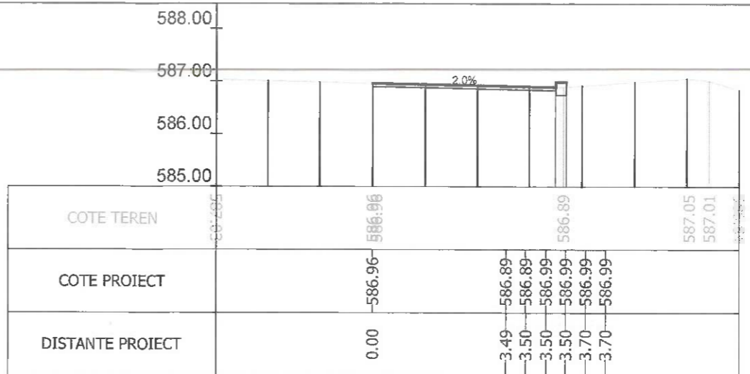
Sectiunea 101 - Km 1+392.440 Ax-Traseul 1
