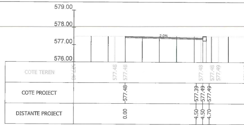
Sectiunea 384 - Km 5+300 Ax-Traseul 1
