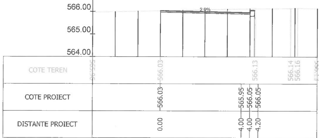
Sectiunea 245 - Km 3+346.491 Ax-Traseul 1
