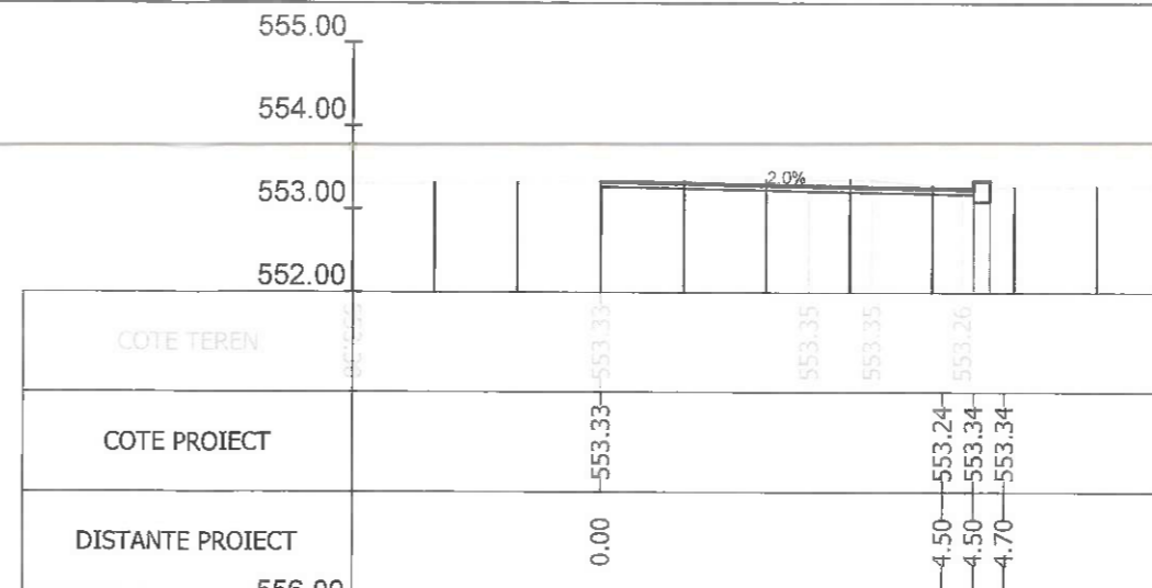
Sectiunea 49 - Km 0+800 Ax-Traseul 2
