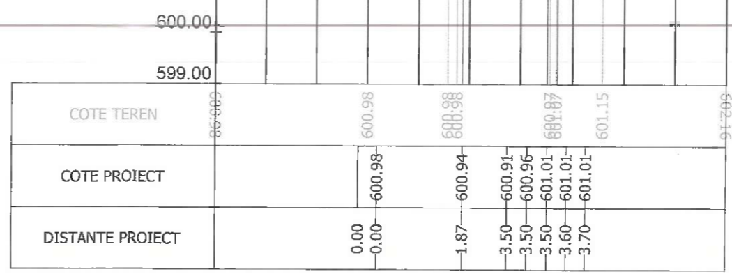
Sectiunea 33 - Km 0+325 Ax-Traseul 1
