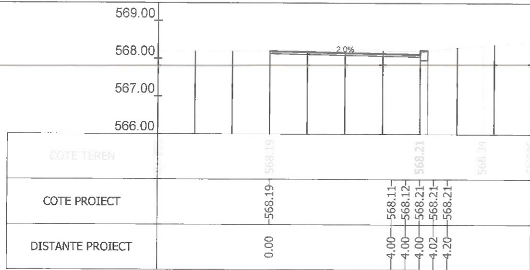
Sectiunea 284 - Km 4+170.989
