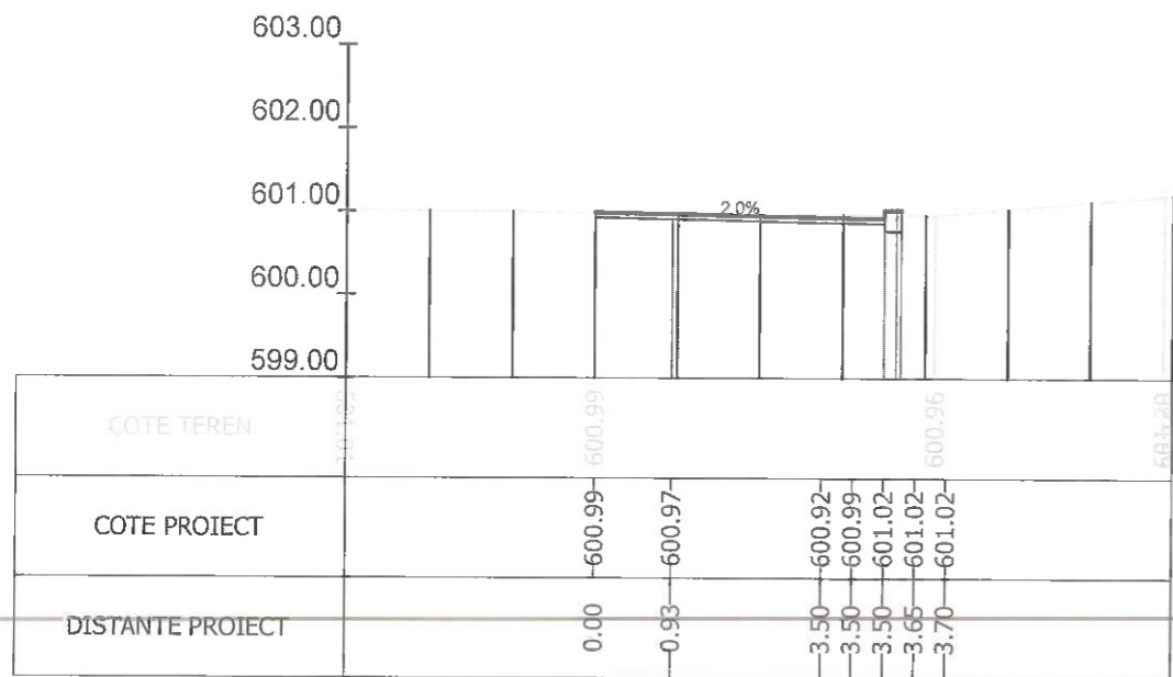
Sectiunea 464 - Km 6+925 Ax-Traseul 2
