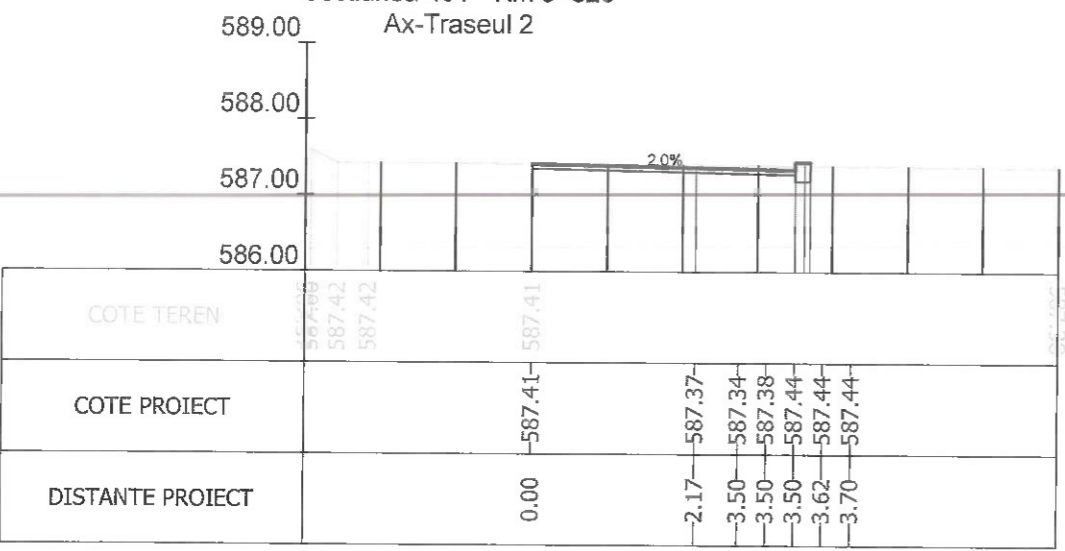
Sectiunea 403 - Km 5+875 Ax-Traseul 2
