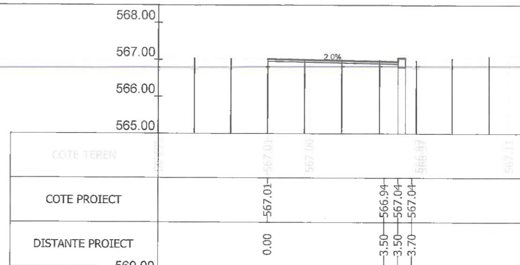
Sectiunea 48 - Km 0+618.168 Ax-Traseul 3_2
