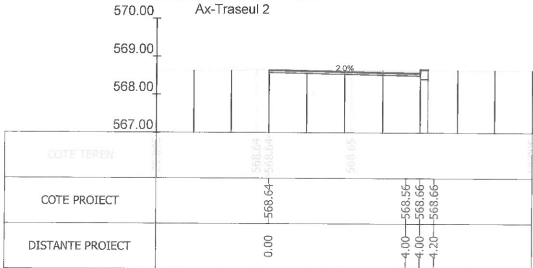
Sectiunea 286 - Km 4+200
