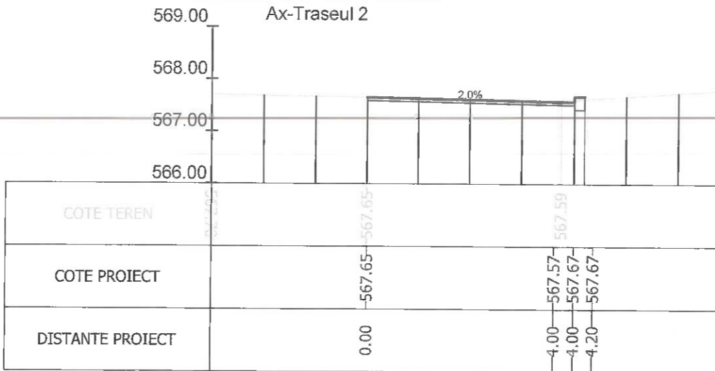
Sectiunea 277 - Km 4+100
