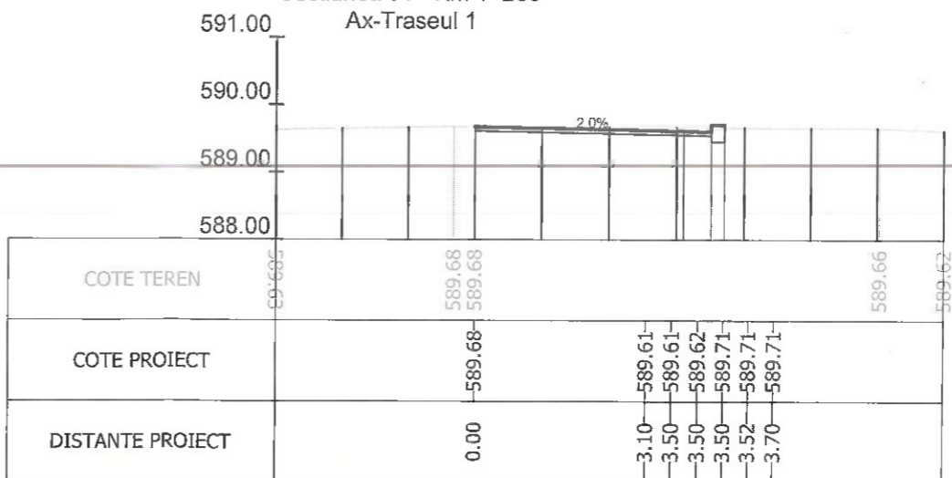
Sectiunea 93 - Km 1+275 Ax-Traseul 1
