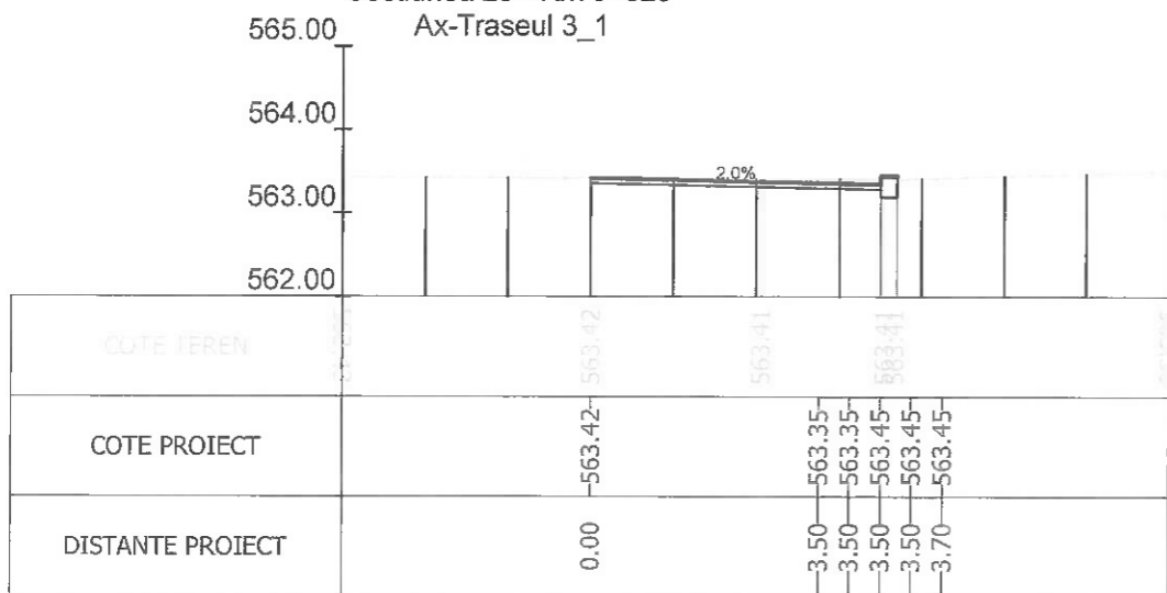
Sectiunea 27 - Km 0+368.749 Ax-Traseul 3_1
