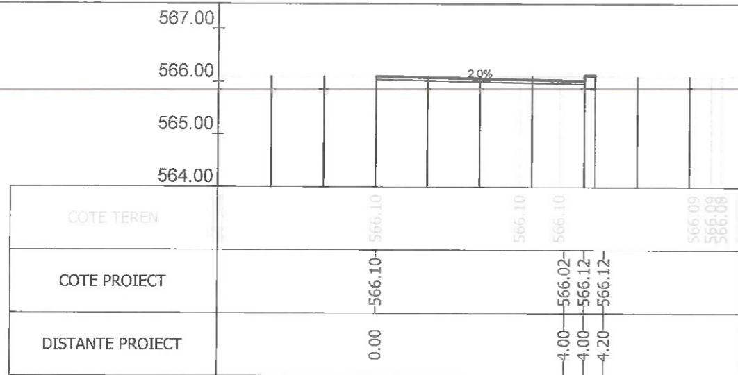
Sectiunea 248 - Km 3+600 Ax-Traseul 2
