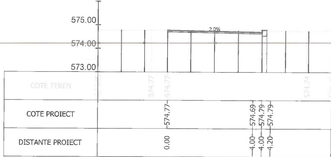
Sectiunea 205 - Km 2+950
