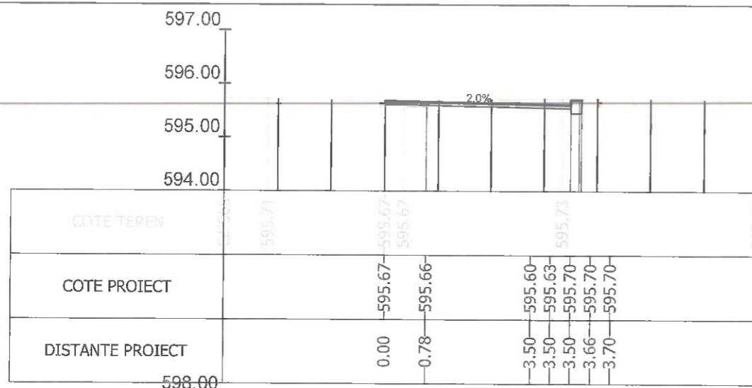
Sectiunea 438 - Km 6+450 Ax-Traseul 2
