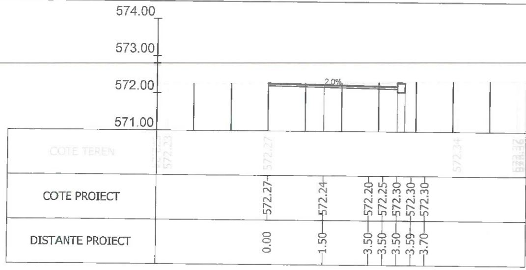
Sectiunea 127 - Km 1+975 Ax-Traseul 2
