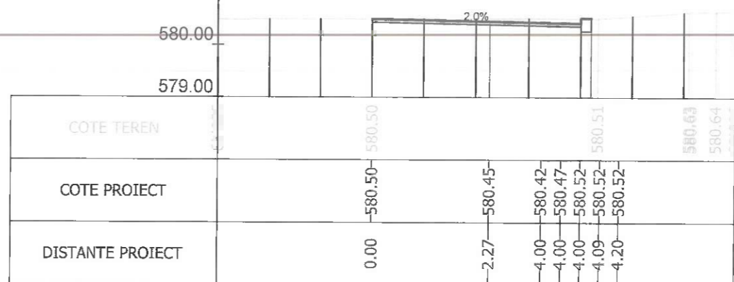
Sectiunea 362 - Km 5+250 Ax-Traseul 2
