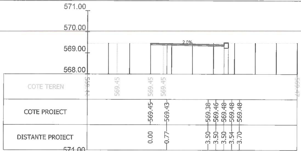
Sectiunea 429 - Km 5+775 Ax-Traseul 1
