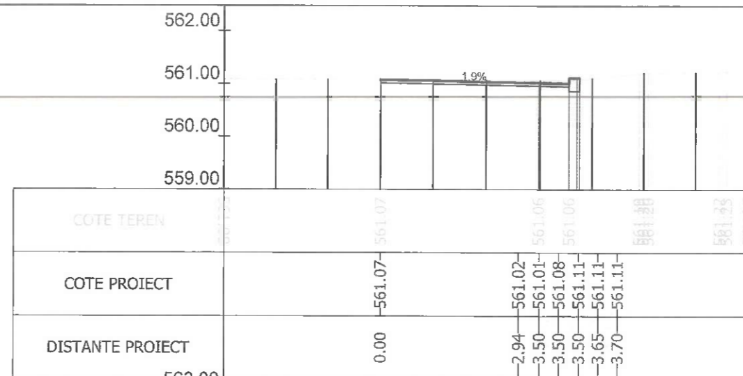
Sectiunea 2 - Km 0+010.322 Ax-Traseul 3_2
