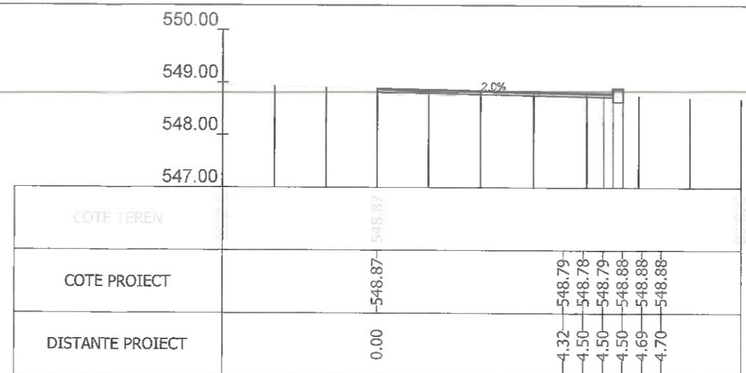
Sectiunea 31 - Km 0+450 Ax-Traseul 2
