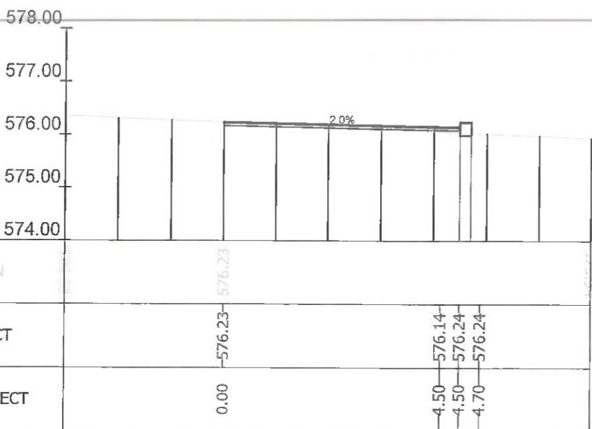
Sectiunea 192 - Km 2+821.758
