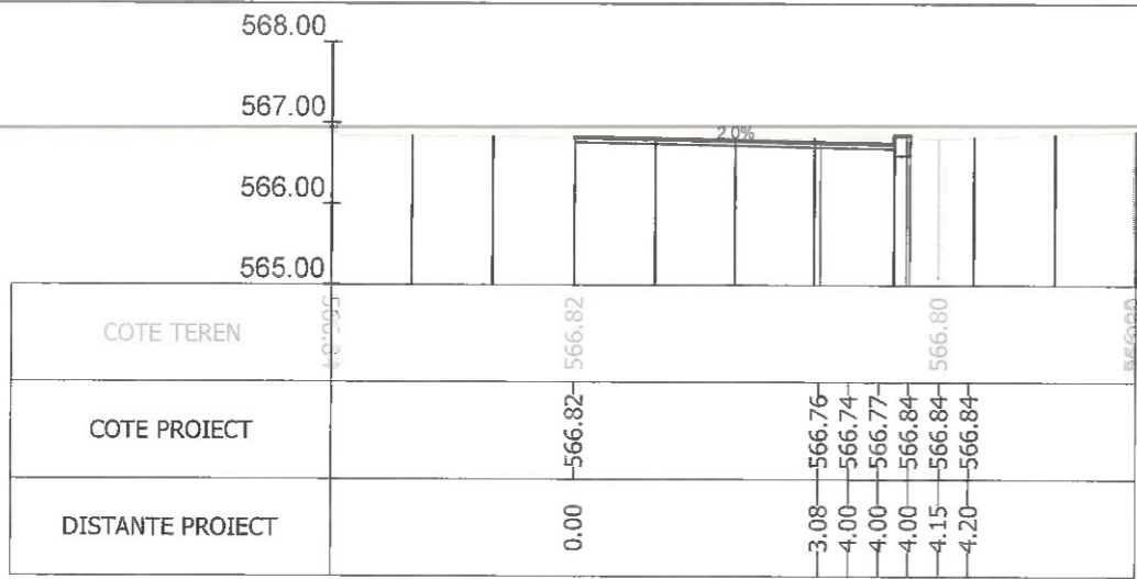
Sectiunea 231 - Km 3+175 Ax-Traseul 1
