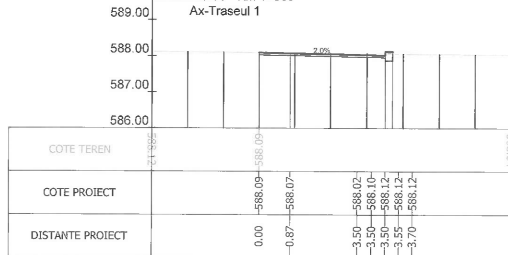
Sectiunea 97 - Km 1+325 Ax-Traseul 1
