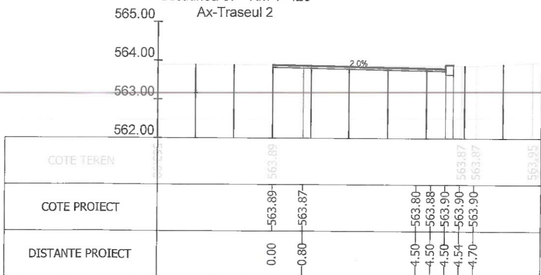
Sectiunea 89 - Km 1+475 Ax-Traseul 2
