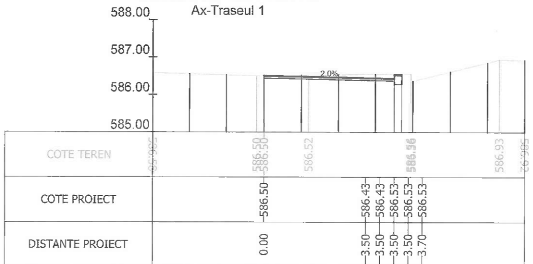
Sectiunea 103 - Km 1+408.577 Ax-Traseul 1
