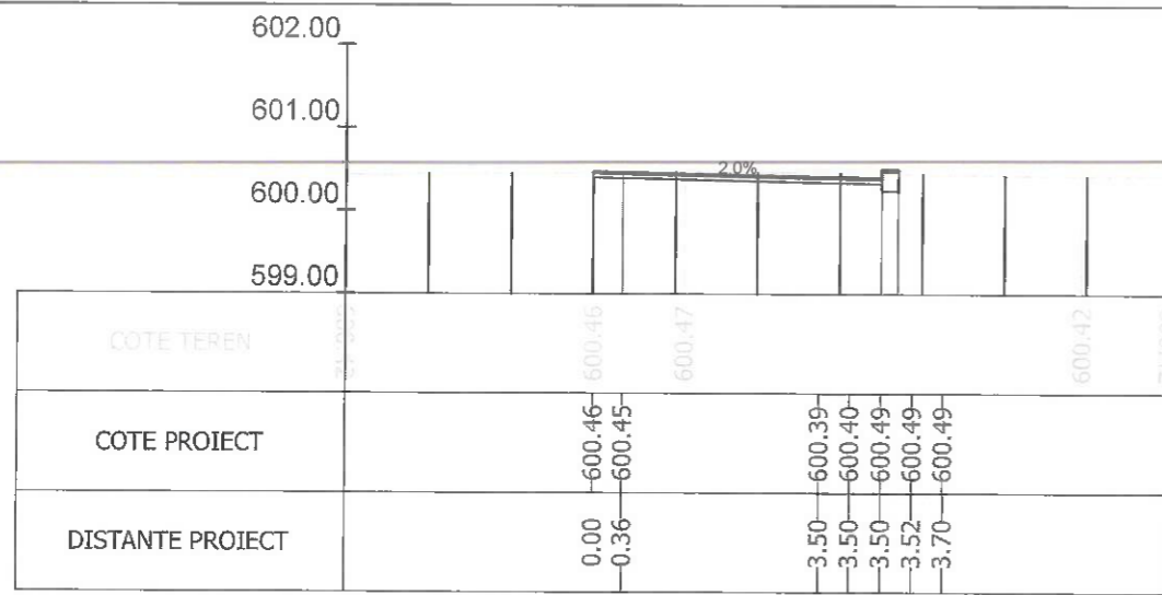
Sectiunea 462 - Km 6+875 Ax-Traseul 2
