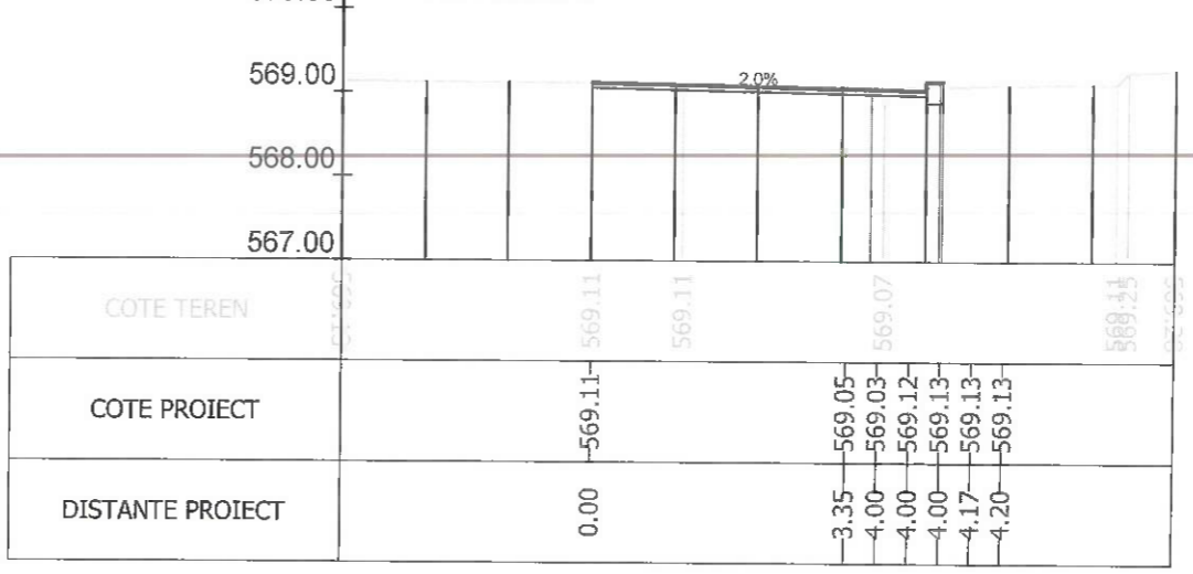
Sectiunea 289 - Km 4+250
