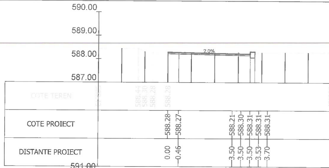
Sectiunea 405 - Km 5+925 Ax-Traseul 2
