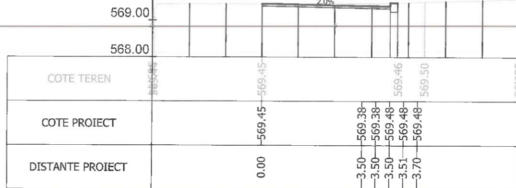
Sectiunea 428 - Km 5+770.571 Ax-Traseul 1
