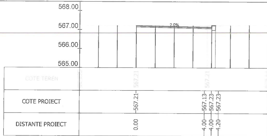
Sectiunea 272 - Km 4+000
