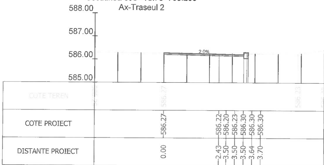
Sectiunea 395 - Km 5+750 Ax-Traseul 2
