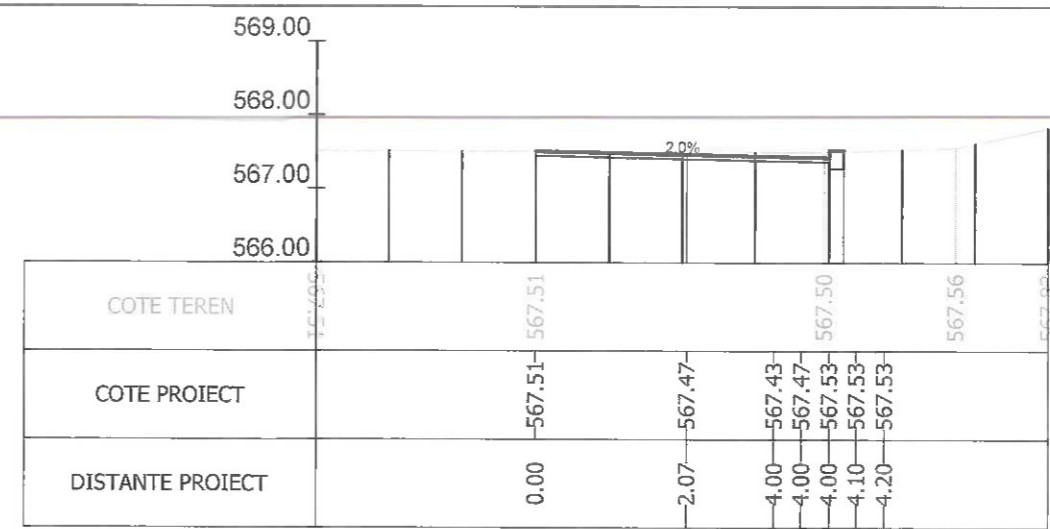
Sectiunea 225 - Km 3+075 Ax-Traseul 1
