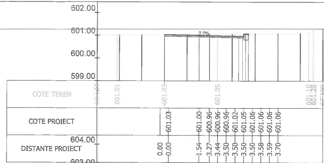
Sectiunea 29 - Km 0+267 Ax-Traseul 1
