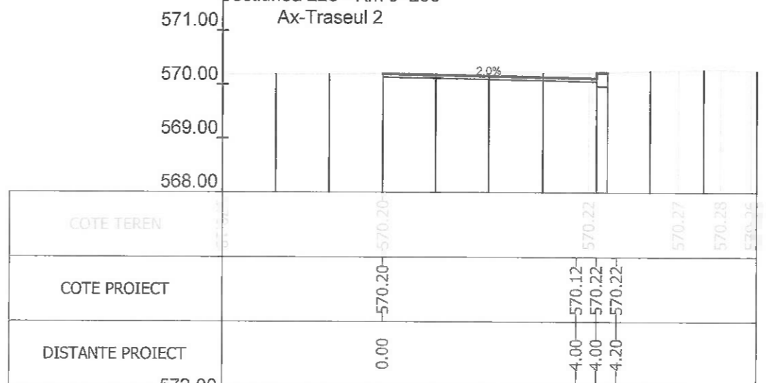
Sectiunea 227 - Km 3+300 Ax-Traseul 2
