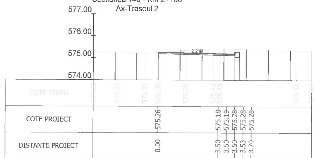
Sectiunea 142 - Km 2+144.542 Ax-Traseul 2
