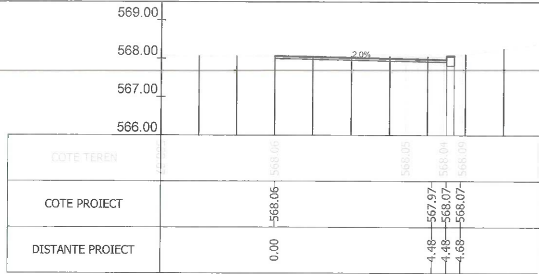
Sectiunea 108 - Km 1+725.215 Ax-Traseul 2
