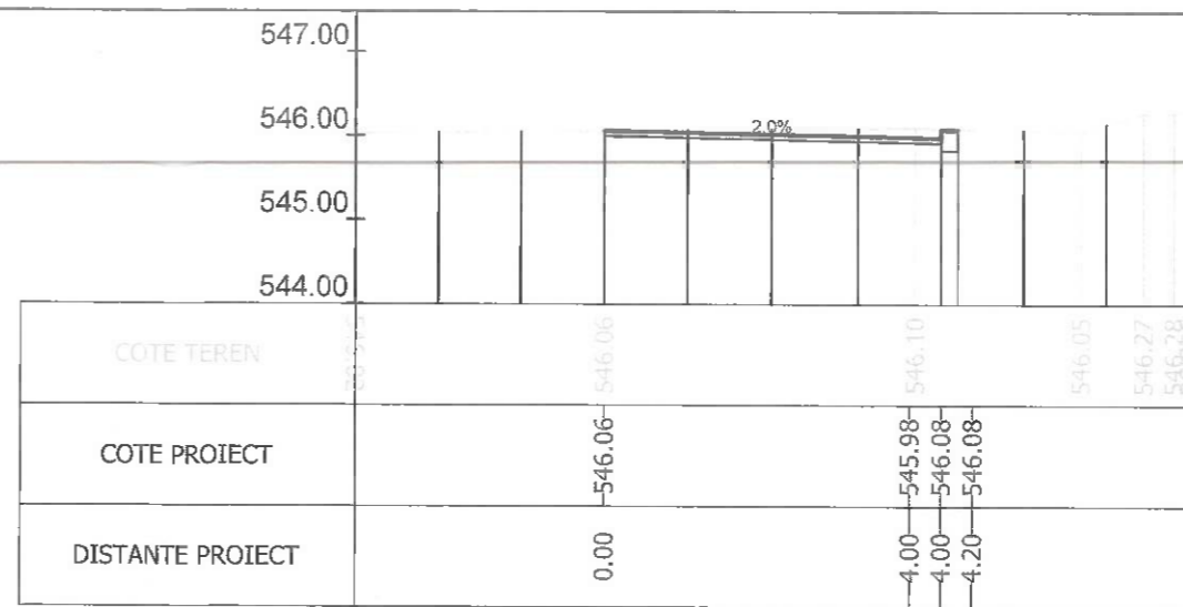
Sectiunea 4 - Km 0+063.802 Ax-Traseul 2
