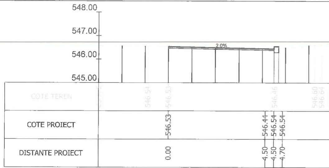
Sectiunea 12 - Km 0+148.927
