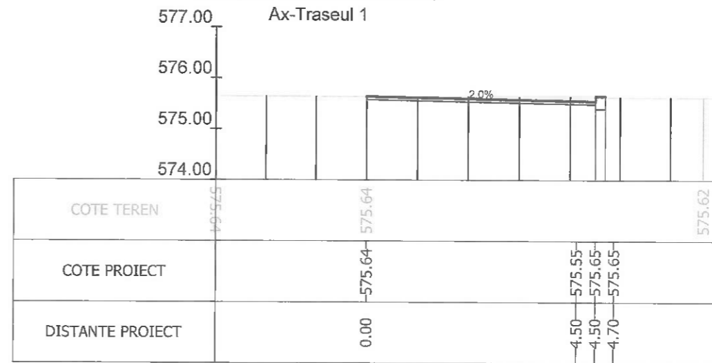
Sectiunea 368 - Km 4+963.278
