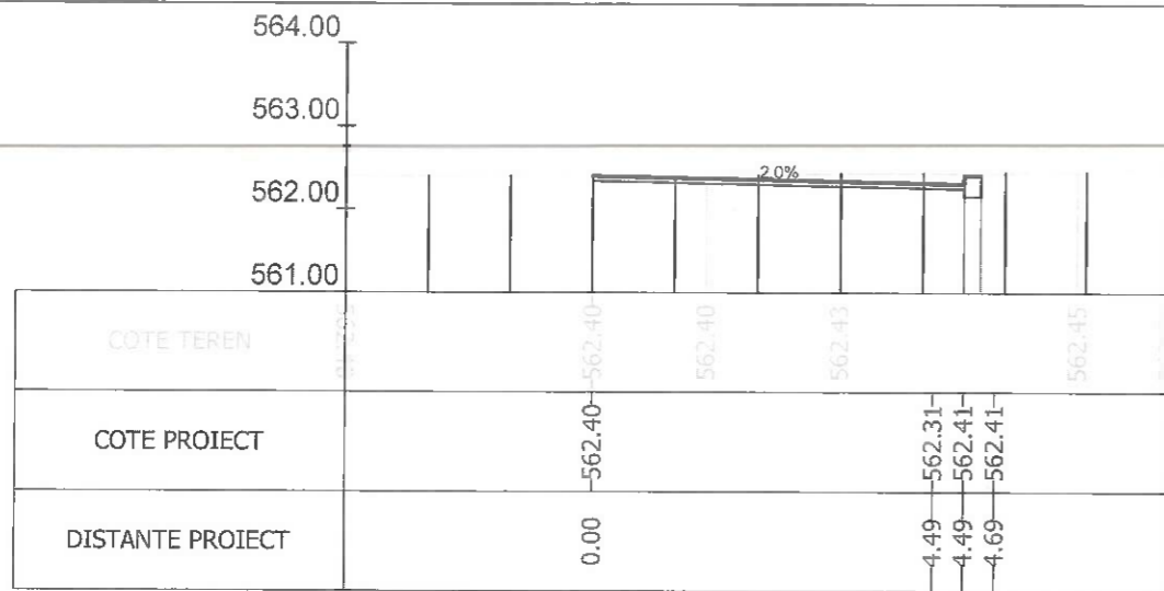
Sectiunea 84 - Km 1+391.567 Ax-Traseul 2
