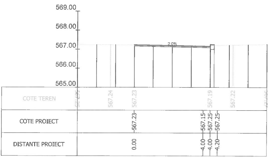
Sectiunea 226 - Km 3+100 Ax-Traseul 1
