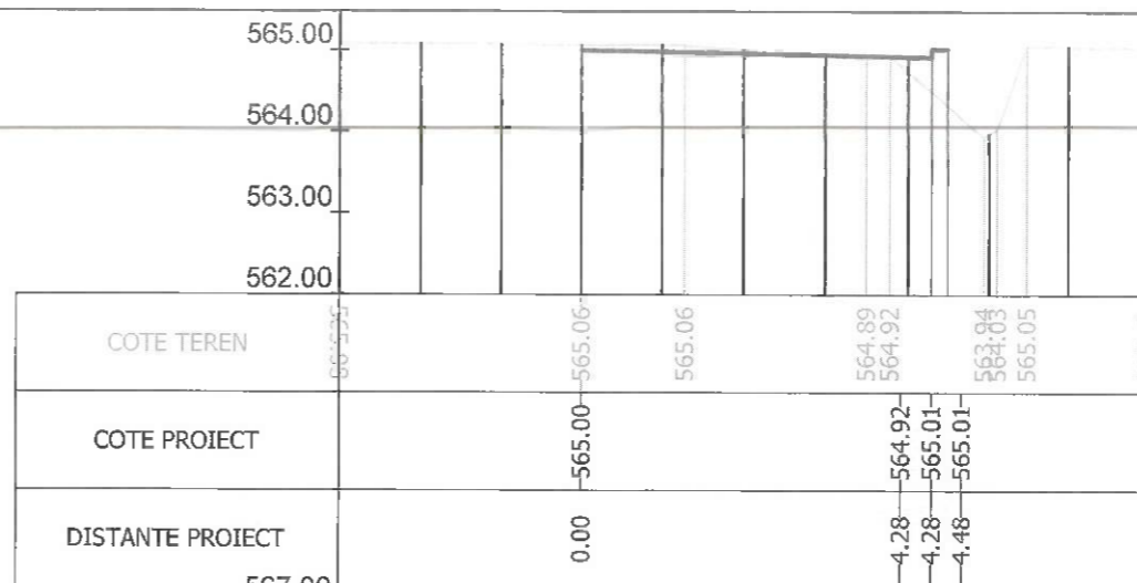
Sectiunea 299 - Km 4+155.384 Ax-Traseul 1
