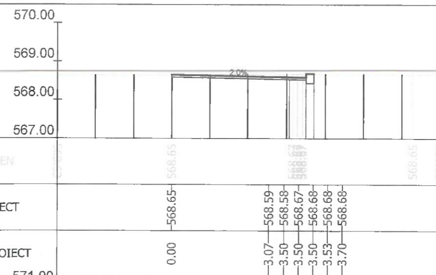
Sectiunea 110 - Km 1+750 Ax-Traseul 2
