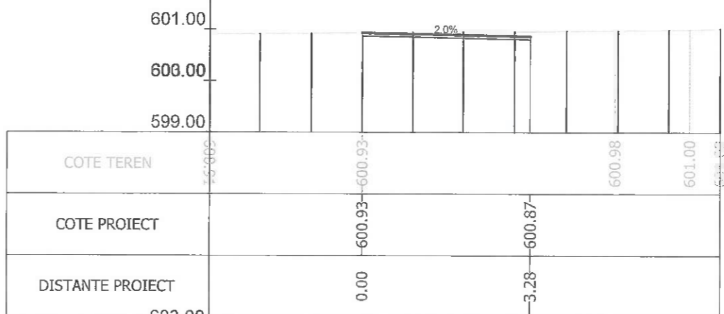
Sectiunea 18 - Km 0+128.325 Ax-Traseul 1
