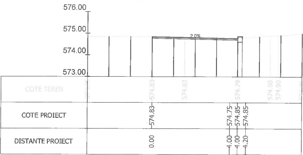
Sectiunea 204 - Km 2+928.965
