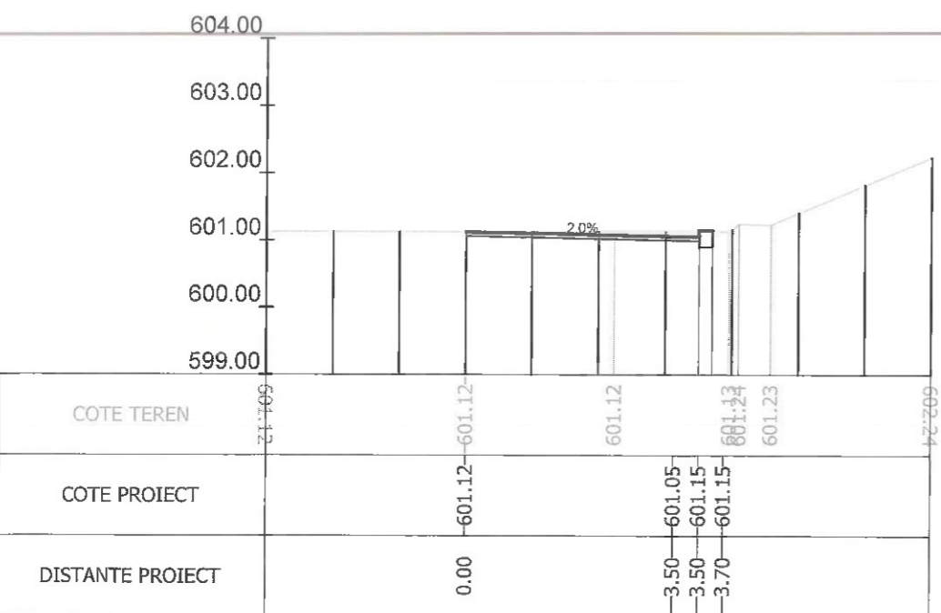
Sectiunea 32 - Km 0+300 Ax-Traseul 1
