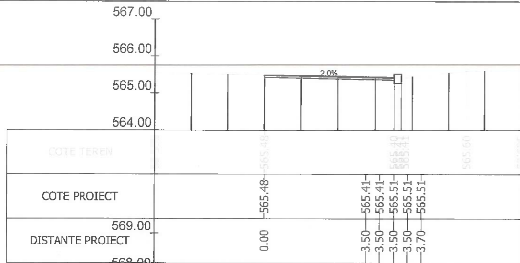
Sectiunea 13 - Km 0+167.654 Ax-Traseul 3_1
