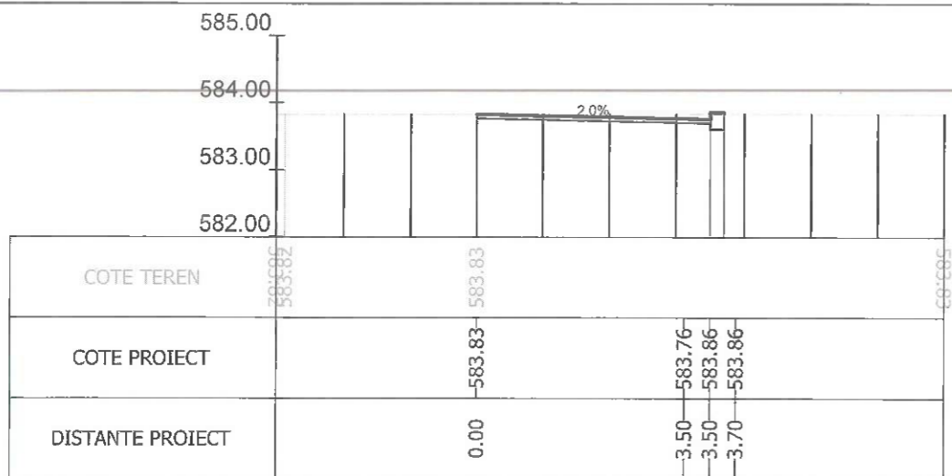
Sectiunea 124 - Km 1+700 Ax-Traseul 1
