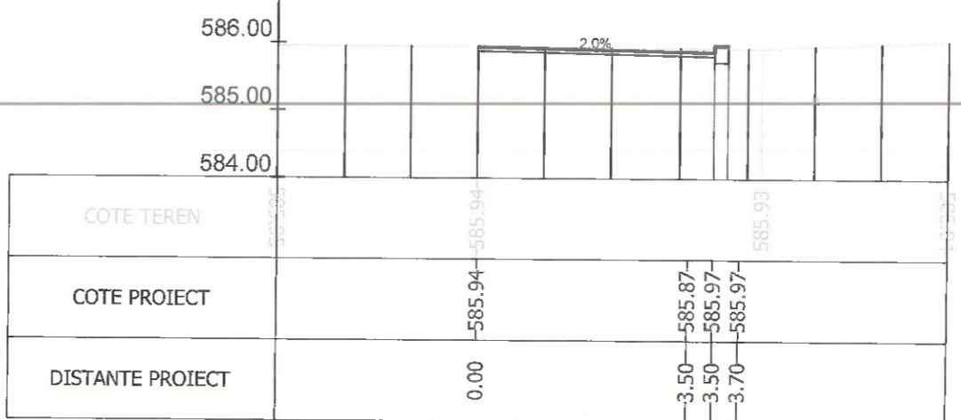
Sectiunea 392 - Km 5+700 Ax-Traseul 2
