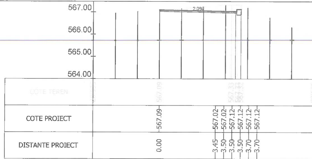
Sectiunea 37 - Km 0+478.413
