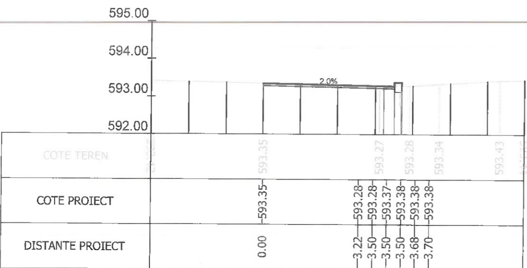
Sectiunea 424 - Km 6+218.755 Ax-Traceul 2
