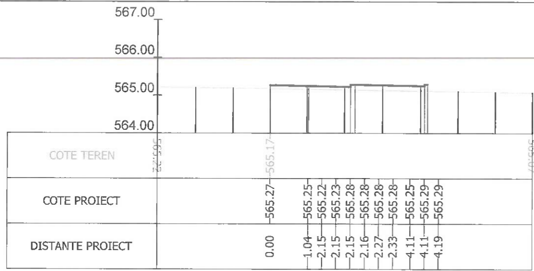
Sectiunea 292 - Km 4+068.619
