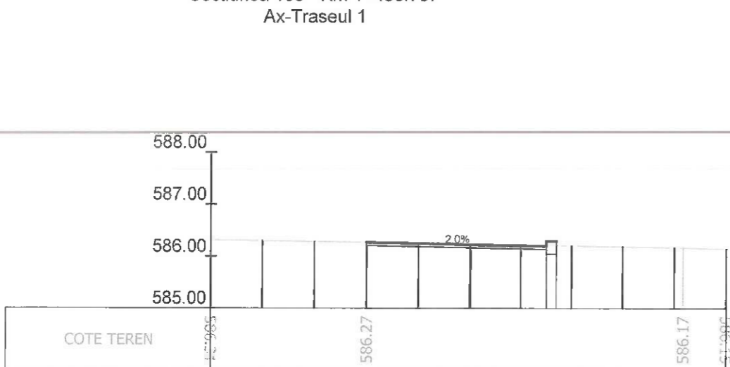
Sectiunea 108 - Km 1+486.737
