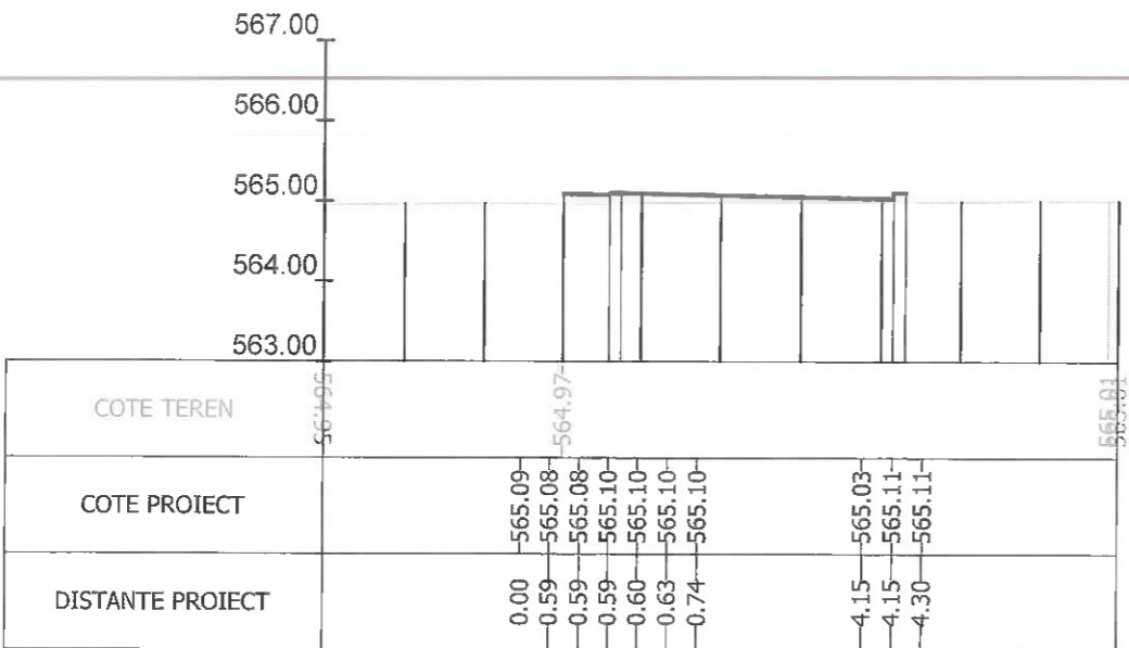
Sectiunea 296 - Km 4+125
