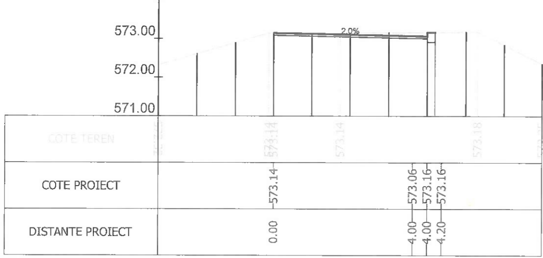
Sectiunea 292 - Km 4+300 Ax-Traseul 2
