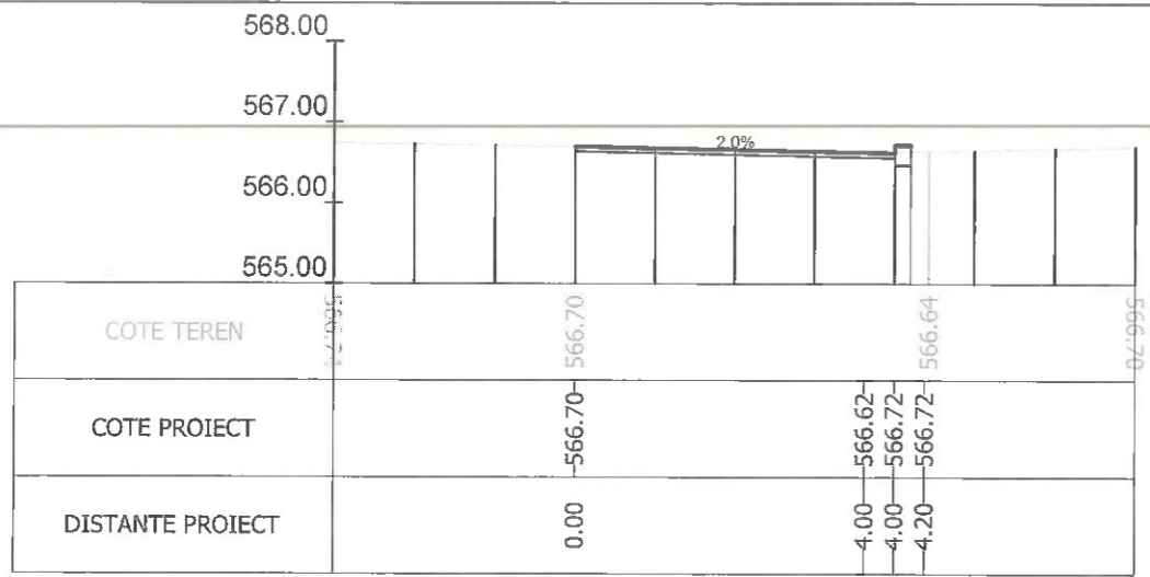
Sectiunea 262 - Km 3+600 Ax-Traseul 1
