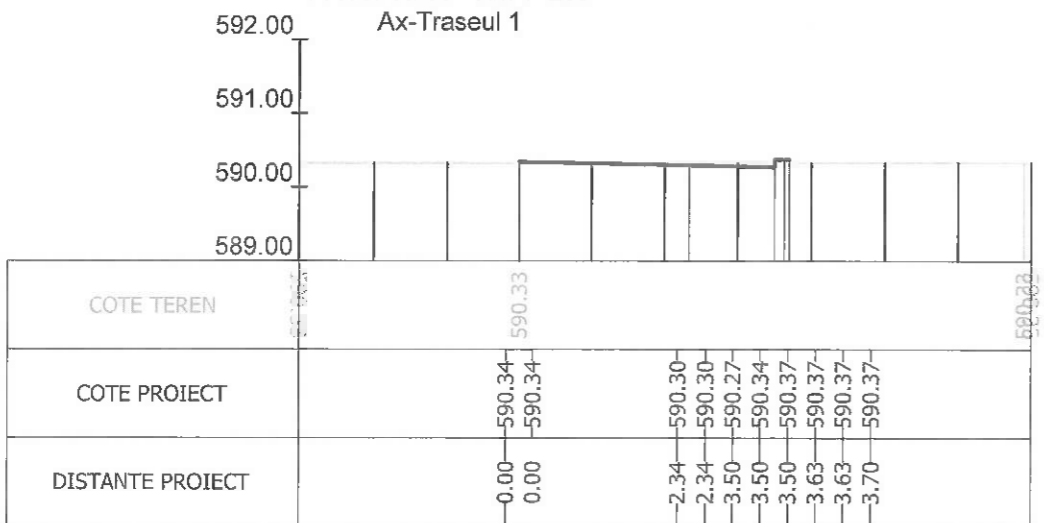
Sectiunea 90 - Km 1+225 Ax-Traseul 1
