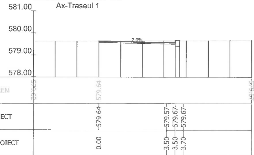
Sectiunea 158 - Km 2+100 Ax-Traseul 1
