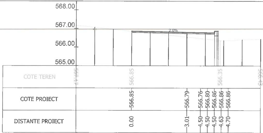
Sectiunea 280 - Km 3+850 Ax-Traseul 1
