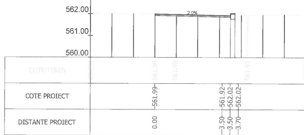
Sectiunea 40 - Km 0+525 Ax-Traseul 3_1
