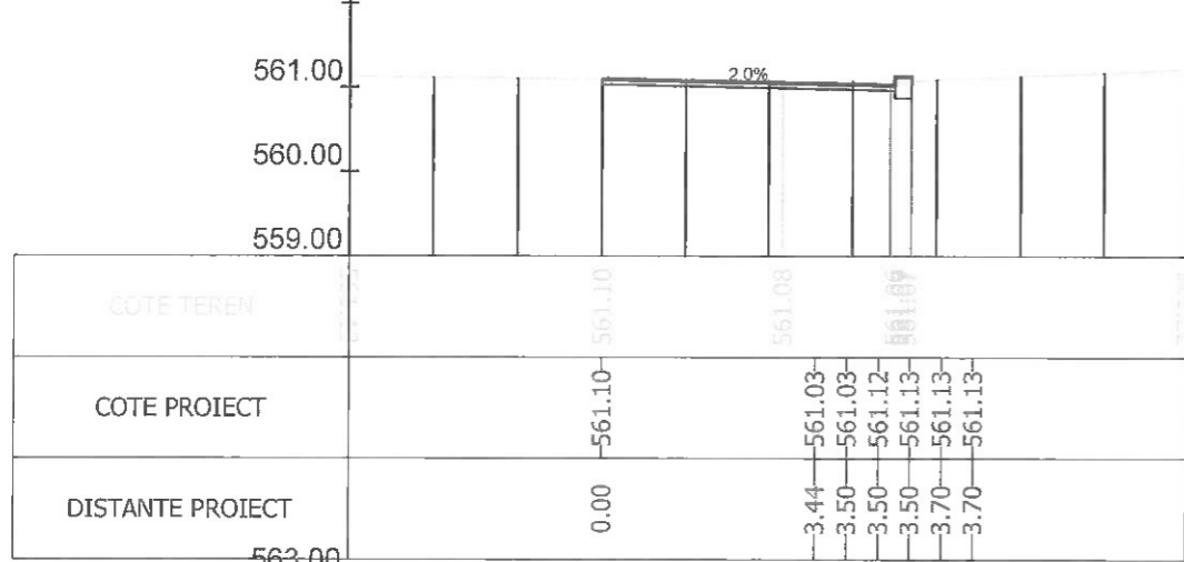
Sectiunea 3 - Km 0+017.825 Ax-Traseul 3_2
