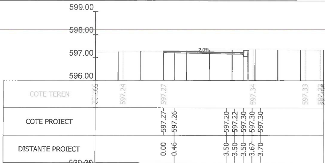
Sectiunea 46 - Km 0+550 Ax-Traseul 1
