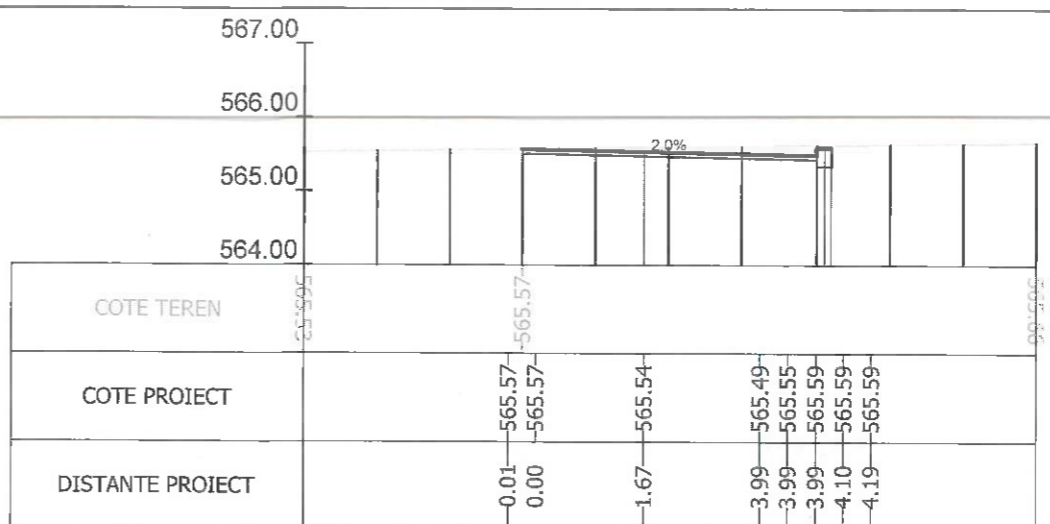
Sectiunea 250 - Km 3+425 Ax-Traseul 1
