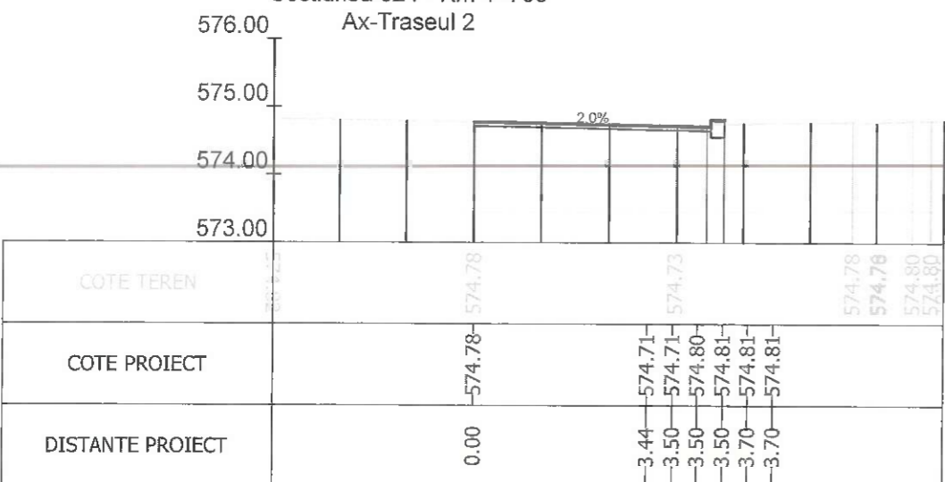
Sectiunea 326 - Km 4+729.059
