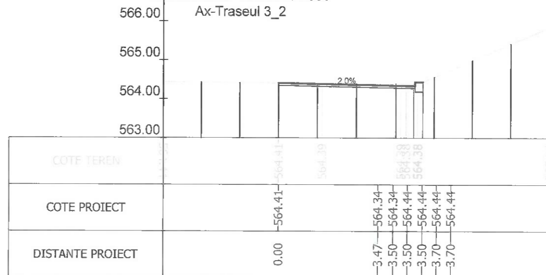
Sectiunea 27 - Km 0+358.010 Ax-Traseul 3_2
