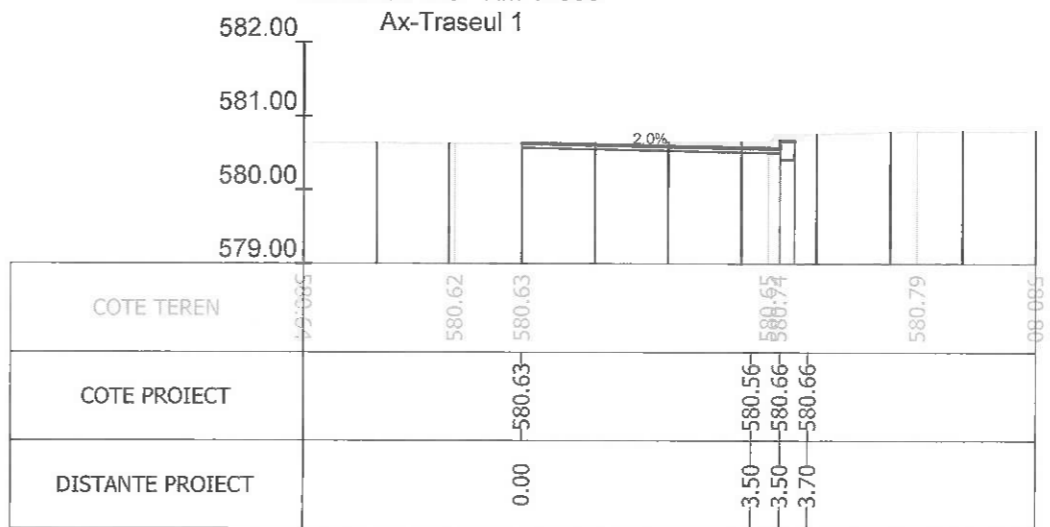
Sectiunea 145 - Km 1+982.925 Ax-Traseul 1
