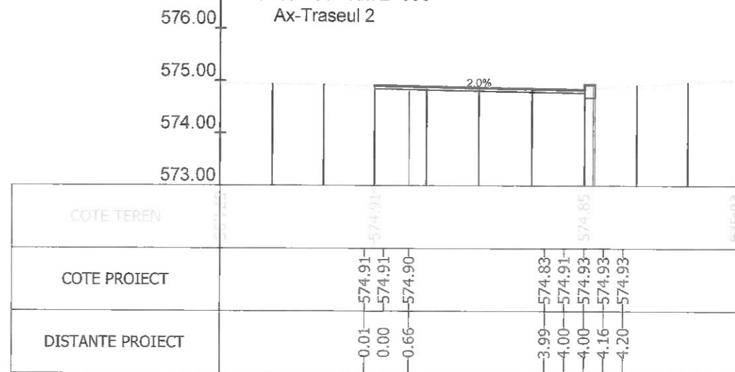
Sectiunea 203 - Km 2+925
