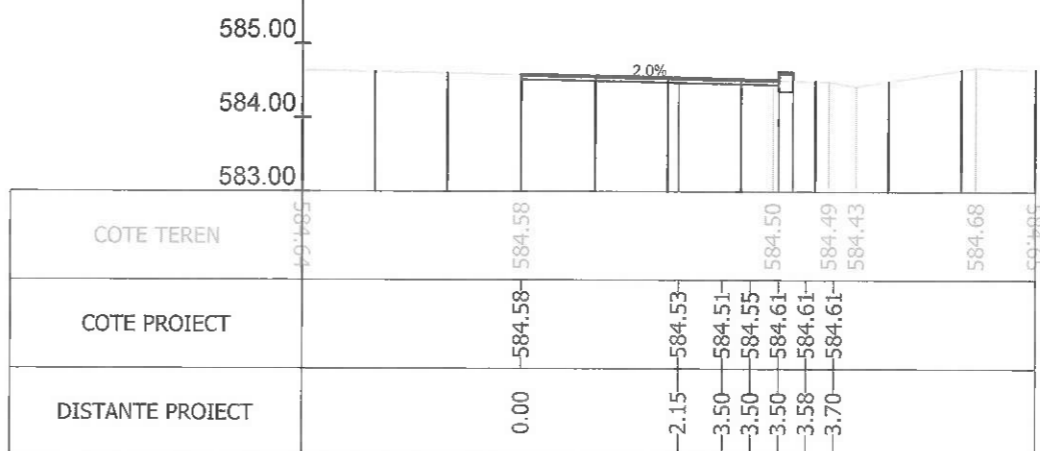
Sectiunea 115 - Km 1+625 Ax-Traseul 1
