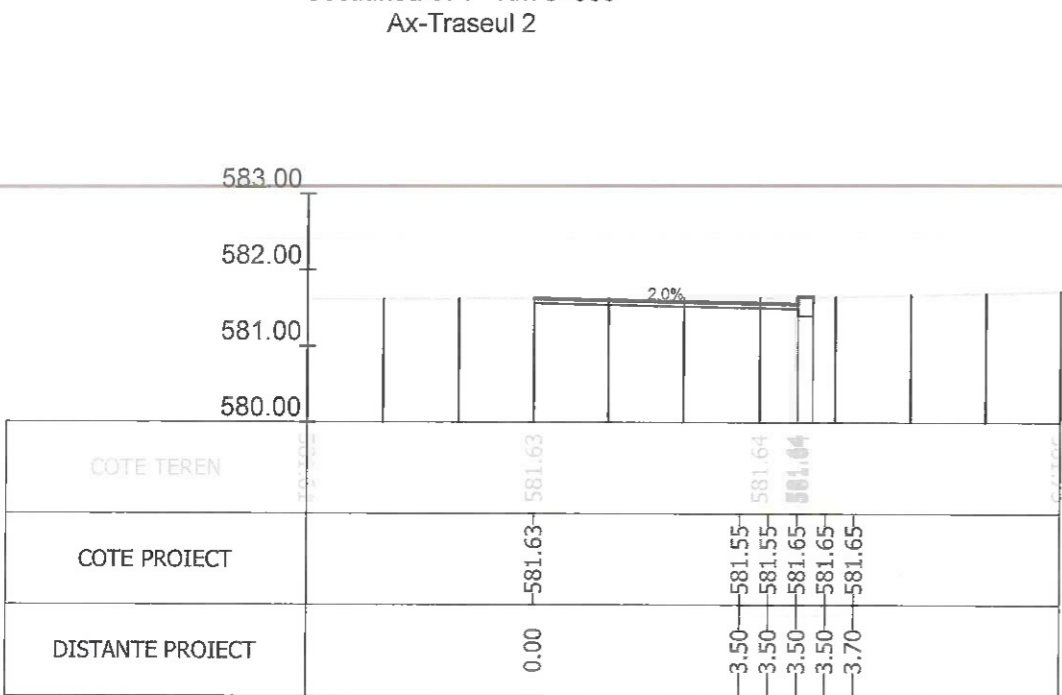
Sectiunea 373 - Km 5+370.688
