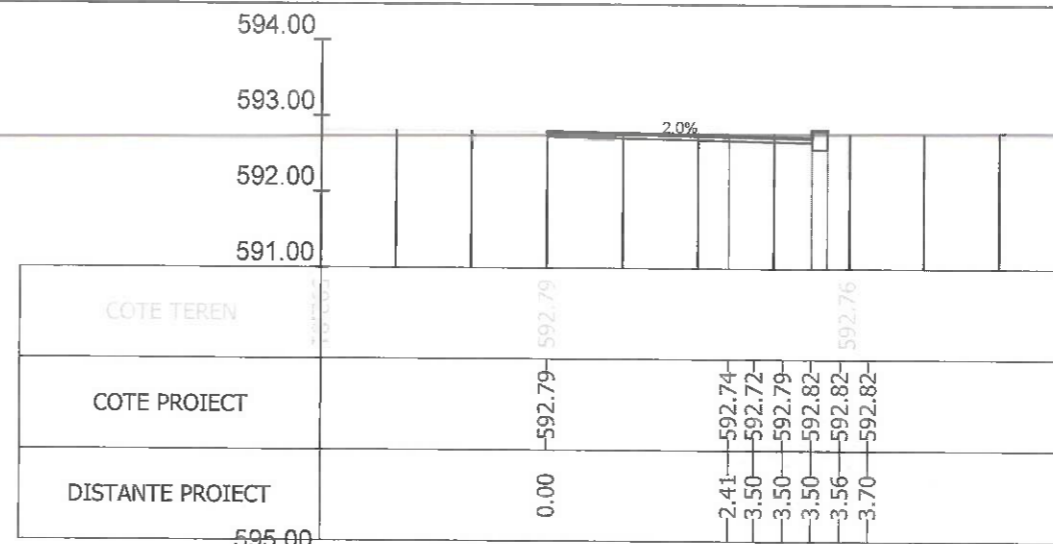
Sectiunea 421 - Km 6+175 Ax-Traceul 2
