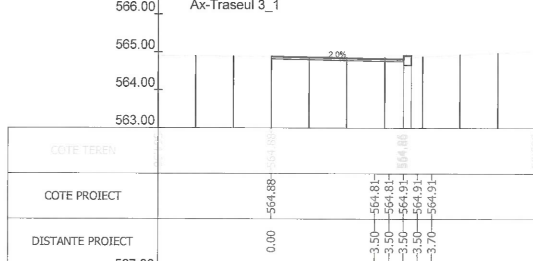
Sectiunea 16 - Km 0+221.372 Ax-Traseul 3_1
