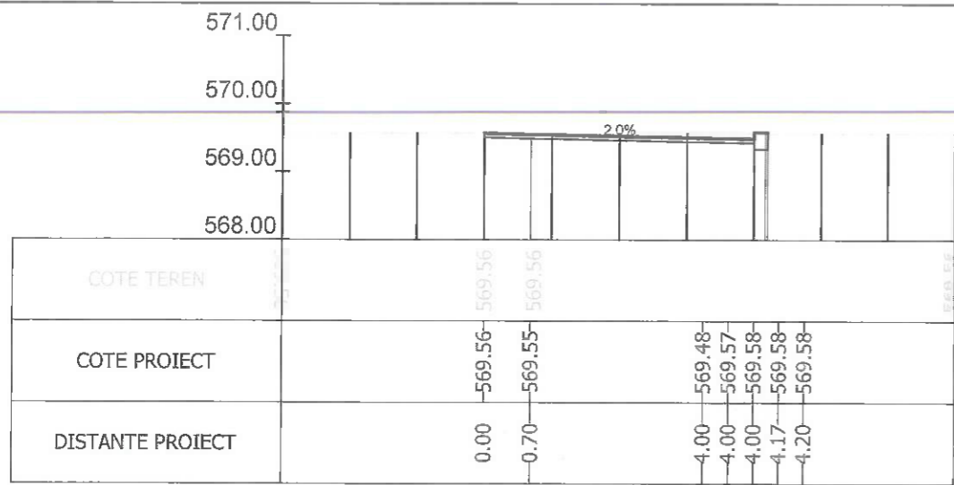
Sectiunea 236 - Km 3+350 Ax-Traseul 2
