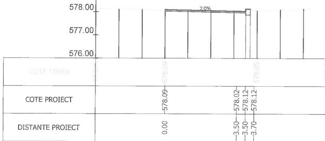
Sectiunea 342 - Km 5+015.780 Ax-Traceul 2
