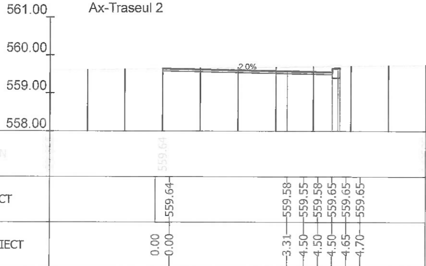
Sectiunea 74 - Km 1+225 Ax-Traseul 2
