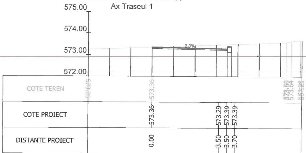
Sectiunea 410 - Km 5+550
