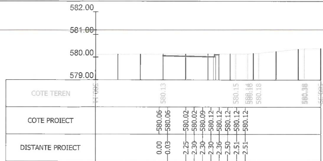
Sectiunea 149 - Km 2+025 Ax-Traseul 1
