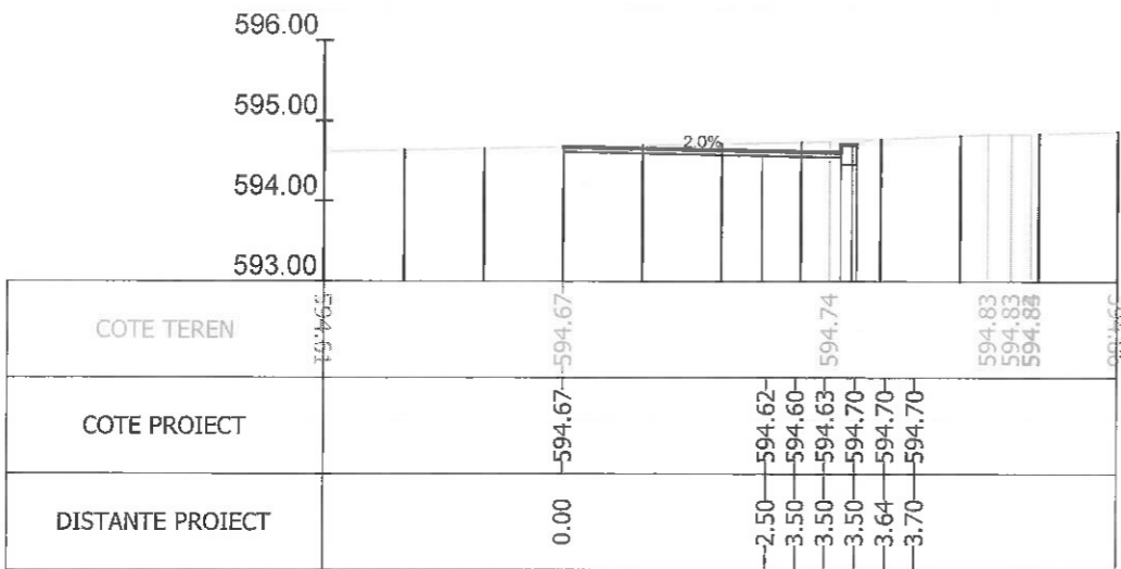
Sectiunea 68 - Km 0+925 Ax-Traseul 1
