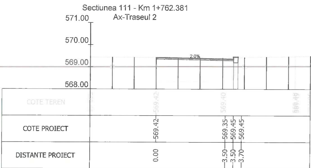
Sectiunea 111 - Km 1+762.381 Ax-Traseul 2
