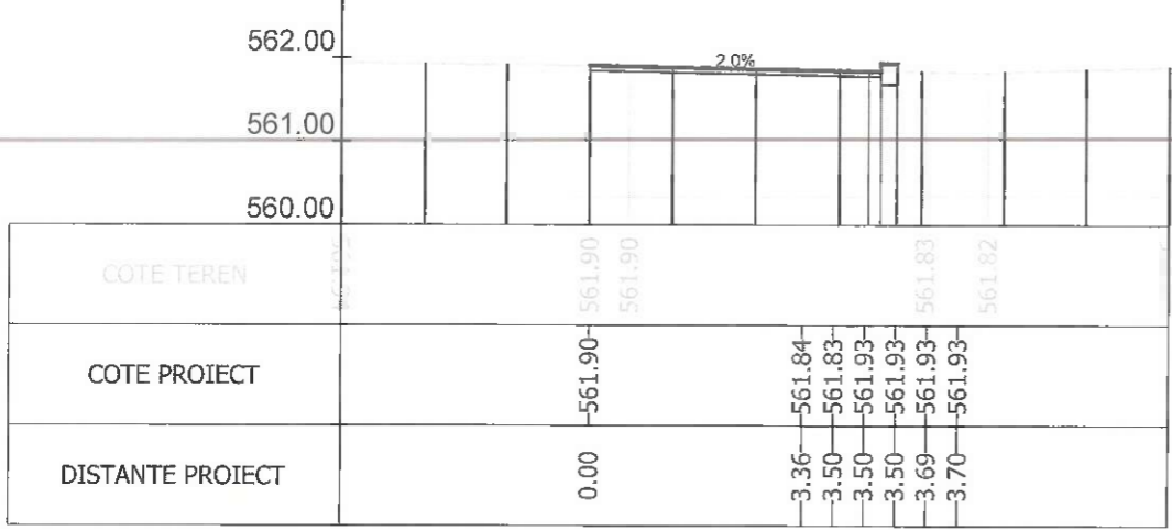
Sectiunea 41 - Km 0+532.427 Ax-Traseul 3_1
