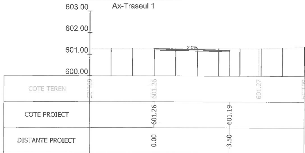
Sectiunea 11 - Km 0+069.738 Ax-Traseul 1
