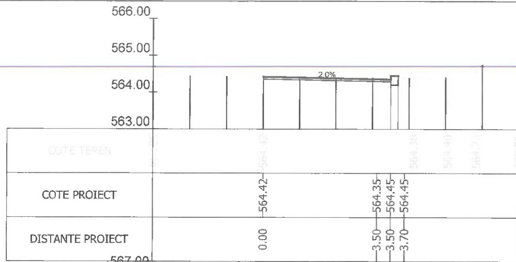
Sectiunea 25 - Km 0+350 Ax-Traseul 3_2
