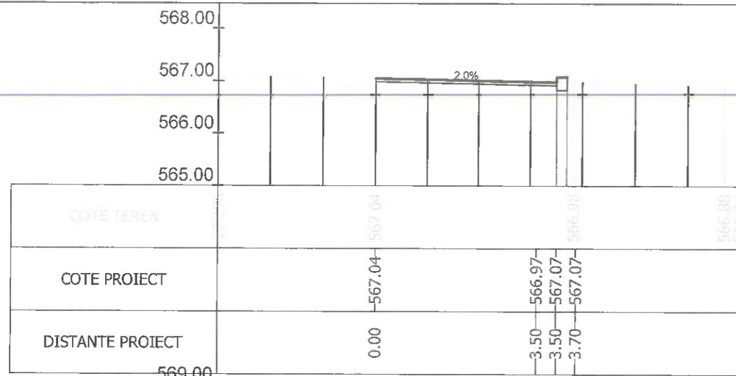
Sectiunea 47 - Km 0+603.332 Ax-Traseul 3_2
