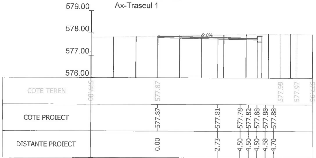
Sectiunea 379 - Km 5+175 Ax-Traseul 1
