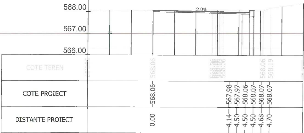
Sectiunea 105 - Km 1+700 Ax-Traseul 2
