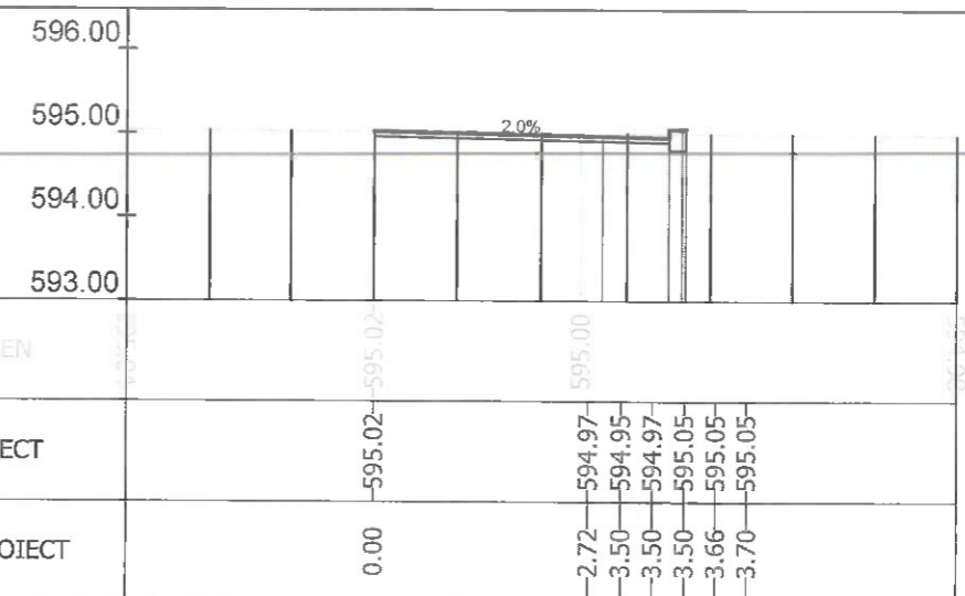
Sectiunea 433 - Km 6+350 Ax-Traseul 2
