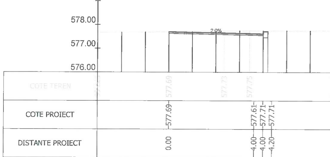
Sectiunea 184 - Km 2+752.645
