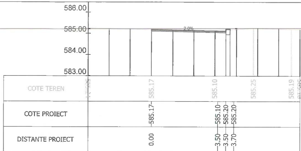
Sectiunea 113 - Km 1+600 Ax-Traseul 1
