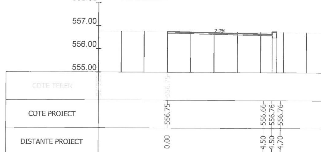
Sectiunea 63 - Km 1+050 Ax-Traseul 2
