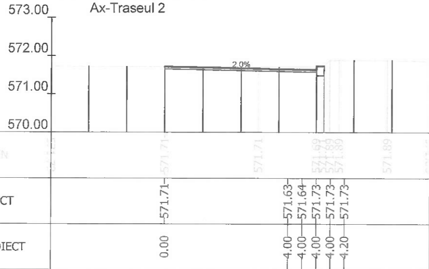
Sectiunea 310 - Km 4+556.043
