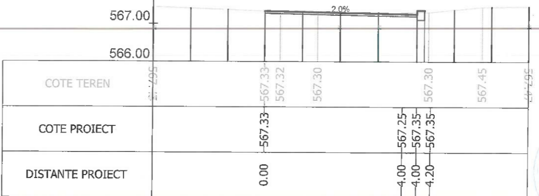
Sectiunea 267 - Km 3+679.003
