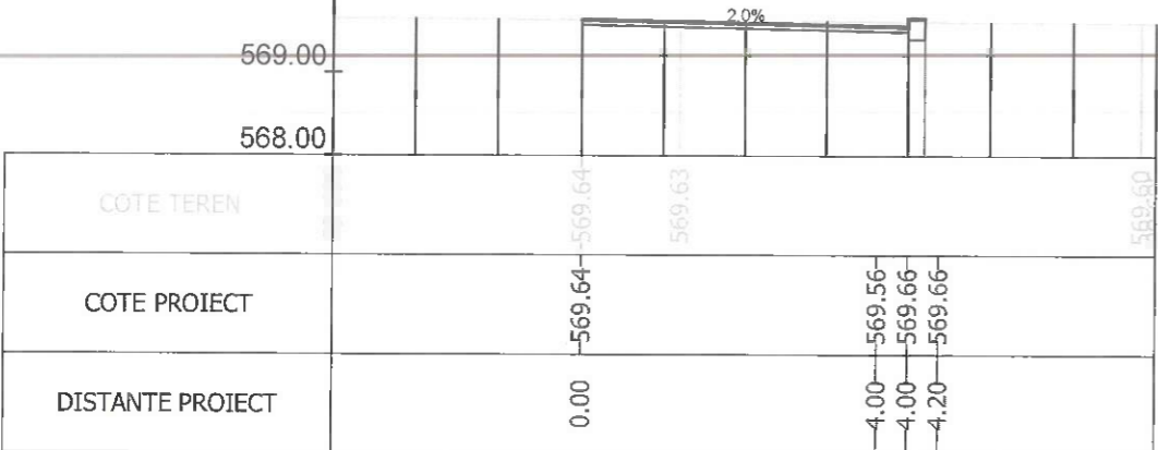
Sectiunea 234 - Km 3+333.018 Ax-Traseul 2
