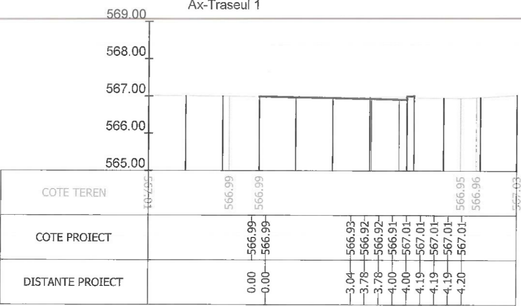
Sectiunea 229 - Km 3+150 Ax-Traseul 1
