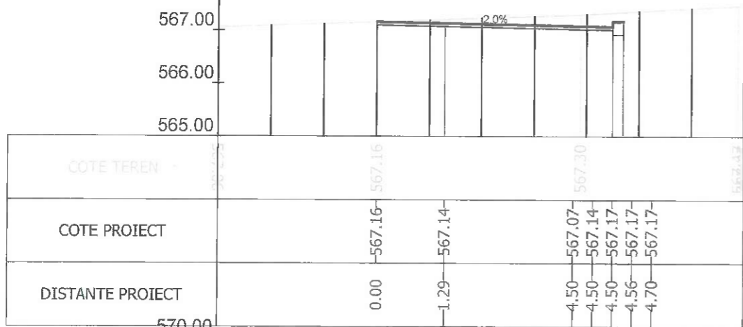
Sectiunea 102 - Km 1+641.875 Ax-Traseul 2
