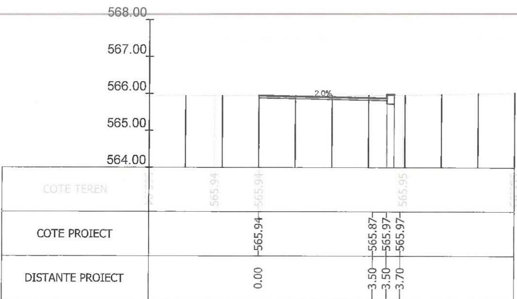
Sectiunea 11 - Km 0+125
