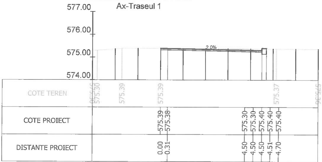
Sectiunea 365 - Km 4+944.447
