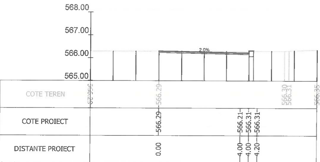
Sectiunea 235 - Km 3+234.653 Ax-Traseul 1
