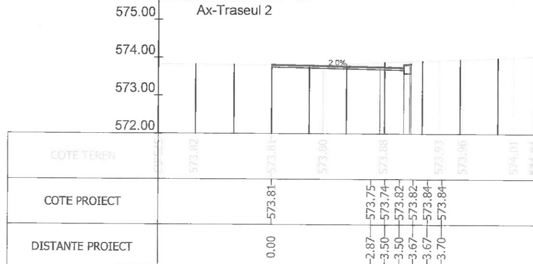
Sectiunea 136 - Km 2+075 Ax-Traseul 2
