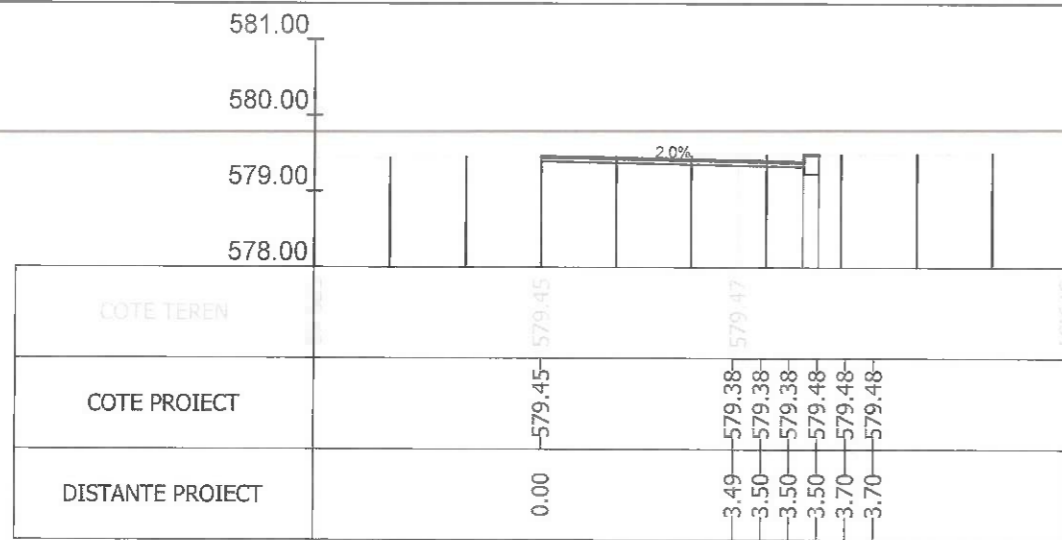
Sectiunea 352 - Km 5+125 Ax-Traseul 2
