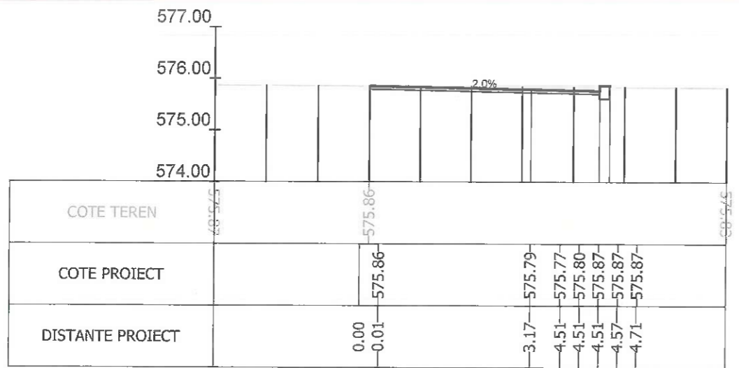
Sectiunea 369 - Km 4+975
