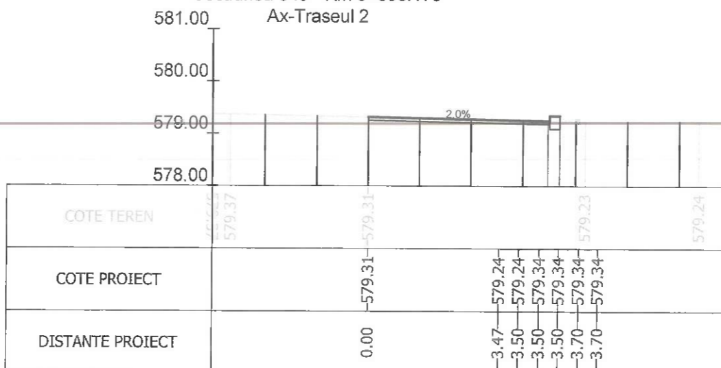
Sectiunea 351 - Km 5+102.576
