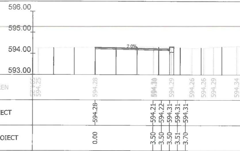
Sectiunea 71 - Km 0+957.321 Ax-Traseul 1
