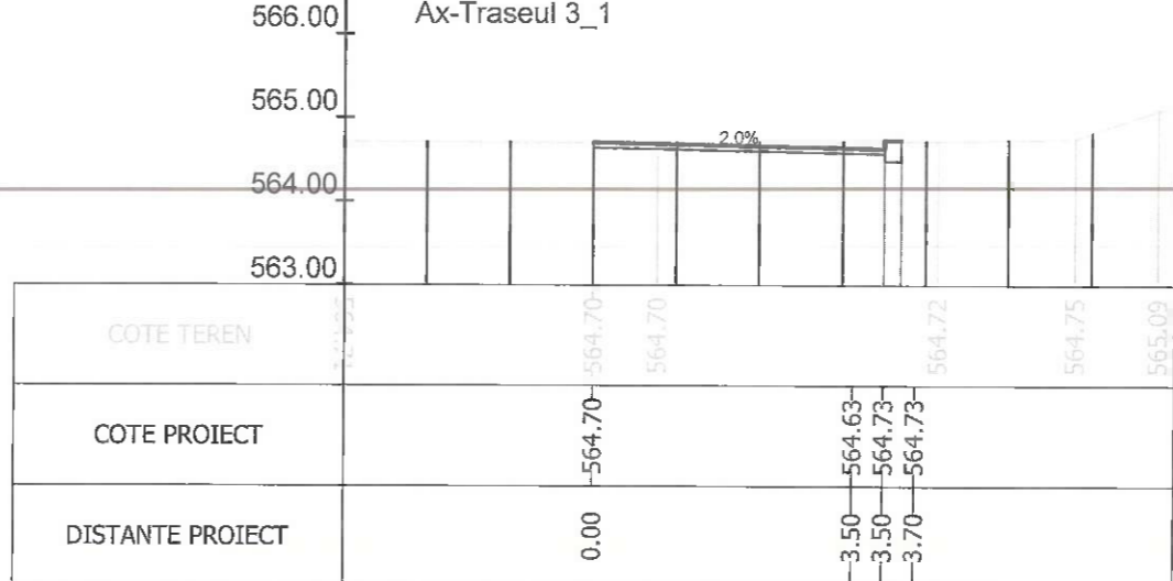
Sectiunea 18 - Km 0+250 Ax-Traseul 3_1
