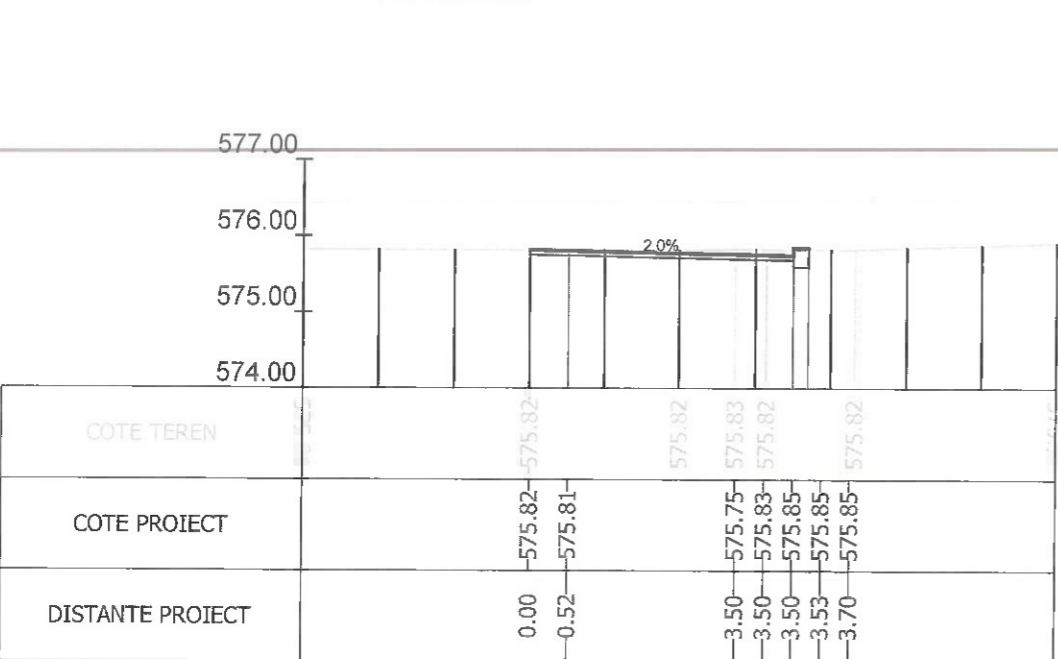
Sectiunea 332 - Km 4+825
