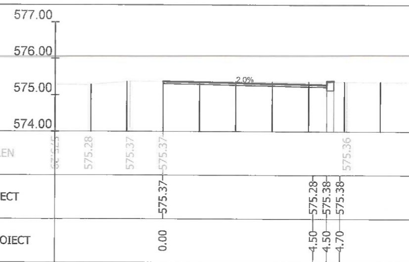
Sectiunea 366 - Km 4+949.248
