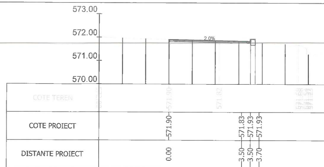
Sectiunea 122 - Km 1+933.733 Ax-Traseul 2
