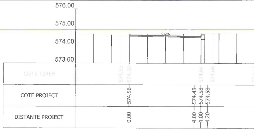
Sectiunea 206 - Km 2+955.677
