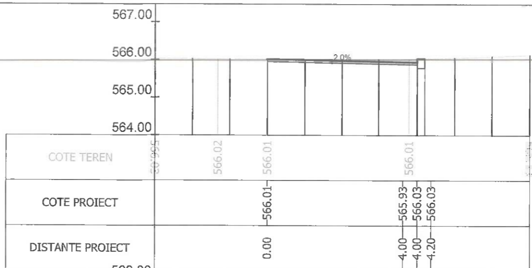
Sectiunea 238 - Km 3+269.946 Ax-Traseul 1
