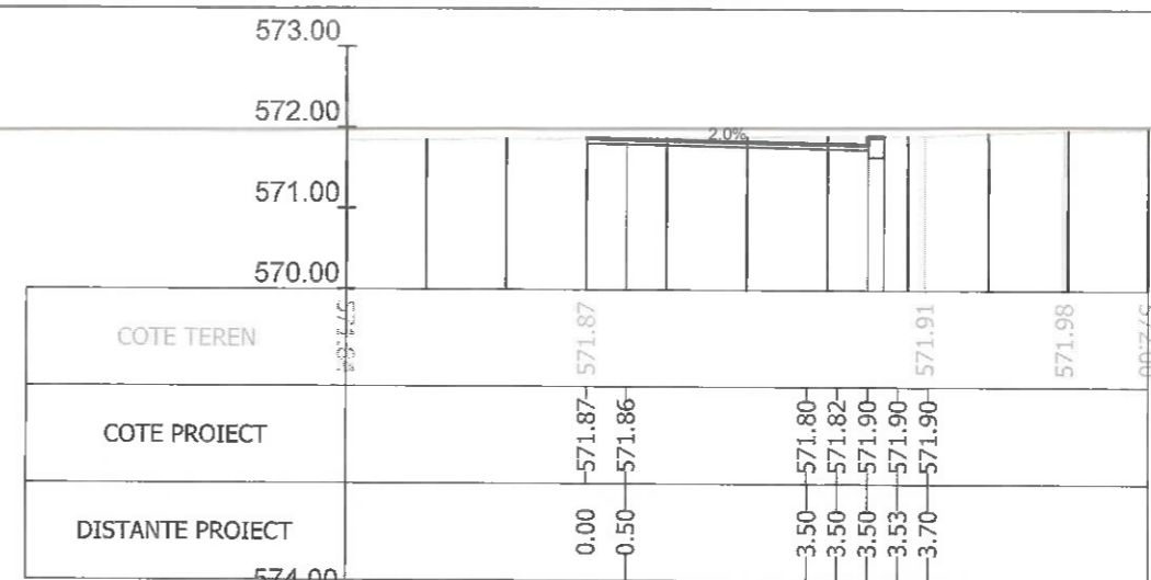
Sectiunea 418 - Km 5+625 Ax-Traseul 1
