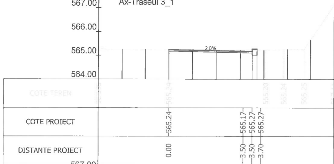
Sectiunea 15 - Km 0+200 Ax-Traseul 3_1
