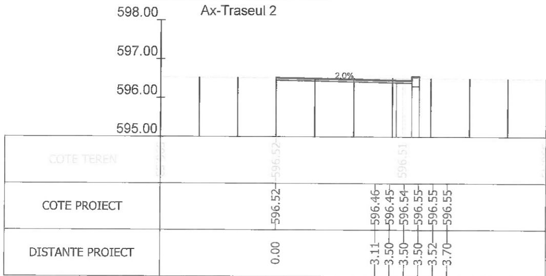
Sectiunea 446 - Km 6+550 Ax-Traseul 2
