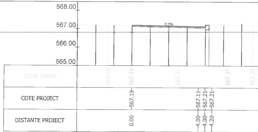
Sectiunea 242 - Km 3+500 Ax-Traseul 2
