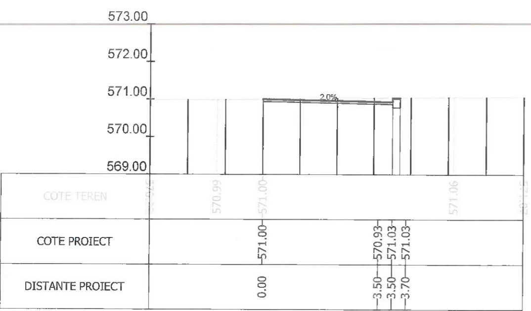
Sectiunea 119 - Km 1+900 Ax-Traseul 2
