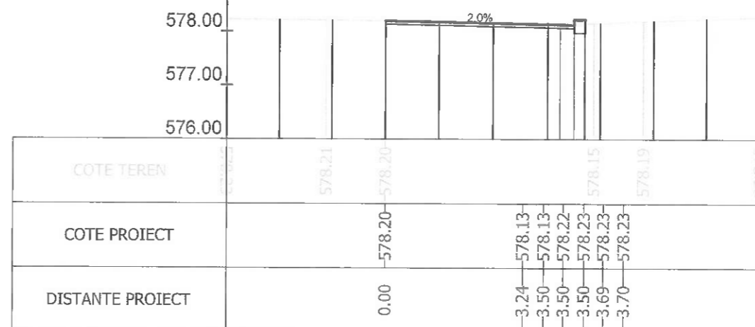
Sectiunea 343 - Km 5+025 Ax-Traceul 2
