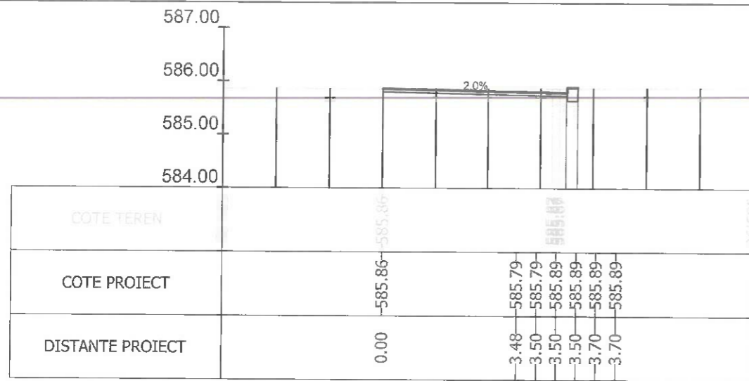
Sectiunea 393 - Km 5+706.293 Ax-Traseul 2
