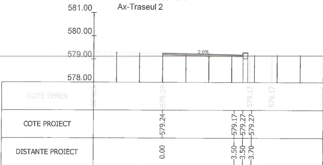
Sectiunea 350 - Km 5+100
