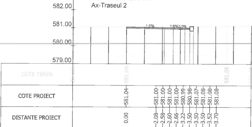
Sectiunea 367 - Km 5+299.634 Ax-Traseul 2
