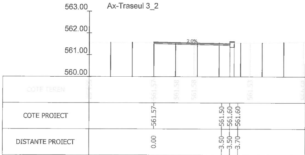
Sectiunea 9 - Km 0+075 Ax-Traseul 3_2
