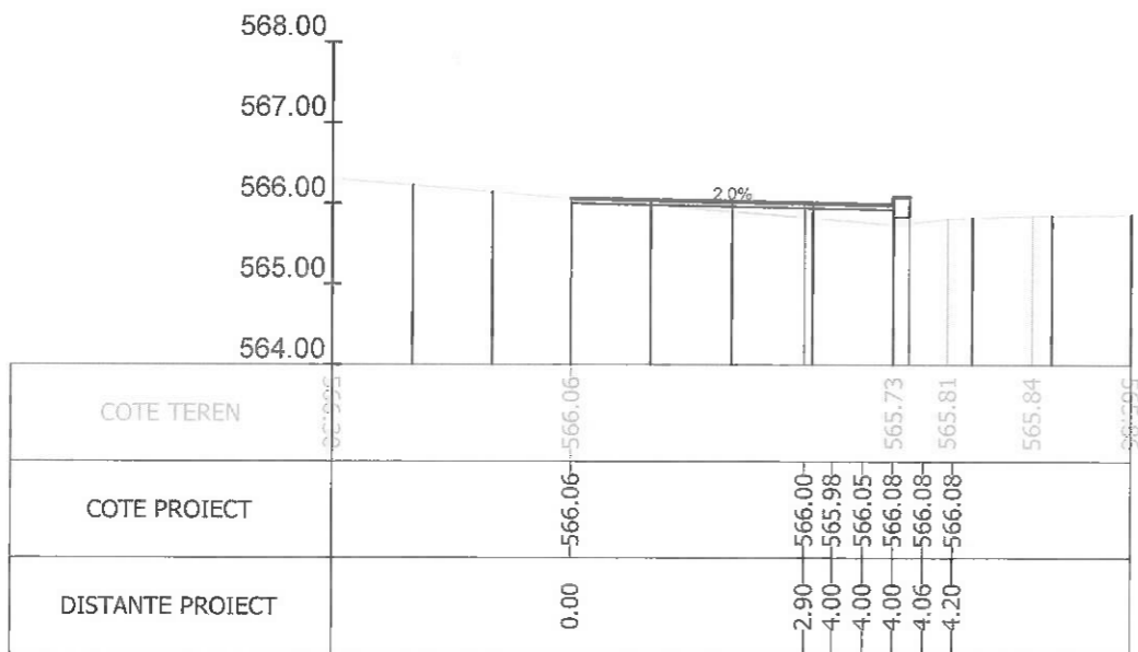
Sectiunea 257 - Km 3+525 Ax-Traseul 1
