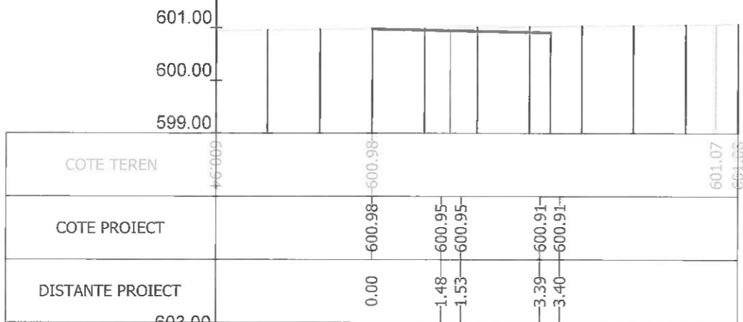
Sectiunea 17 - Km 0+125 Ax-Traseul 1
