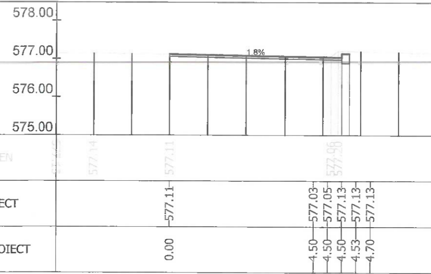
Sectiunea 189 - Km 2+801.230
