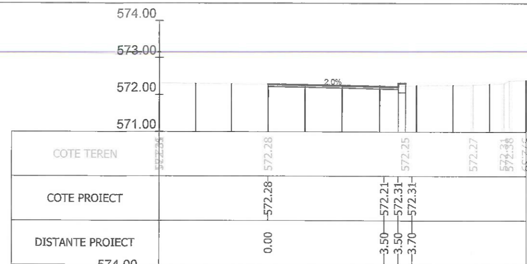
Sectiunea 201 - Km 2+698.439 Ax-Traseul 1
