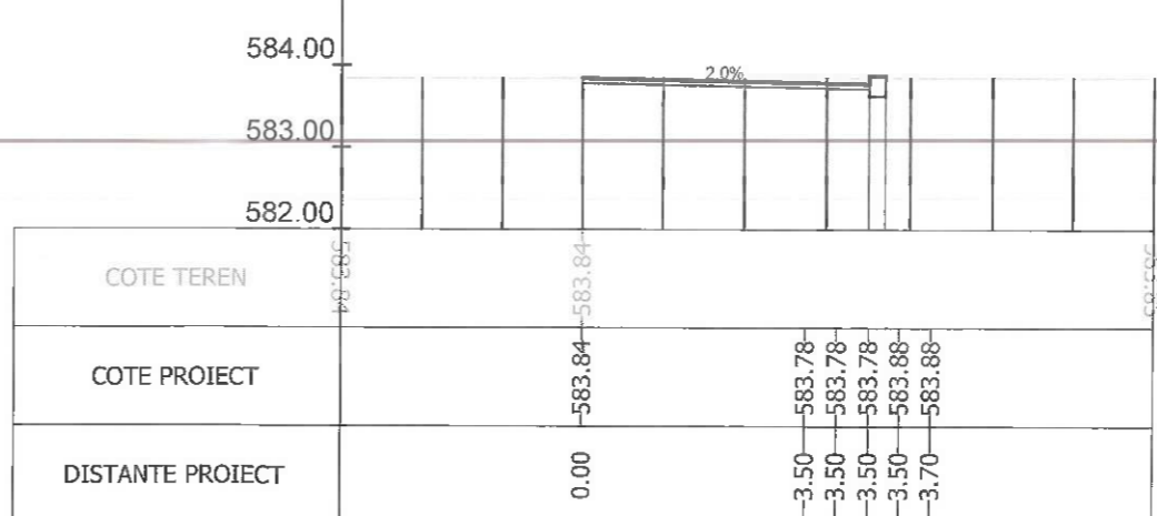
Sectiunea 123 - Km 1+697.595 Ax-Traseul 1
