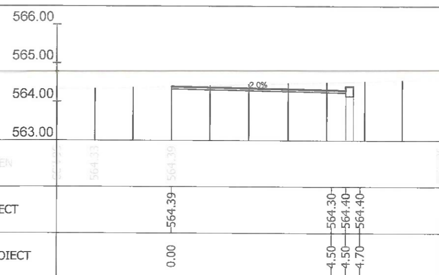
Sectiunea 91 - Km 1+500 Ax-Traceul 2
