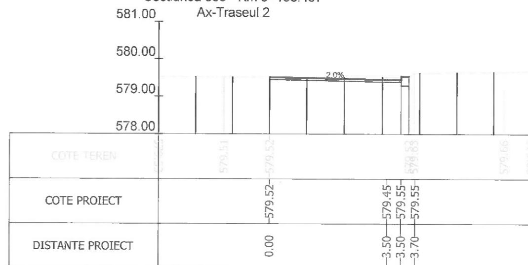
Sectiunea 355 - Km 5+143.984 Ax-Traseul 2
