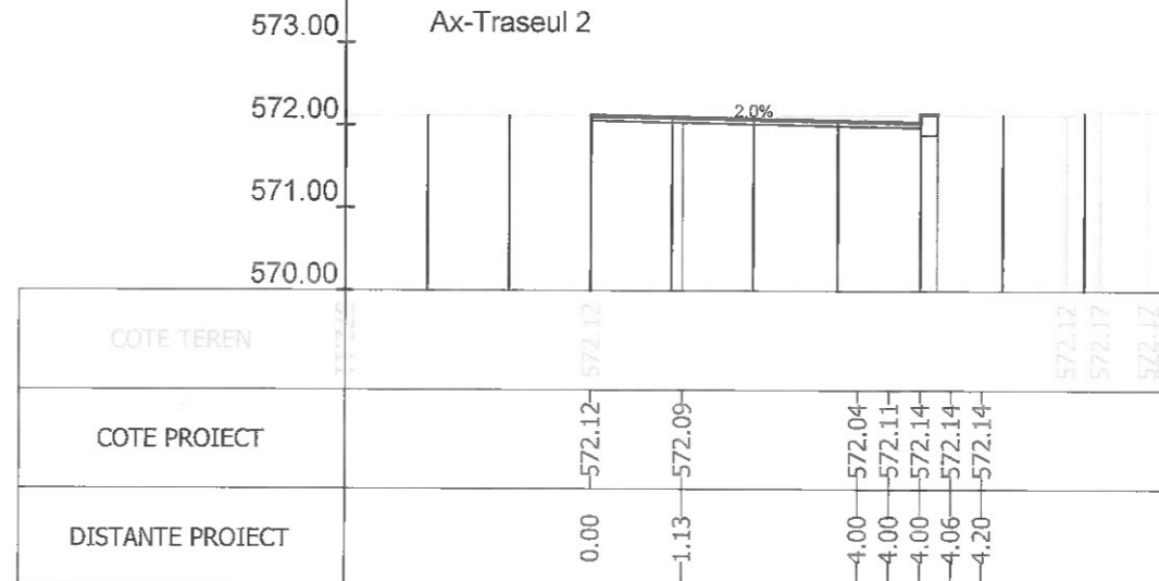
Sectiunea 311 - Km 4+575
