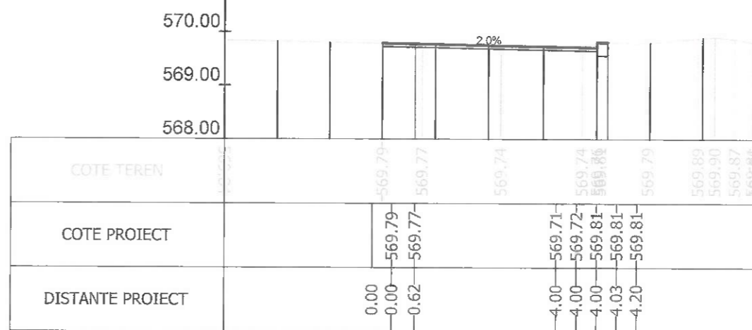
Sectiunea 233 - Km 3+325 Ax-Traseul 2
