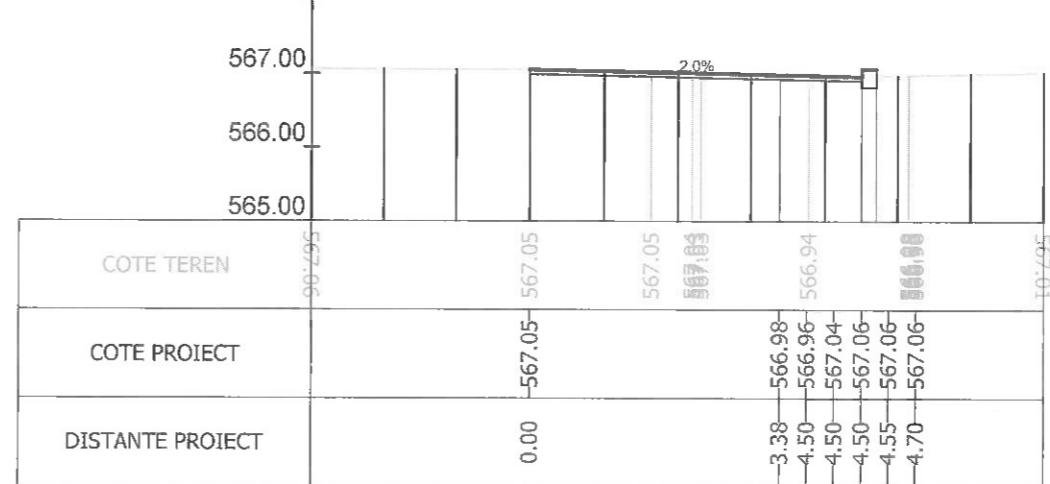
Sectiunea 277 - Km 3+775 Ax-Traseul 1
