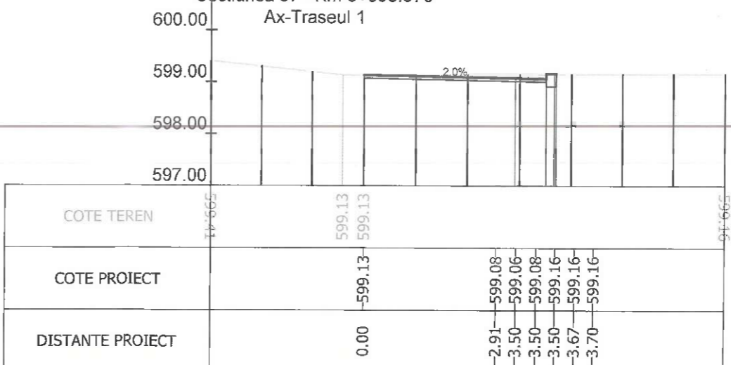
Sectiunea 39 - Km 0+425
