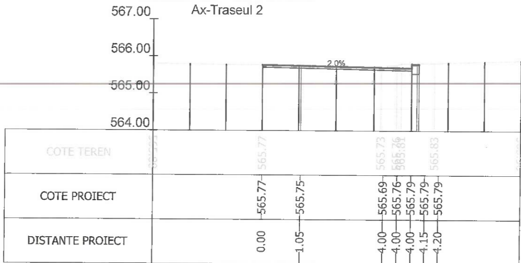
Sectiunea 259 - Km 3+725
