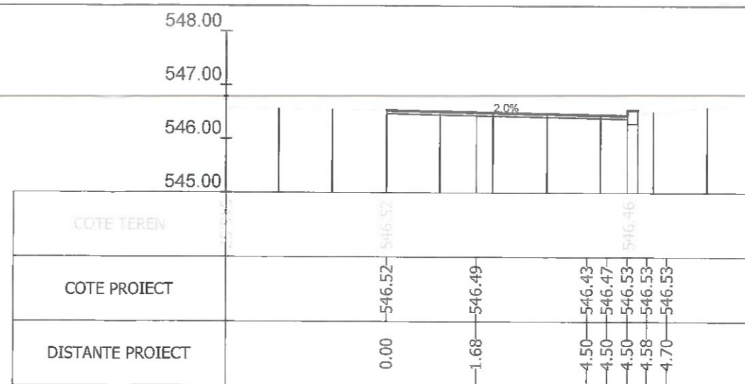
Sectiunea 13 - Km 0+150
