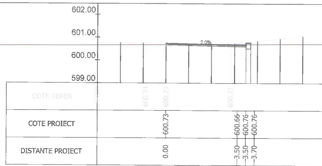
Sectiunea 463 - Km 6+900 Ax-Traseul 2
