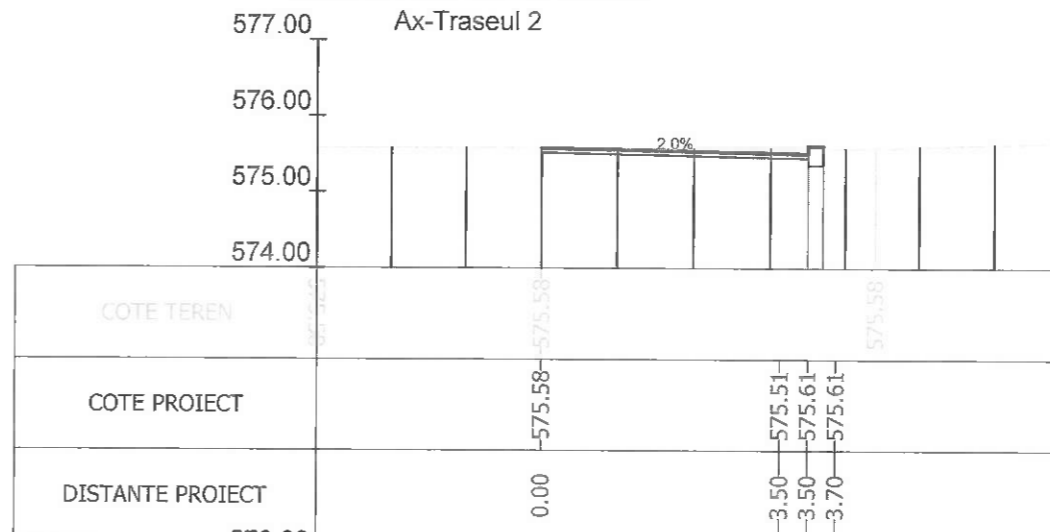
Sectiunea 331 - Km 4+800
