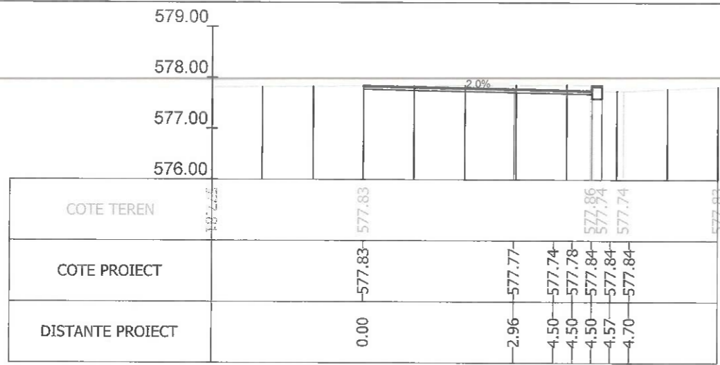
Sectiunea 383 - Km 5+275 Ax-Traseul 1
