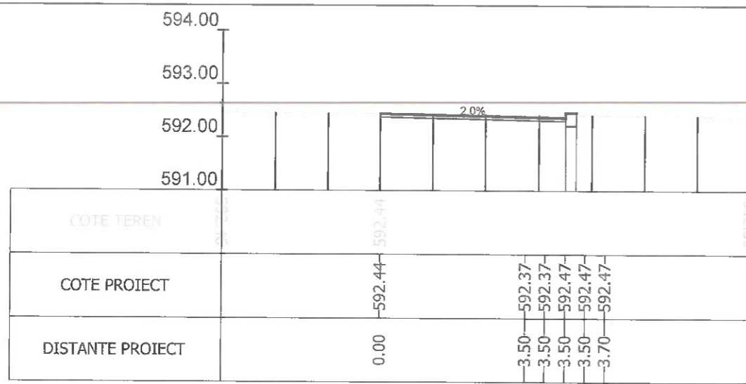
Sectiunea 420 - Km 6+152.423 Ax-Traceul 2
