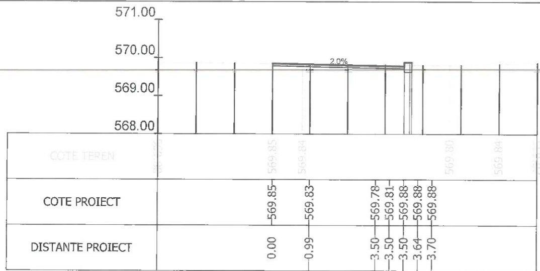
Sectiunea 115 - Km 1+825 Ax-Traseul 2
