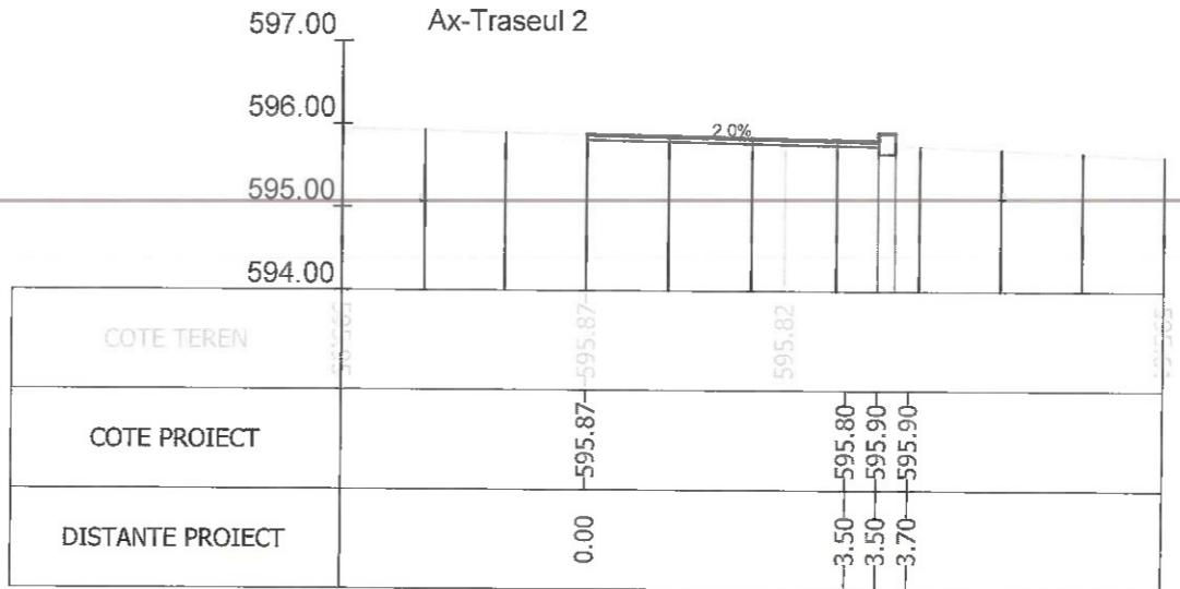
Sectiunea 437 - Km 6+437.558 Ax-Traseul 2
