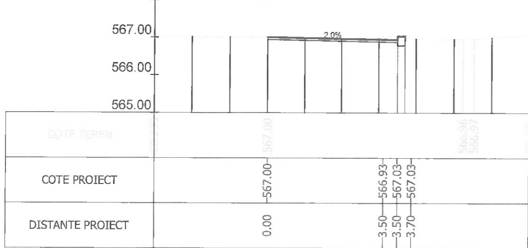
Sectiunea 49 - Km 0+625 Ax-Traseul 3_2
