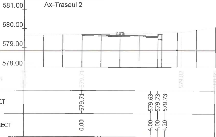
Sectiunea 173 - Km 2+575 Ax-Traseul 2
