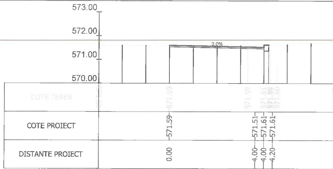
Sectiunea 308 - Km 4+542.260
