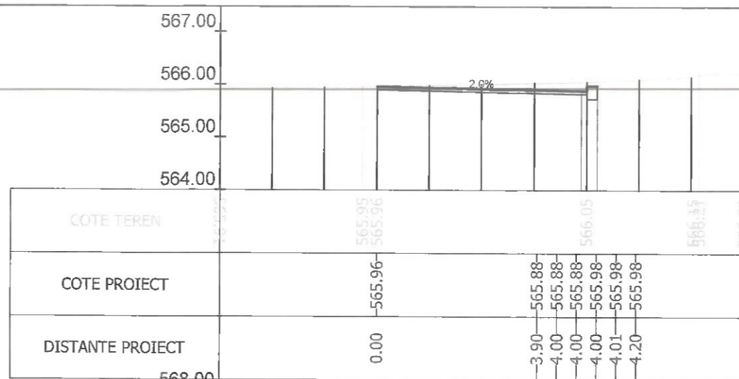
Sectiunea 261 - Km 3+775 Ax-Traseul 2
