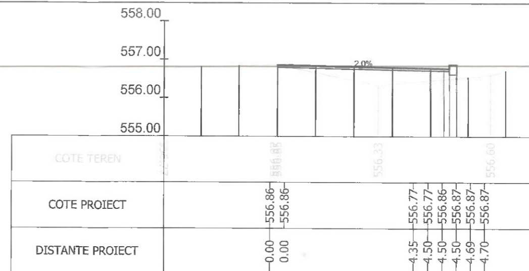
Sectiunea 61 - Km 1+025 Ax-Traseul 2
