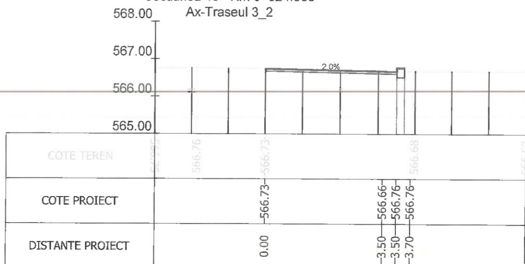
Sectiunea 42 - Km 0+550
