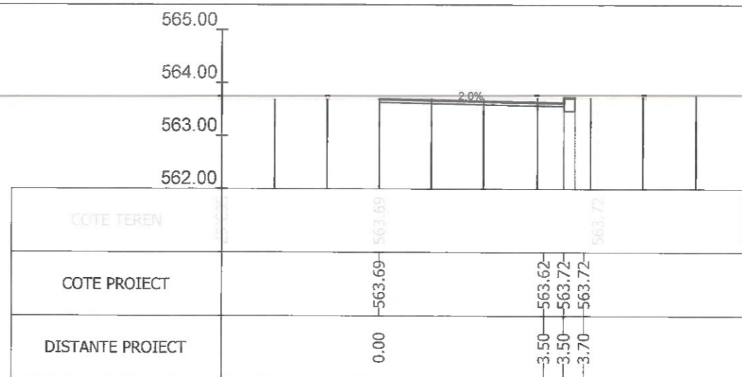
Sectiunea 26 - Km 0+350 Ax-Traseul 3_1
