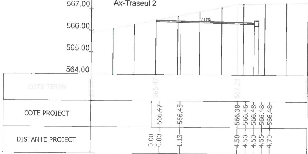
Sectiunea 98 - Km 1+575 Ax-Traseul 2
