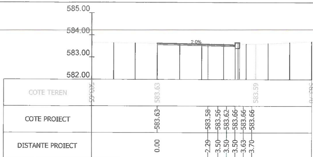
Sectiunea 125 - Km 1+725 Ax-Traseul 1
