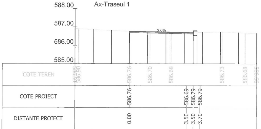
Sectiunea 102 - Km 1+400 Ax-Traseul 1
