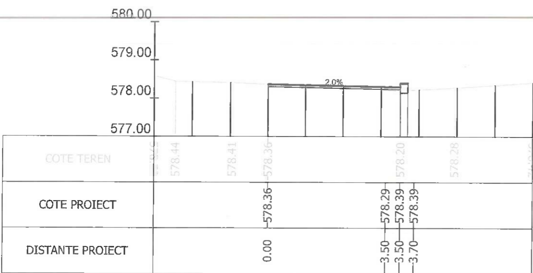
Sectiunea 344 - Km 5+038.588 Ax-Traceul 2
