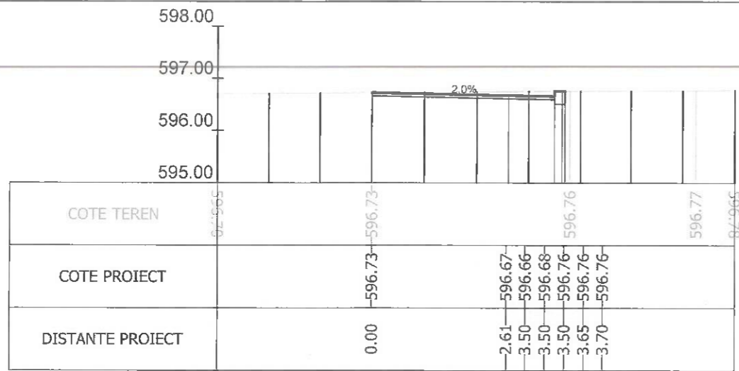
Sectiunea 52 - Km 0+650 Ax-Traseul 1
