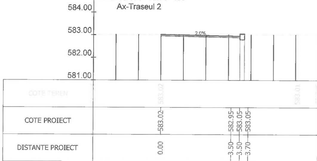
Sectiunea 377 - Km 5+446.626 Ax-Traseul 2
