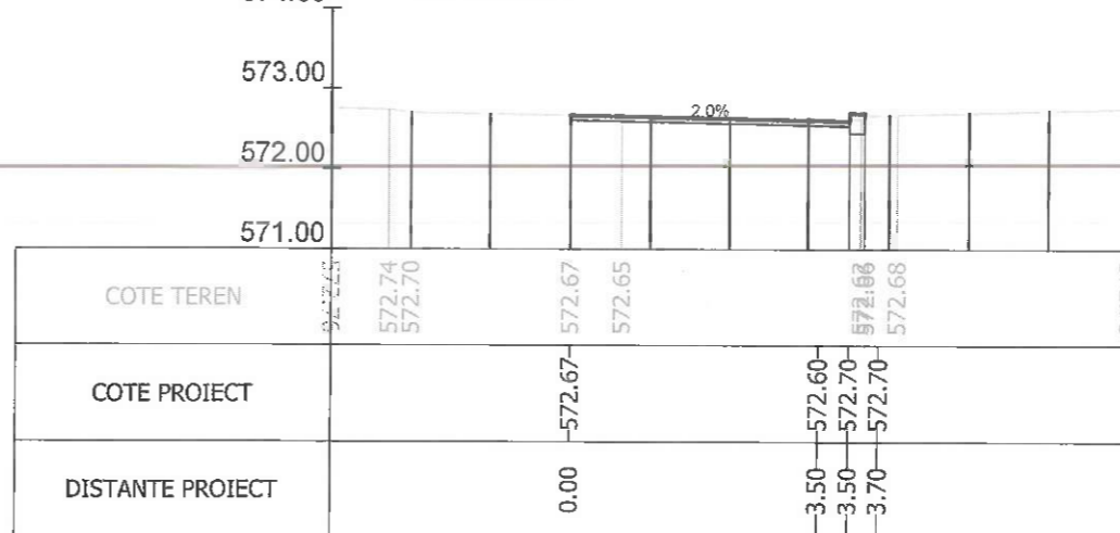
Sectiunea 199 - Km 2+669.020 Ax-Traseul 1
