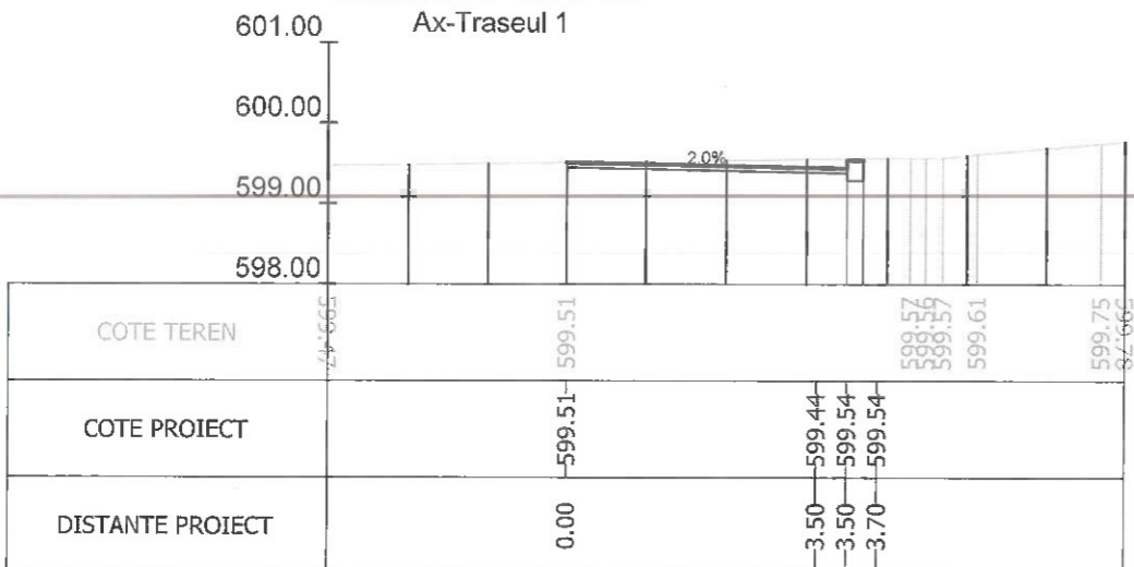
Sectiunea 38 - Km 0+400 Ax-Traseul 1
