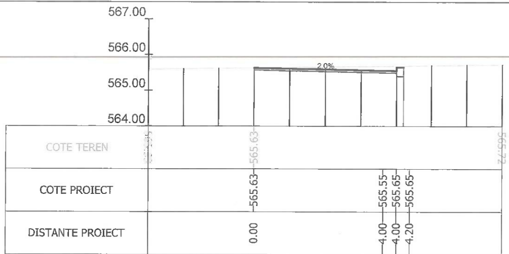
Sectiunea 249 - Km 3+421.270 Ax-Traseul 1
