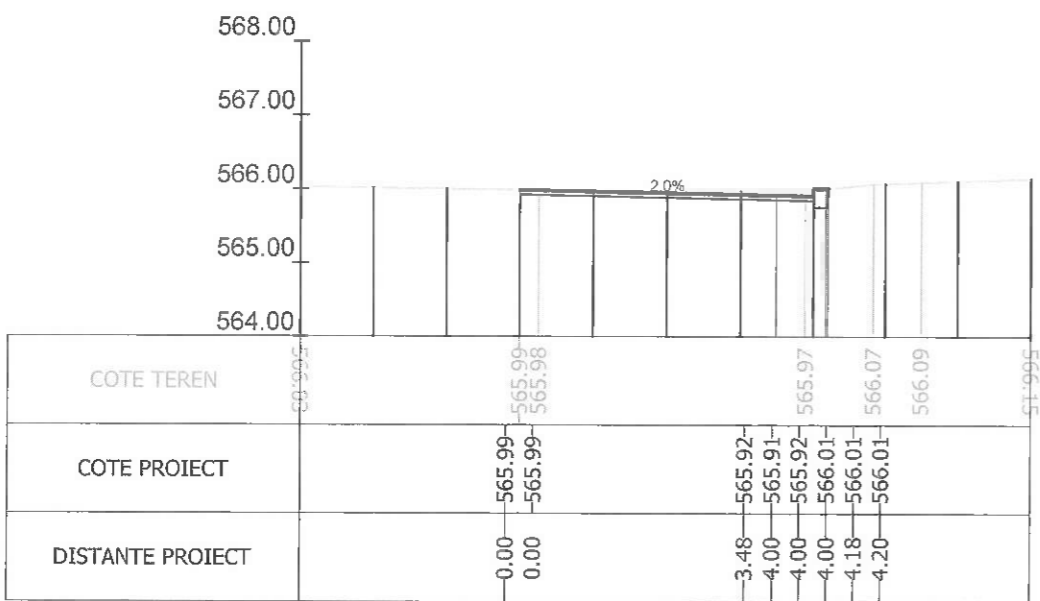
Sectiunea 239 - Km 3+275 Ax-Traseul 1
