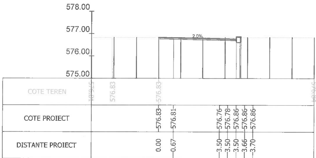
Sectiunea 175 - Km 2+350 Ax-Traseul 1
