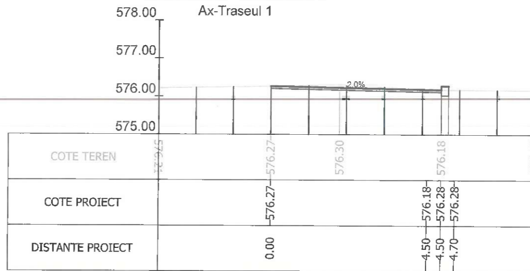
Sectiunea 370 - Km 4+993.682
