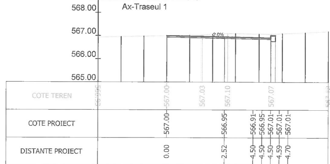
Sectiunea 319 - Km 4+425 Ax-Traseul 1
