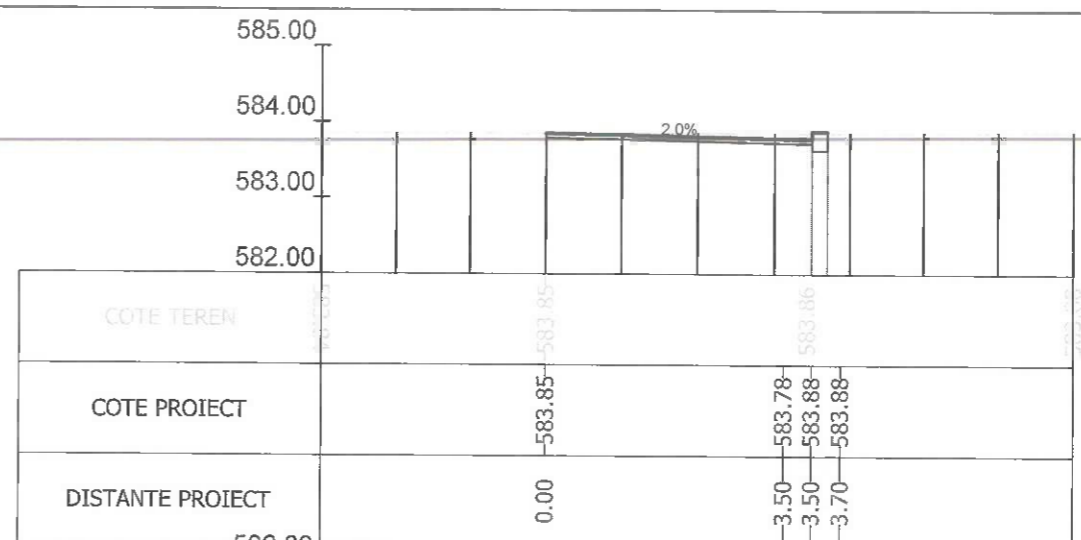
Sectiunea 382 - Km 5+543.857 Ax-Traseul 2
