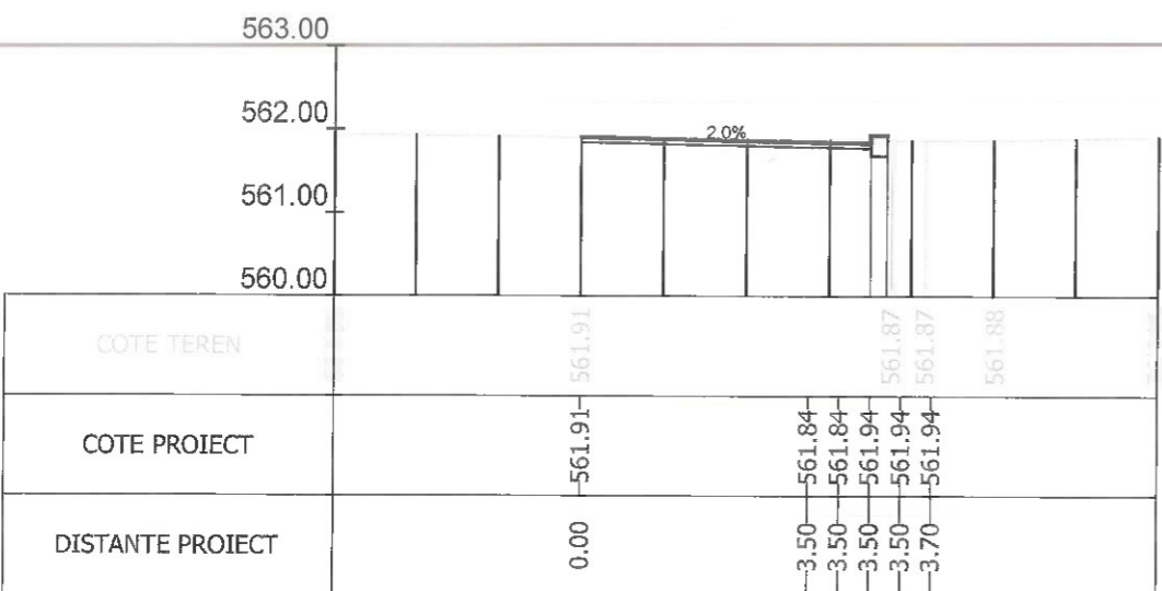
Sectiunea 11 - Km 0+097.873 Ax-Traseul 3_2
