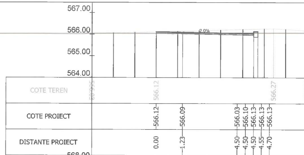
Sectiunea 287 - Km 3+975 Ax-Traseul 1
