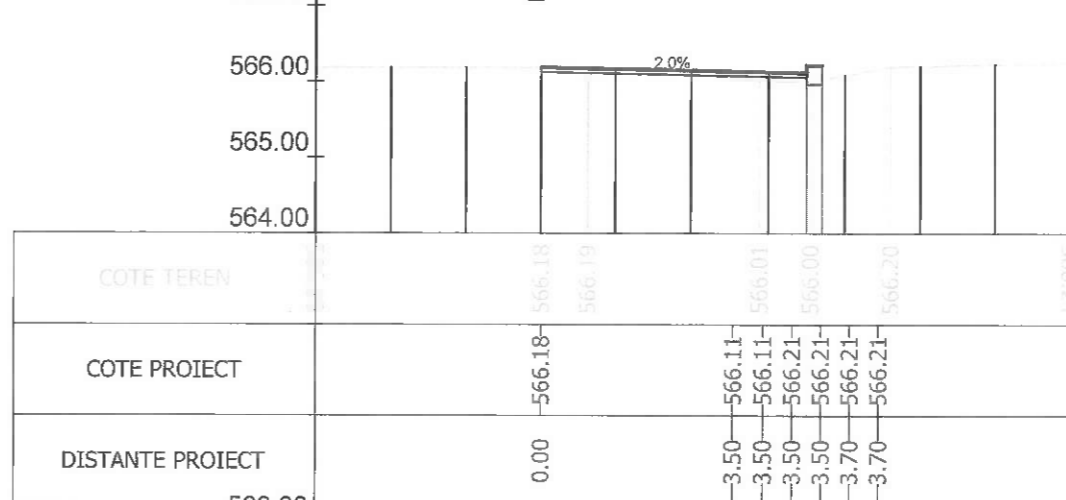
Sectiunea 10 - Km 0+110.489
