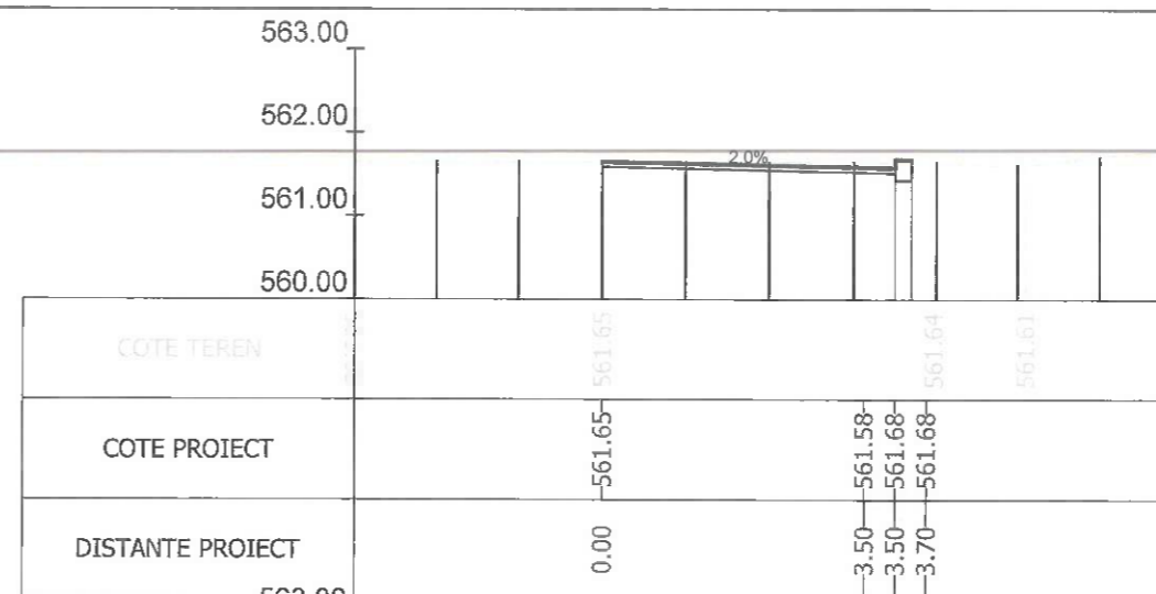
Sectiunea 44 - Km 0+550 Ax-Traseul 3_1
