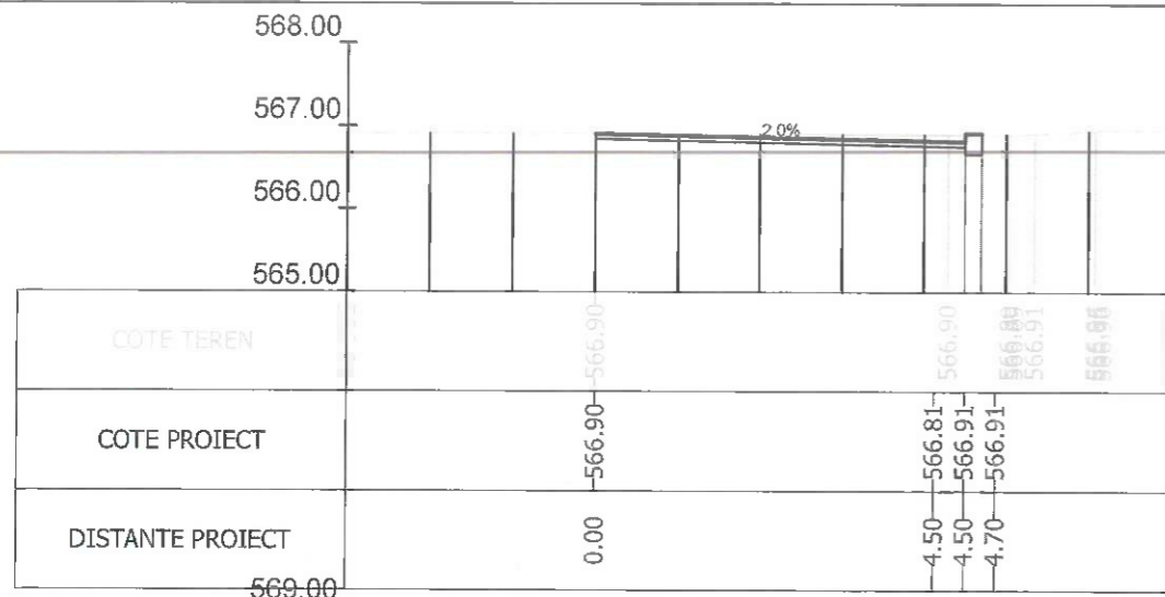
Sectiunea 102 - Km 1+641.875 Ax-Traseul 2
