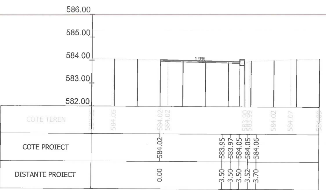
Sectiunea 385 - Km 5+584.258 Ax-Traseul 2
