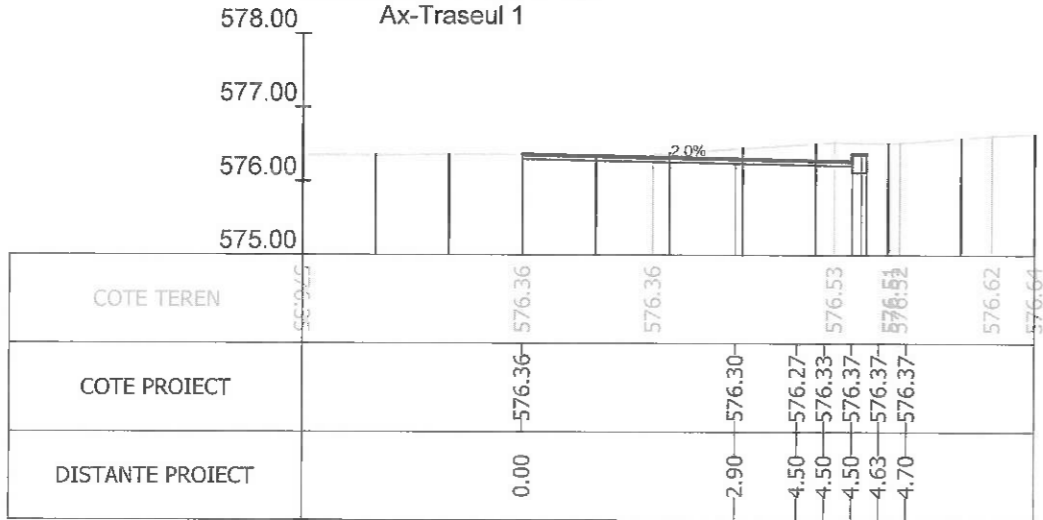
Sectiunea 371 - Km 5+000 Ax-Traseul 1
