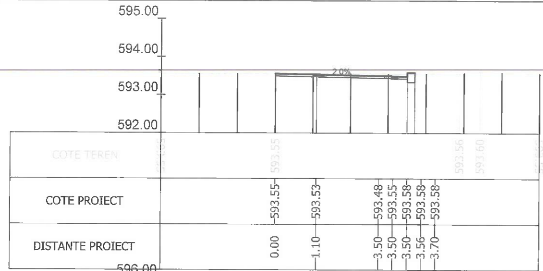
Sectiunea 426 - Km 6+225 Ax-Traseul 2
