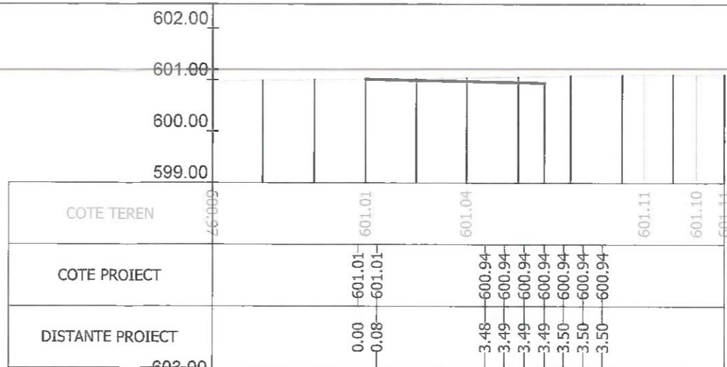
Sectiunea 16 - Km 0+122.288 Ax-Traseul 1
