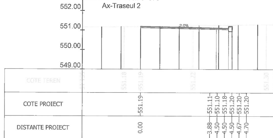
Sectiunea 39 - Km 0+625 Ax-Traseul 2
