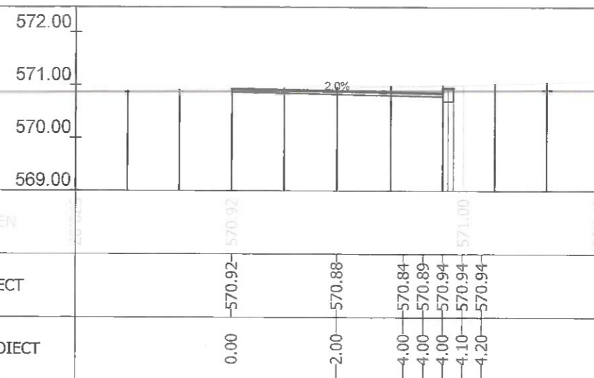
Sectiunea 303 - Km 4+450 Ax-Traseul 2
