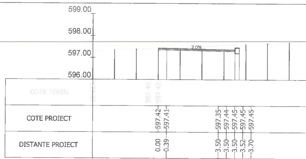
Sectiunea 451 - Km 6+675 Ax-Traseul 2
