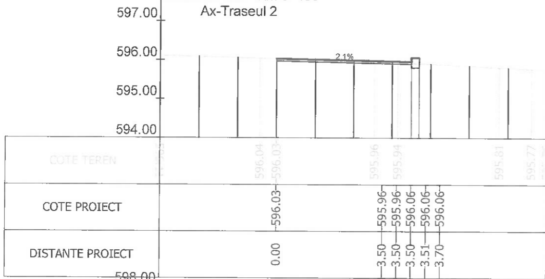
Sectiunea 440 - Km 6+477.457 Ax-Traseul 2
