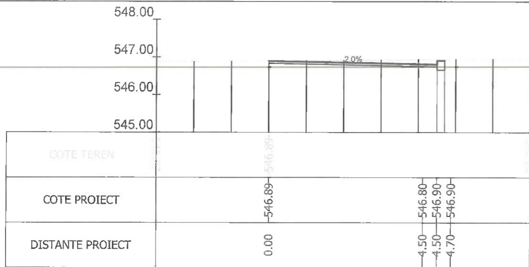
Sectiunea 18 - Km 0+200 Ax-Traseul 2
