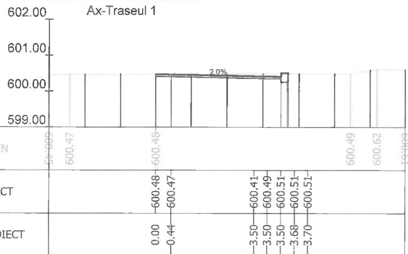
Sectiunea 36 - Km 0+375 Ax-Traseul 1
