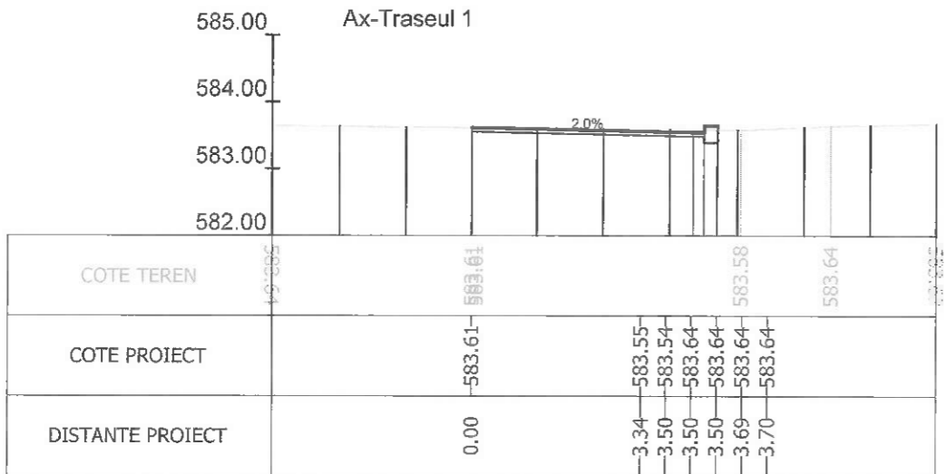
Sectiunea 126 - Km 1+727.772 Ax-Traseul 1
