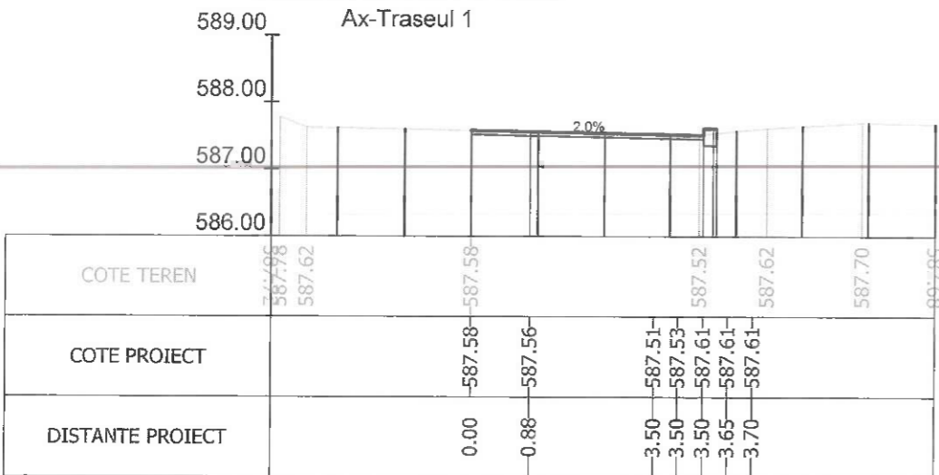
Sectiunea 98 - Km 1+350 Ax-Traseul 1
