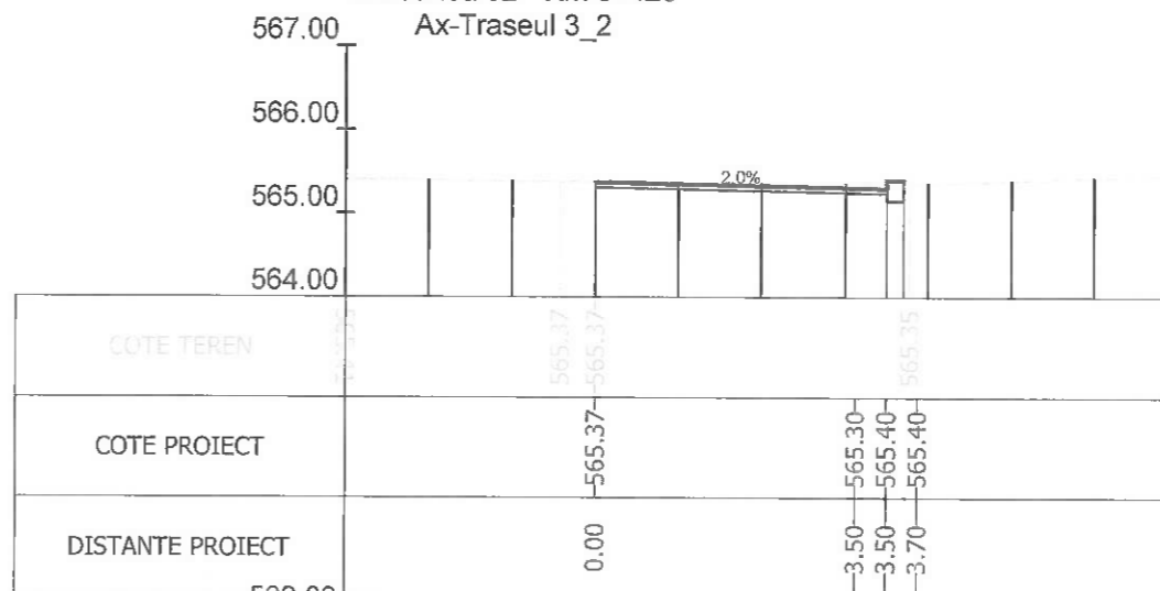
Sectiunea 34 - Km 0+450 Ax-Traseul 3_2
