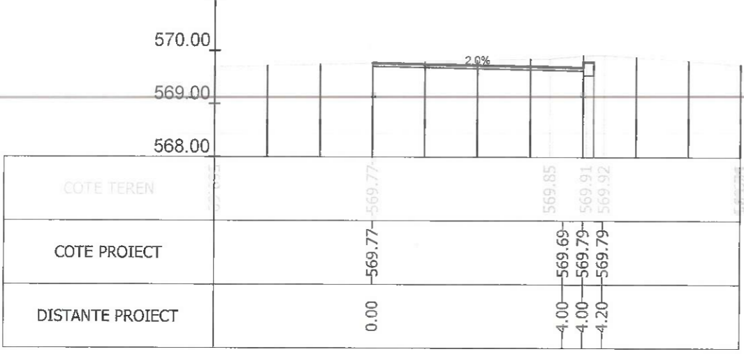
Sectiunea 294 - Km 4+313.052 Ax-Traseul 2
