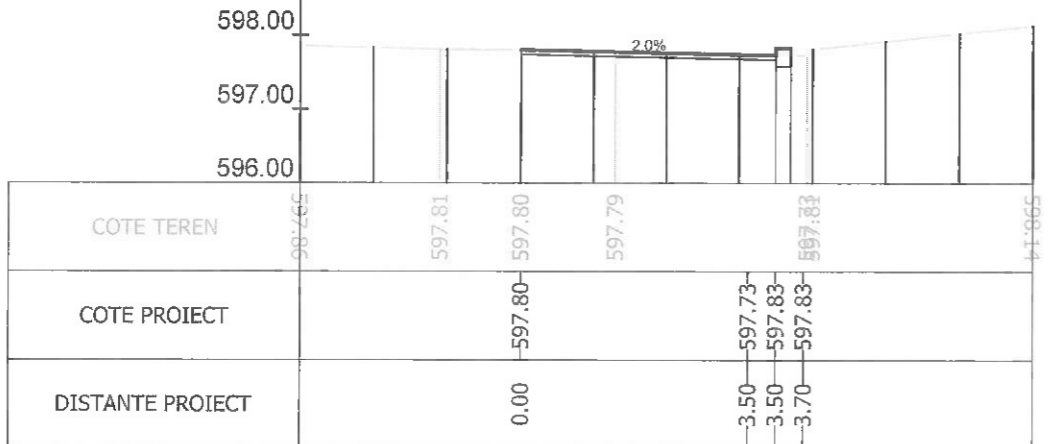
Sectiunea 42 - Km 0+477.766 Ax-Traseul 1
