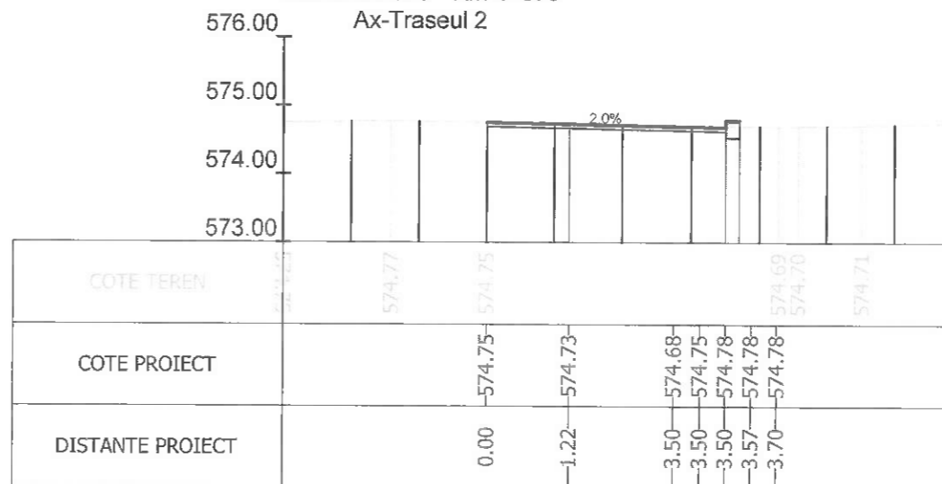
Sectiunea 325 - Km 4+725
