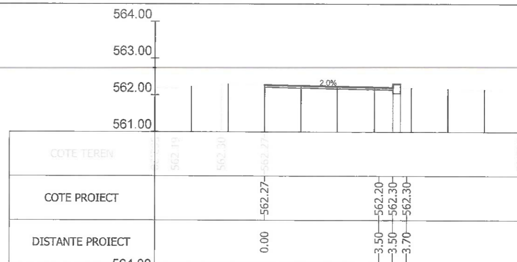
Sectiunea 38 - Km 0+500 Ax-Traseul 3_1
