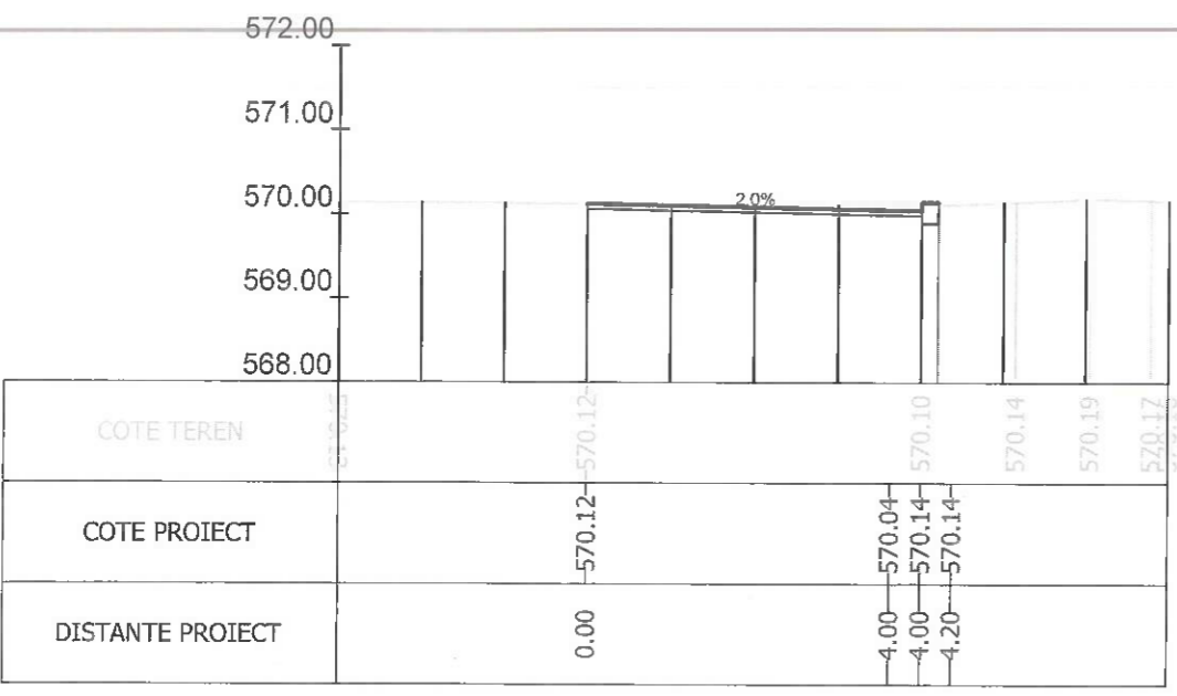
Sectiunea 228 - Km 3+307.281 Ax-Traseul 2
