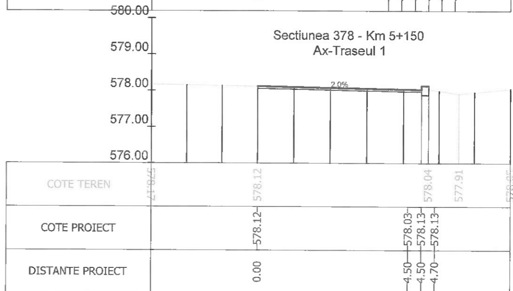
Sectiunea 380 - Km 5+200 Ax-Traseul 1
