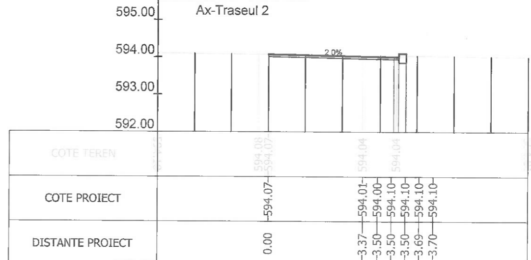
Sectiunea 429 - Km 6+275 Ax-Traseul 2
