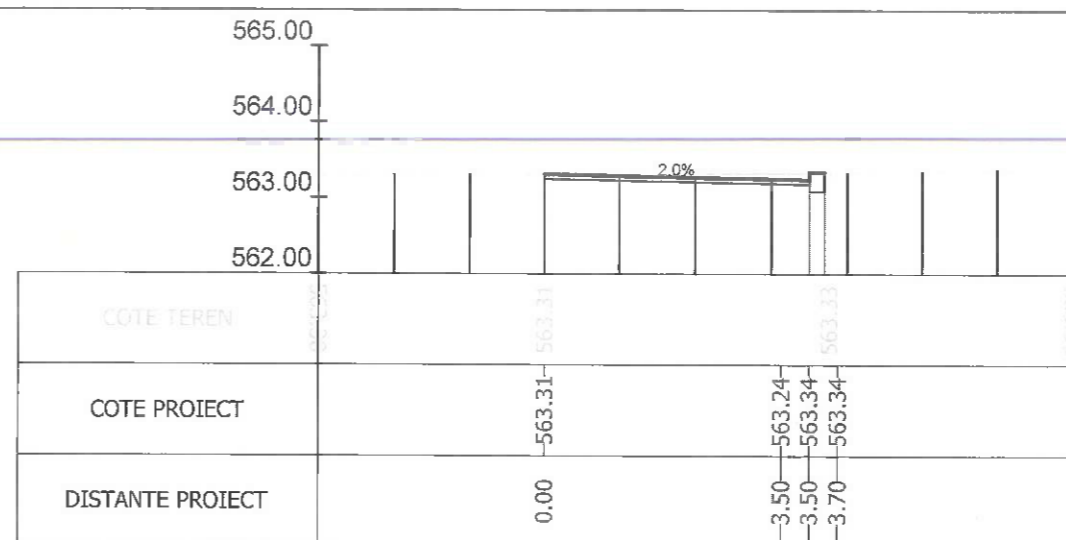
Sectiunea 20 - Km 0+250 Ax-Traseul 3_2
