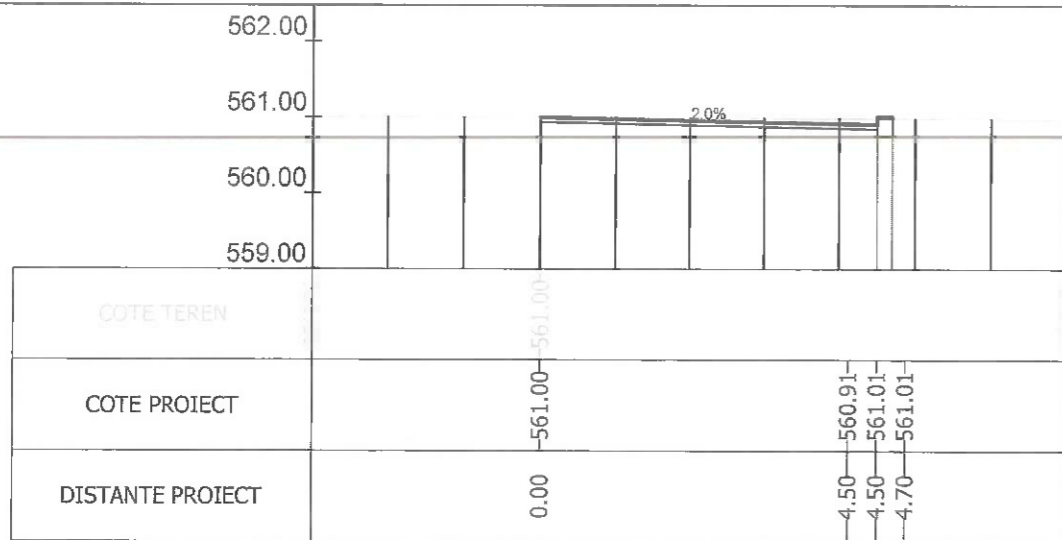
Sectiunea 79 - Km 1+300 Ax-Traseul 2
