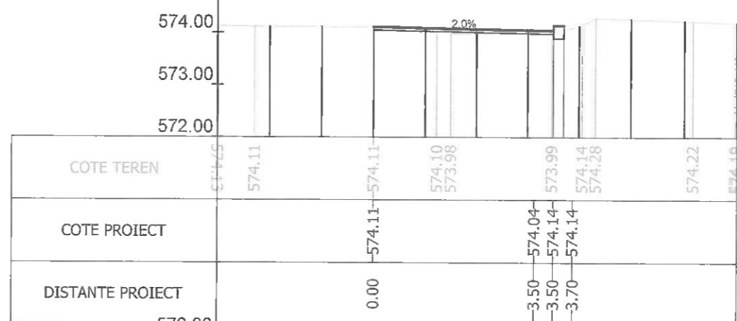
Sectiunea 402 - Km 5+484.815 Ax-Traseul 1
