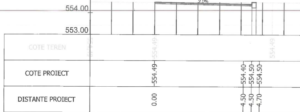
Sectiunea 53 - Km 0+900
