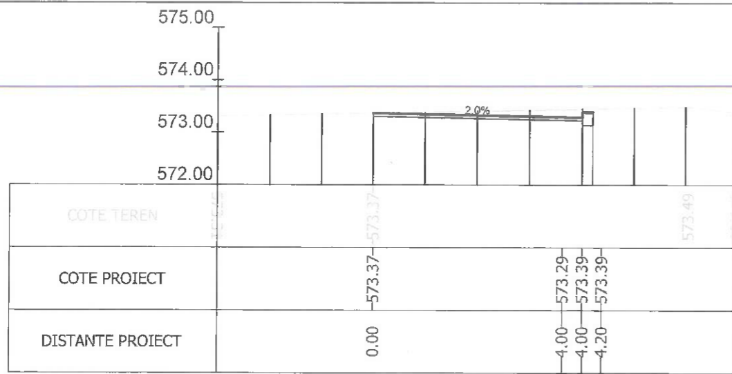
Sectiunea 212 - Km 3+050 Ax-Traseul 2
