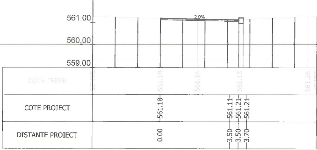
Sectiunea 5 - Km 0+025 Ax-Traseul 3_2
