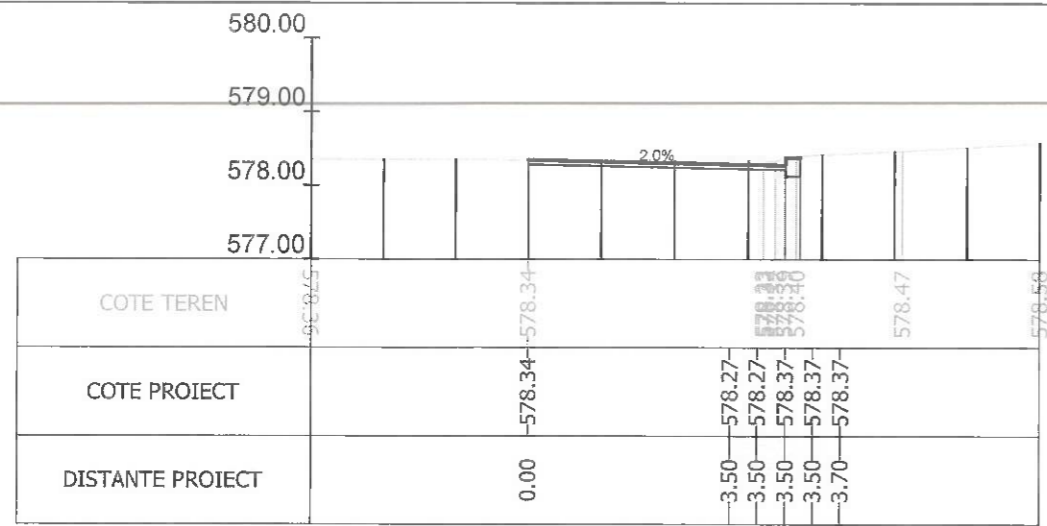
Sectiunea 167 - Km 2+213.762 Ax-Traseul 1
