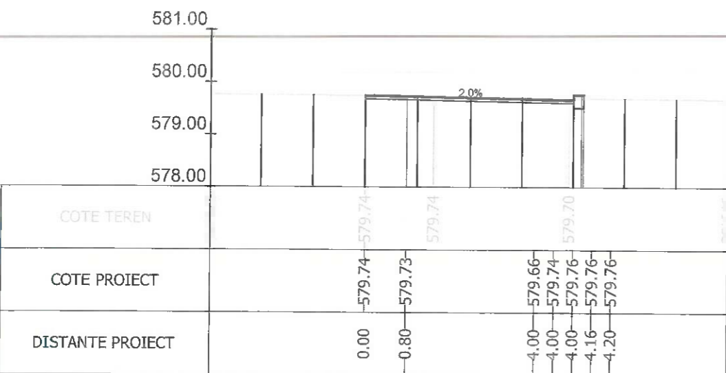
Sectiunea 168 - Km 2+475 Ax-Traseul 2
