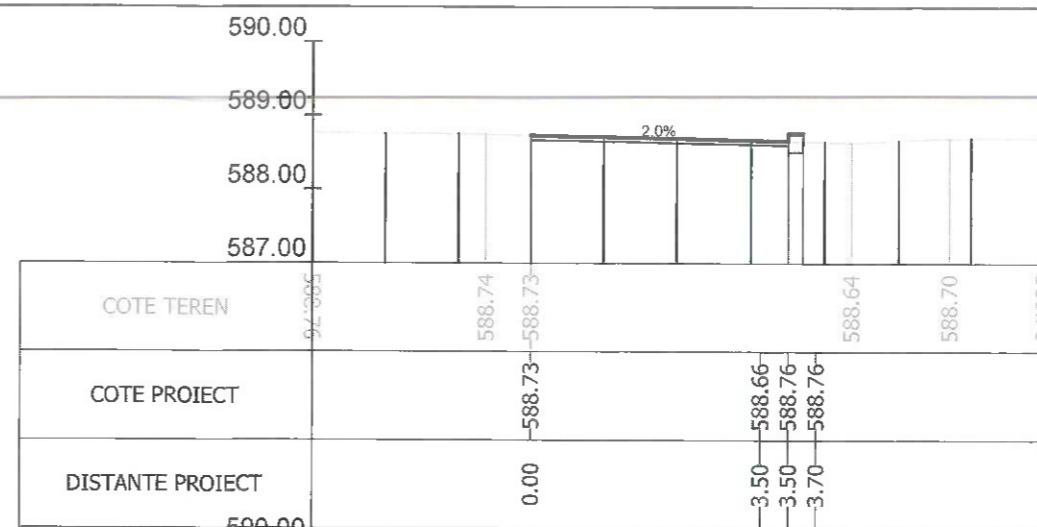
Sectiunea 95 - Km 1+300 Ax-Traseul 1
