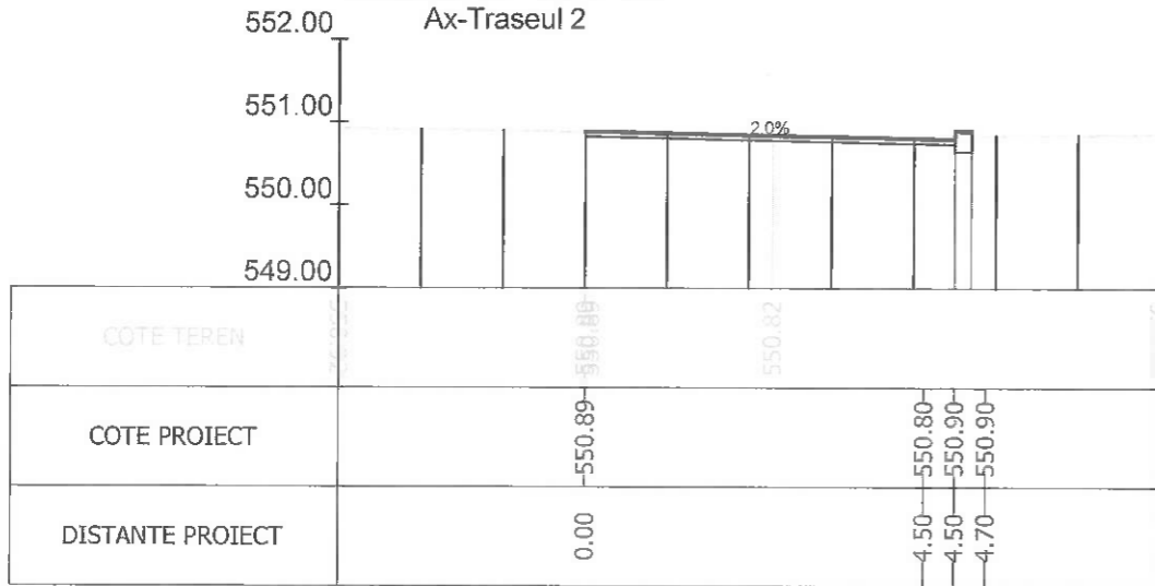
Sectiunea 38 - Km 0+600 Ax-Traseul 2
