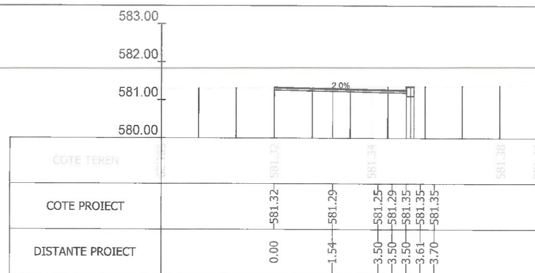
Sectiunea 370 - Km 5+325
