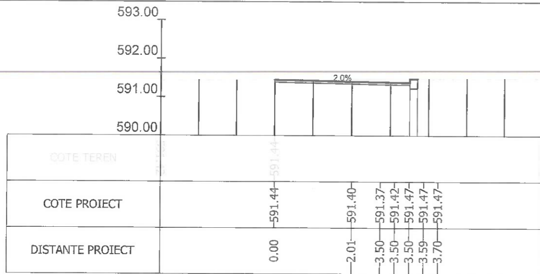
Sectiunea 414 - Km 6+075 Ax-Traseul 2
