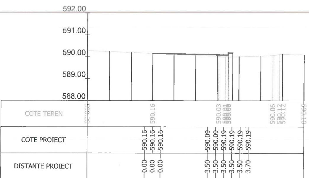
Sectiunea 92 - Km 1+255.707 Ax-Traseul 1
