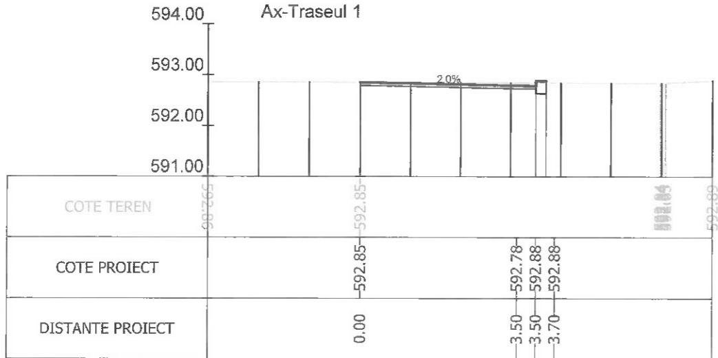
Sectiunea 78 - Km 1+058.629 Ax-Traseul 1
