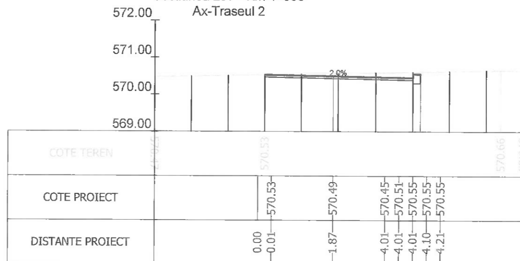
Sectiunea 299 - Km 4+375 Ax-Traseul 2
