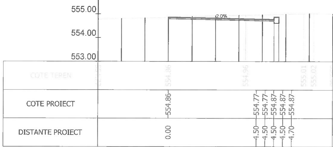
Sectiunea 56 - Km 0+925.617 Ax-Traseul 2
