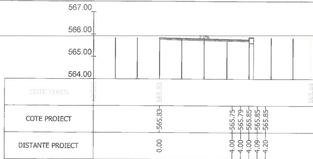
Sectiunea 249 - Km 3+624.840 Ax-Traseul 2
