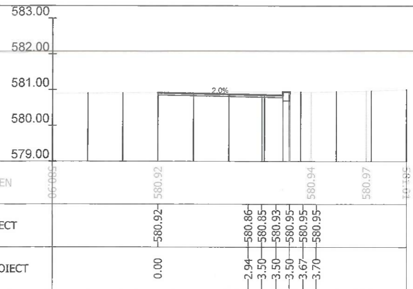
Sectiunea 143 - Km 1+950 Ax-Traseul 1
