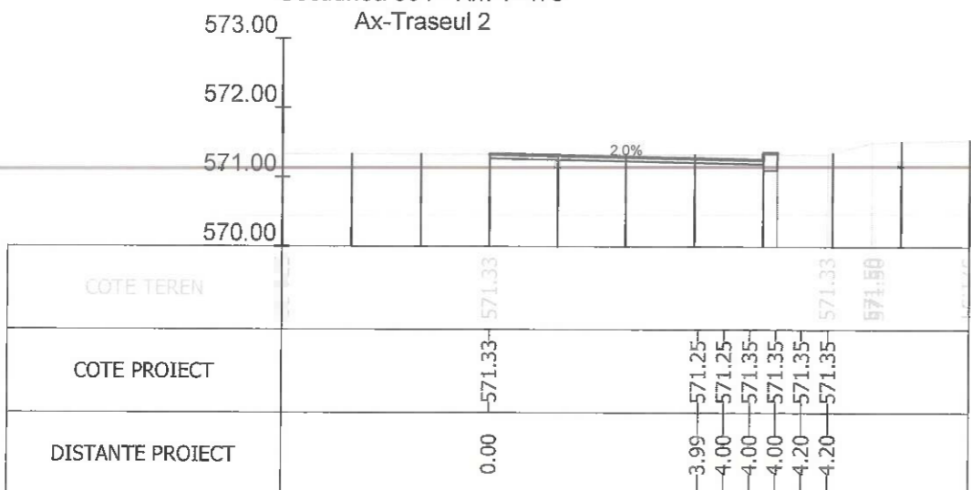
Sectiunea 306 - Km 4+508.474 Ax-Traseul 2
