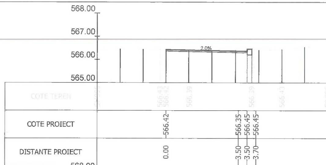
Sectiunea 8 - Km 0+075
