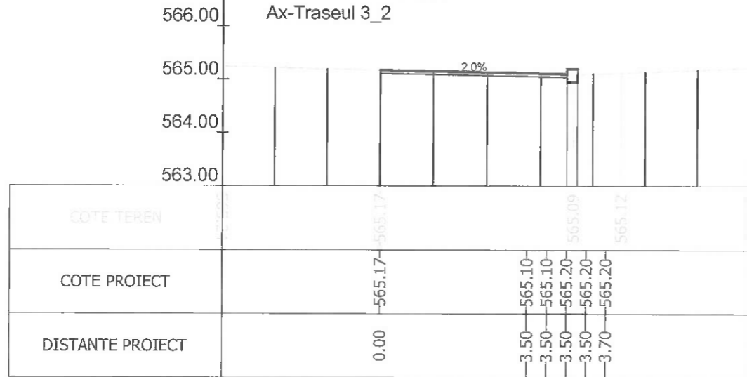
Sectiunea 33 - Km 0+431.692 Ax-Traseul 3_2
