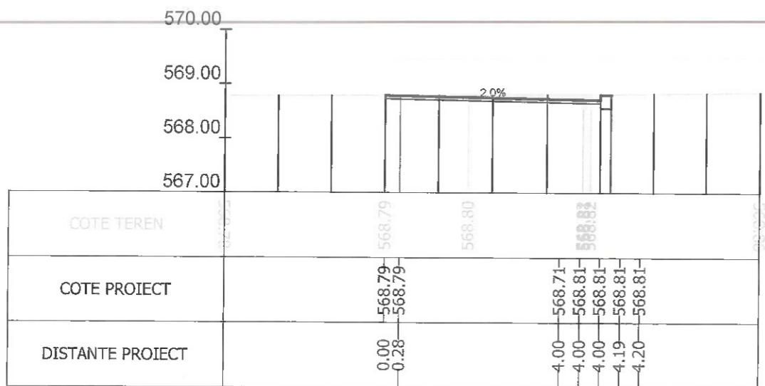
Sectiunea 288 - Km 4+225
