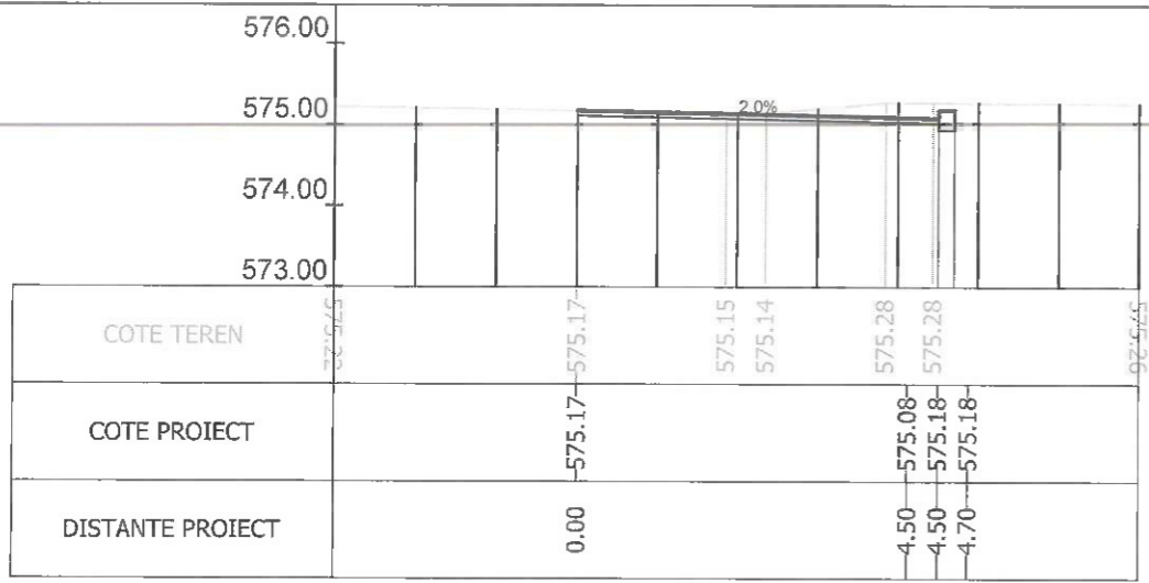
Sectiunea 365 - Km 4+944.447
