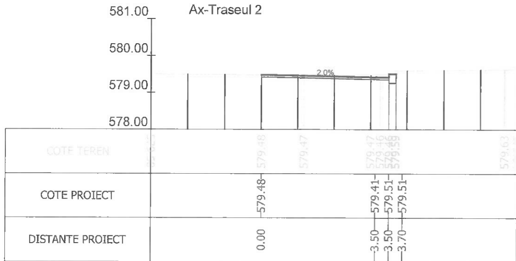
Sectiunea 354 - Km 5+141.220 Ax-Traseul 2
