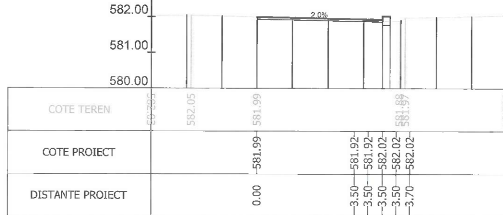
Sectiunea 133 - Km 1+845.988 Ax-Traseul 1
