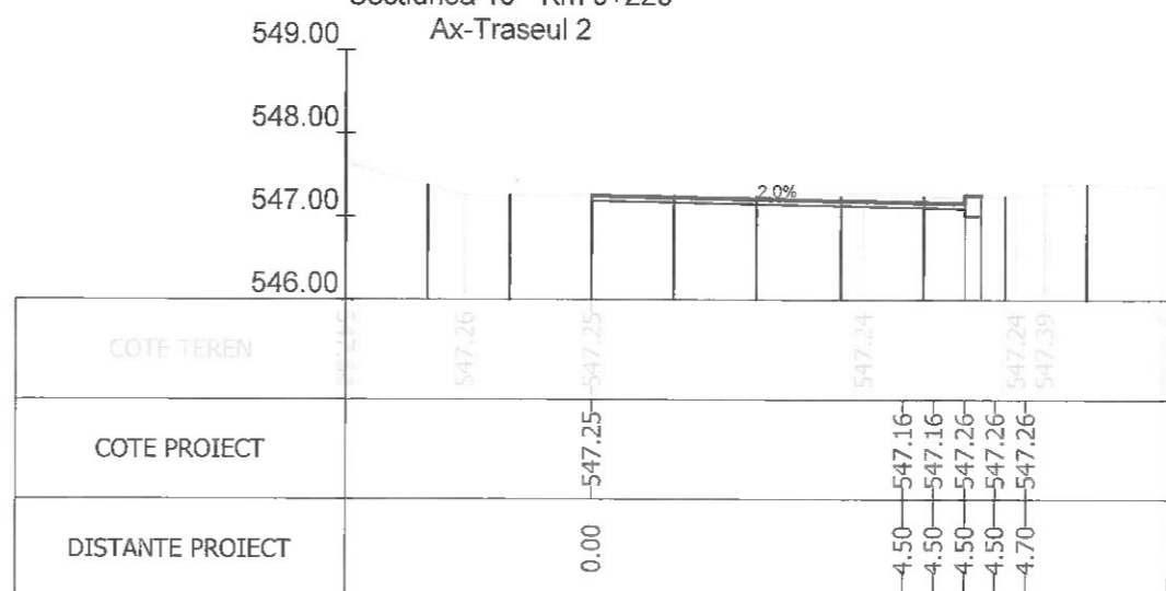
Sectiunea 20 - Km 0+250 Ax-Traseul 2
