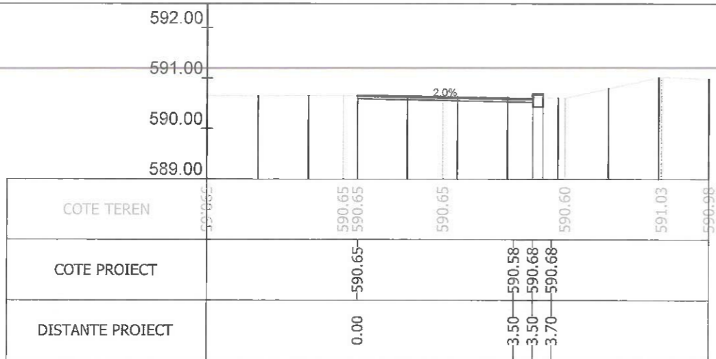
Sectiunea 88 - Km 1+200 Ax-Traseul 1
