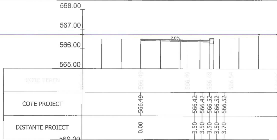
Sectiunea 43 - Km 0+565.515 Ax-Traseul 3_2
