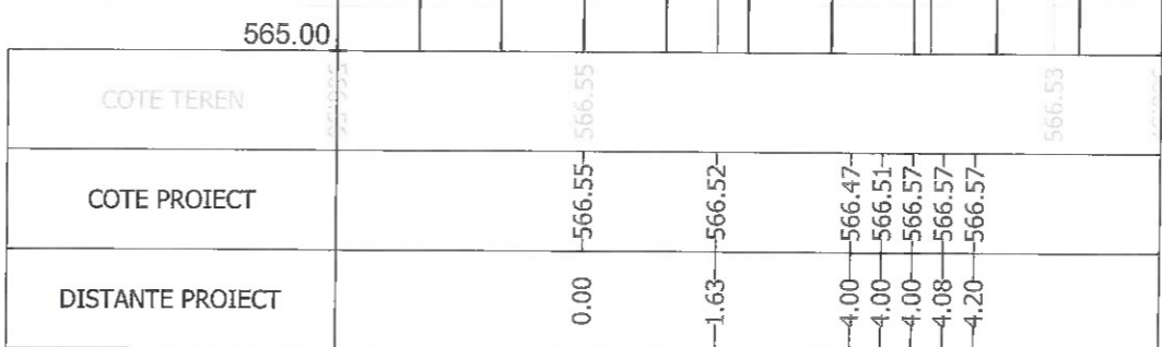
Sectiunea 265 - Km 3+875 Ax-Traseul 2
