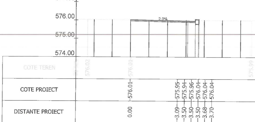
Sectiunea 333 - Km 4+850
