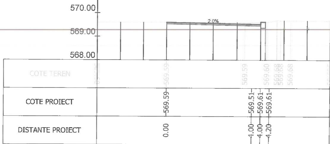
Sectiunea 235 - Km 3+342.806 Ax-Traseul 2
