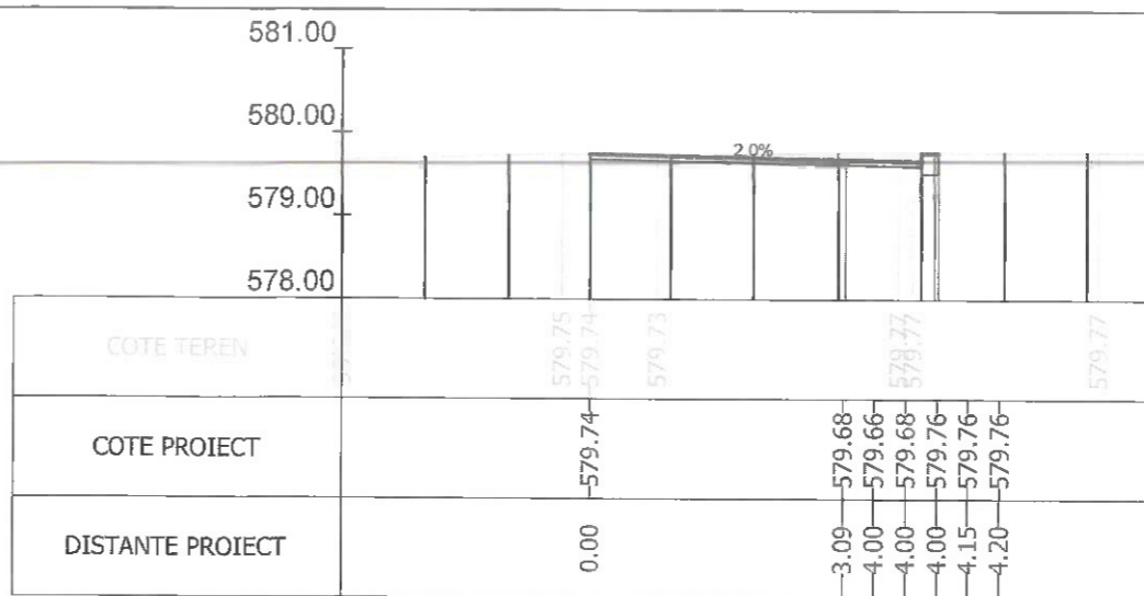
Sectiunea 165 - Km 2+425 Ax-Traseul 2
