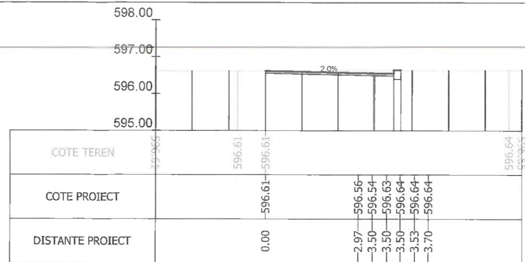
Sectiunea 53 - Km 0+675 Ax-Traseul 1
