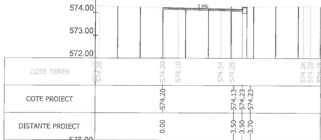
Sectiunea 401 - Km 5+480.669 Ax-Traseul 1
