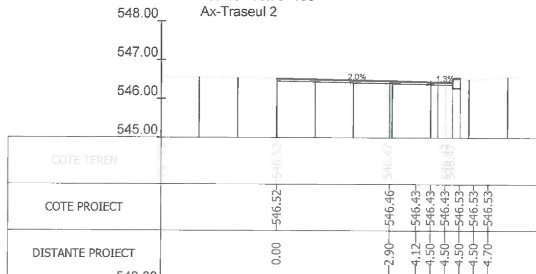
Sectiunea 15 - Km 0+153.971
