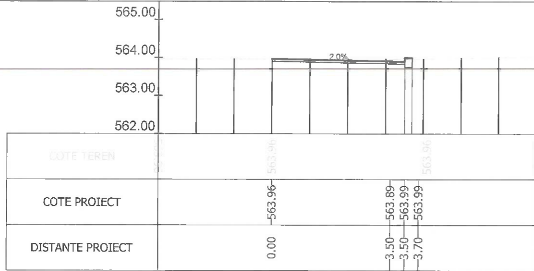
Sectiunea 25 - Km 0+325 Ax-Traseul 3_1
