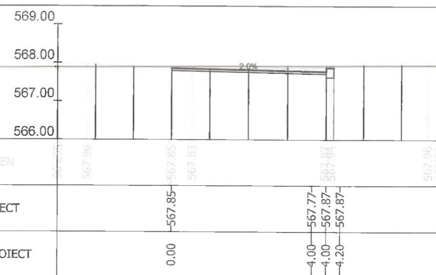
Sectiunea 279 - Km 4+121.505
