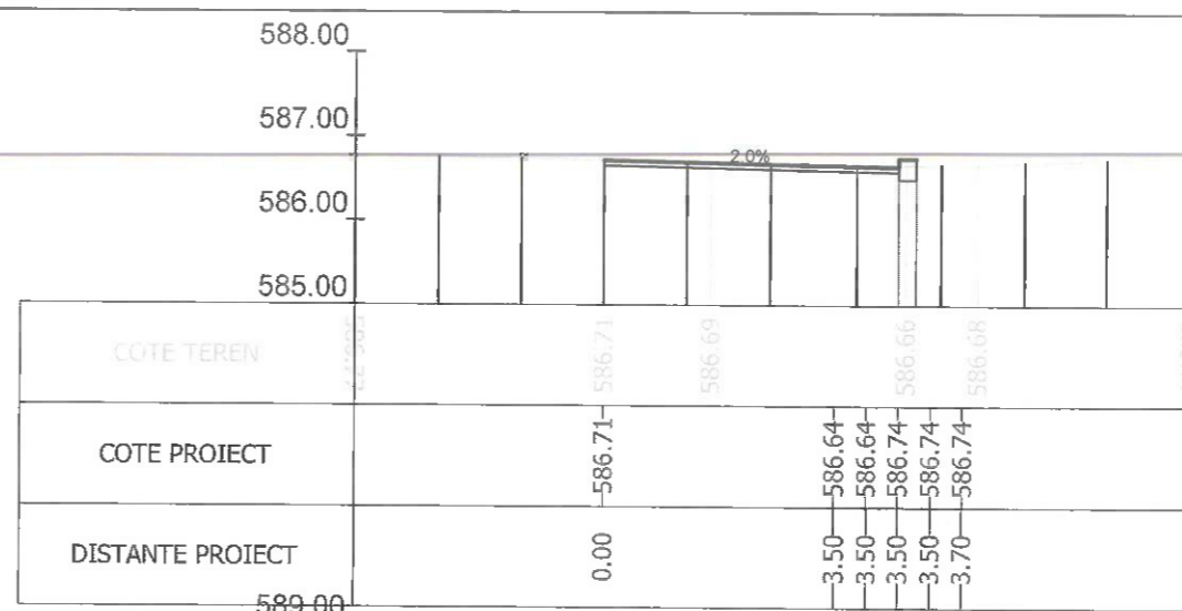
Sectiunea 400 - Km 5+821.197 Ax-Traseul 2
