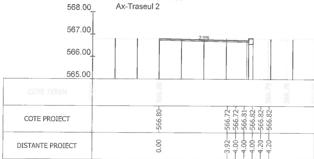
Sectiunea 244 - Km 3+543.804 Ax-Traseul 2
