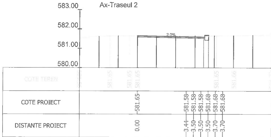
Sectiunea 371 - Km 5+350
