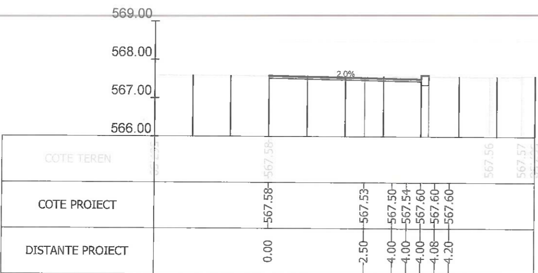
Sectiunea 276 - Km 4+075
