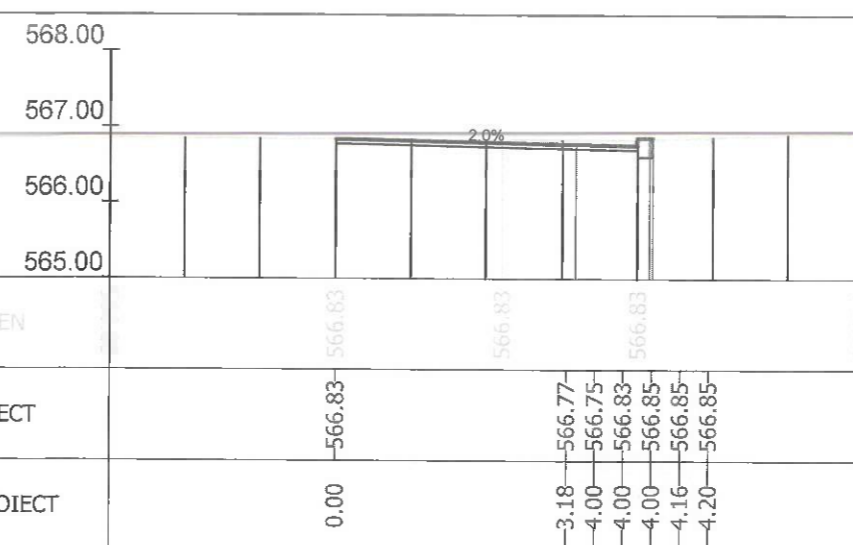
Sectiunea 243 - Km 3+525 Ax-Traseul 2
