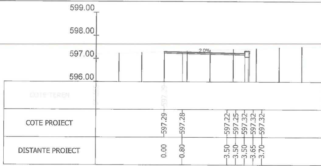
Sectiunea 450 - Km 6+650 Ax-Traseul 2
