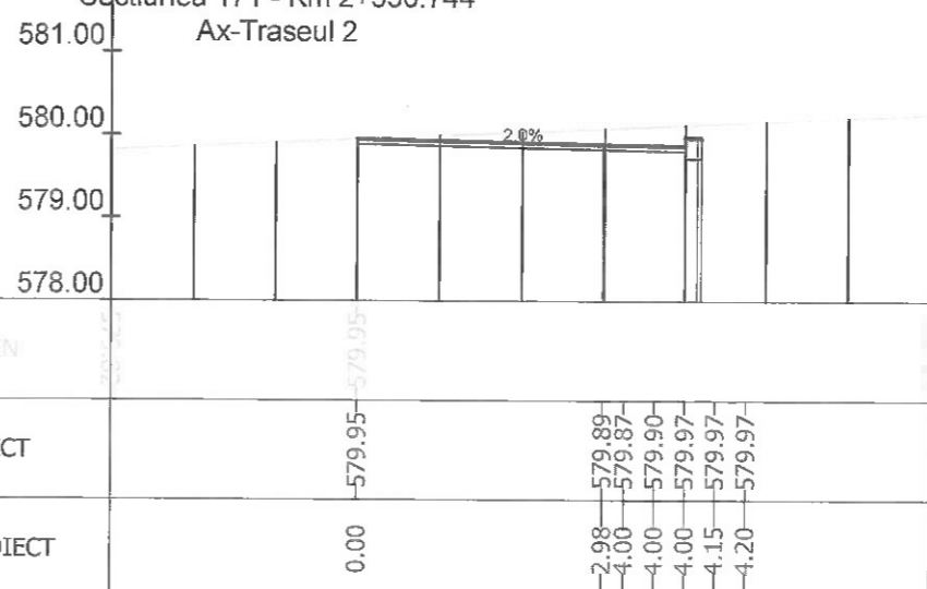
Sectiunea 172 - Km 2+550 Ax-Traseul 2
