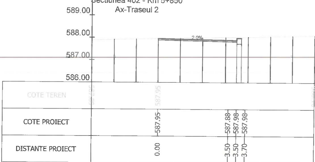
Sectiunea 404 - Km 5+900 Ax-Traseul 2
