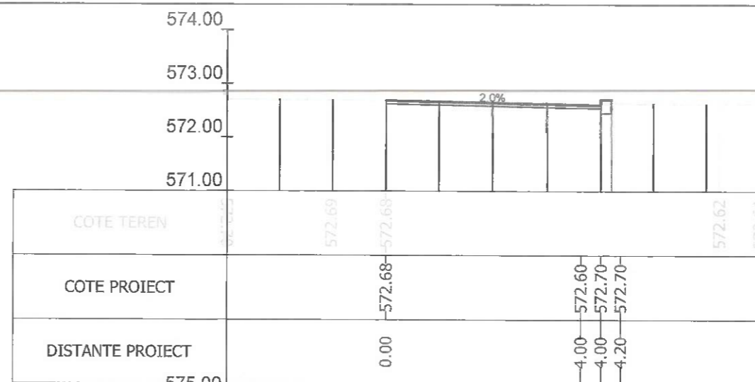
Sectiunea 315 - Km 4+610.652 Ax-Traseul 2
