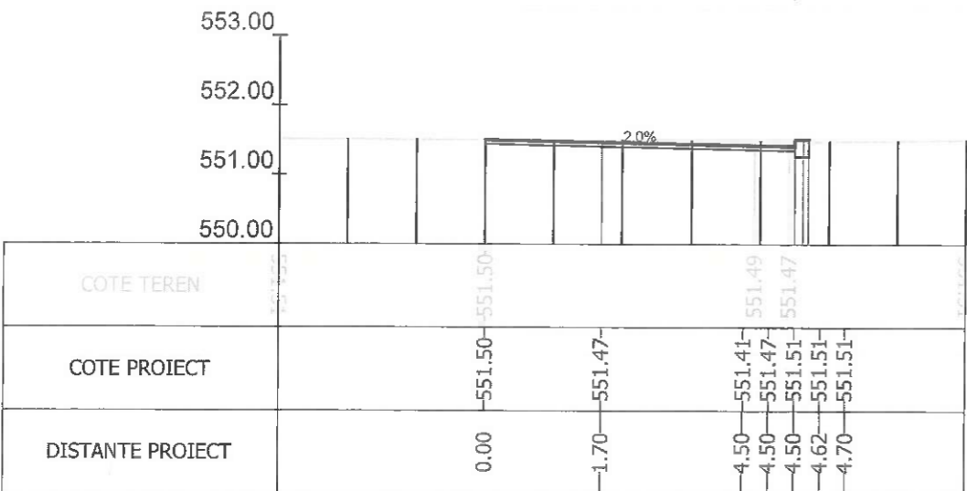
Sectiunea 40 - Km 0+650 Ax-Traseul 2
