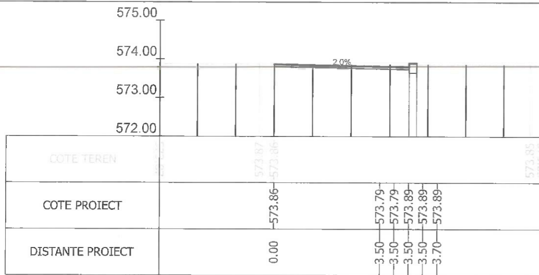
Sectiunea 322 - Km 4+662.054
