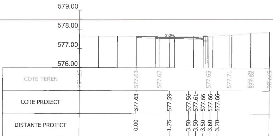
Sectiunea 171 - Km 2+275 Ax-Traseul 1
