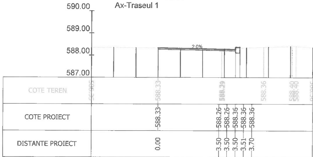
Sectiunea 96 - Km 1+312.640 Ax-Traseul 1
