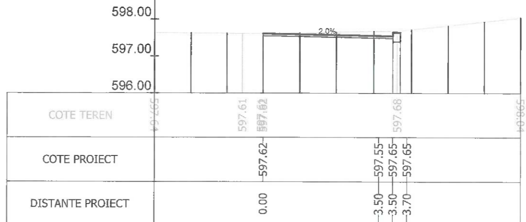
Sectiunea 43 - Km 0+483.601 Ax-Traseul 1
