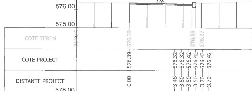
Sectiunea 176 - Km 2+374.997 Ax-Traseul 1
