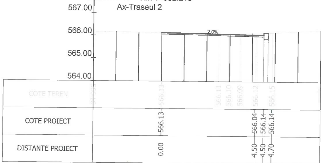
Sectiunea 99 - Km 1+597.045 Ax-Traseul 2
