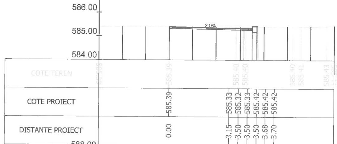
Sectiunea 390 - Km 5+650 Ax-Traseul 2
