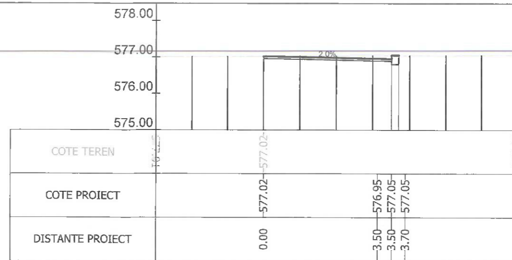
Sectiunea 174 - Km 2+335.246 Ax-Traseul 1
