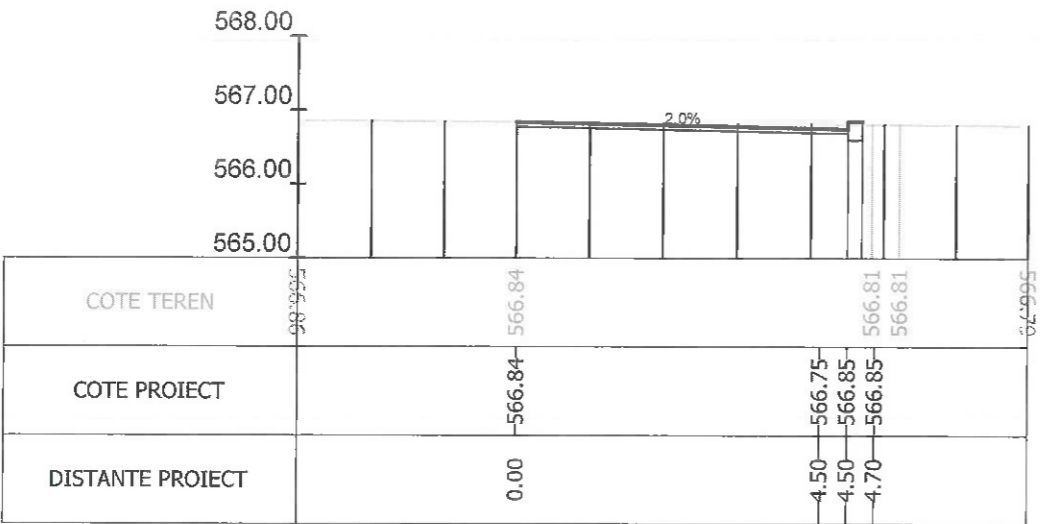
Sectiunea 278 - Km 3+800 Ax-Traseul 1
