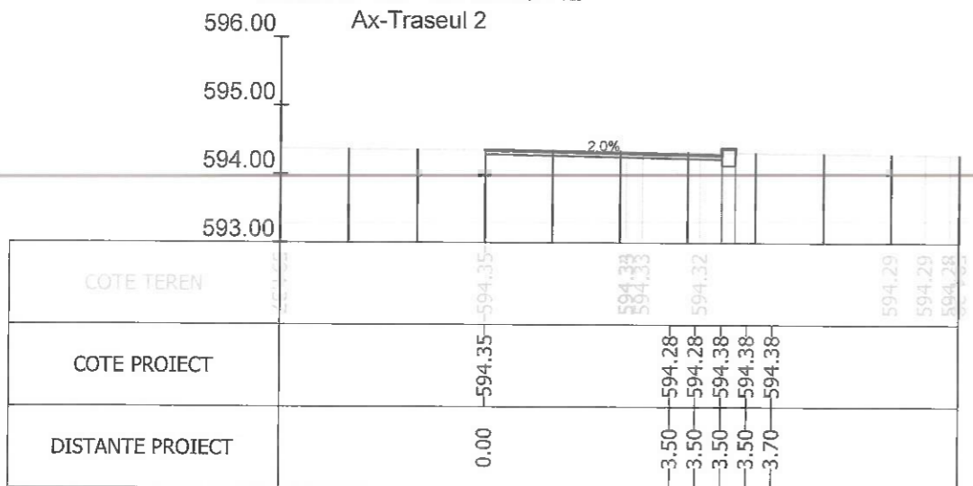
Sectiunea 430 - Km 6+296.849 Ax-Traseul 2
