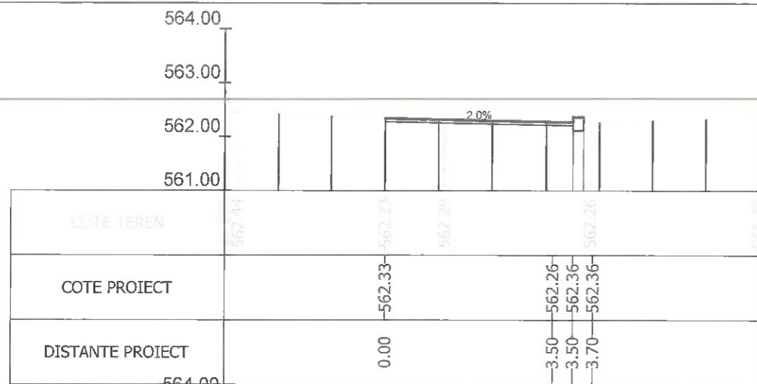
Sectiunea 37 - Km 0+482.969 Ax-Traseul 3_1
