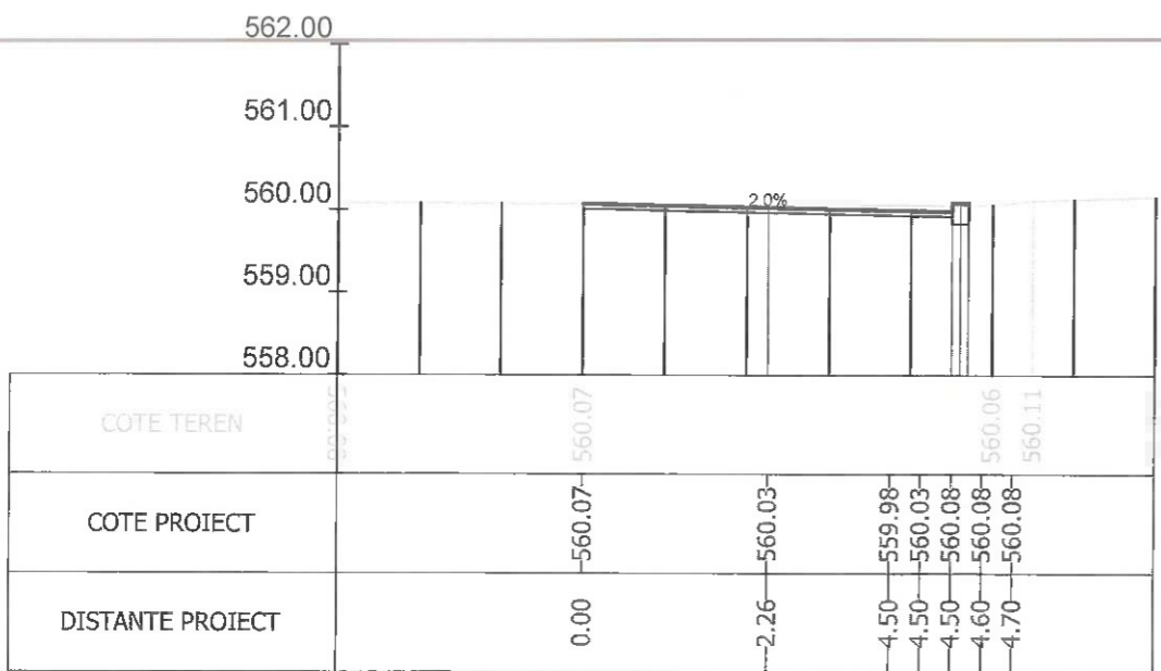
Sectiunea 76 - Km 1+250 Ax-Traseul 2
