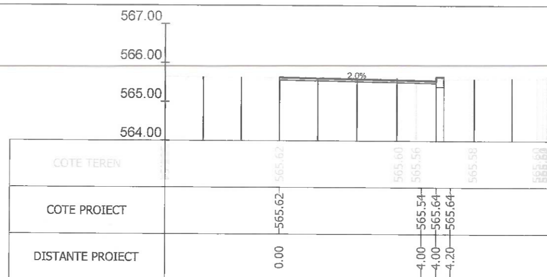
Sectiunea 255 - Km 3+661.970
