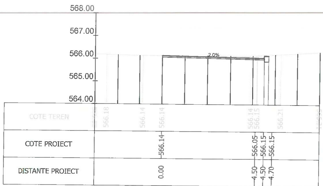
Sectiunea 100 - Km 1+600 Ax-Traseul 2
