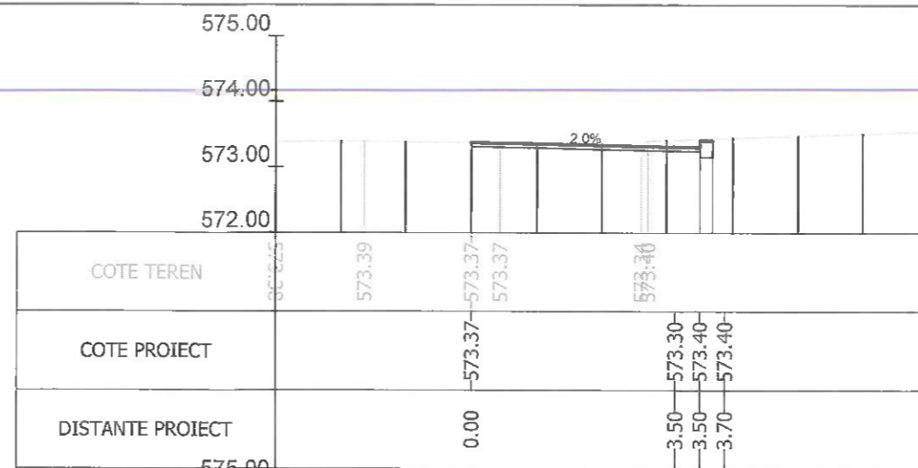
Sectiunea 195 - Km 2+620.246 Ax-Traseul 1
