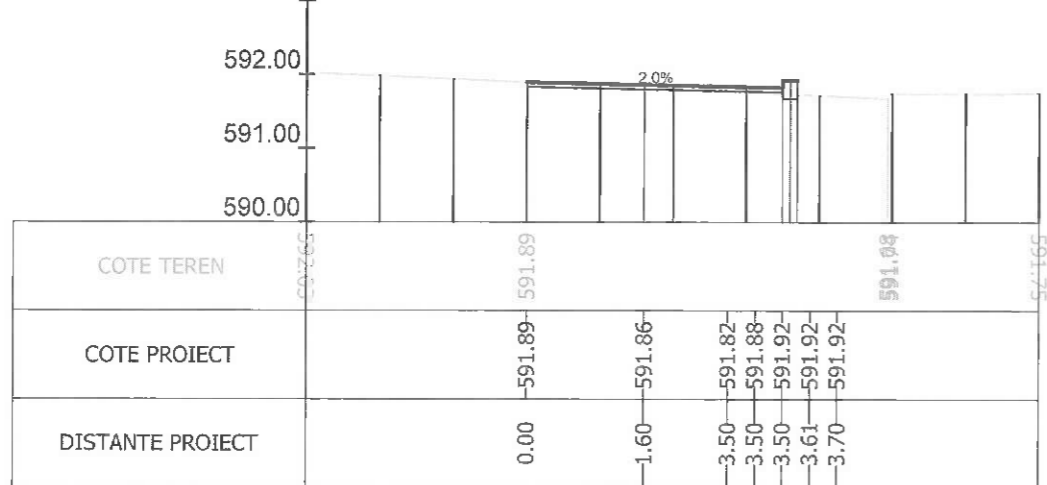
Sectiunea 82 - Km 1+100 Ax-Traseul 1
