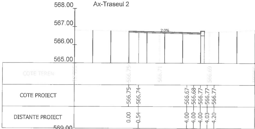
Sectiunea 268 - Km 3+925 Ax-Traseul 2
