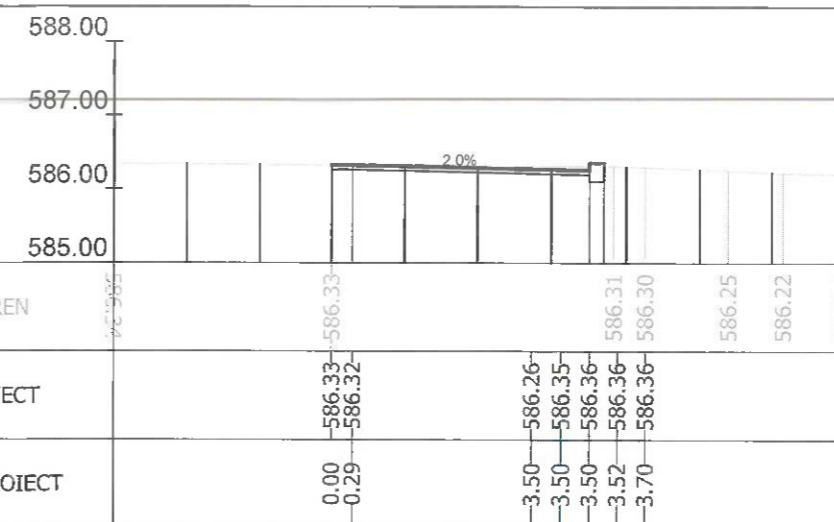
Sectiunea 107 - Km 1+475
