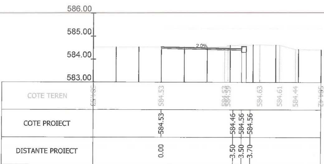
Sectiunea 116 - Km 1+635.090 Ax-Traseul 1
