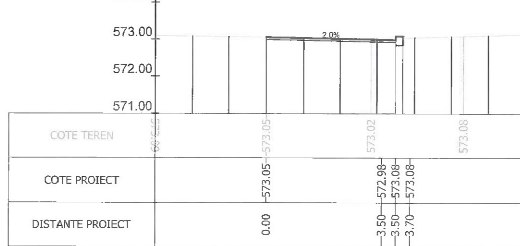
Sectiunea 197 - Km 2+639.600 Ax-Traseul 1
