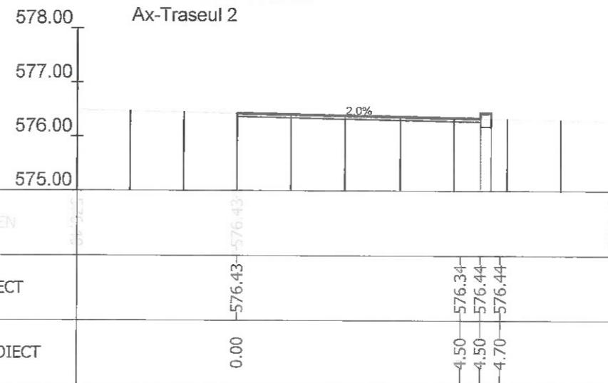
Sectiunea 191 - Km 2+812.996
