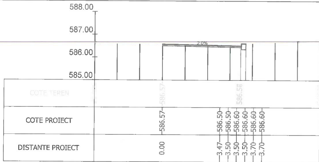
Sectiunea 399 - Km 5+805.792 Ax-Traseul 2
