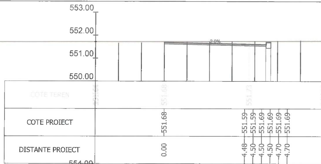
Sectiunea 42 - Km 0+669.469 Ax-Traseul 2
