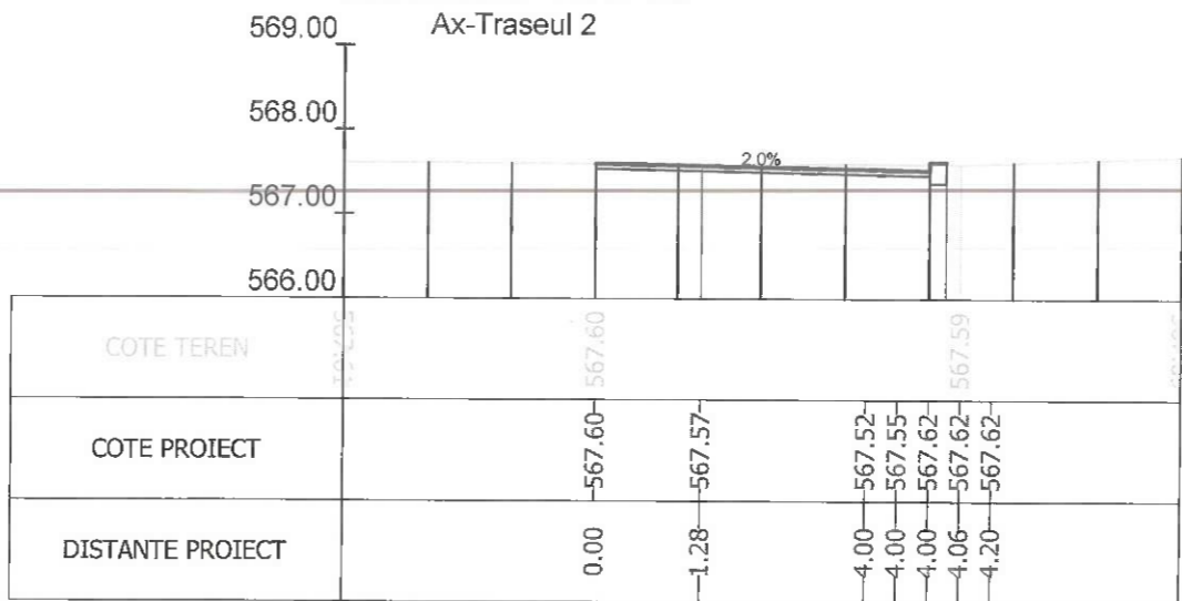
Sectiunea 241 - Km 3+475 Ax-Traseul 2
