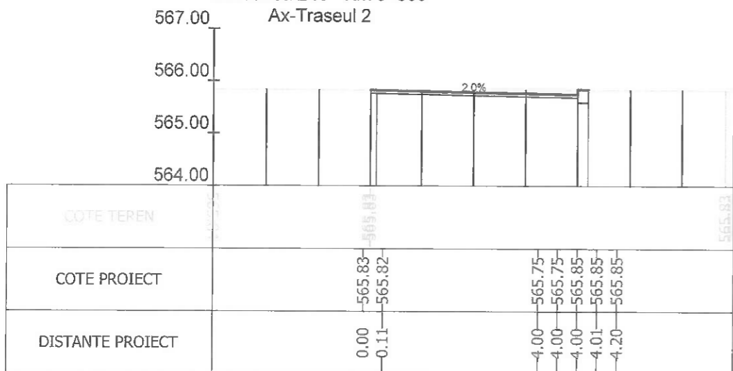
Sectiunea 250 - Km 3+625 Ax-Traseul 2
