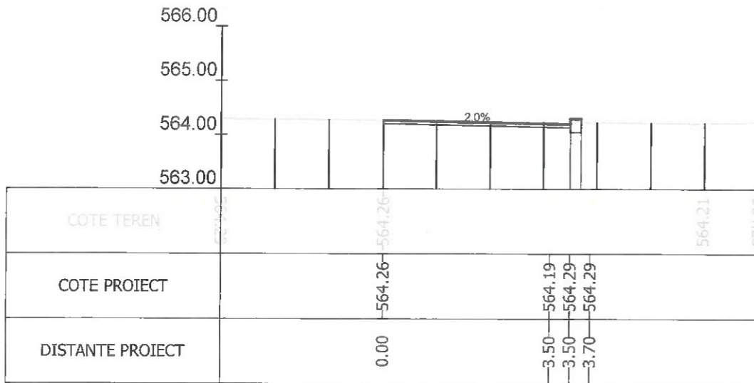
Sectiunea 23 - Km 0+300 Ax-Traseul 3_1
