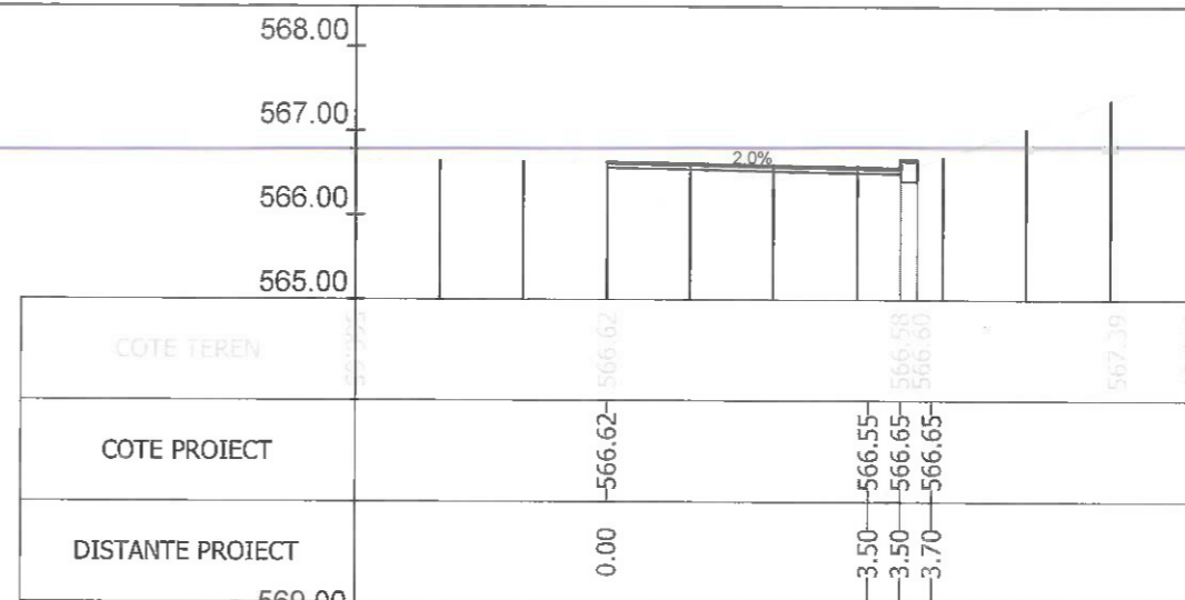
Sectiunea 44 - Km 0+575 Ax-Traseul 3_2
