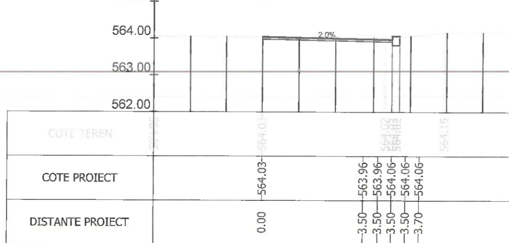
Sectiunea 24 - Km 0+309.342 Ax-Traseul 3_1
