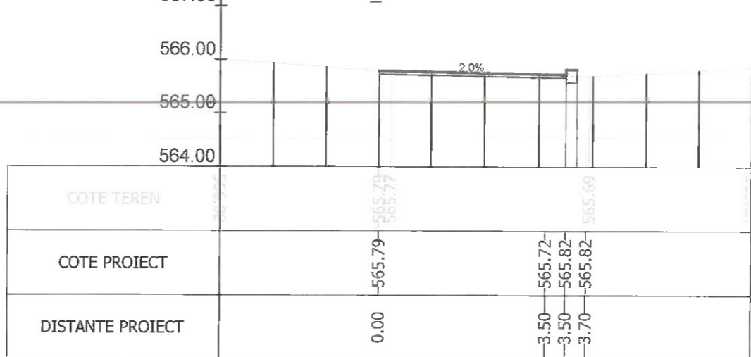
Sectiunea 12 - Km 0+150
