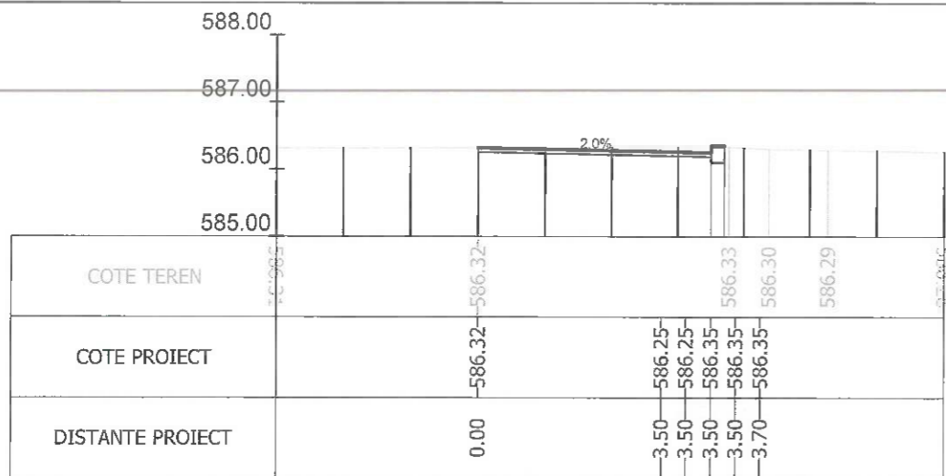
Sectiunea 106 - Km 1+472.530
