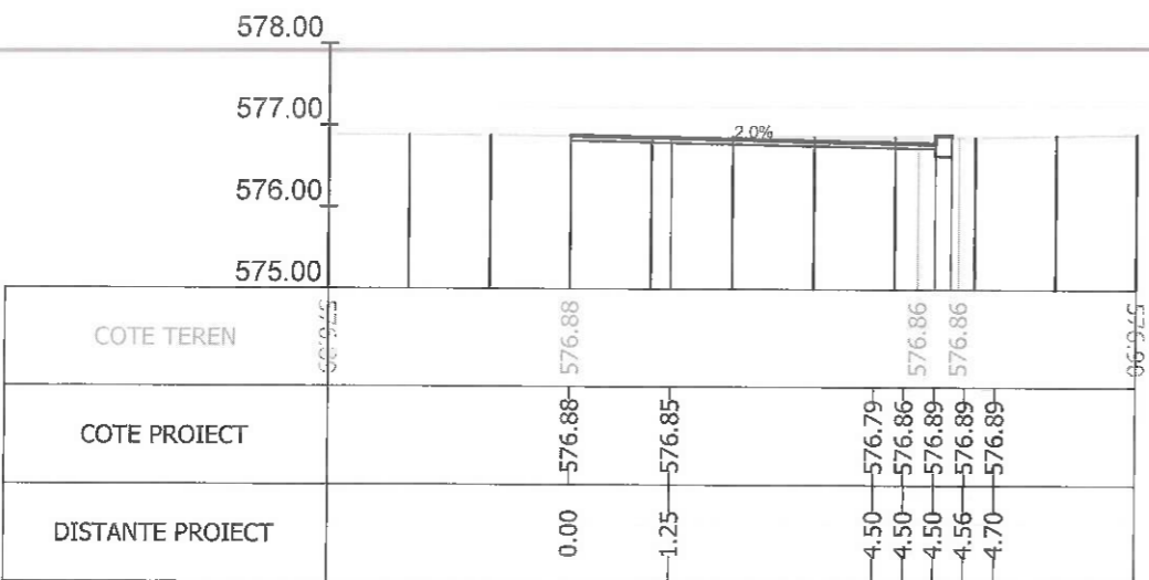
Sectiunea 387 - Km 5+350 Ax-Traseul 1
