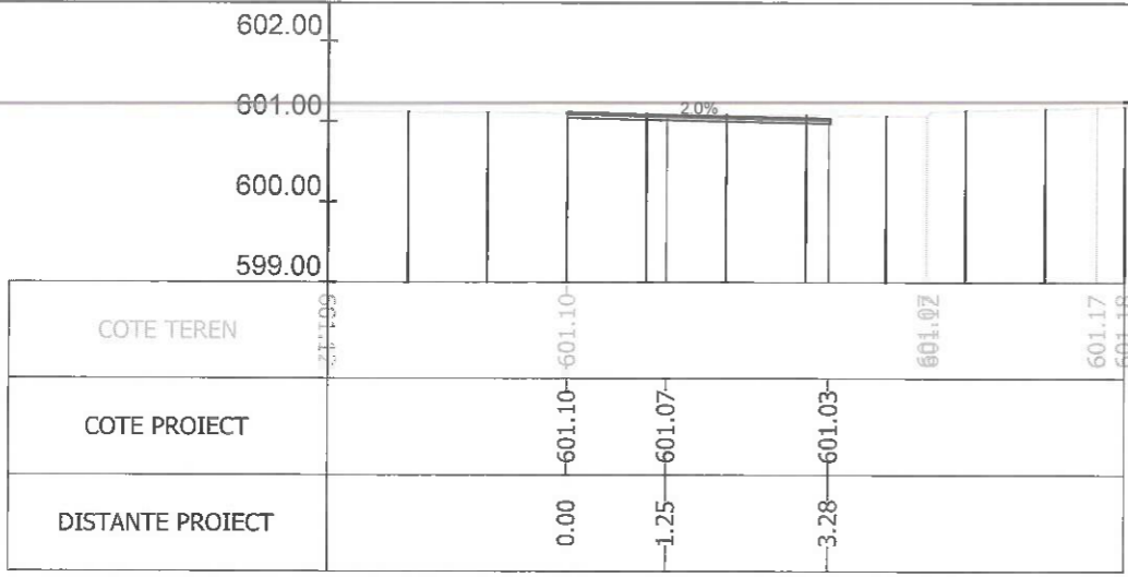
Sectiunea 21 - Km 0+150 Ax-Traseul 1
