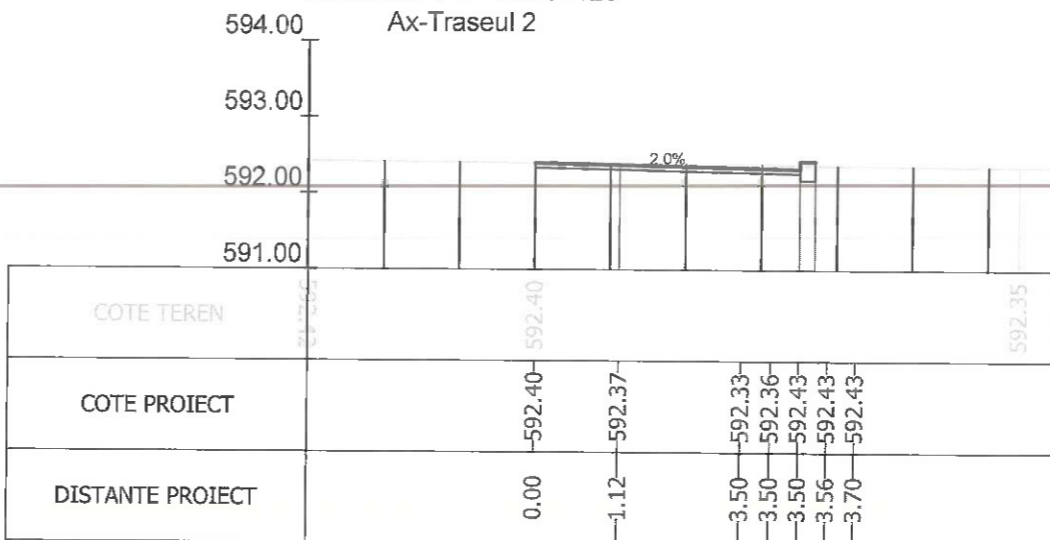
Sectiunea 419 - Km 6+150 Ax-Traseul 2
