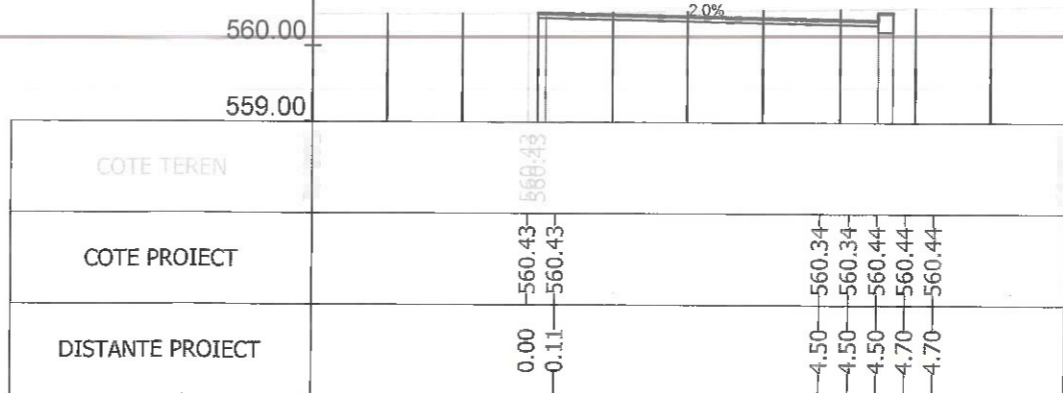
Sectiunea 77 - Km 1+275
