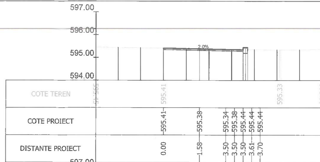
Sectiunea 65 - Km 0+875 Ax-Traseul 1
