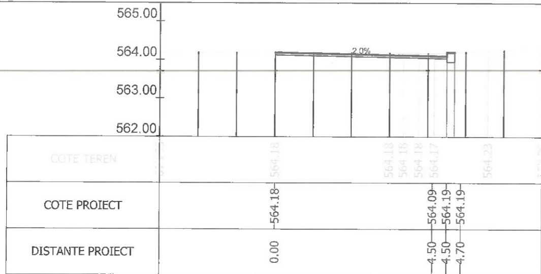
Sectiunea 90 - Km 1+491.116 Ax-Traceul 2
