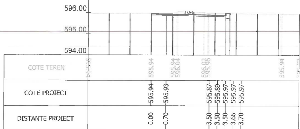
Sectiunea 63 - Km 0+825 Ax-Traseul 1
