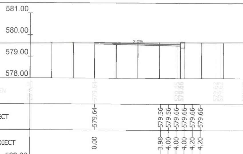
Sectiunea 171 - Km 2+530.744 Ax-Traseul 2
