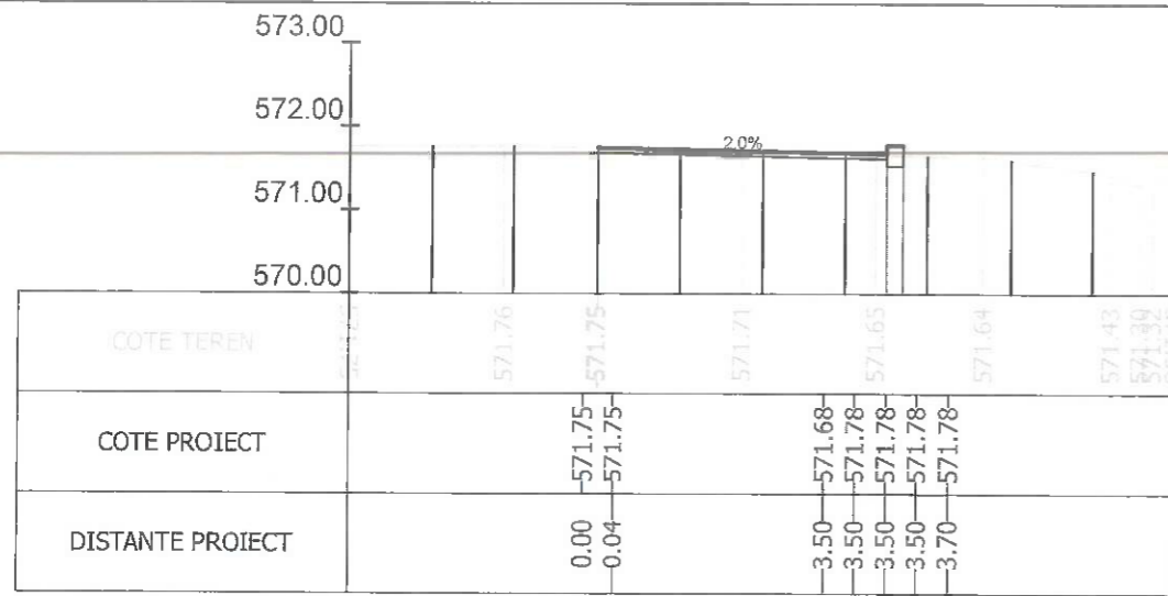
Sectiunea 121 - Km 1+925 Ax-Traseul 2
