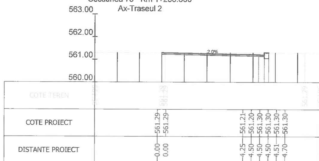
Sectiunea 80 - Km 1+325 Ax-Traseul 2
