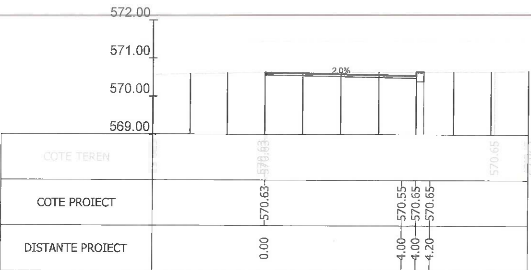
Sectiunea 300 - Km 4+398.395 Ax-Traseul 2
