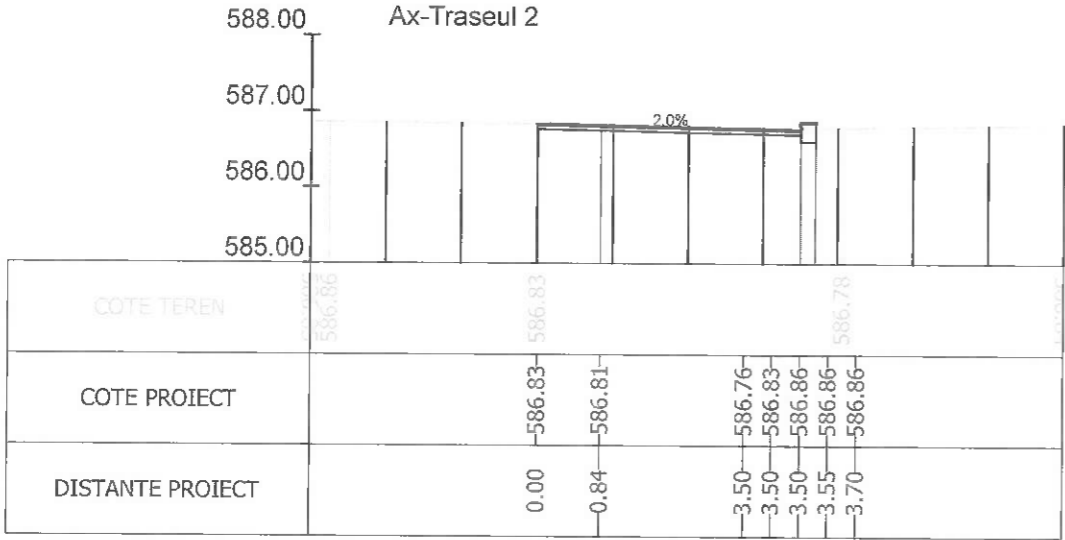
Sectiunea 401 - Km 5+825 Ax-Traseul 2
