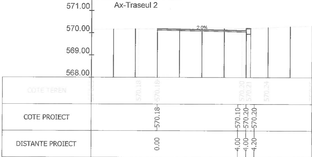
Sectiunea 298 - Km 4+359.832 Ax-Traseul 2
