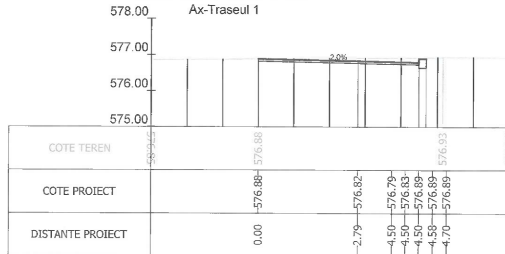
Sectiunea 373 - Km 5+025 Ax-Traseul 1
