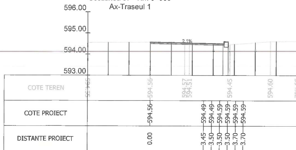
Sectiunea 69 - Km 0+944.692 Ax-Traseul 1
