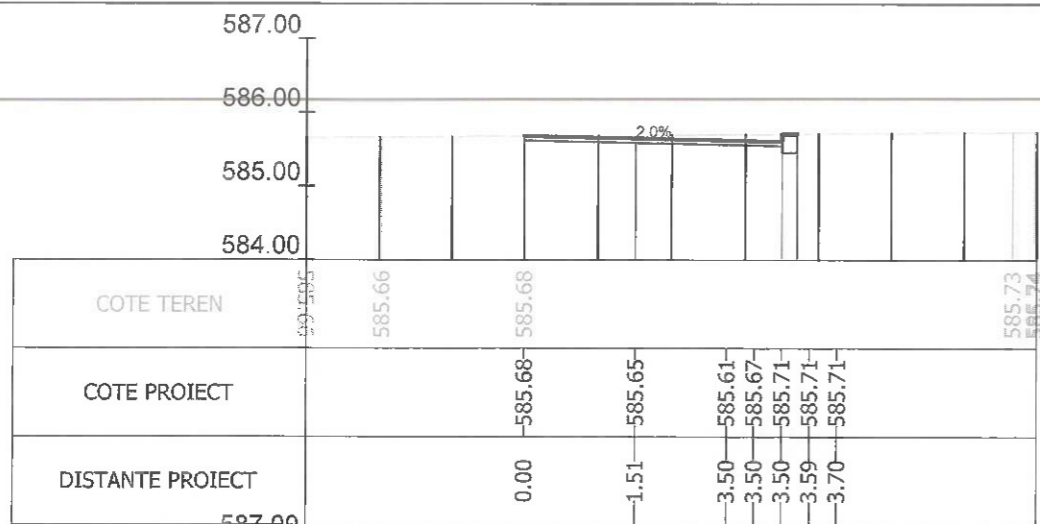
Sectiunea 112 - Km 1+575 Ax-Traseul 1
