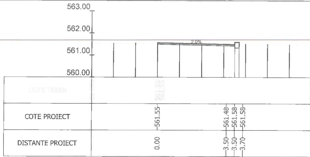
Sectiunea 7 - Km 0+050 Ax-Traseul 3_2
