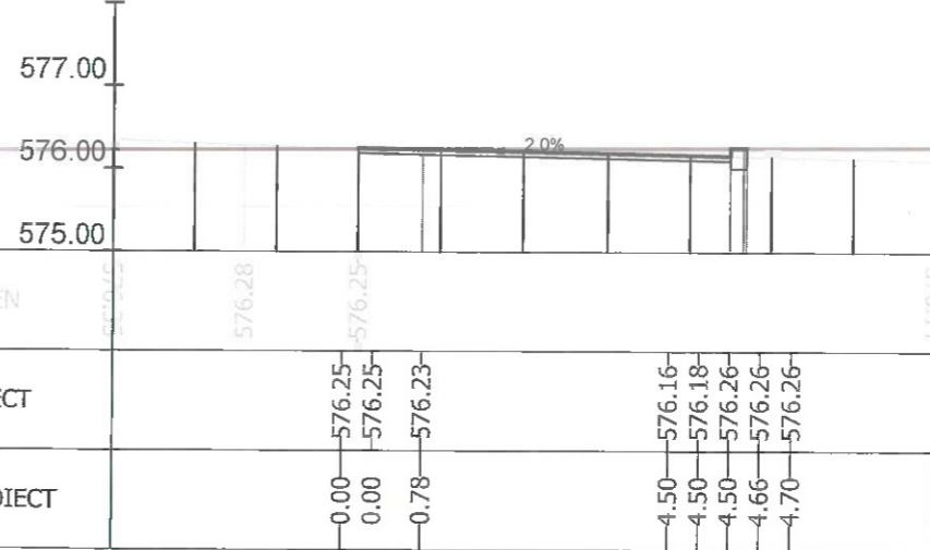
Sectiunea 193 - Km 2+825
