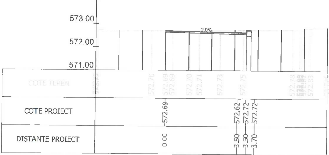
Sectiunea 127 - Km 1+975 Ax-Traseul 2
