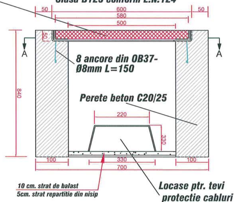
VEDERE B-B Rama si capac canalizare necarosabil 600x600 -capac fonta. Clasa B125 conform E.N.124
