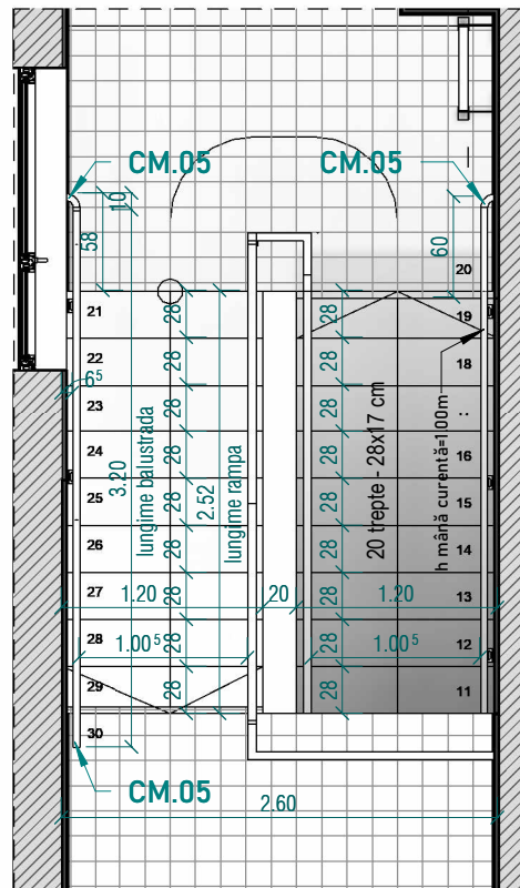
VEDERE PLAN
