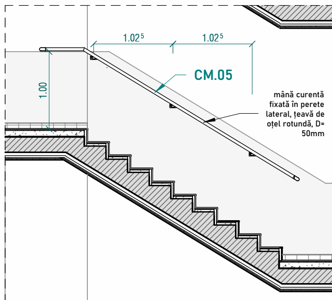
SECȚIUNE
