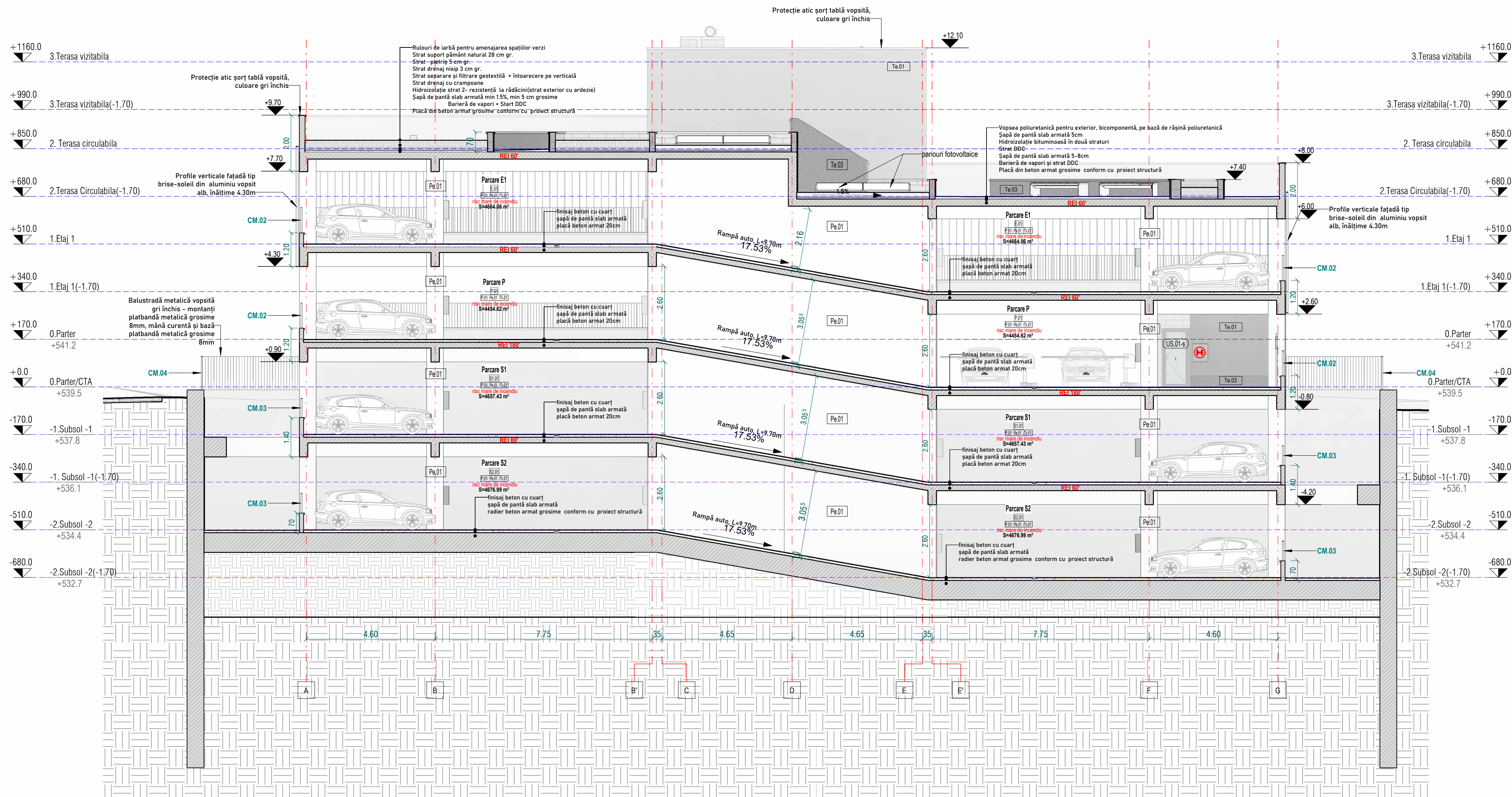
1 Secțiune transversală 03 1 : 100
