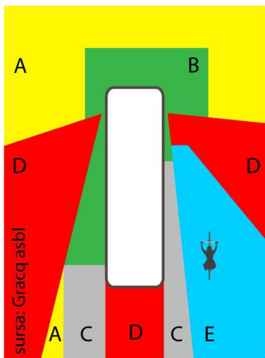
Figura 37. Evidențierea unghiurilor cu vizibilitate redusă, vizibilitate distorsionată și fără vizibilitate în cazul conducătorilor de autobuze sau vehicule de mare tonaj
