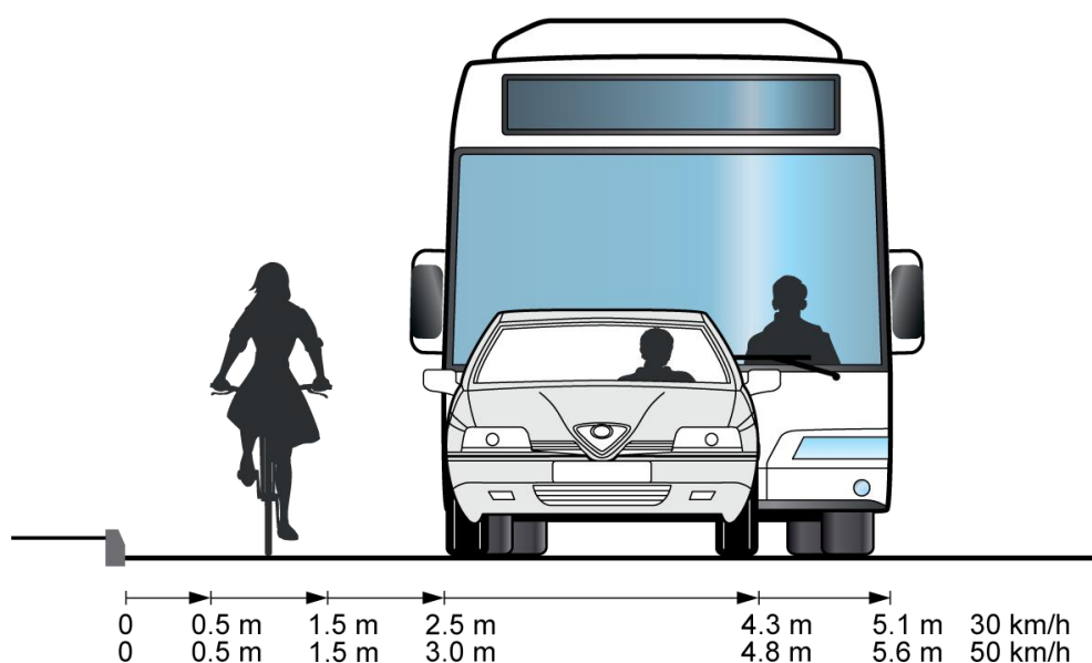
Figura 2. Distanța laterală recomandată în traficul general
