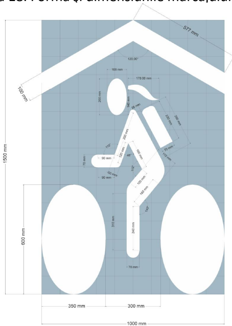
Figura 18. Forma și dimensiunile marcăului traseul
