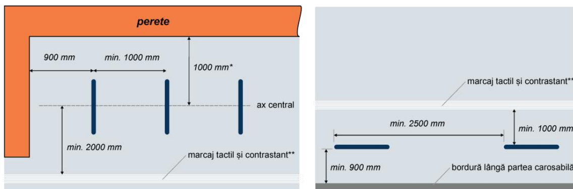
Figura 88. Exemple de amplasare a rastelelor lângă o clădire sau lângă bordura ce delimitează trotuarul de partea carosabilă
