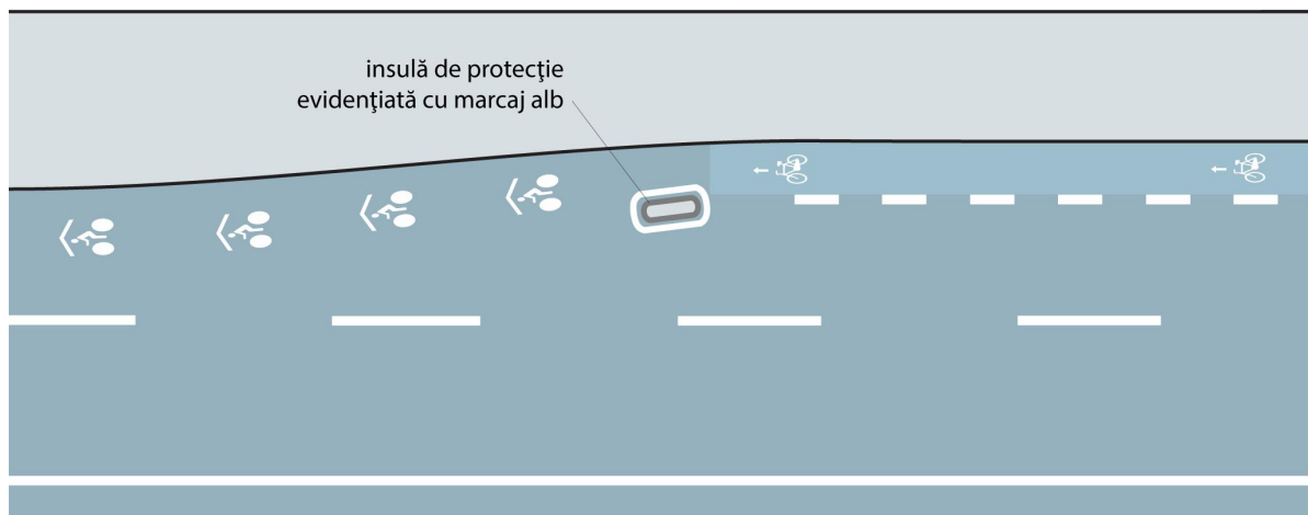
Figura 65. Exemplu de utilizare a insulei de protecție pentru a determina conducătorii auto să protejeze bicicliștii în situațiile în care drumul se îngustează.
