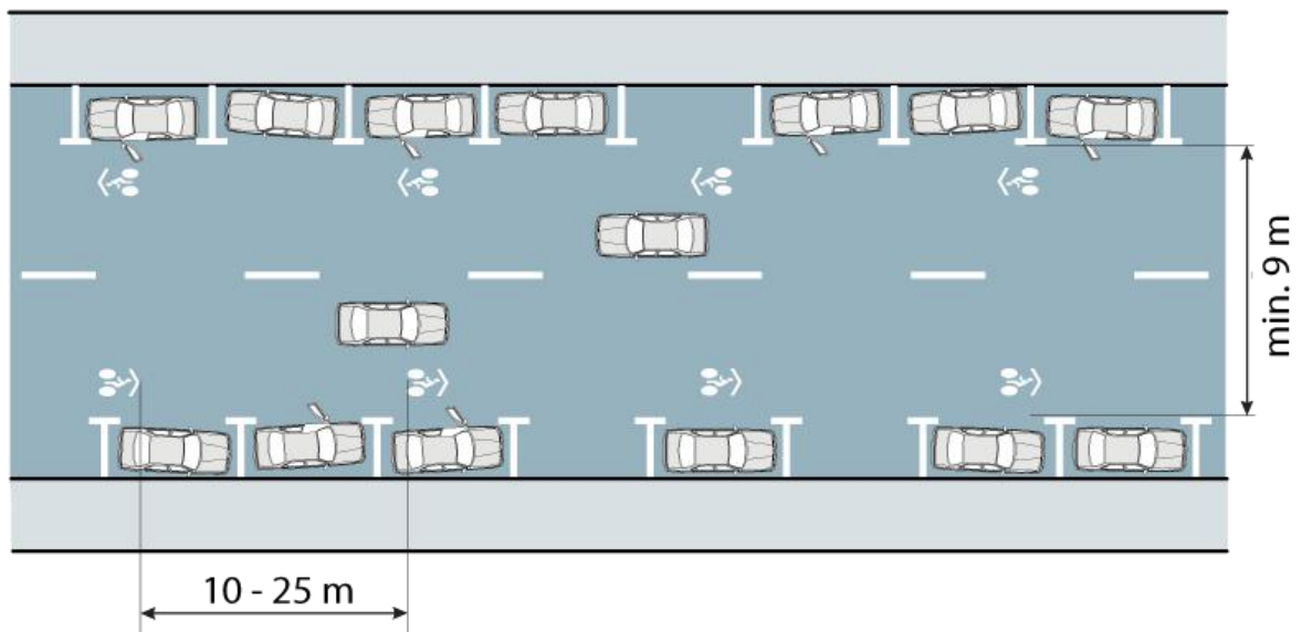
Figura 27. Amplasare laterală a marcajului pentru traseul sugerat pentru biciclete, cu rol de ghidare, pentru benzi de circulație mai late de 4,5 m (lângă parcări laterale)
