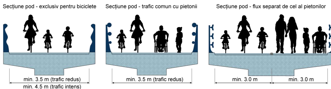
Figura 47. Secțiune poduri
