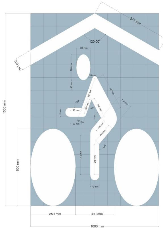
Figura 18. Forma și dimensiunile marcăului traseul
