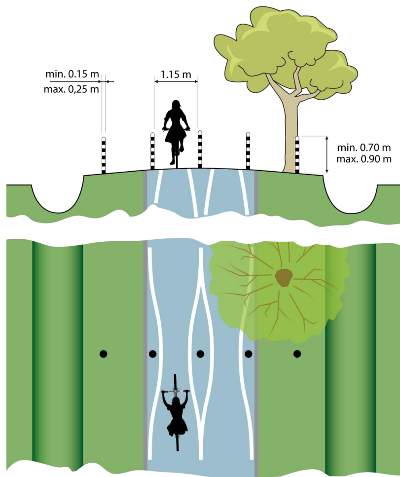
Figura 82. Exemplu de blocare a accesului autovehiculelor și căruțelor pe traseele interurbane, cu rigole și bolarzi
