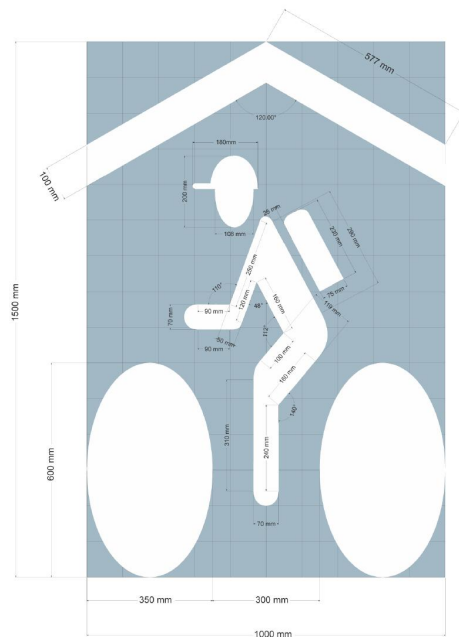
Figura 20 - Forma și dimensiunile marcăului pentru traseul sugerat pentru biciclete – băiat
