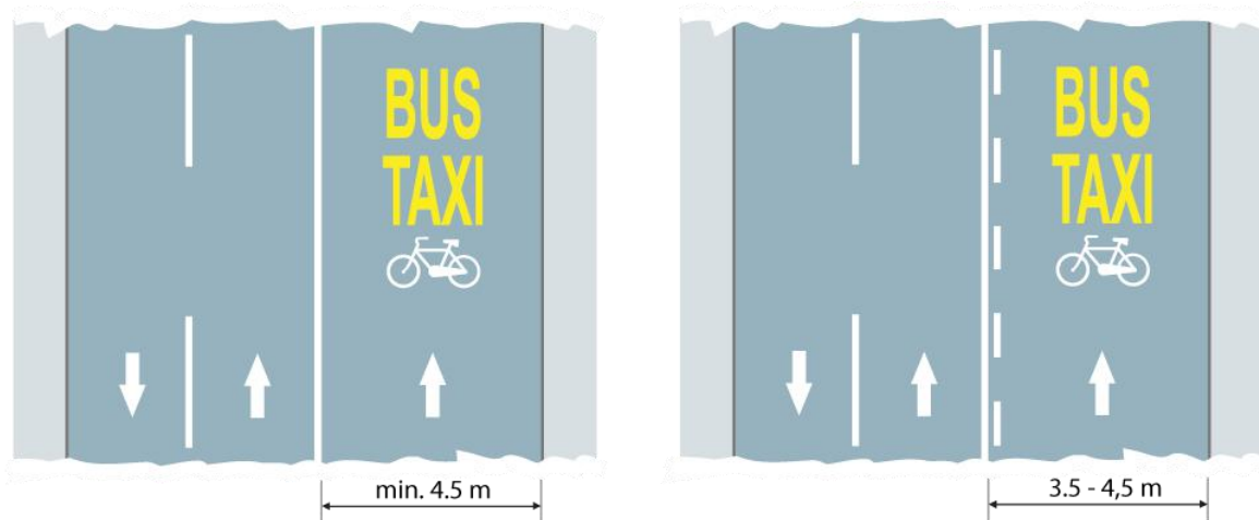
Figura 36. Exemple de marcaje de delimitare a benzilor rezervate bicicletelor și transportului public de persoane
