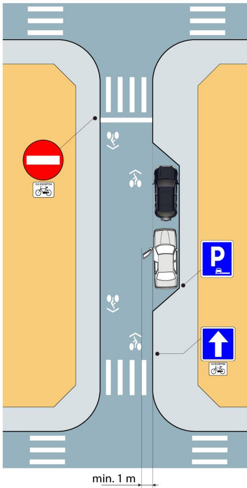
Figura 35. Contrasens deschis bicicletelor cu marcaj "traseu sugerat pentru biciclete" pe ambele sensuri
