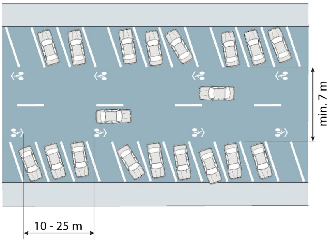
Figura 25. Amplasare laterală a marcajului pentru traseul sugerat pentru biciclete, cu rol de ghidare, pentru benzi de circulație mai late de 3,5 m
