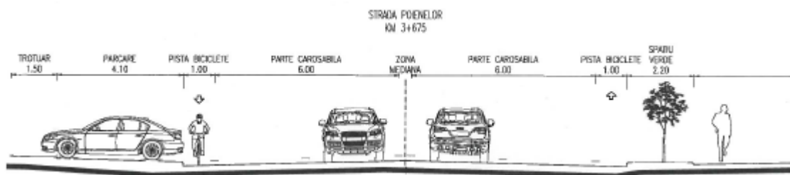
Fig.27 - Profil transversal str. Poienelor ( cerinta )
