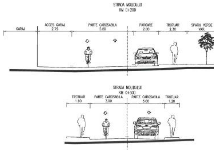
Fig.22 - Profile transversale str. Molidului
