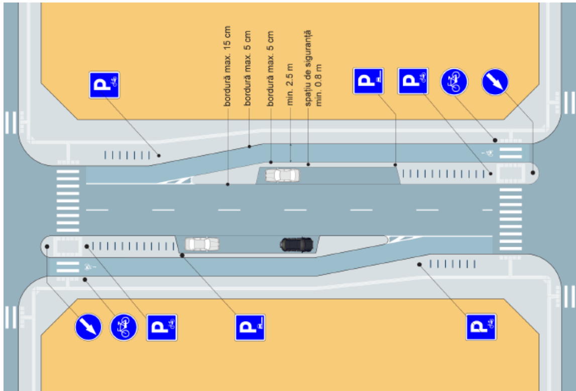
Fig.29 - Exemple de amplasare a rastelelor
