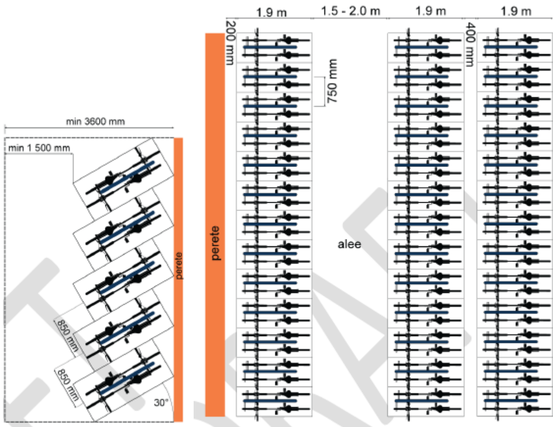
Fig.28 - Model parcare de lunga durata 10-20 locuri ( scoli ) si respectiv peste 20 locuri ( birouri )
