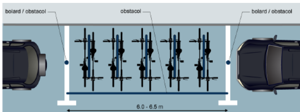
Fig.28 - Model amplasare rastele pe un loc de parcare
