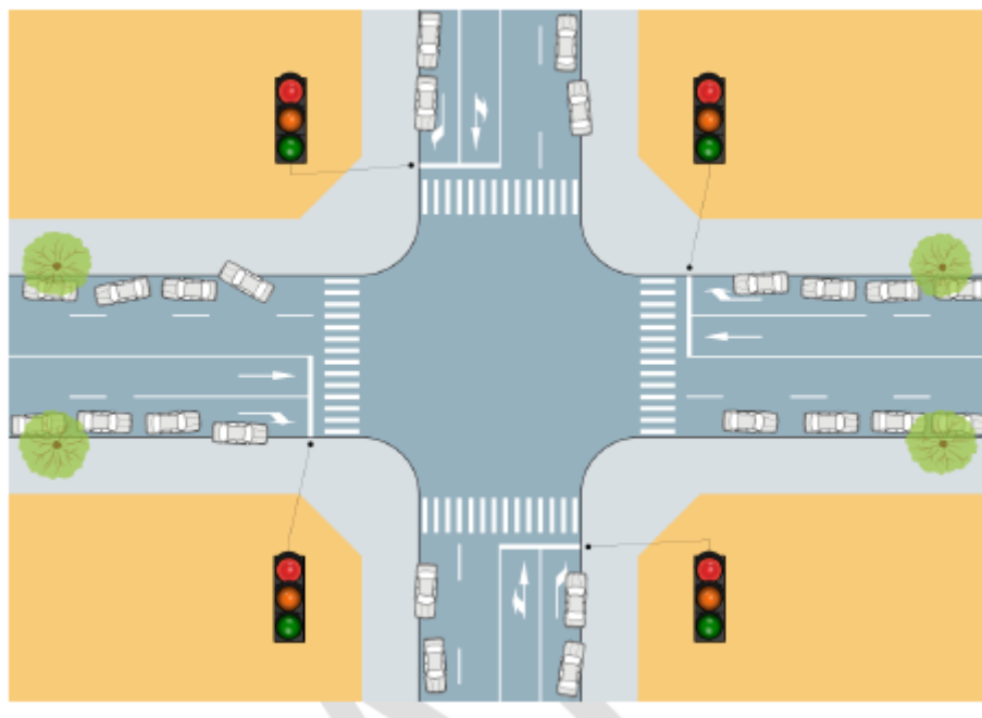
Fig.5- Intersecție tradițională cu grad scăzut de siguranță
