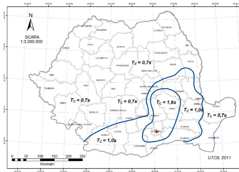
Fig. 4 Zonarea teritoriului României in termeni de perioada de control (colt), T_c a spectrului de răspuns (P100-1/2013)
