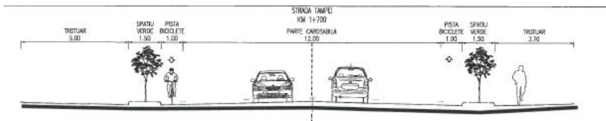
Fig.24 - Profil transversal str. Tampei( cerinta )
