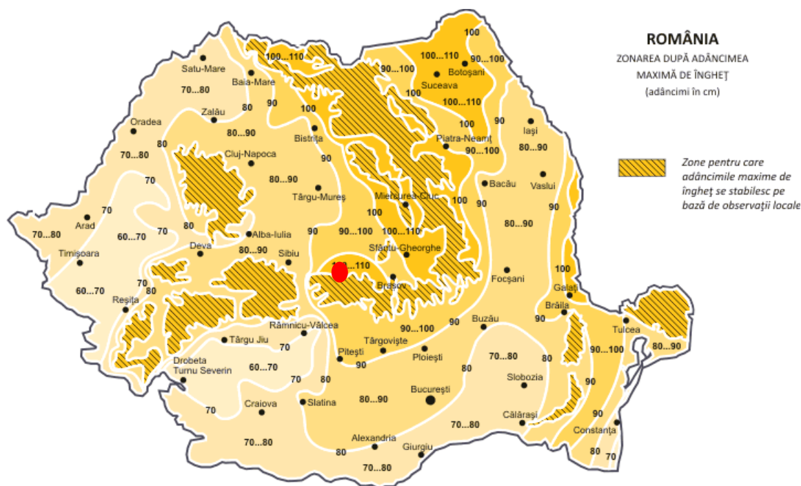
Fig. 1 Adâncimi maxime de îngheț – Zona teritoriului României
