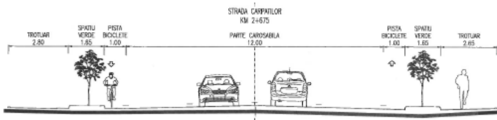
Fig.26 - Profil transversal str. Carpatilor( cerinta )
