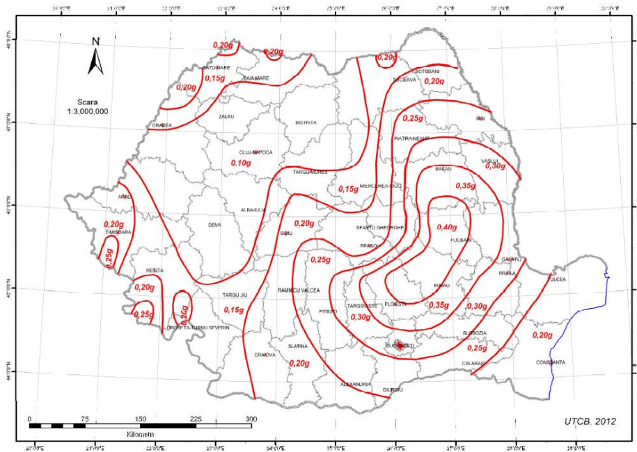
Fig.3 - Zonarea teritoriului României in termeni de valori de vârf ale accelerației terenului pentru proiectare a_g (P100-1/2013).
